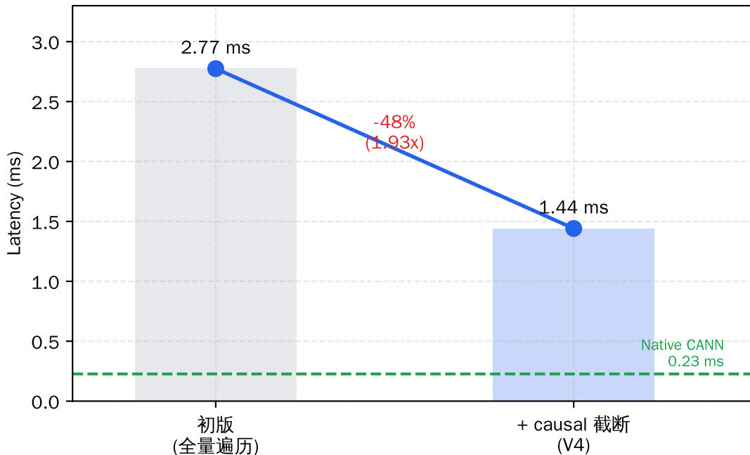
优化历程: 写法粒度贡献分解 (S=2k D=128 H=16 causal)
