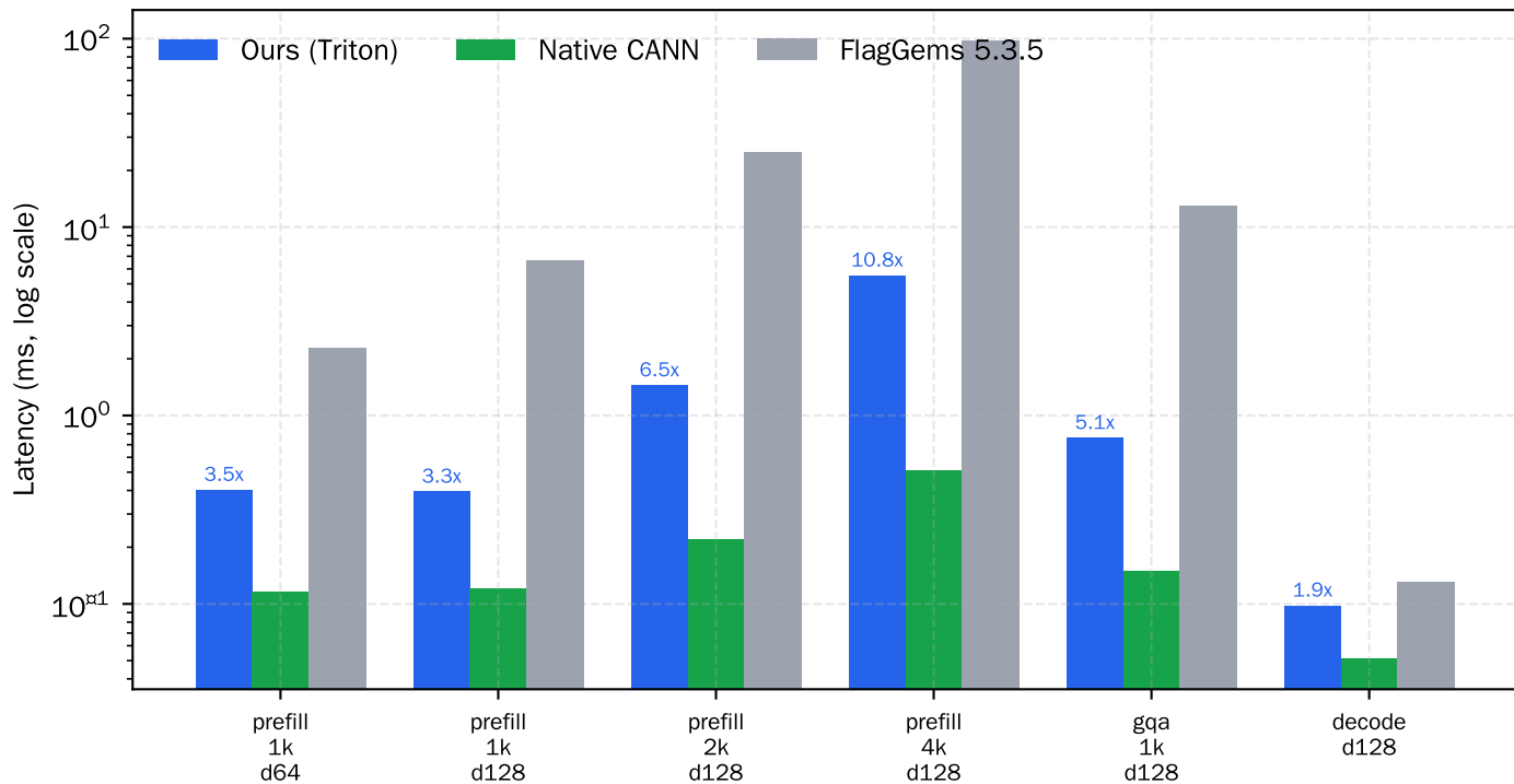
SDPA 三方性能对比 (fp16, causal)
