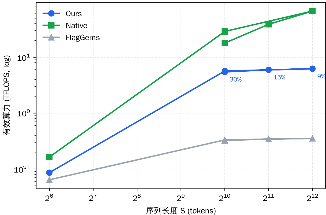
有效算力 vs 序列长度 (D=128, fp16, causal)
