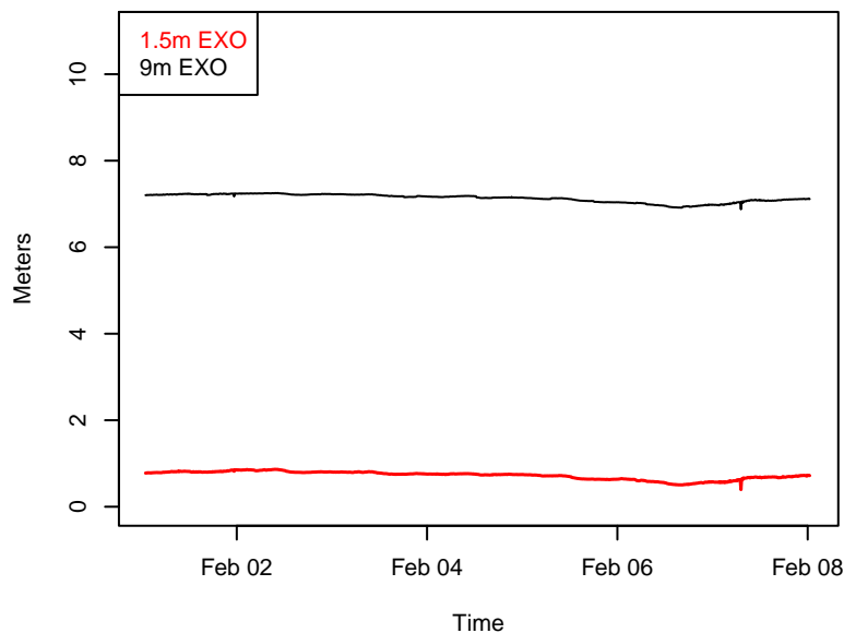
EXO Depth
