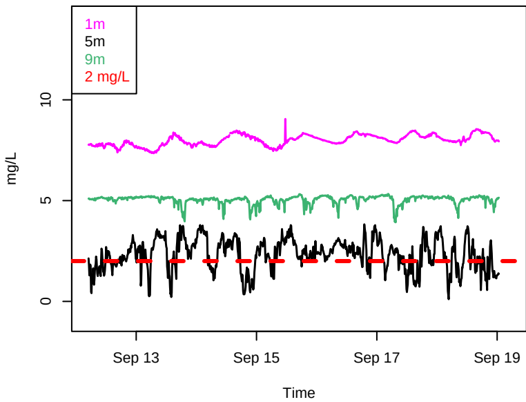
DO
