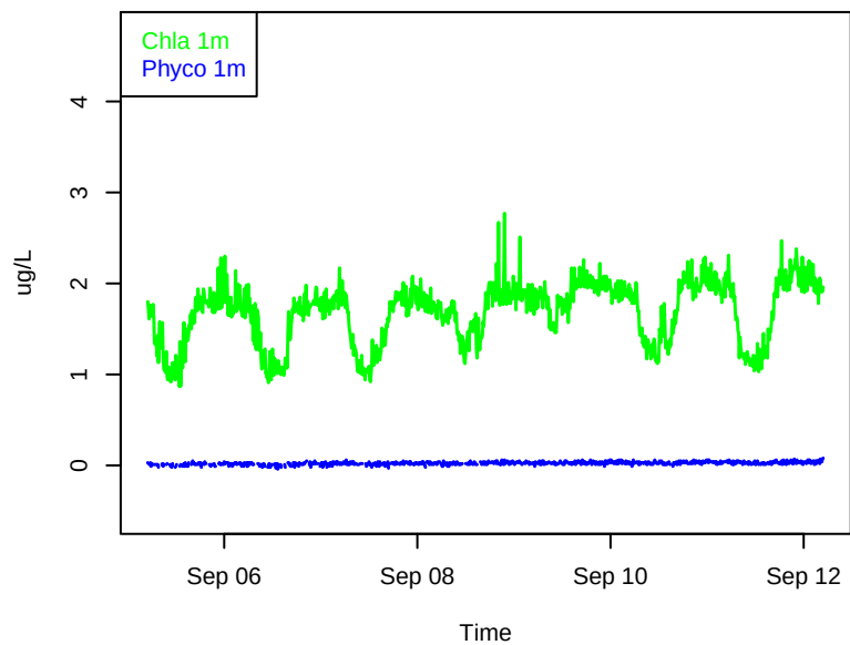
Chla, Phyco @ 1.0m
