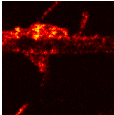
DDIM
