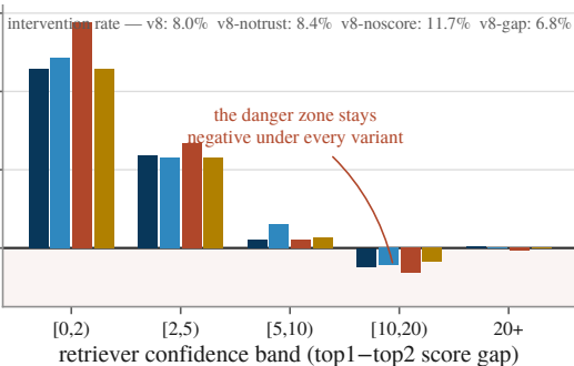
BC5CDR
