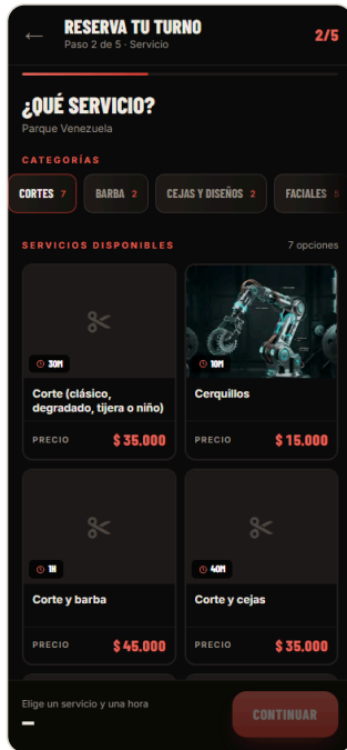
Reservar · servicio · movil
