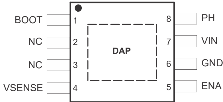
图 4-1. DDA 封装 8 引脚 SOIC (带散热焊盘) 俯视图
