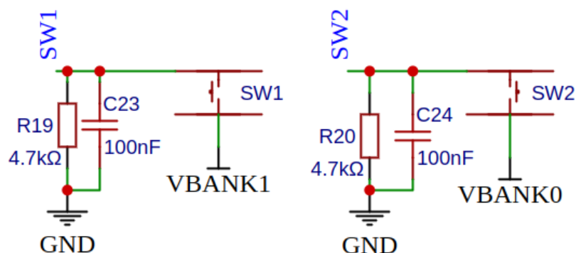
Figura 8: Esquemático de los 2 botones de usuario
