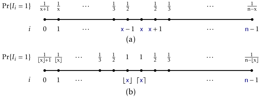
Slika 7.4: Verjetnost, da je element na iskalni poti za x kadar (a) x je celo število in (b) kadar x ni celo število.
