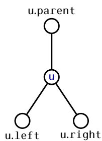
Slika 6.1: Starš, levi otrok, desni otrok vozlišča u v dvojiškem drevesu (BinaryTree).
