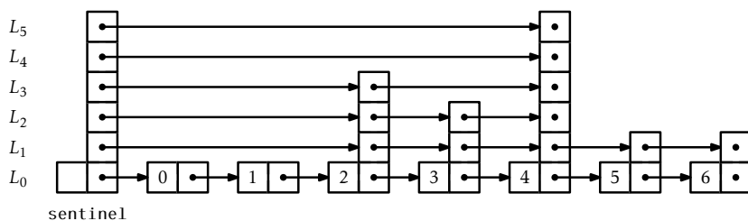
Slika 4.1: Preskočni seznam s sedmimi elementi.
