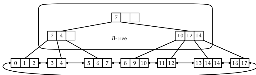
Slika 14.11: B^+ -drevo je B -drevo na vrhu dvojno povezanega seznama blokov.
