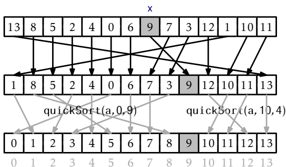
Slika 11.3: Primer izvajanja quickSort(a, 0, 14)
