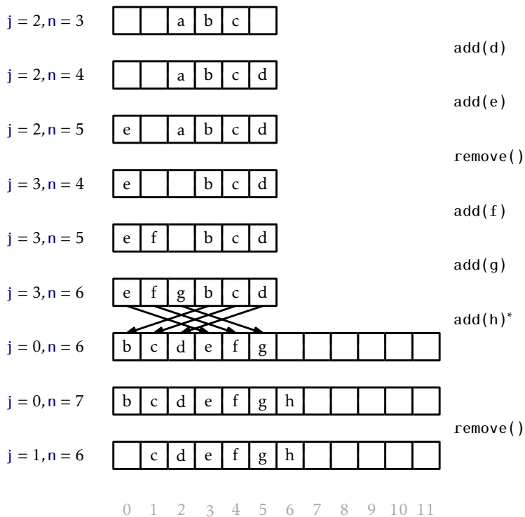
Slika 2.2: Zaporedje operacij \text{add}(x) in \text{remove}(i) nad ArrayQueue . Puščice označujejo kopiranje elementov. Operacije, ki se zaključijo s klicem resize() so označene z zvezdico.
