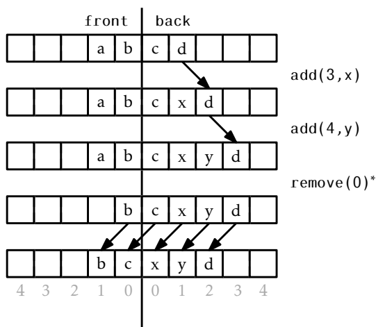
Slika 2.4: Zaporedje operacij \text{add}(i, x) in \text{remove}(i) nad DualArrayDeque . Puščice označujejo prestavljanje elementov. Operacije, po katerih se seznam uravnoteži s klicem balance() , so označene z zvezdico.
