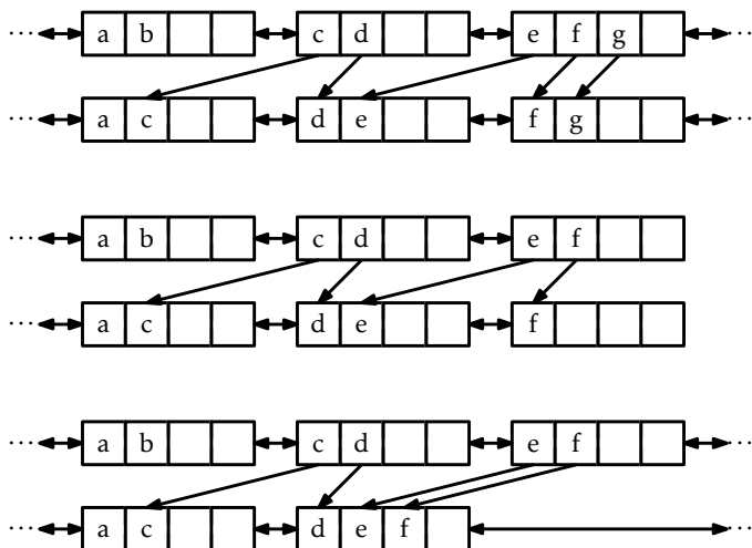
Slika 3.5: Trije scenariji, ki se zgodijo ob odstranjevanju predmeta x znotraj podatkovne strukture SEL list . (Velikost bloka tega SEL lista je b = 3 .)
