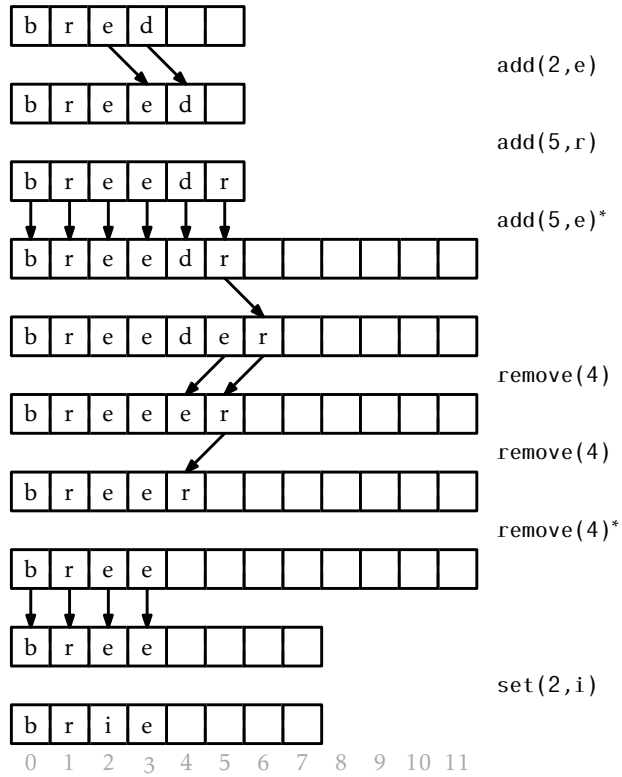
Slika 2.1: Zaporedje operacij \text{add}(i, x) in \text{remove}(i) v ArrayStack . Puščice označujejo elemente, ki jih je potrebno kopirati. Operacije, po katerih moramo klicati metodo resize() so označene z zvezdico.
