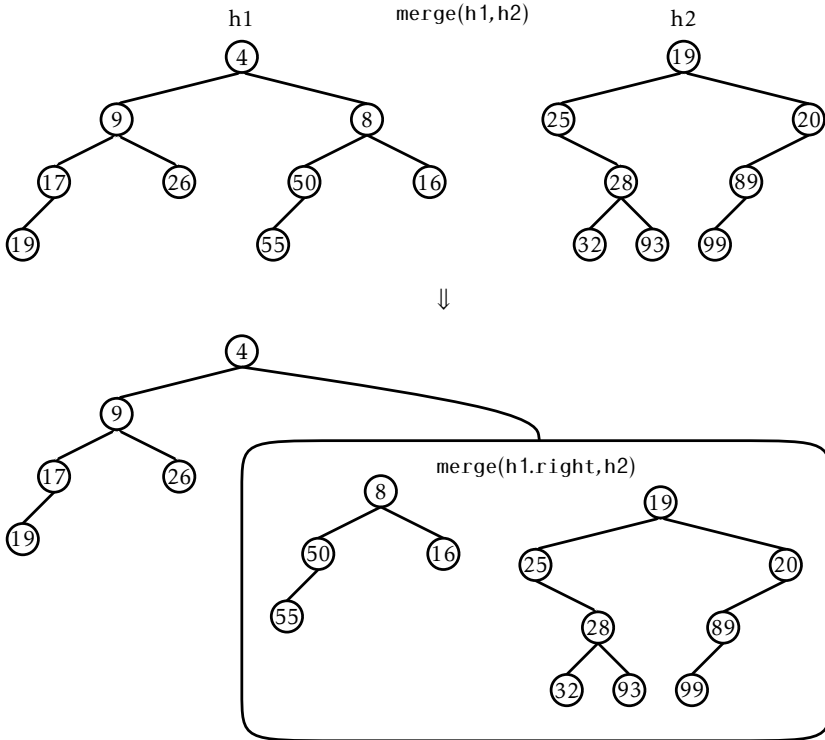
Slika 10.4: Zlivanje h1 in h2 opravimo z združitvijo h2 in h1.left oz. h1.right .
