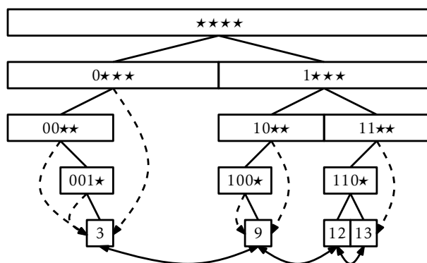
Slika 13.2: BinaryTrie z jump kazalci, prikazanami kot prekinjene ukrivljene povezave.
