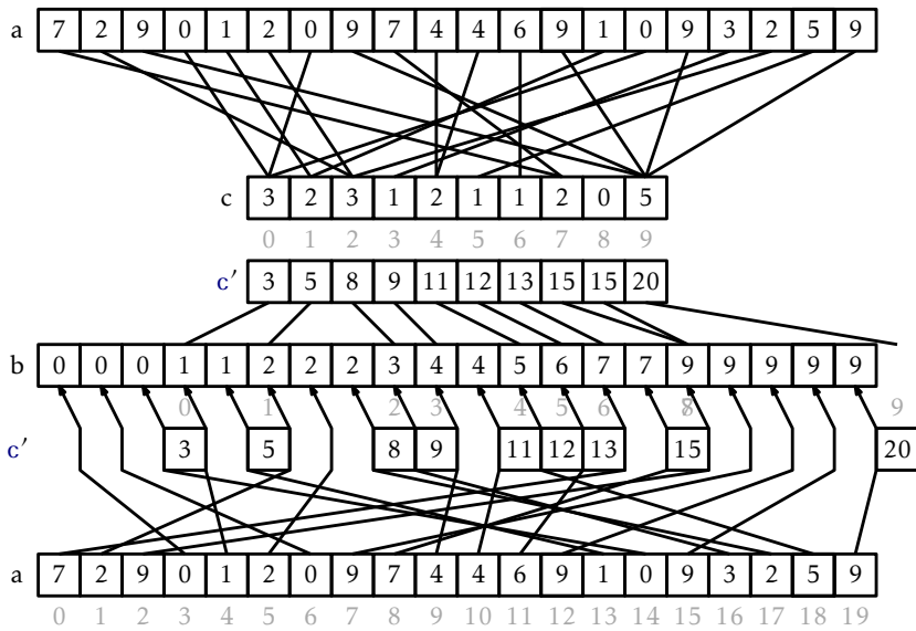
Slika 11.7: Operacija urejanja s štejetjem na polju velikosti n = 20 , ki shrani 0, \dots, k-1 = 9 števil.
