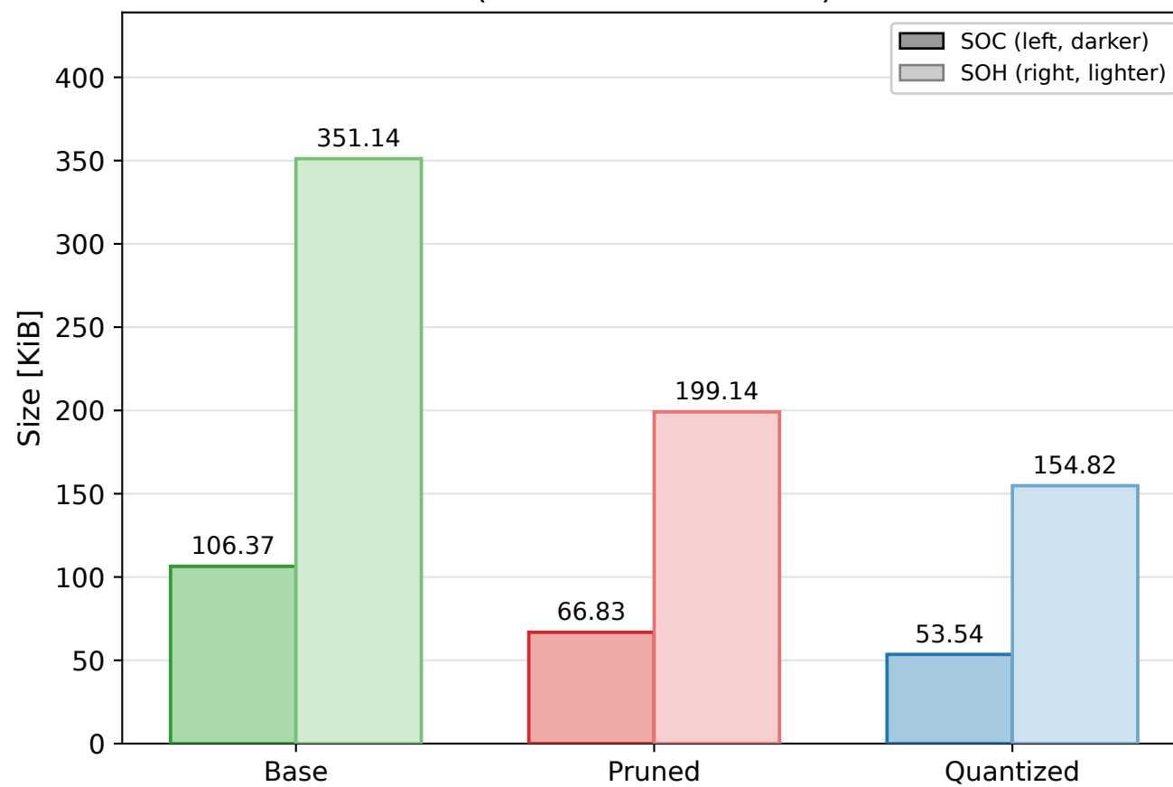
Firmware flash (available ELF builds)
