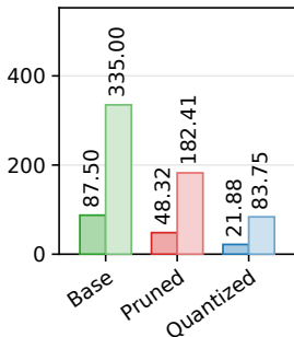
(d) RAM [KiB] static + peak stack
