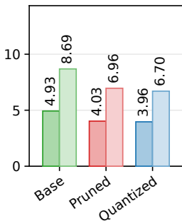
(d) RAM [KiB] static + peak stack
