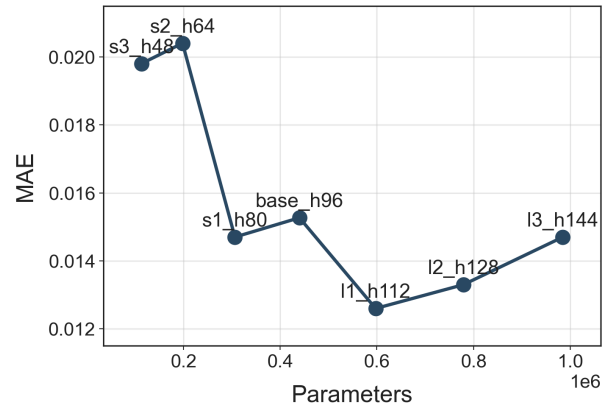
(d) TCN
