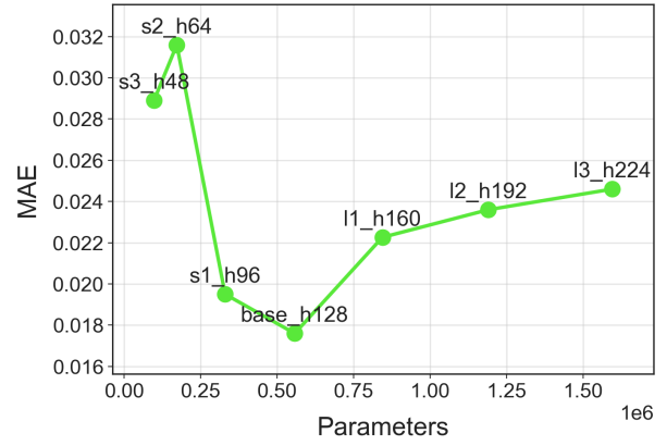
(b) GRU
