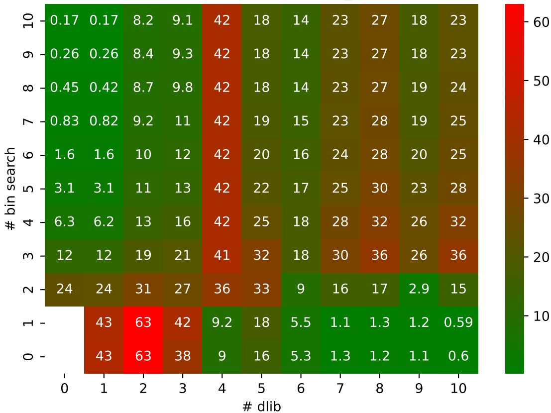
QVAPOR SZ3 pressio:abs MAPE: bin_search vs dlib
