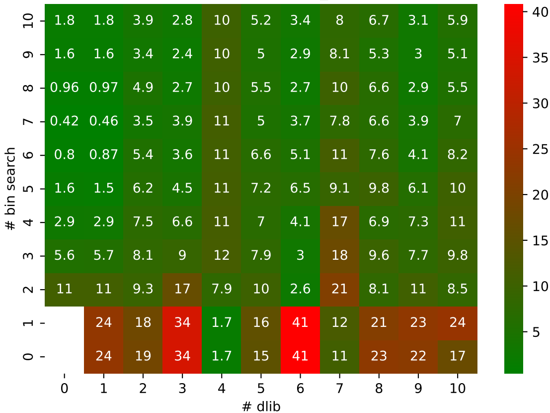
TC SZ3 pressio:abs MAPE: bin_search vs dlib
