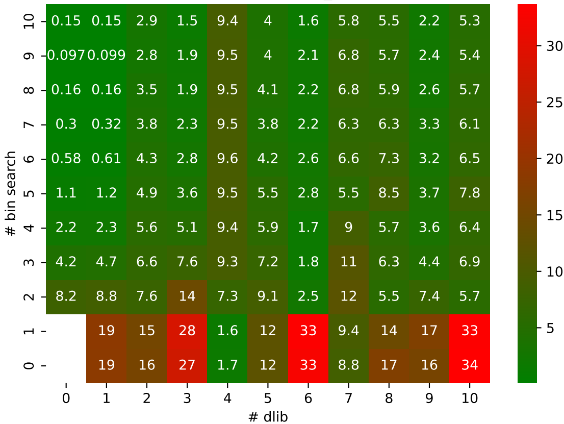
V SZ3 pressio:abs MAPE: bin_search vs dlib
