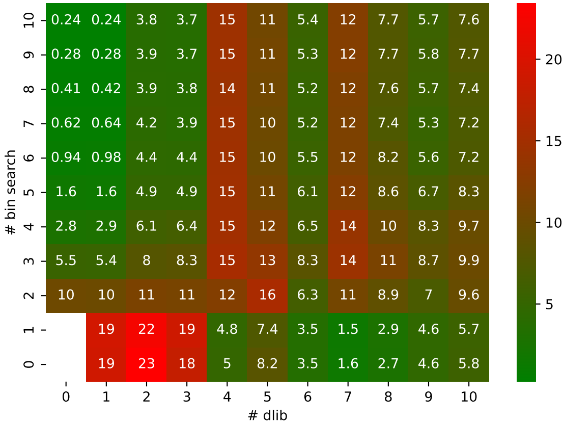
QICE SZ3 pressio:abs MAPE: bin_search vs dlib
