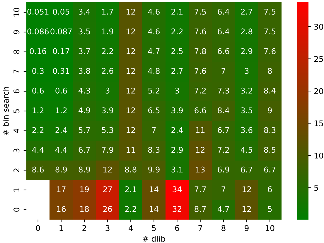
W SZ3 pressio:abs MAPE: bin_search vs dlib
