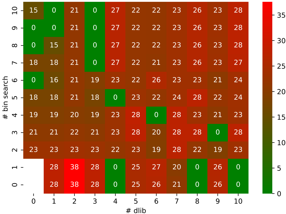
QVAPOR ZFP pressio:abs MAPE: bin_search vs dlib
