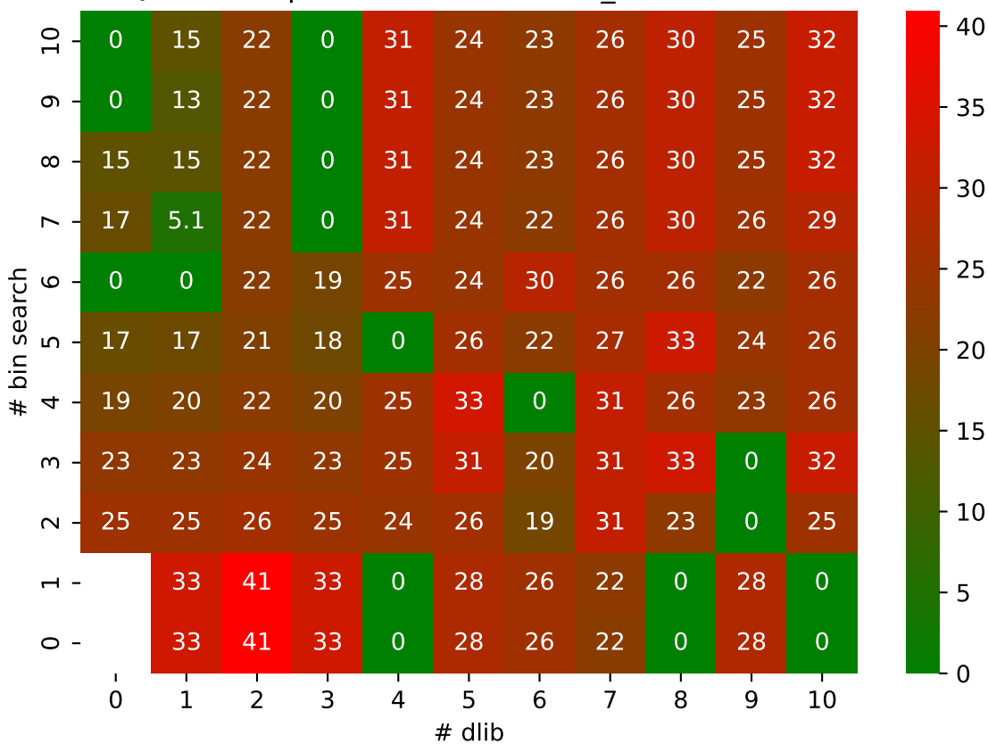
QRAIN ZFP pressio:abs MAPE: bin_search vs dlib
