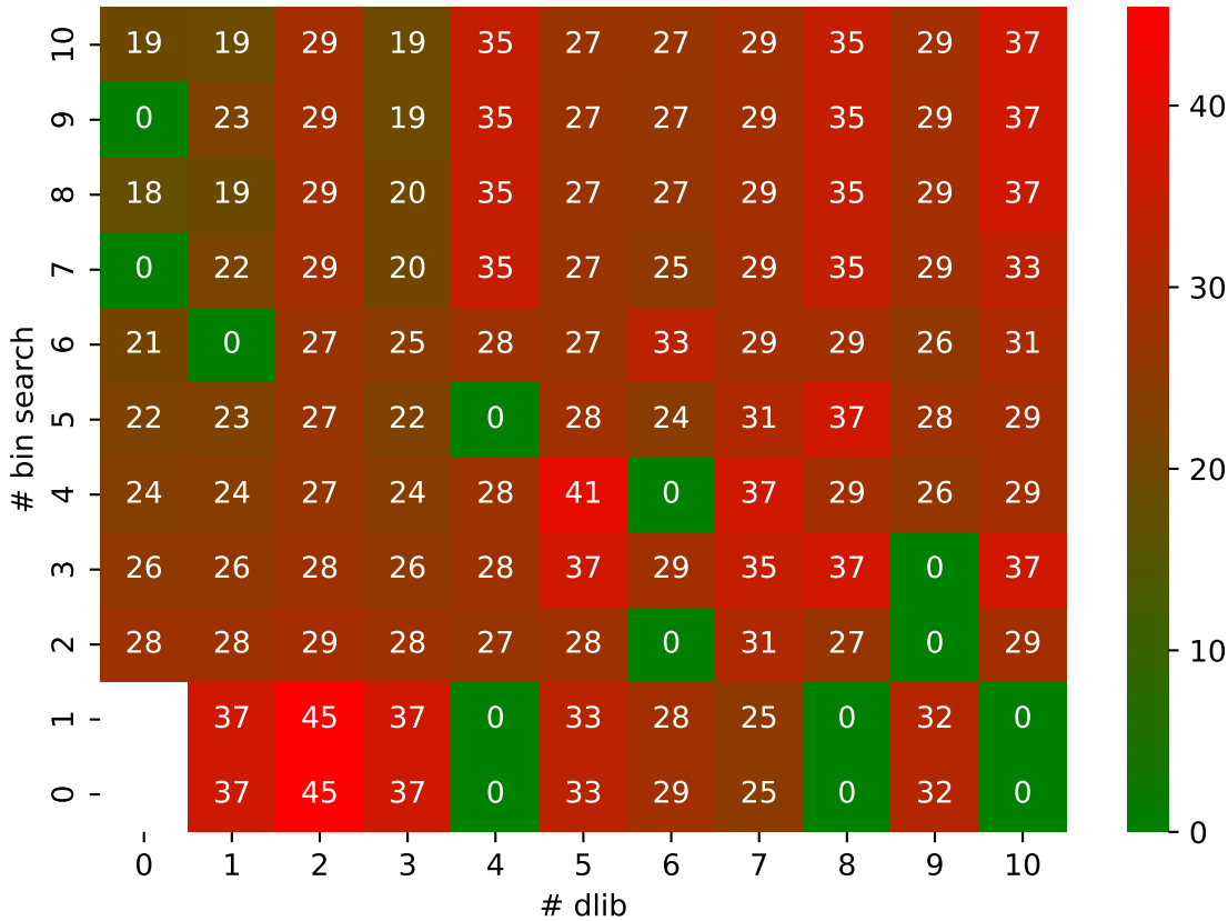
PRECIP ZFP pressio:abs MAPE: bin_search vs dlib
