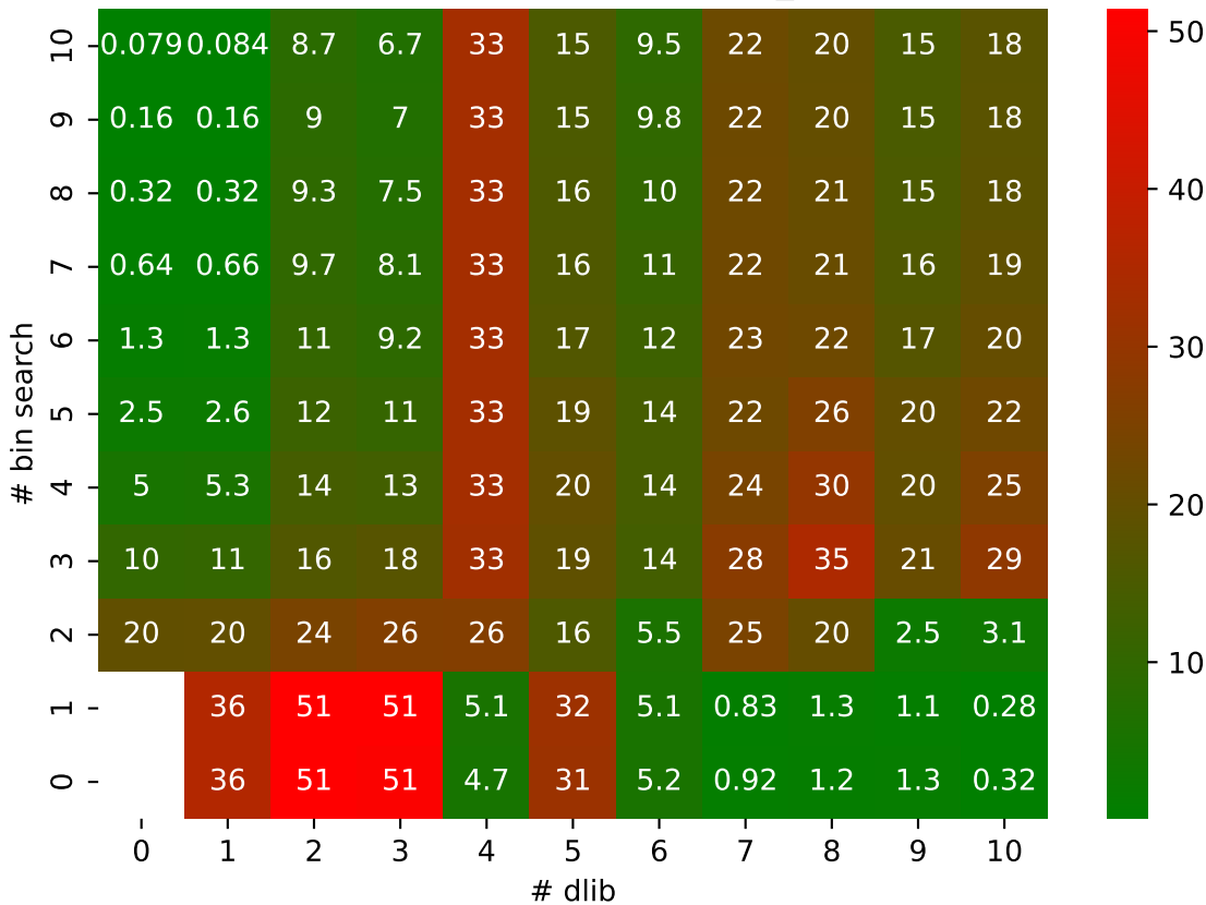
QVAPOR SPERR pressio:abs MAPE: bin_search vs dlib
