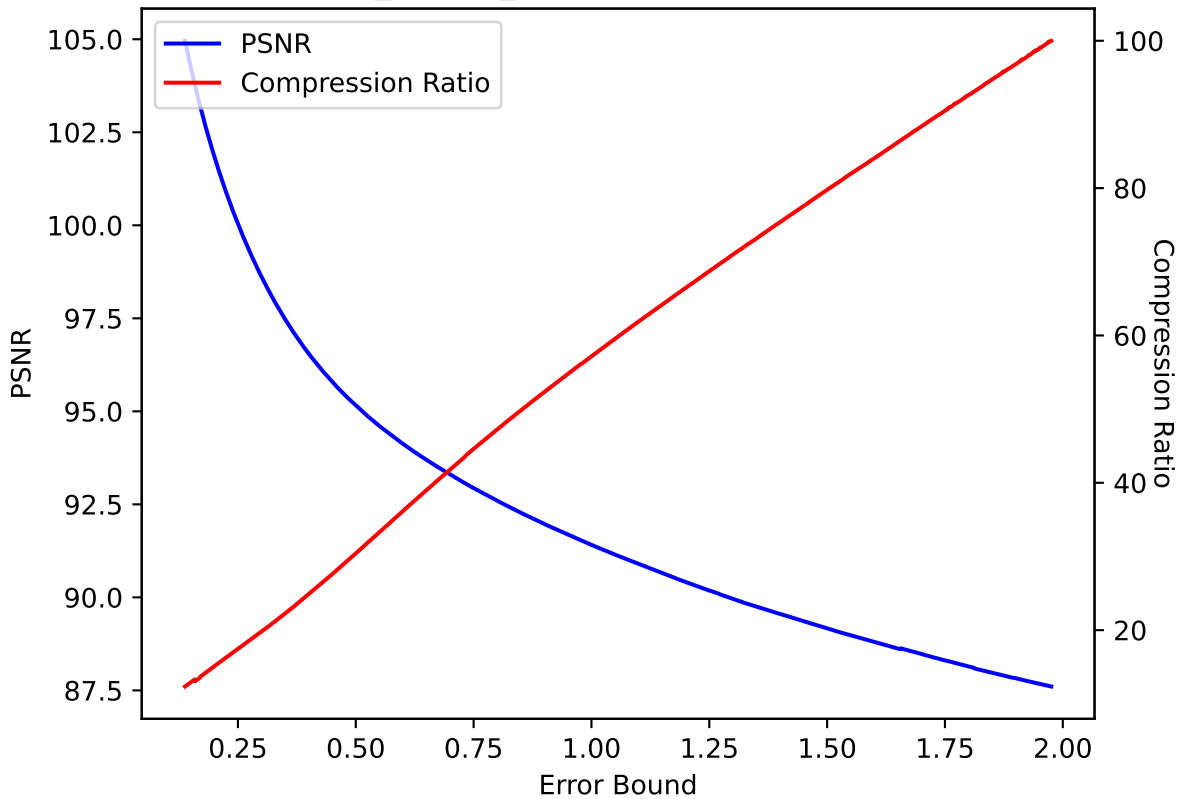
dark_matter_density 01 SZ3 pressio:rel
