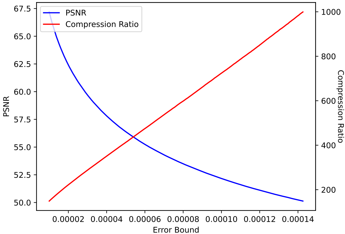
CLOUD 07 SPERR pressio:abs
