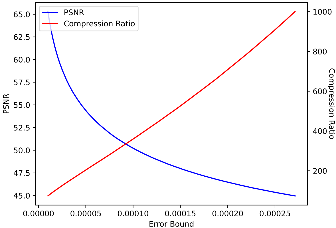
CLOUD 47 SPERR pressio:abs
