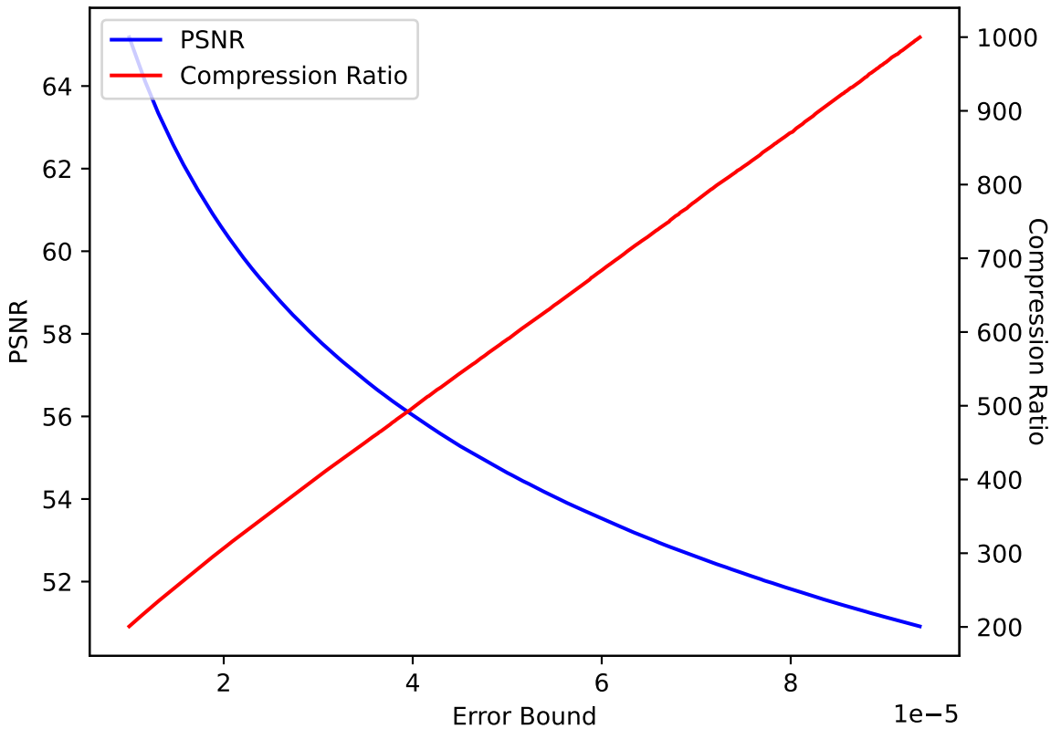
CLOUD 06 SPERR pressio:abs
