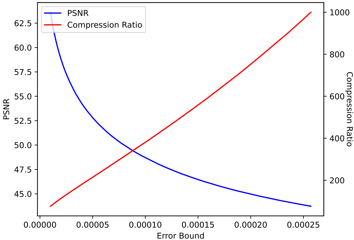
CLOUD 44 SPERR pressio:abs
