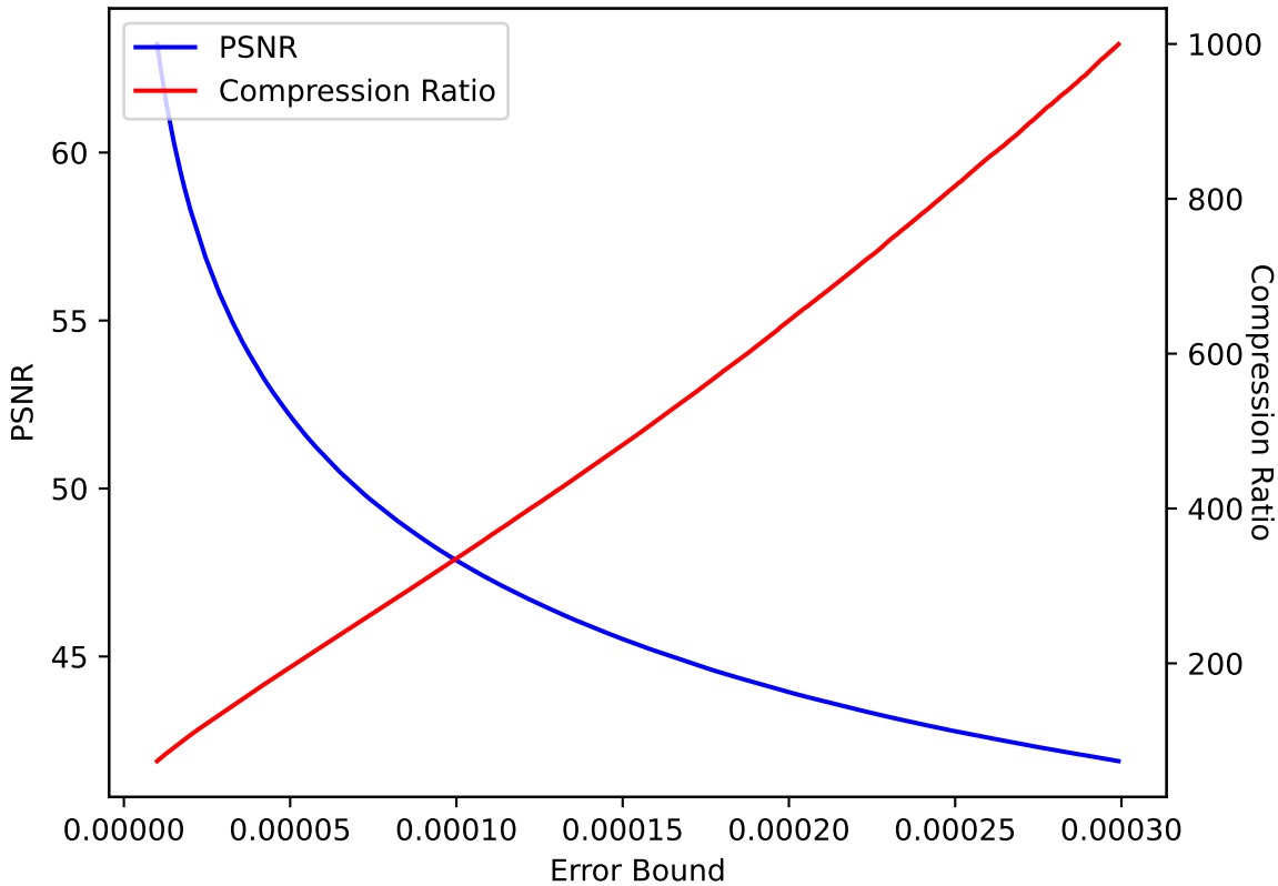
CLOUD 26 SPERR pressio:abs
