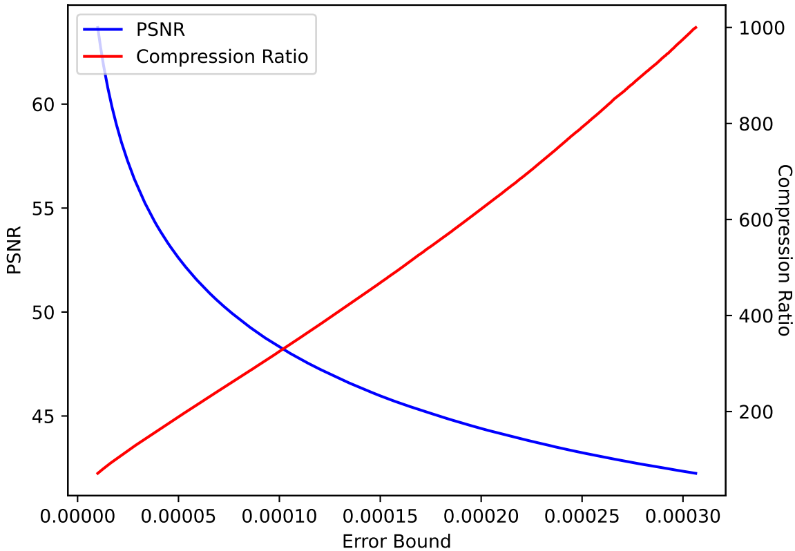
CLOUD 29 SPERR pressio:abs
