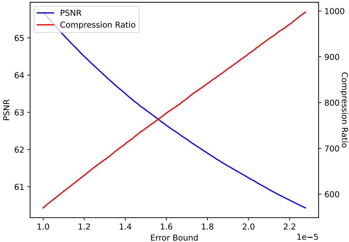
CLOUD 02 SPERR pressio:abs
