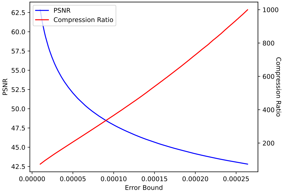
CLOUD 41 SPERR pressio:abs
