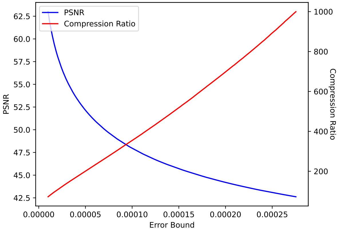
CLOUD 39 SPERR pressio:abs
