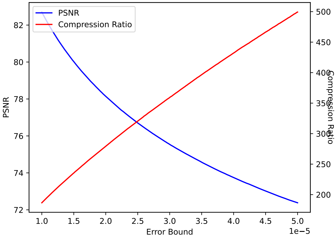
PRECIP 13 SPERR pressio:abs
