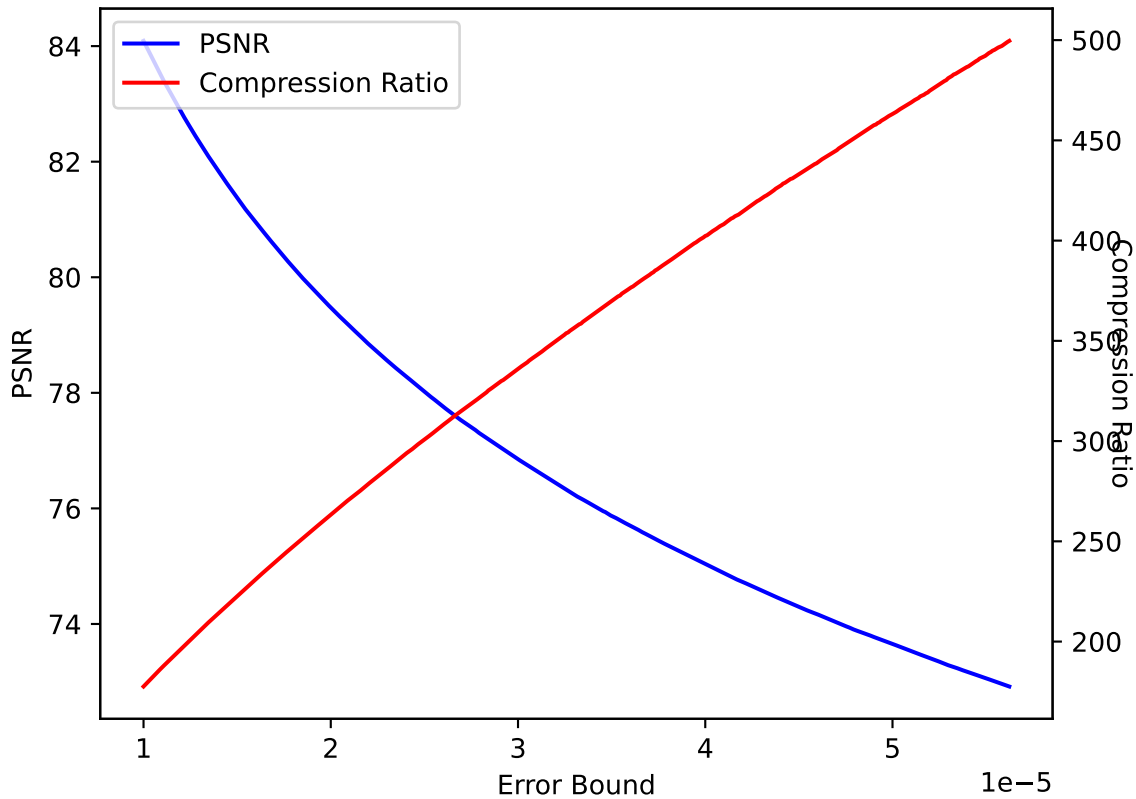
PRECIP 12 SPERR pressio:abs
