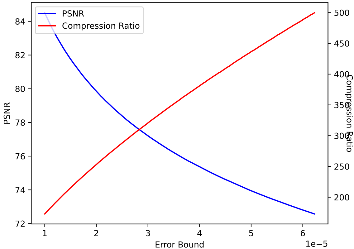
PRECIP 10 SPERR pressio:abs
