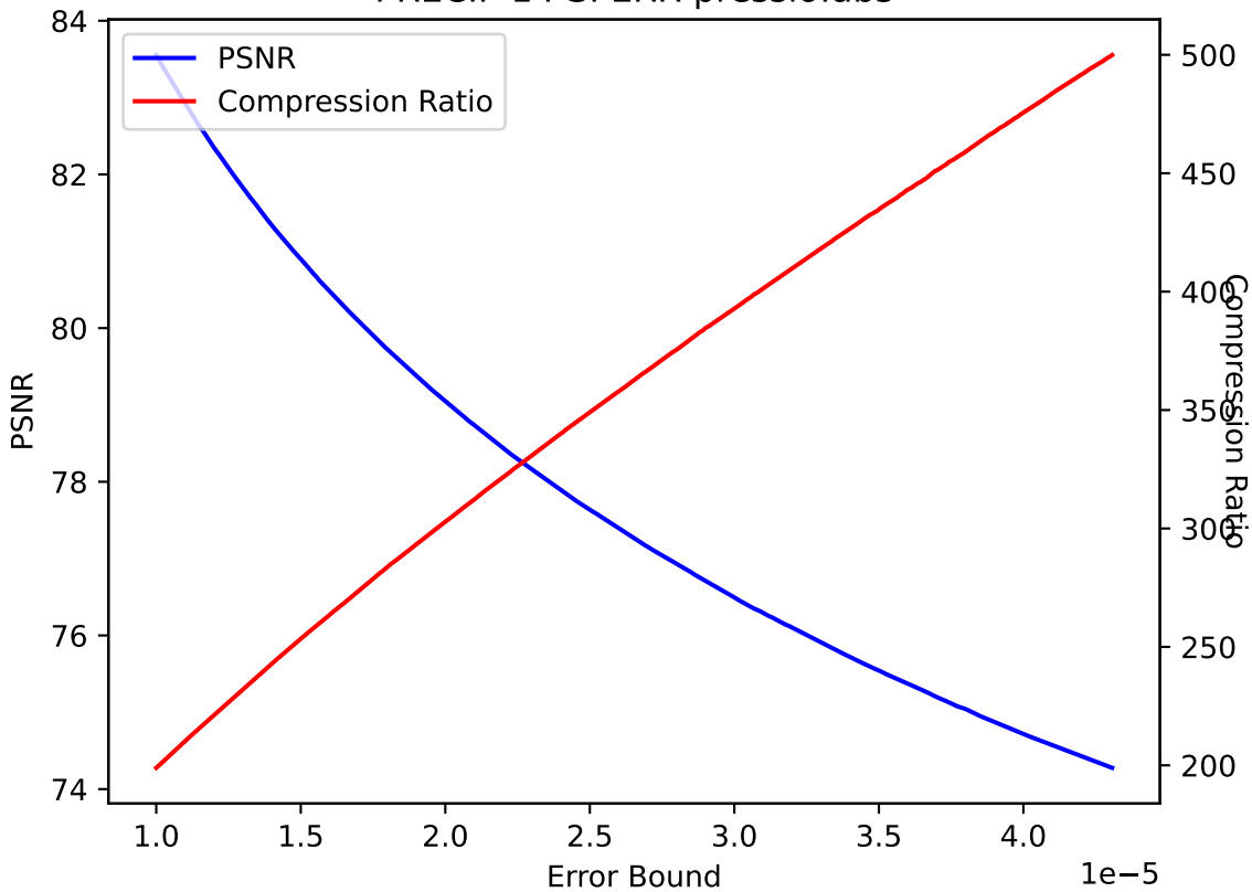
PRECIP 14 SPERR pressio:abs
