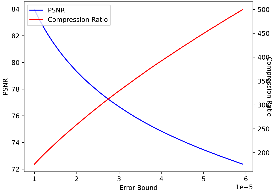
PRECIP 11 SPERR pressio:abs
