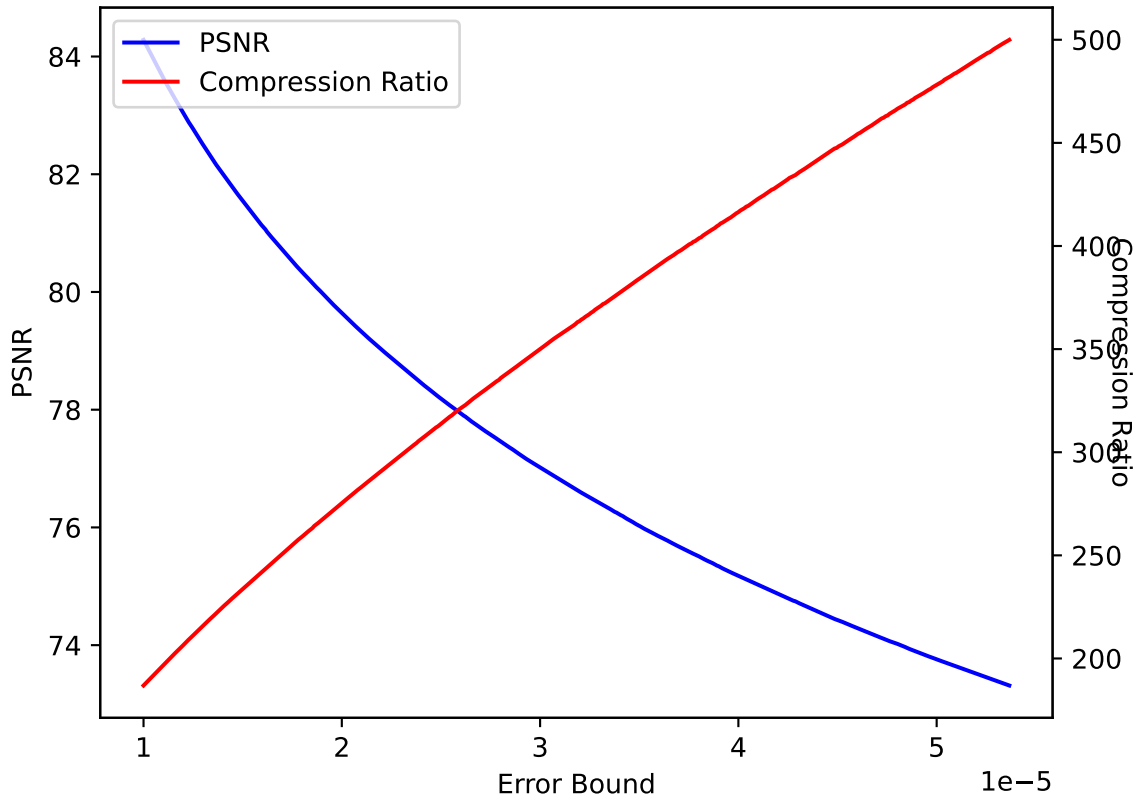
PRECIP 09 SPERR pressio:abs
