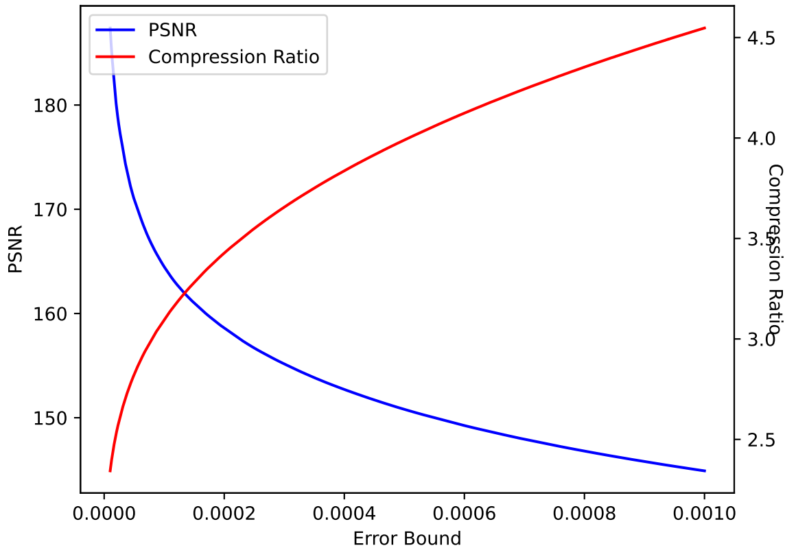
P 17 SPERR pressio:abs
