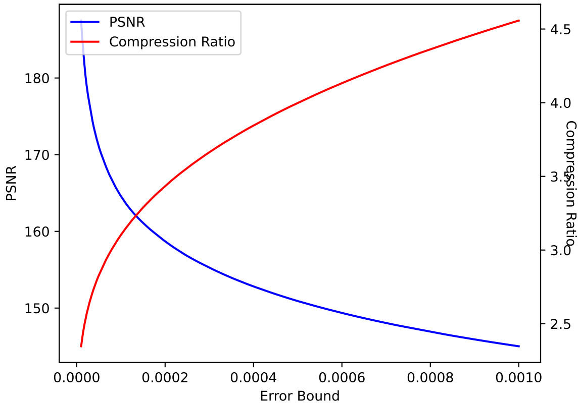
P 13 SPERR pressio:abs
