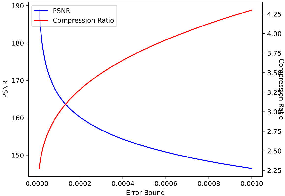
P 31 SPERR pressio:abs
