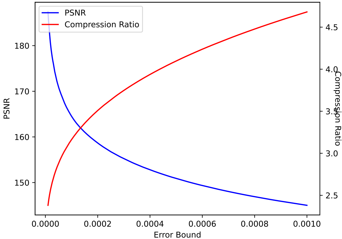
P 11 SPERR pressio:abs
