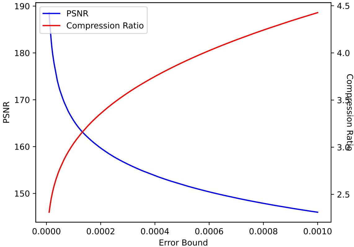
P 42 SPERR pressio:abs
