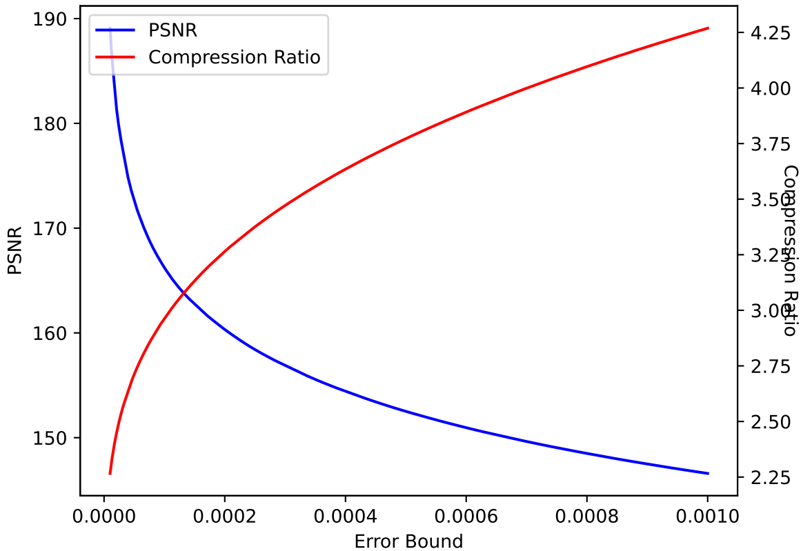
P 34 SPERR pressio:abs
