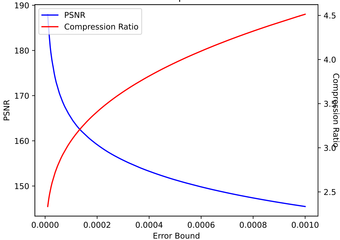
P 45 SPERR pressio:abs
