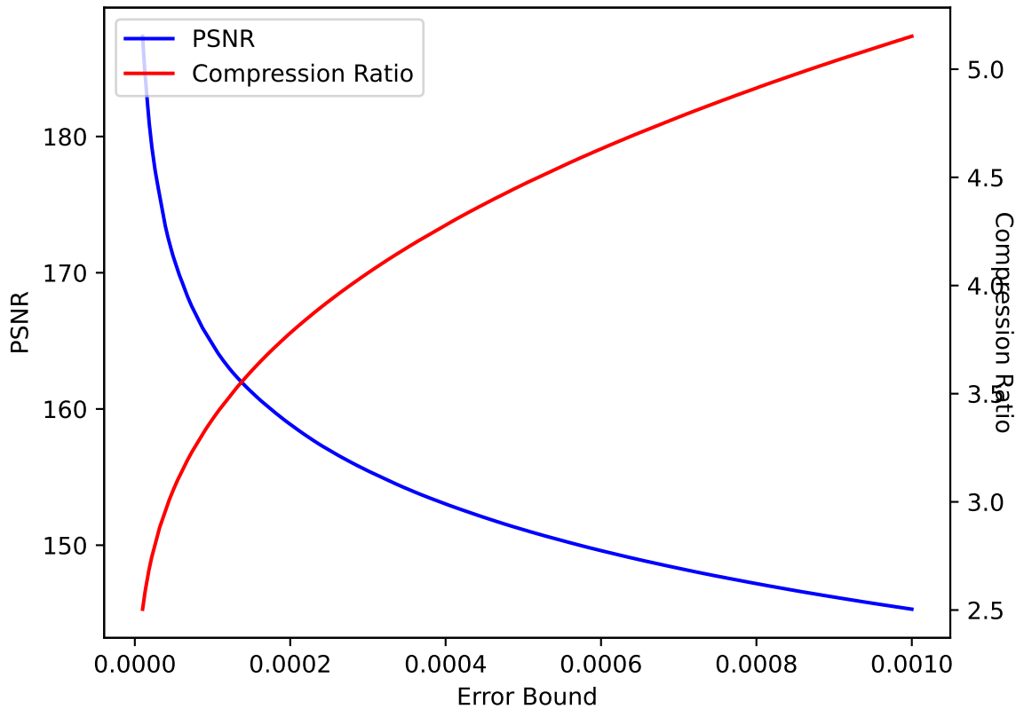
P 08 SPERR pressio:abs
