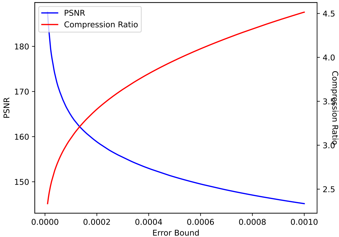
P 20 SPERR pressio:abs
