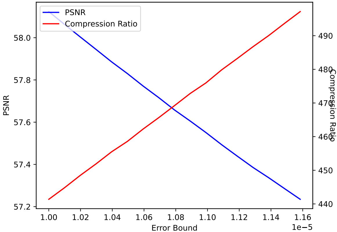
QICE 29 SPERR pressio:abs
