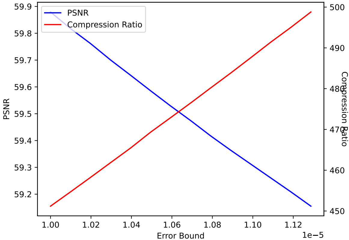
QICE 46 SPERR pressio:abs
