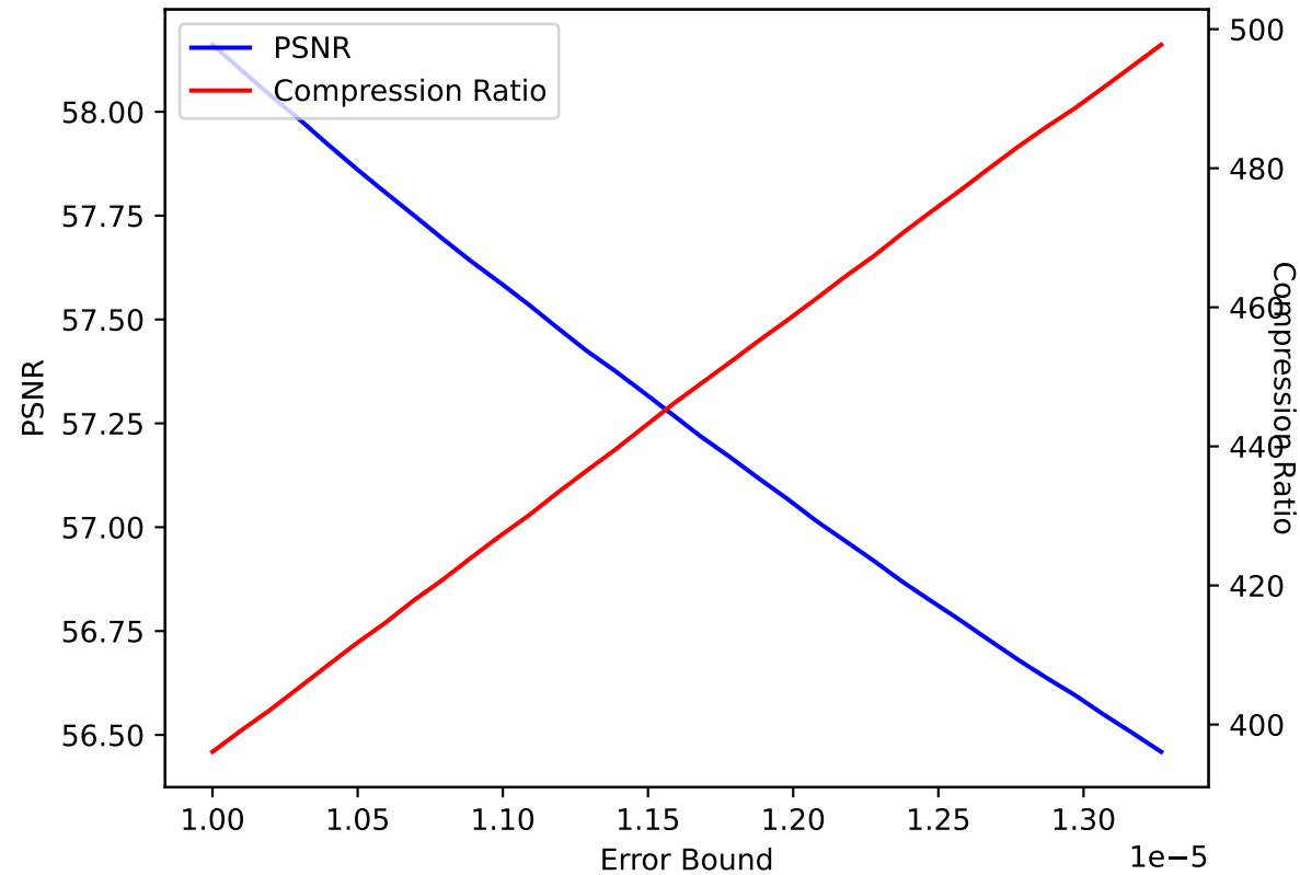
QICE 14 SPERR pressio:abs
