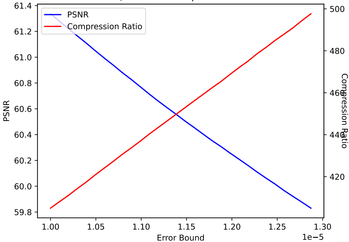
QICE 34 SPERR pressio:abs
