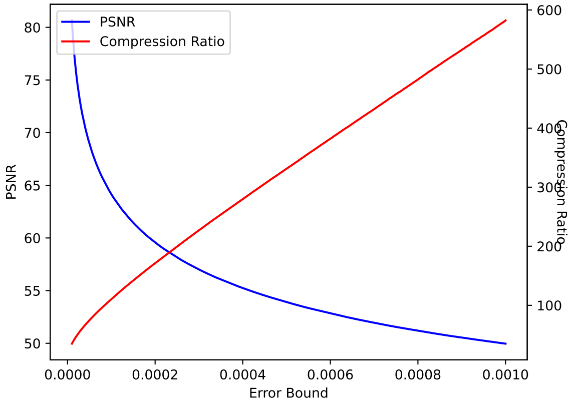
QVAPOR 11 SPERR pressio:abs
