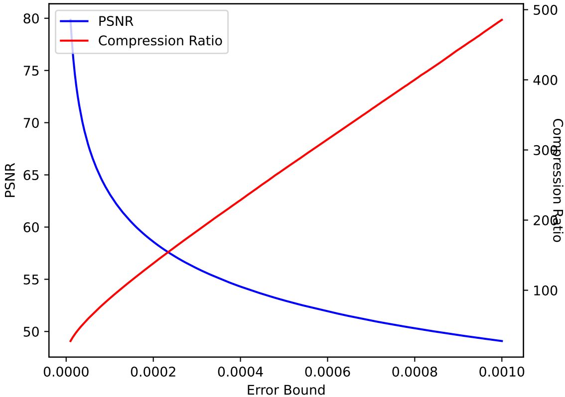
QVAPOR 39 SPERR pressio:abs
