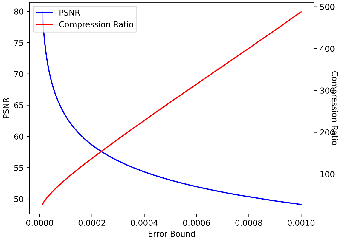
QVAPOR 37 SPERR pressio:abs
