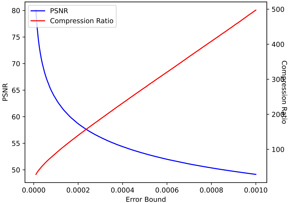
QVAPOR 24 SPERR pressio:abs
