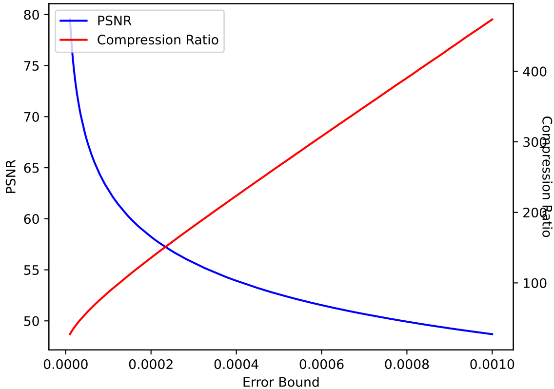
QVAPOR 43 SPERR pressio:abs
