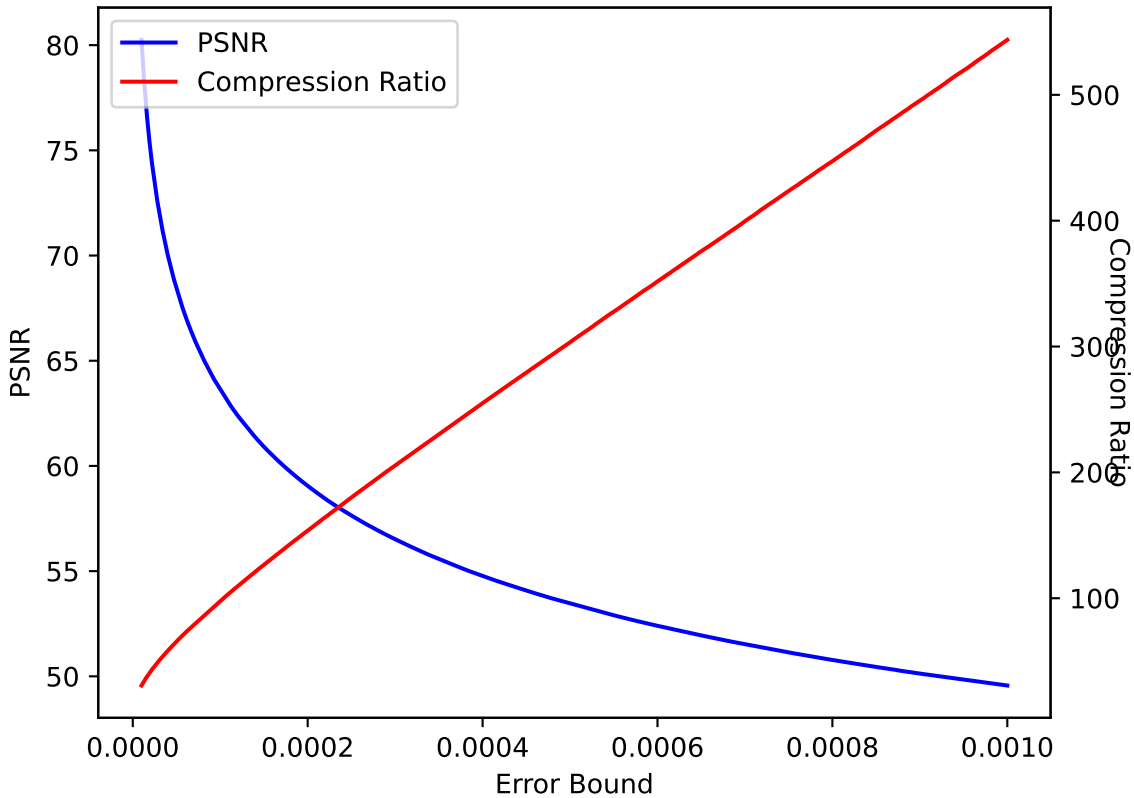
QVAPOR 18 SPERR pressio:abs
