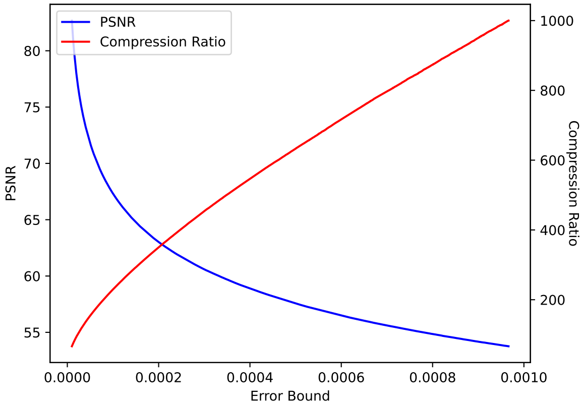
QVAPOR 05 SPERR pressio:abs
