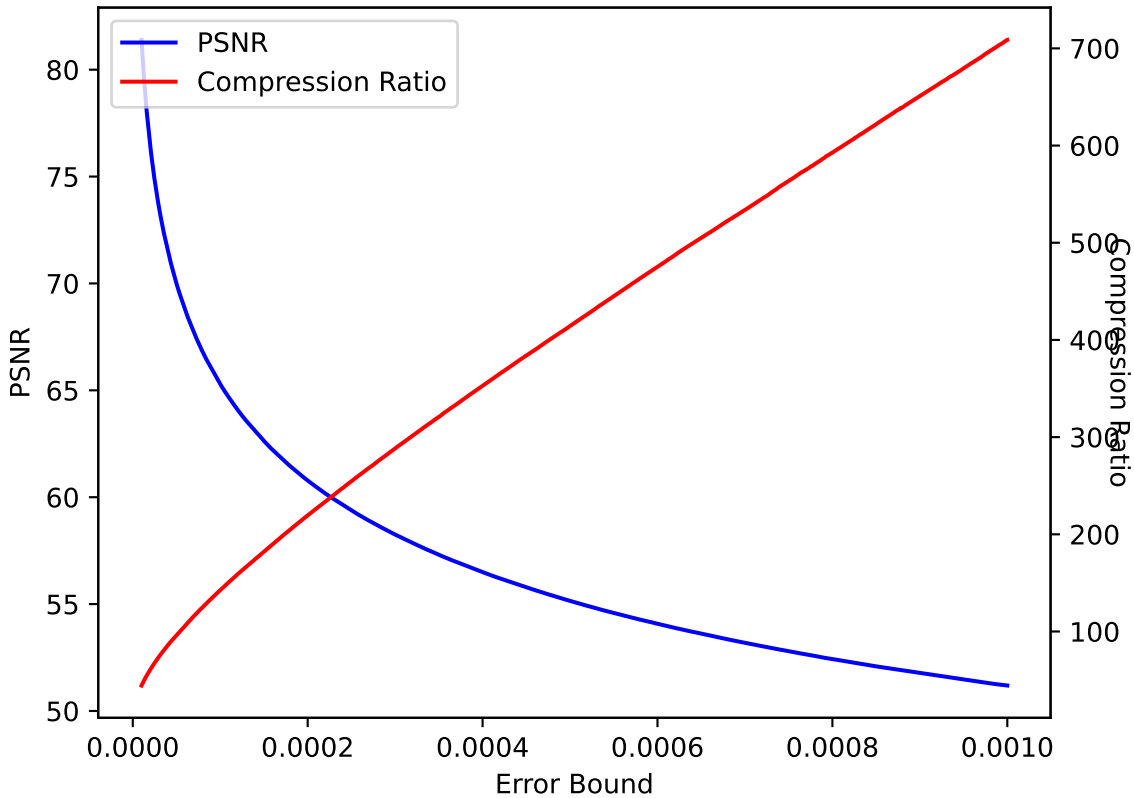
QVAPOR 08 SPERR pressio:abs
