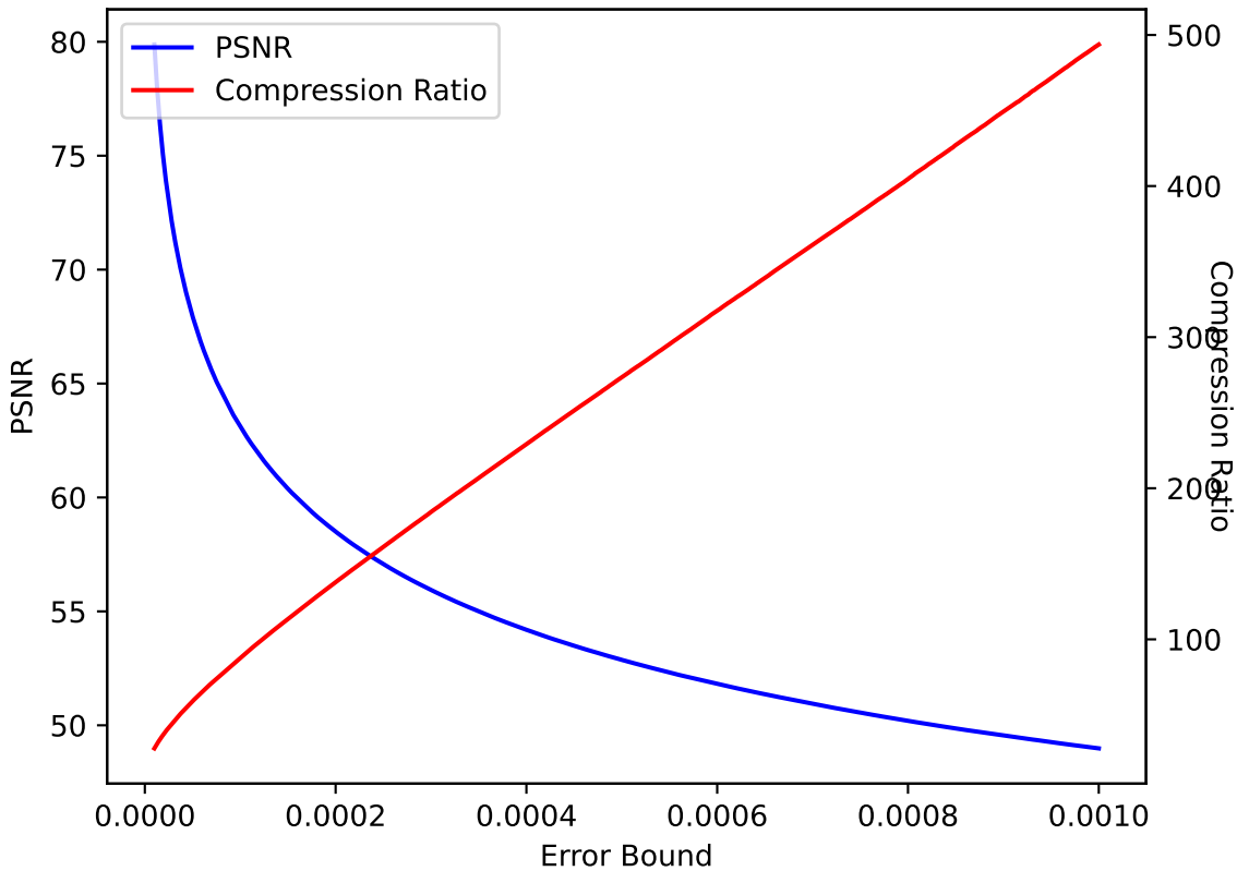
QVAPOR 31 SPERR pressio:abs
