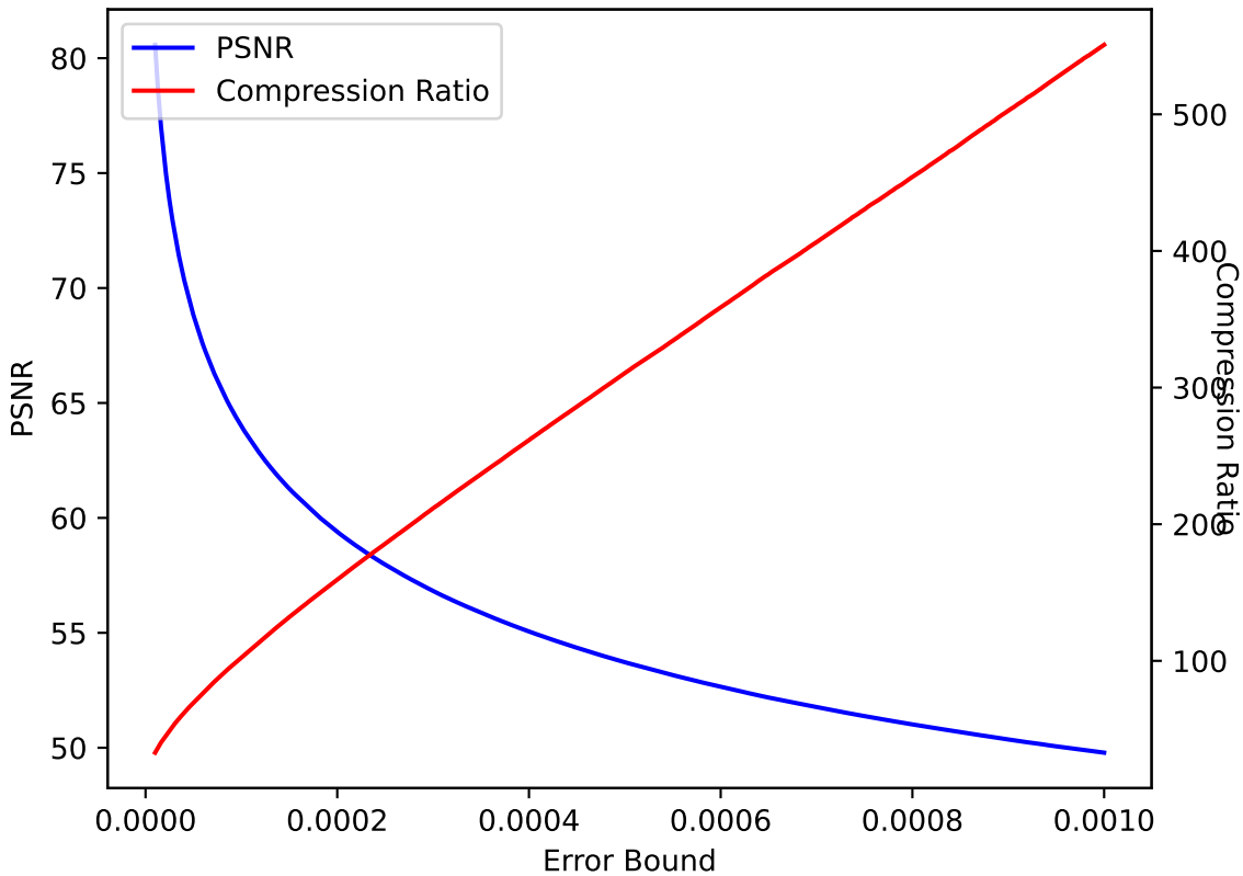
QVAPOR 13 SPERR pressio:abs
