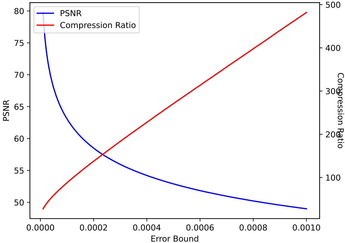
QVAPOR 40 SPERR pressio:abs
