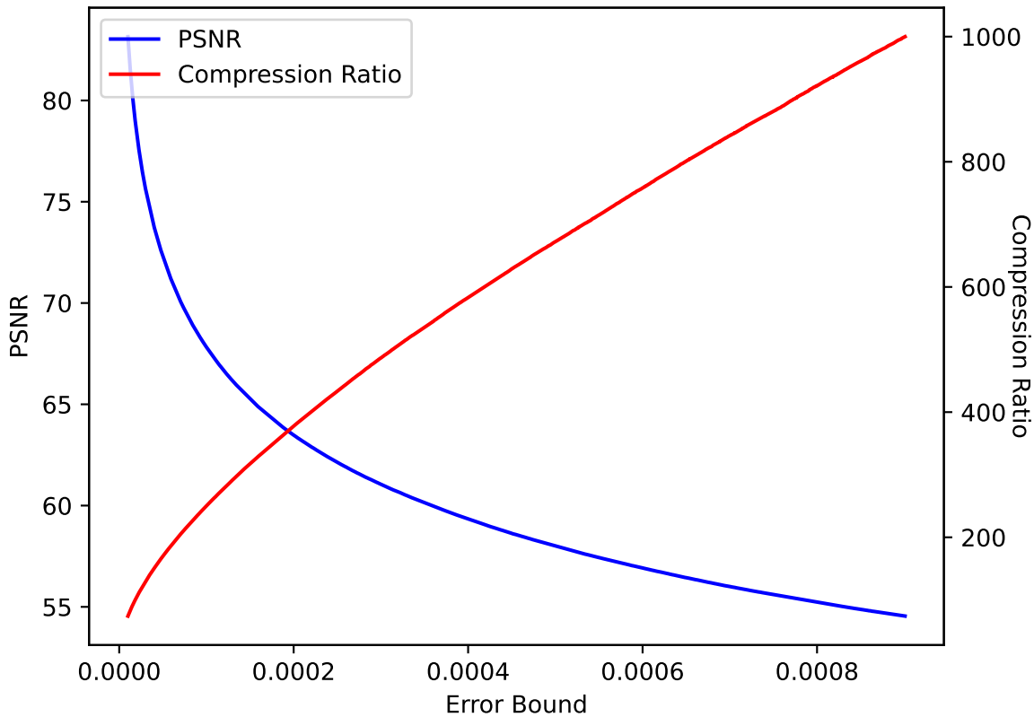
QVAPOR 04 SPERR pressio:abs
