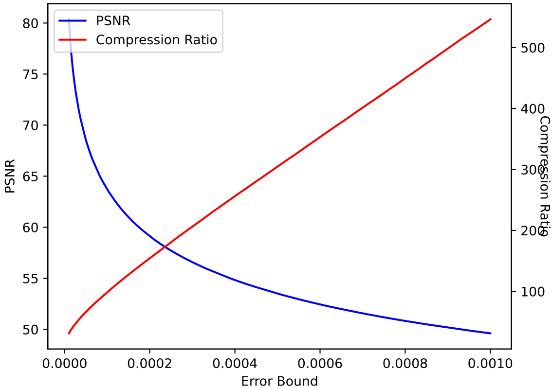
QVAPOR 16 SPERR pressio:abs
