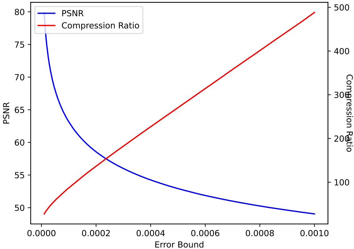
QVAPOR 34 SPERR pressio:abs
