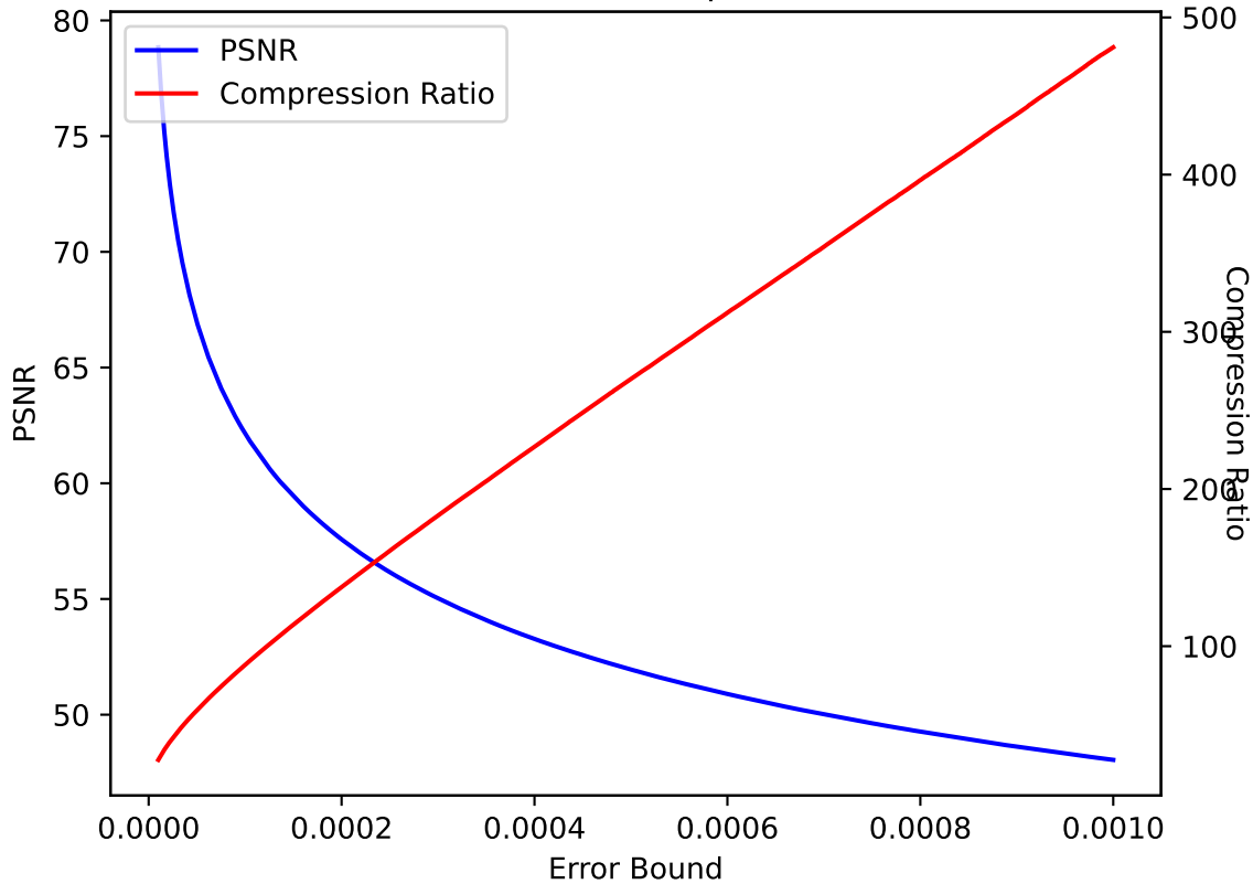
QVAPOR 45 SPERR pressio:abs
