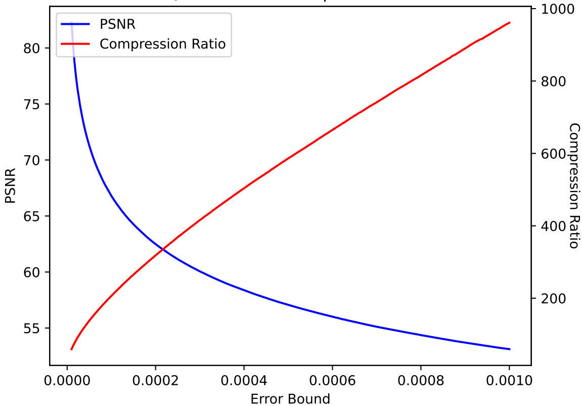
QVAPOR 06 SPERR pressio:abs
