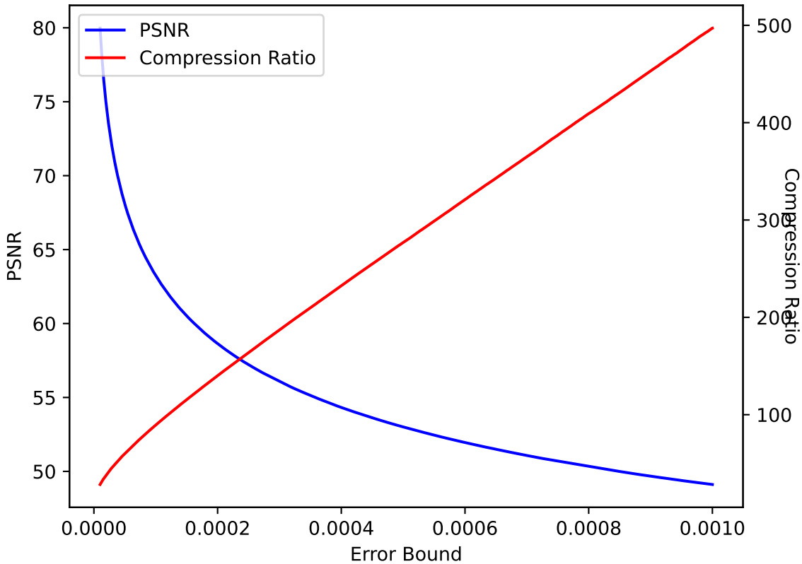
QVAPOR 27 SPERR pressio:abs
