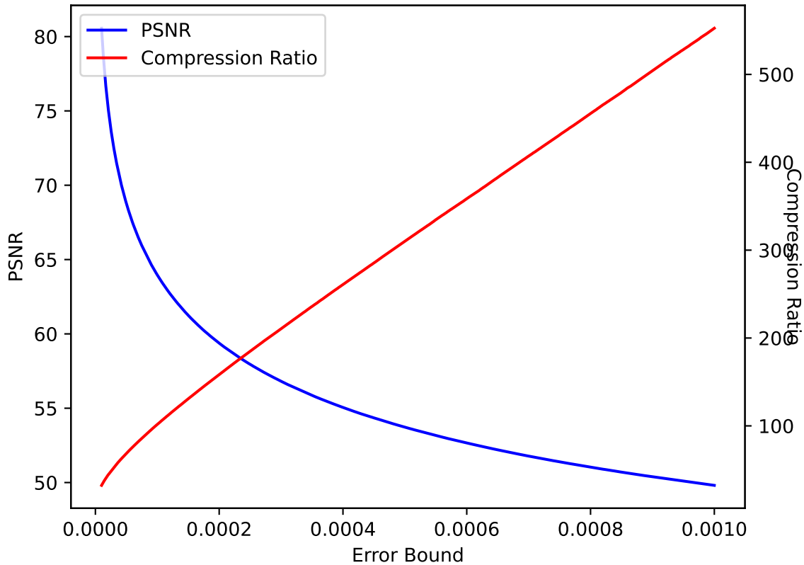
QVAPOR 14 SPERR pressio:abs
