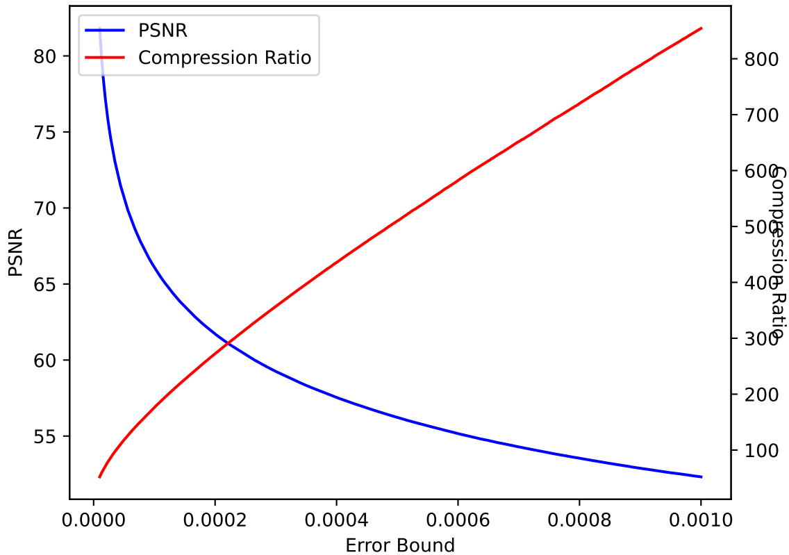
QVAPOR 07 SPERR pressio:abs
