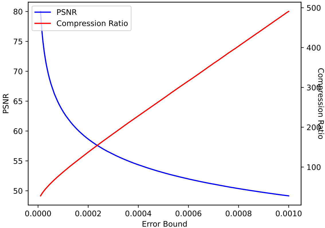
QVAPOR 33 SPERR pressio:abs
