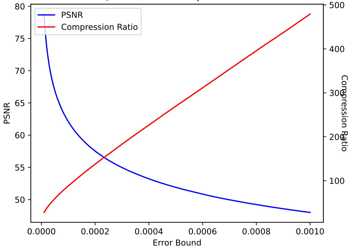
QVAPOR 46 SPERR pressio:abs
