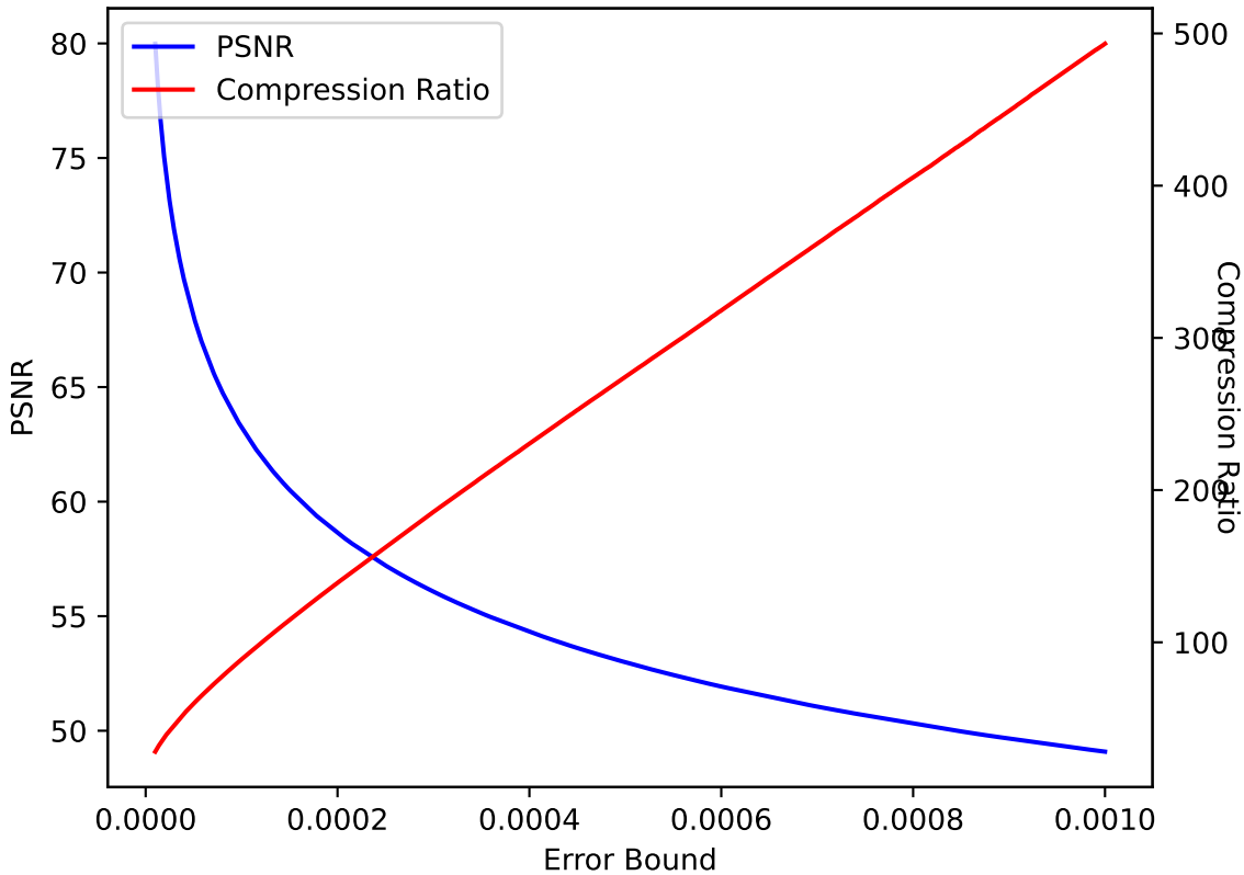
QVAPOR 28 SPERR pressio:abs
