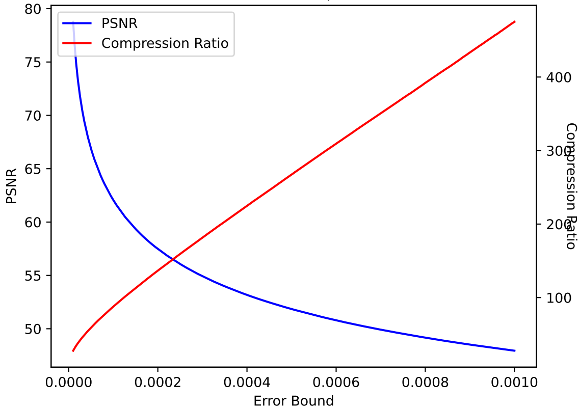
QVAPOR 47 SPERR pressio:abs
