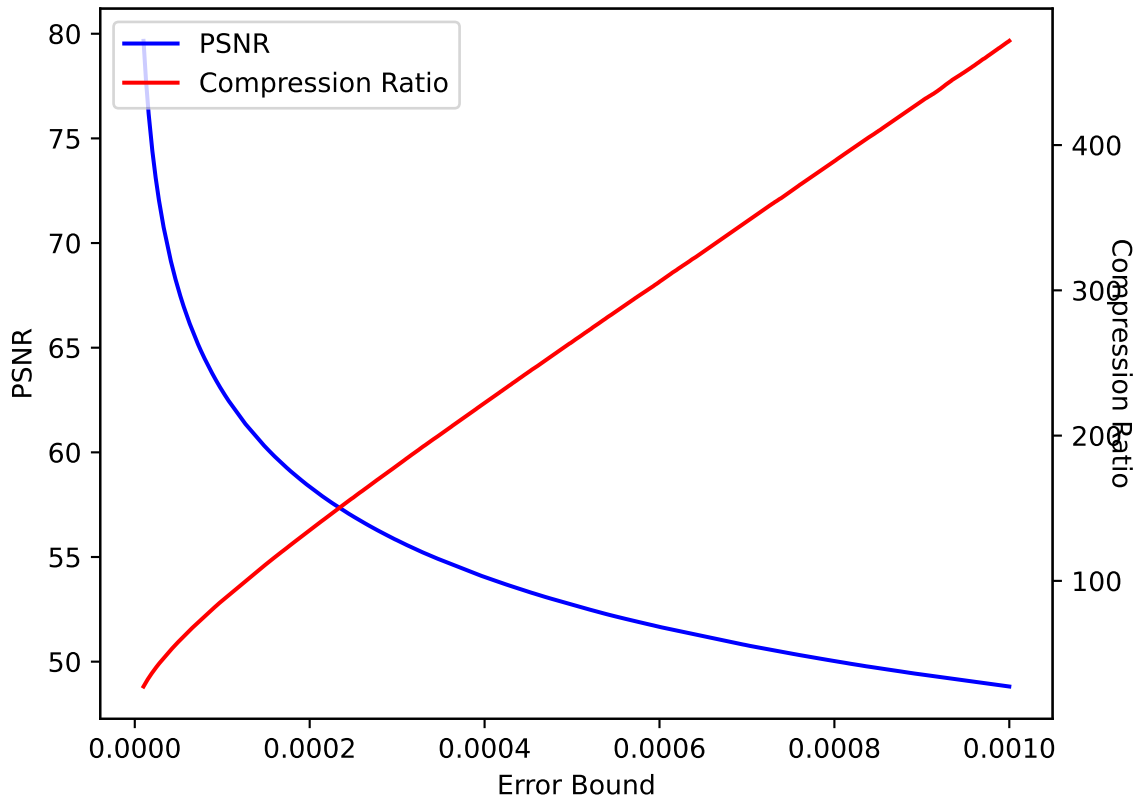
QVAPOR 42 SPERR pressio:abs
