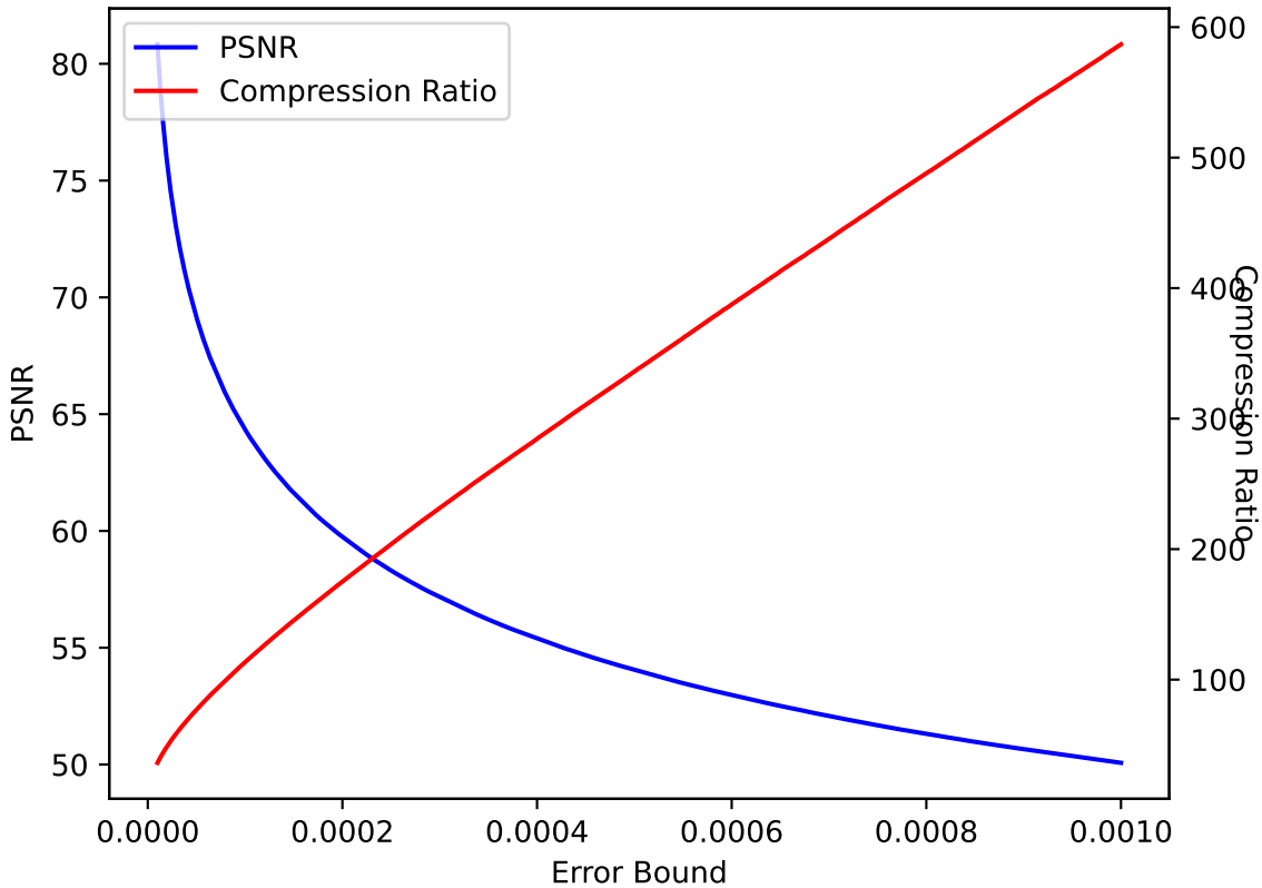
QVAPOR 10 SPERR pressio:abs
