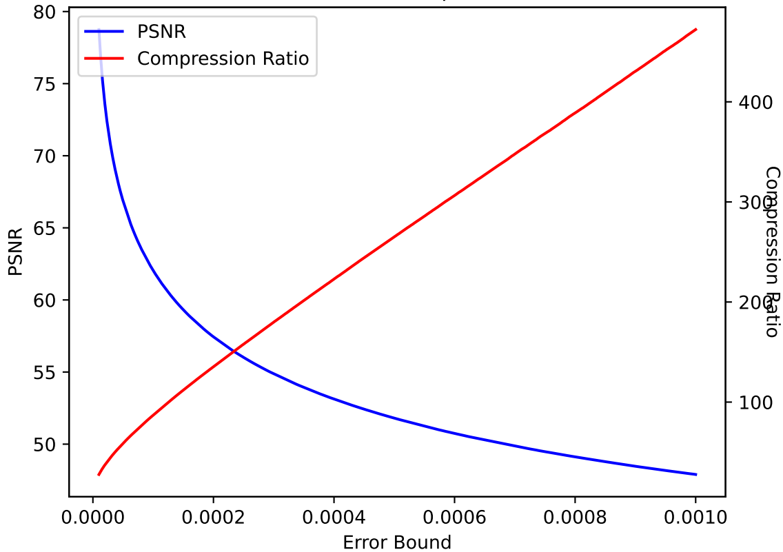
QVAPOR 48 SPERR pressio:abs
