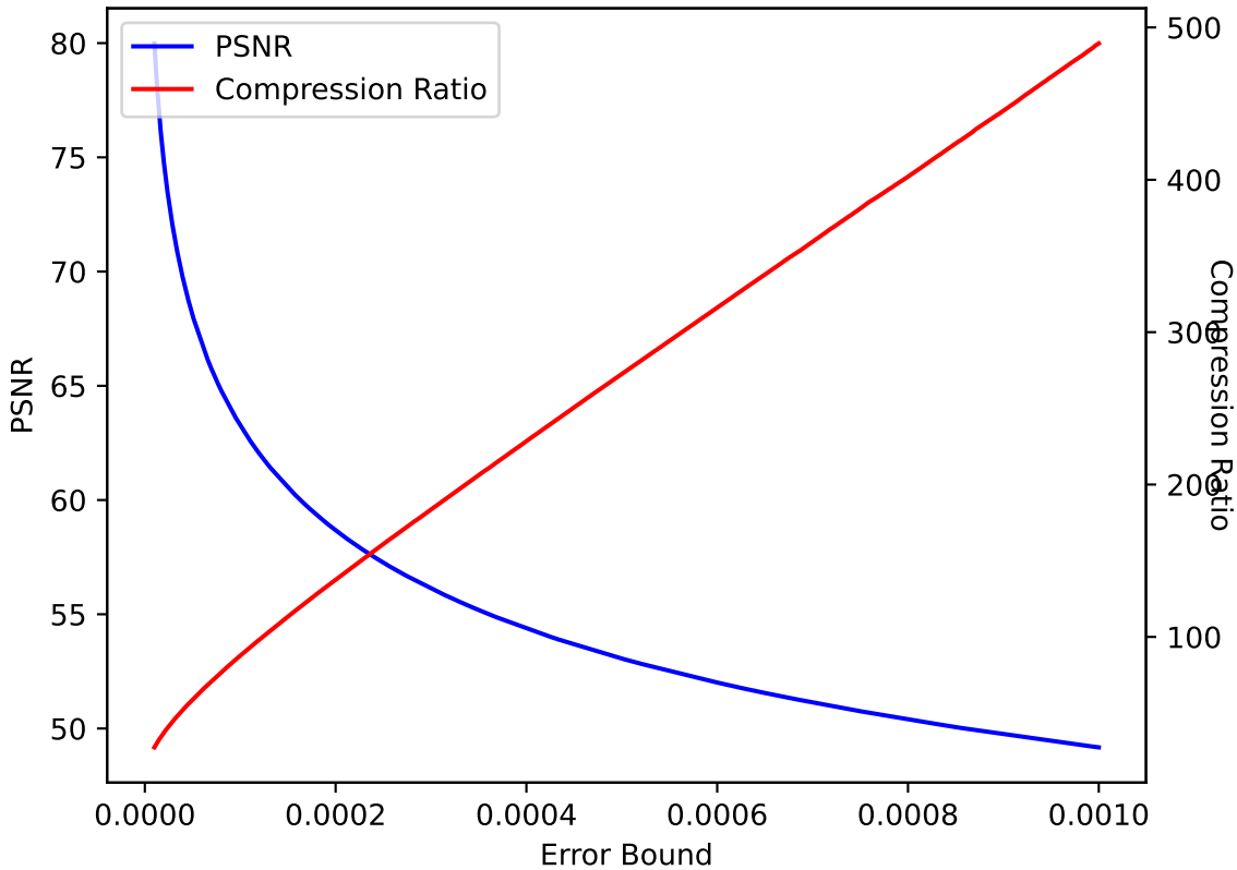
QVAPOR 36 SPERR pressio:abs
