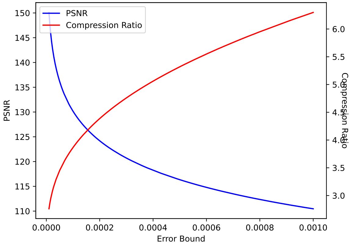
U 40 SPERR pressio:abs
