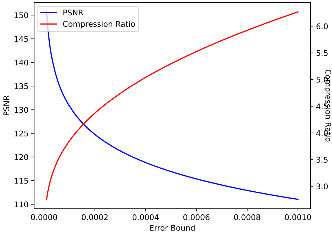
U 39 SPERR pressio:abs
