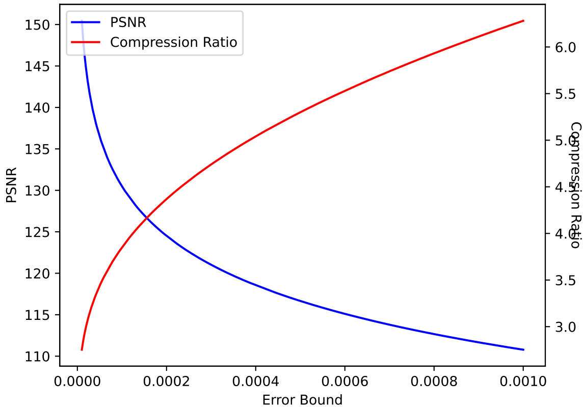
U 26 SPERR pressio:abs
