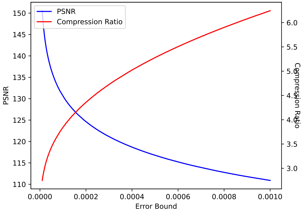
U 38 SPERR pressio:abs
