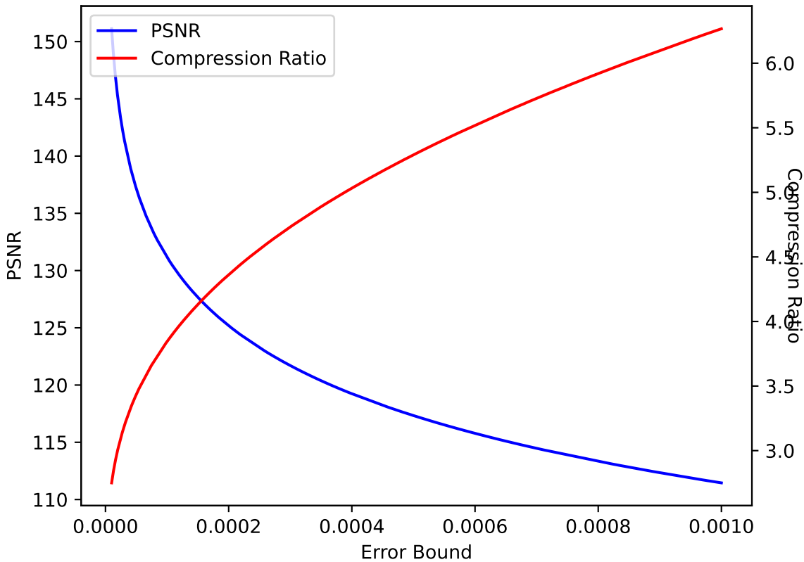
U 27 SPERR pressio:abs
