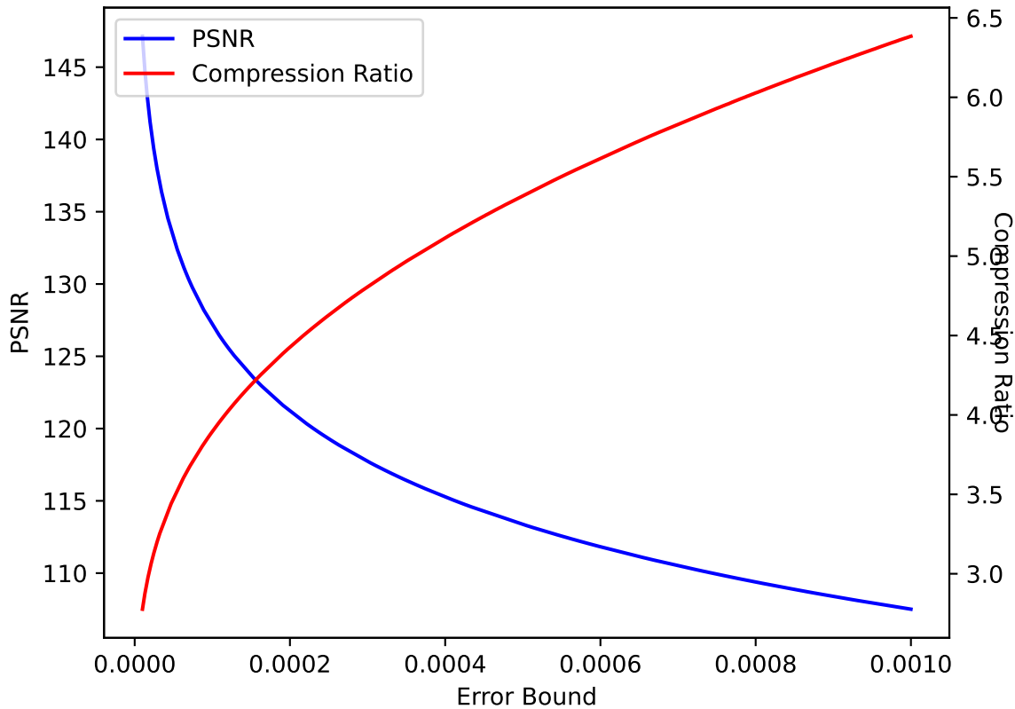
U 48 SPERR pressio:abs
