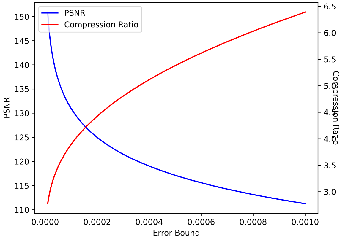
U 23 SPERR pressio:abs
