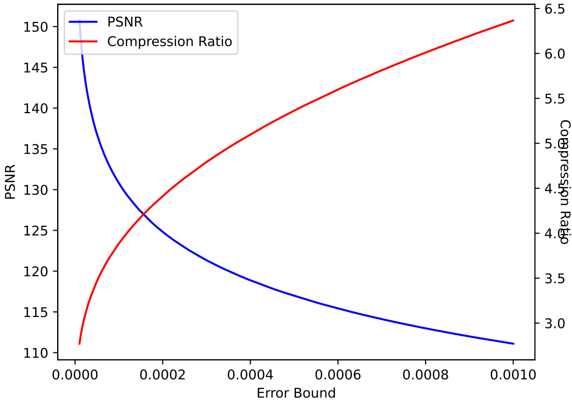
V 24 SPERR pressio:abs
