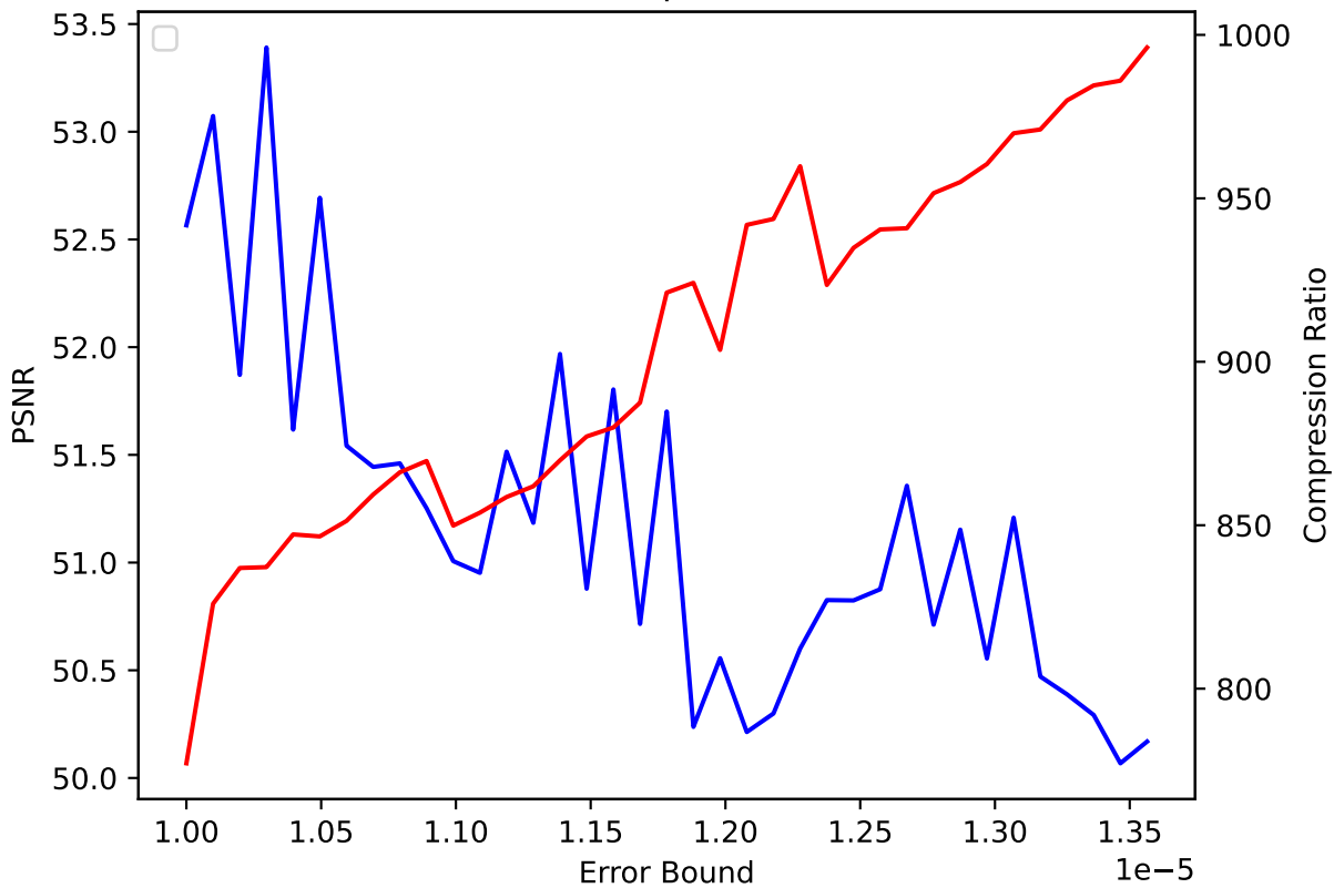
CLOUD 01 pressio:abs
