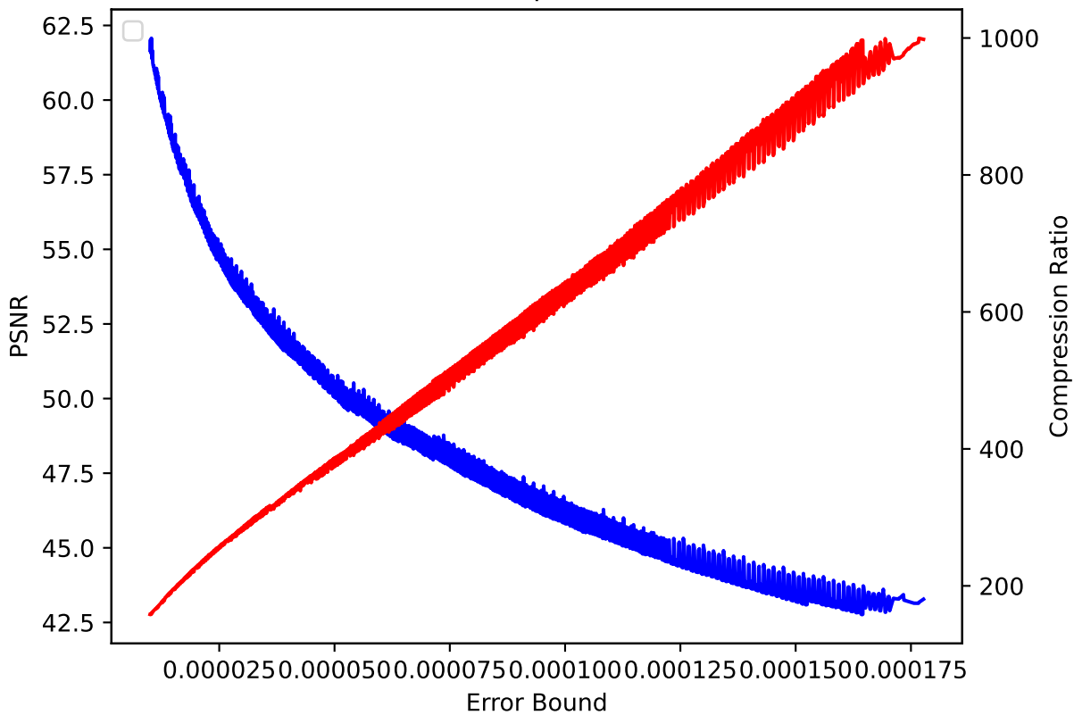
CLOUD 13 pressio:abs
