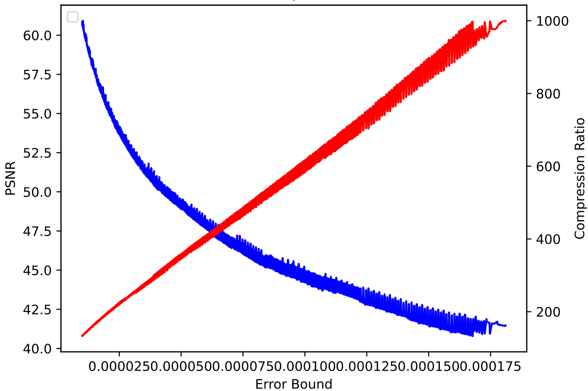
CLOUD 42 pressio:abs
