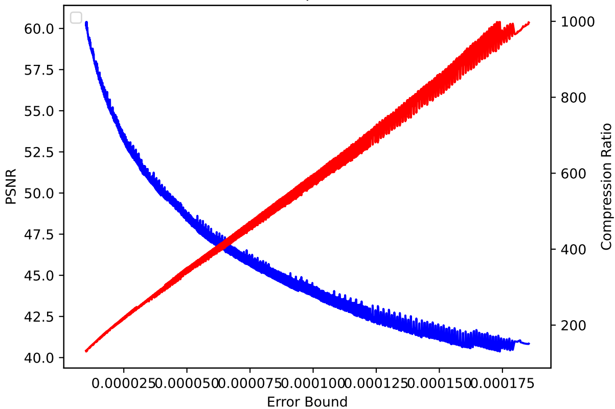
CLOUD 40 pressio:abs
