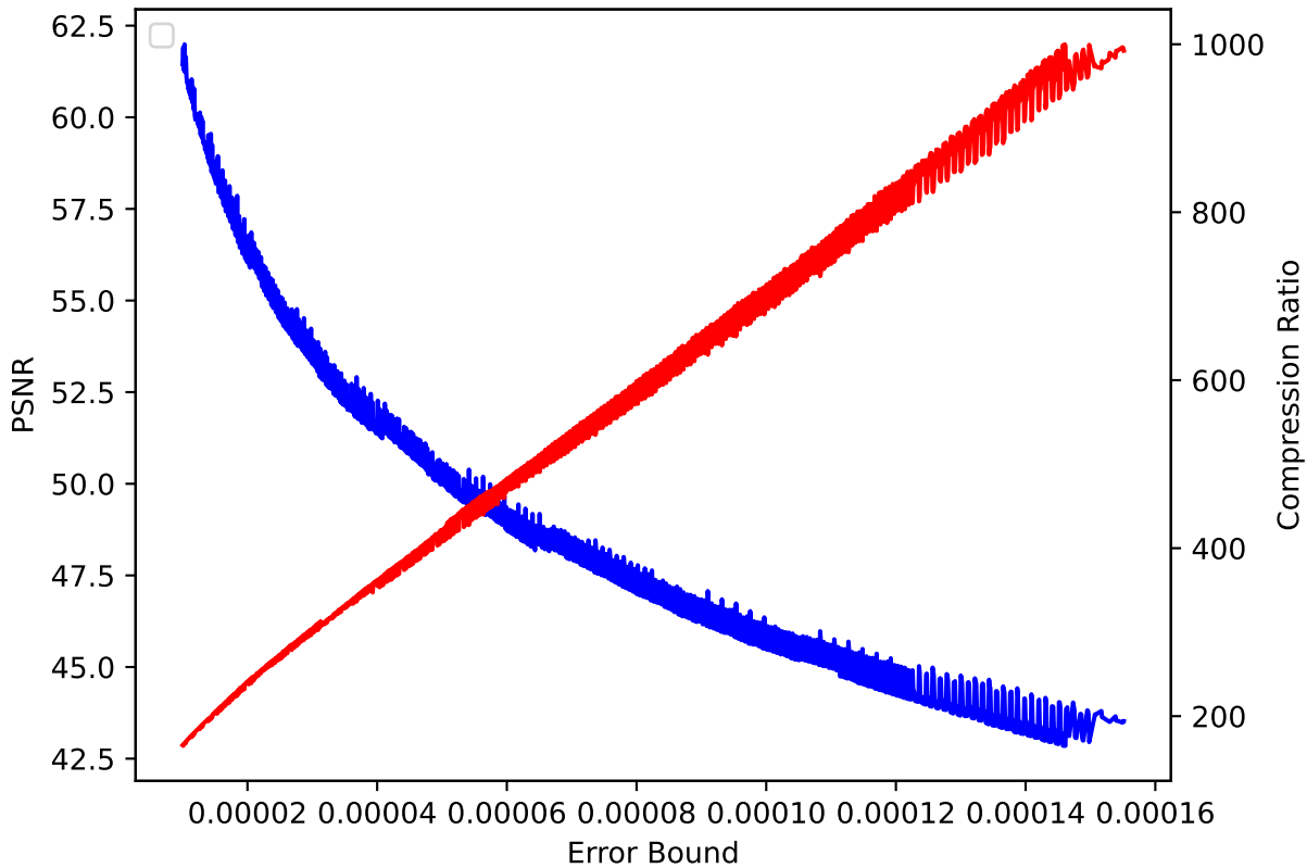
CLOUD 19 pressio:abs
