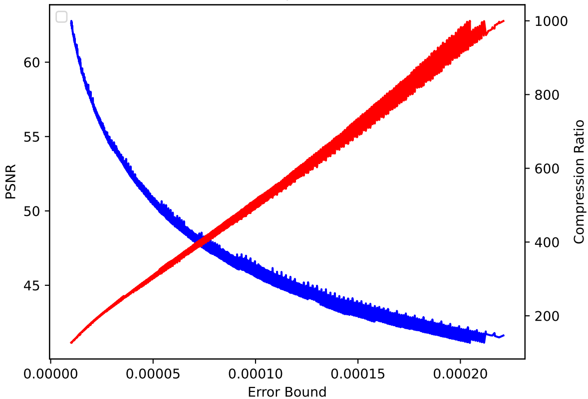
CLOUD 32 pressio:abs
