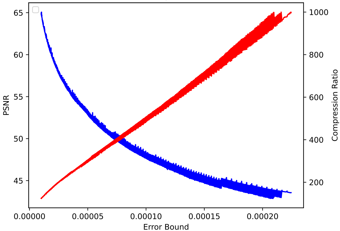
CLOUD 33 pressio:abs
