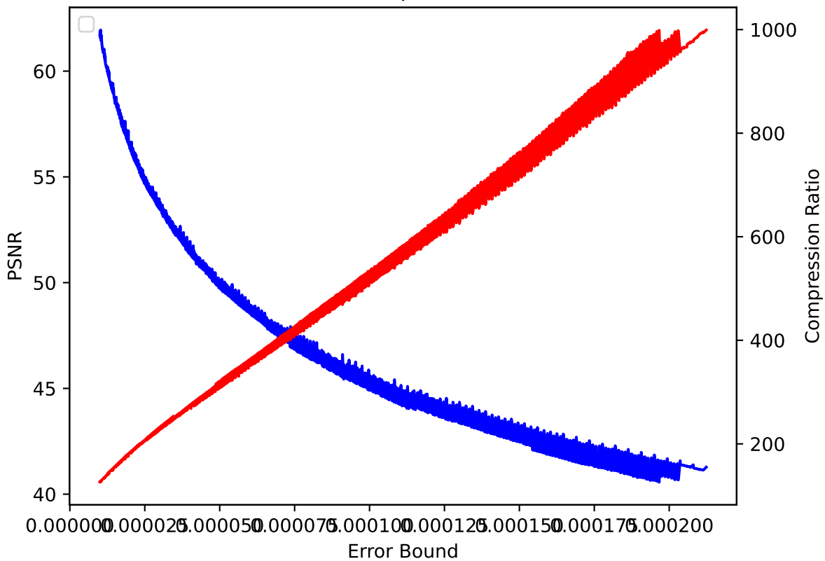
CLOUD 37 pressio:abs
