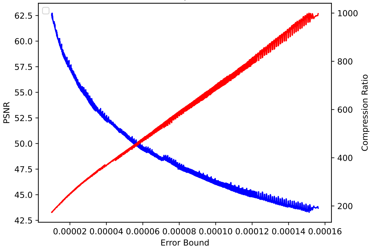
CLOUD 08 pressio:abs
