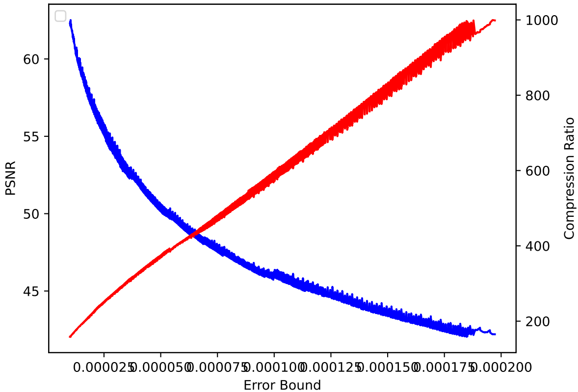
CLOUD 09 pressio:abs
