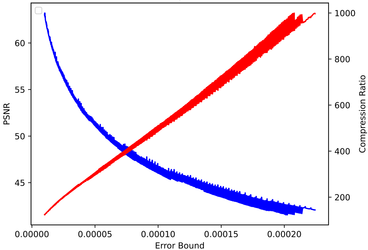
CLOUD 35 pressio:abs
