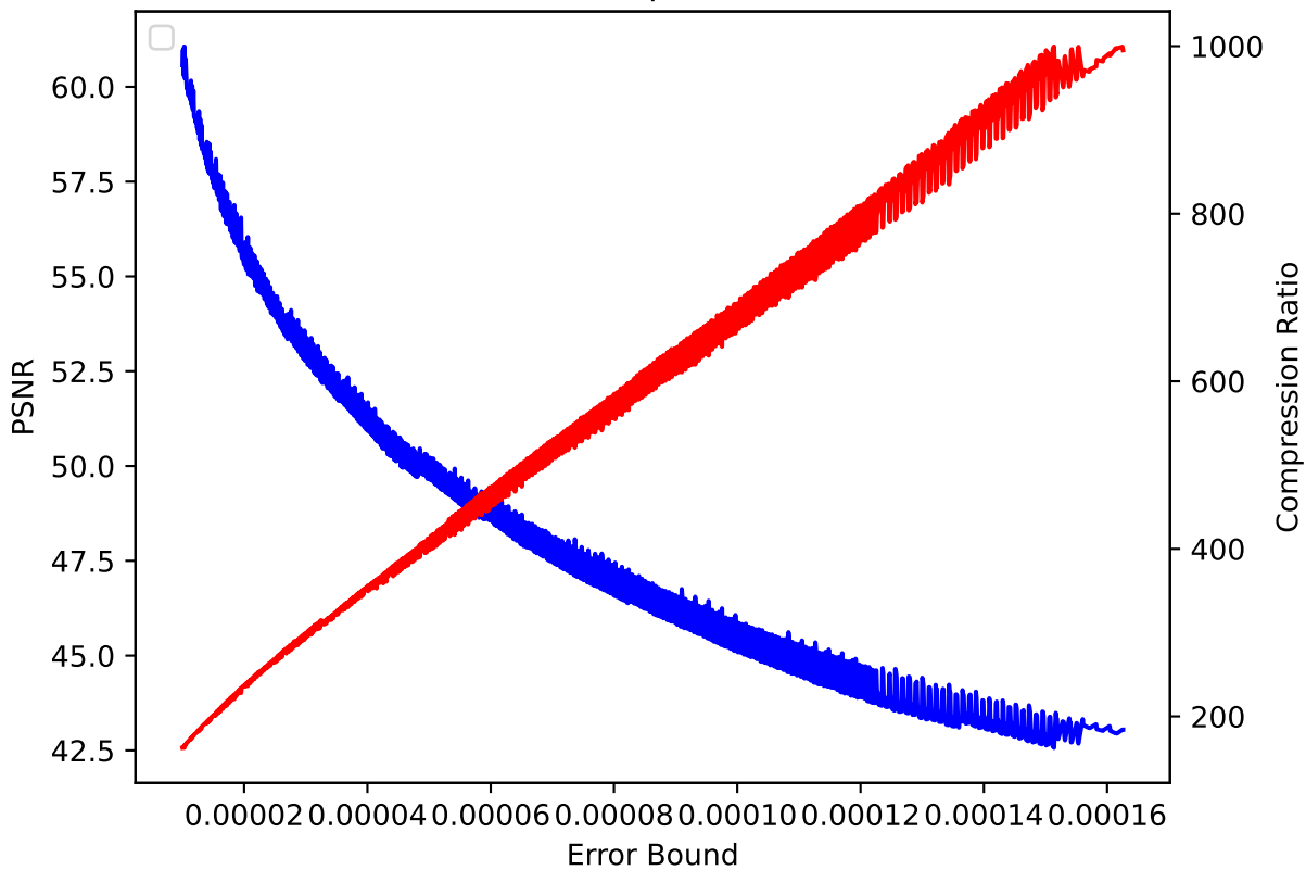
CLOUD 15 pressio:abs
