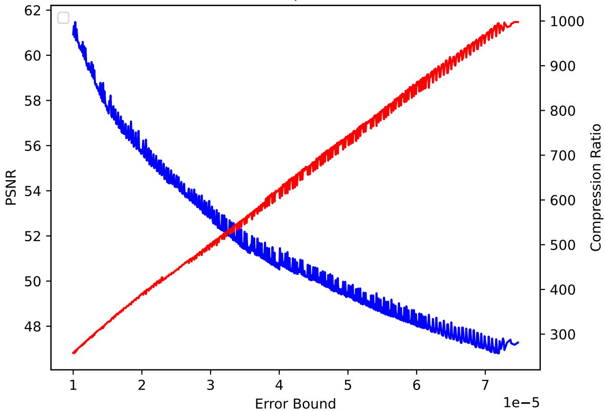
CLOUD 06 pressio:abs
