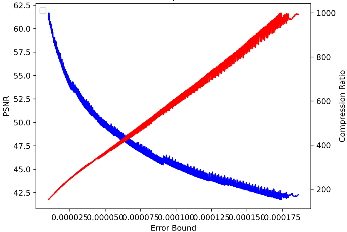
CLOUD 11 pressio:abs
