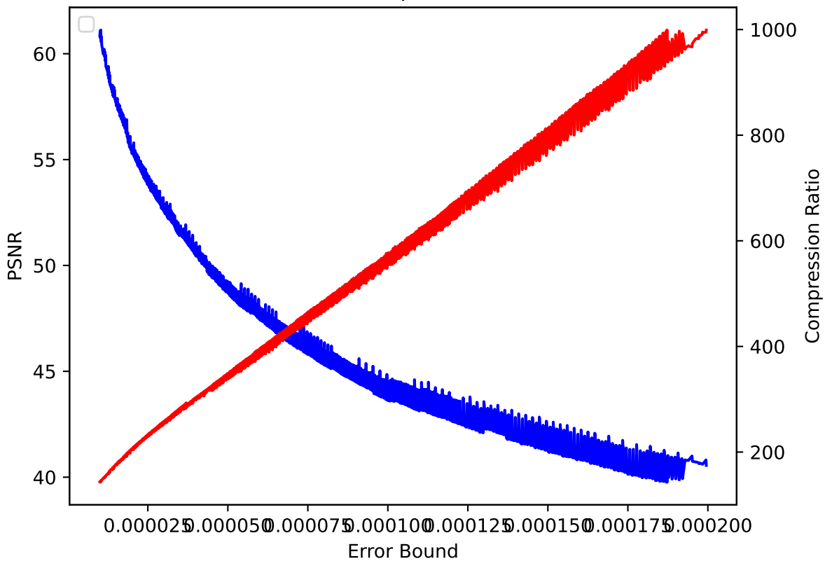
CLOUD 25 pressio:abs
