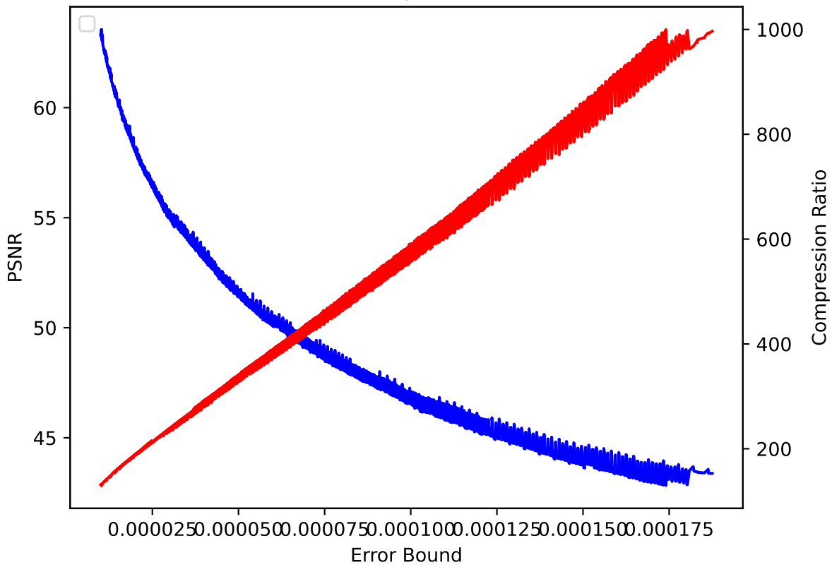
CLOUD 47 pressio:abs
