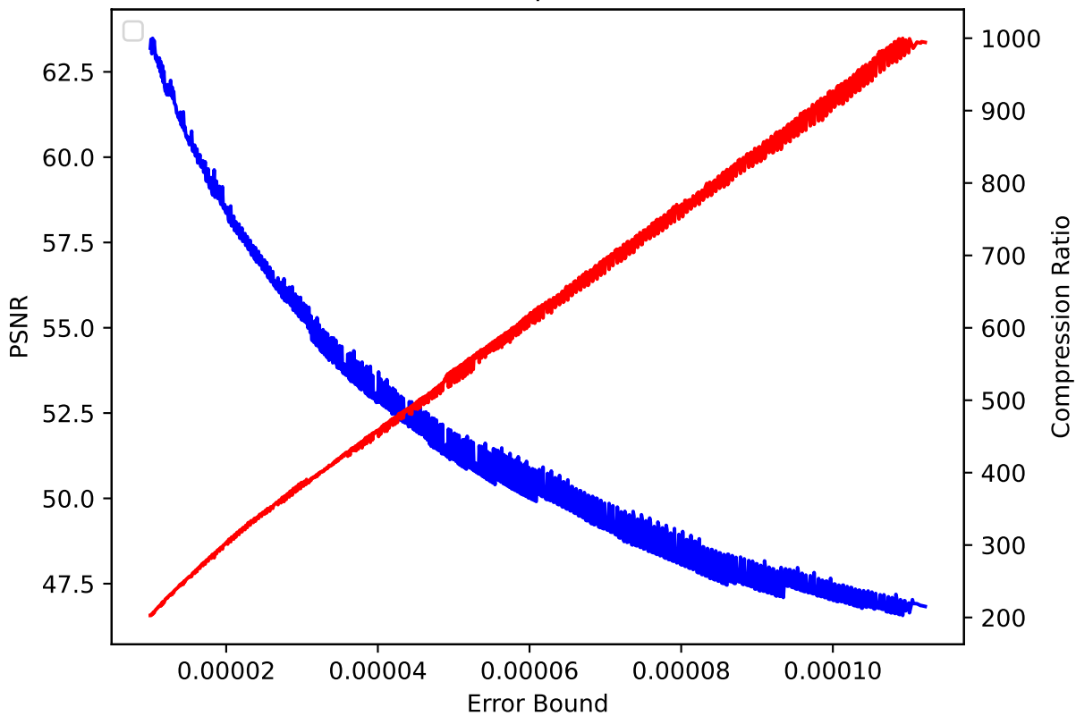
CLOUD 07 pressio:abs
