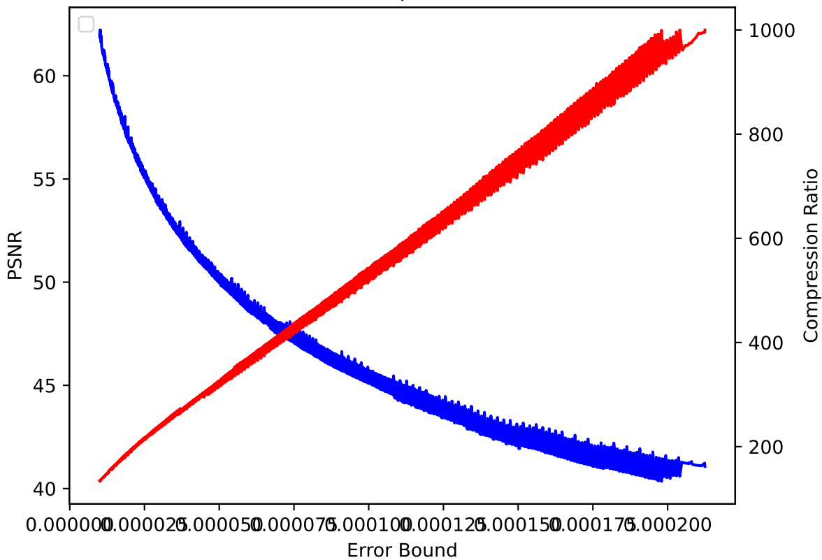
CLOUD 29 pressio:abs
