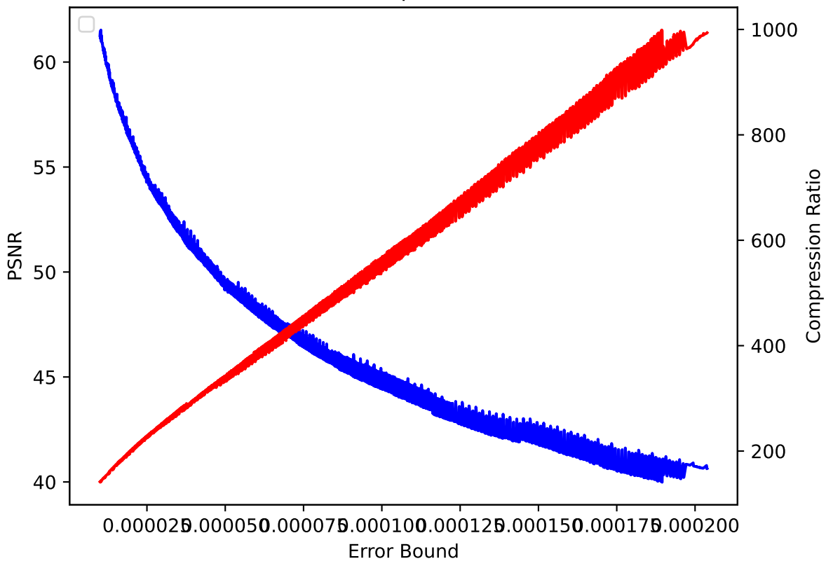
CLOUD 27 pressio:abs
