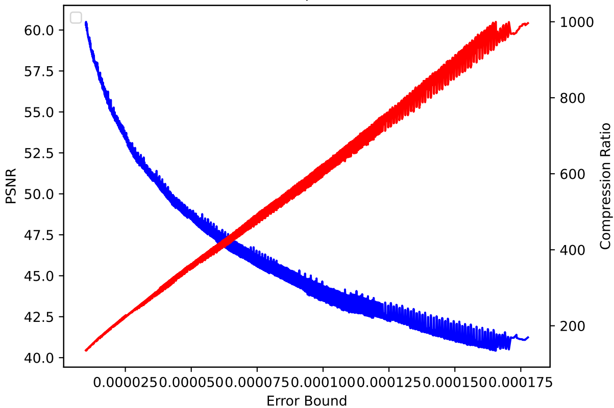
CLOUD 43 pressio:abs
