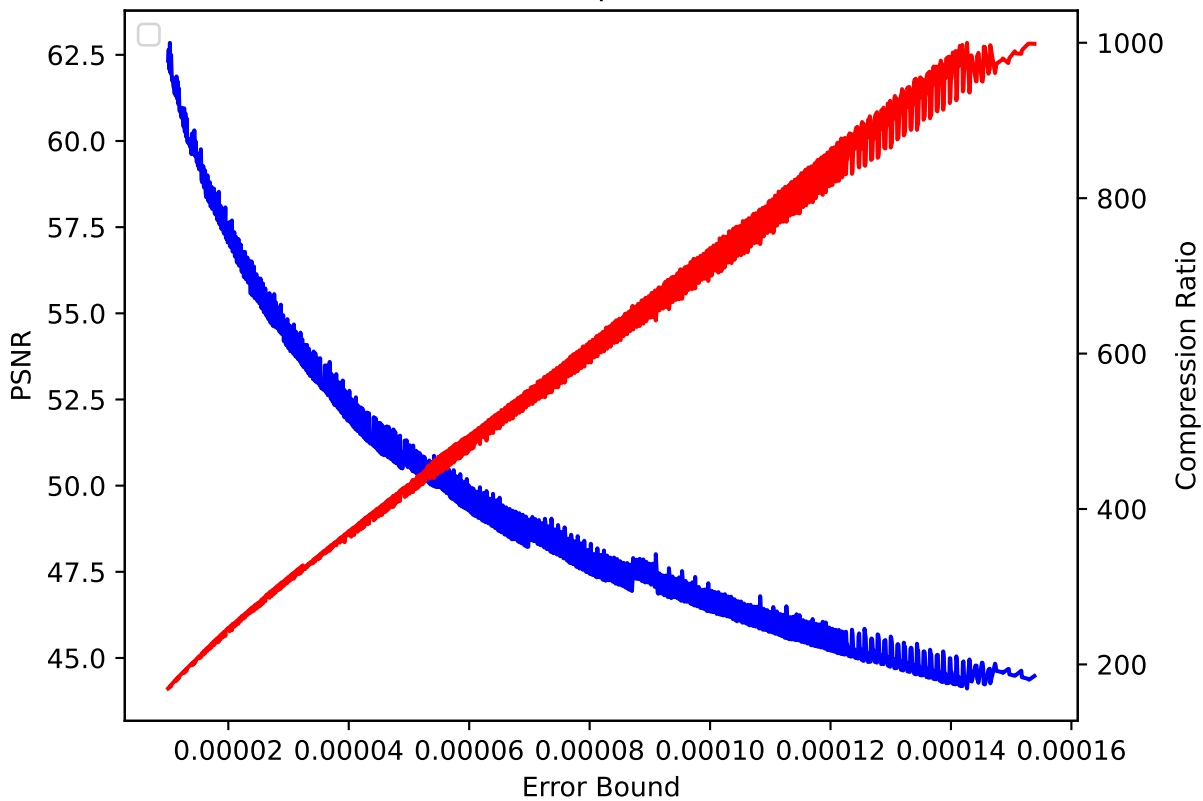
CLOUD 18 pressio:abs
