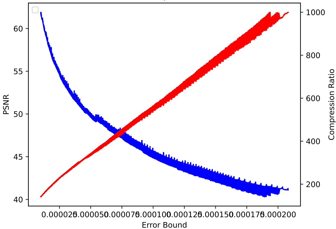
CLOUD 24 pressio:abs
