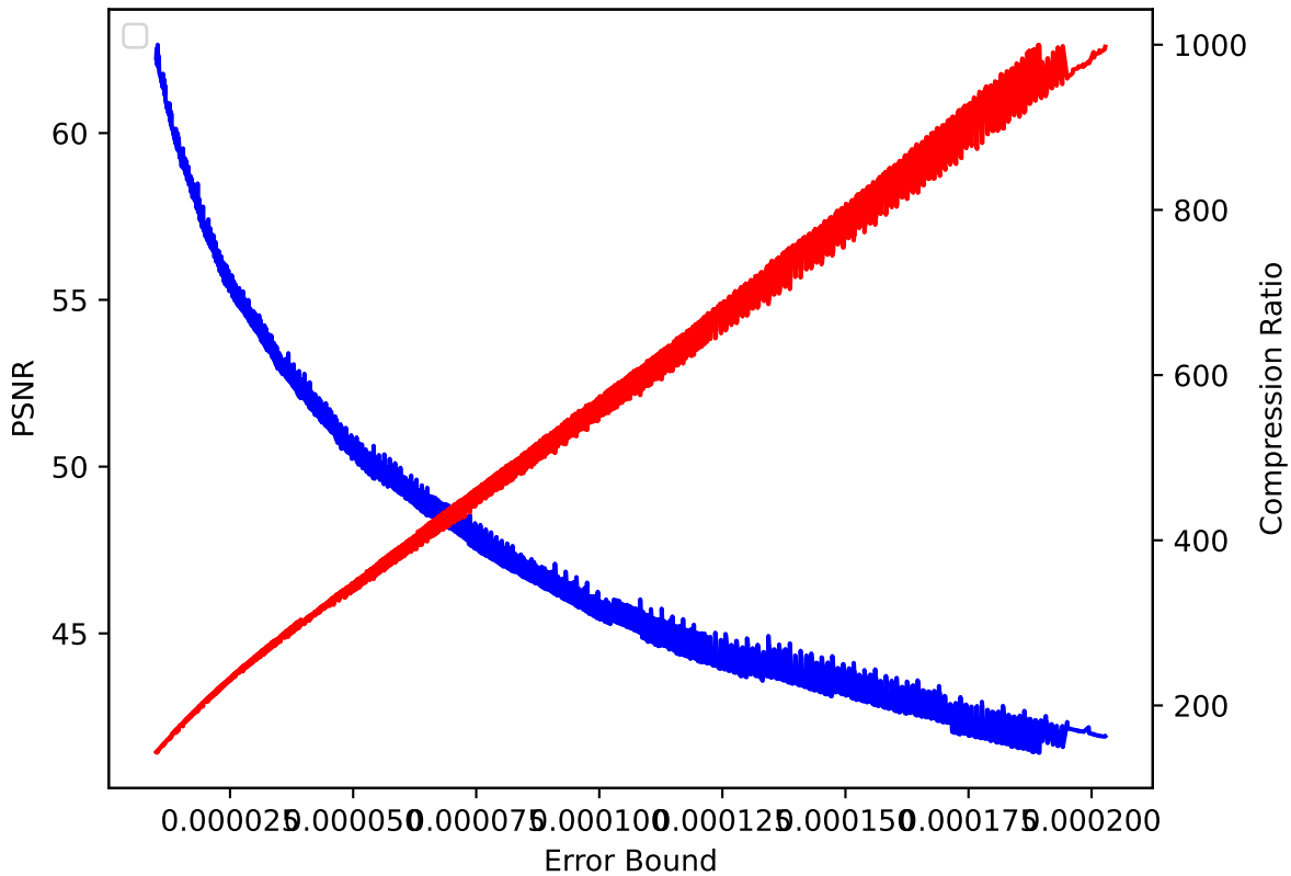
CLOUD 23 pressio:abs
