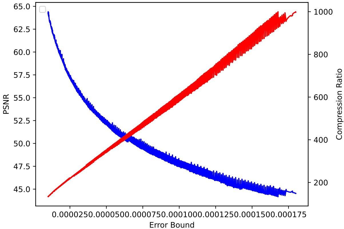
CLOUD 46 pressio:abs
