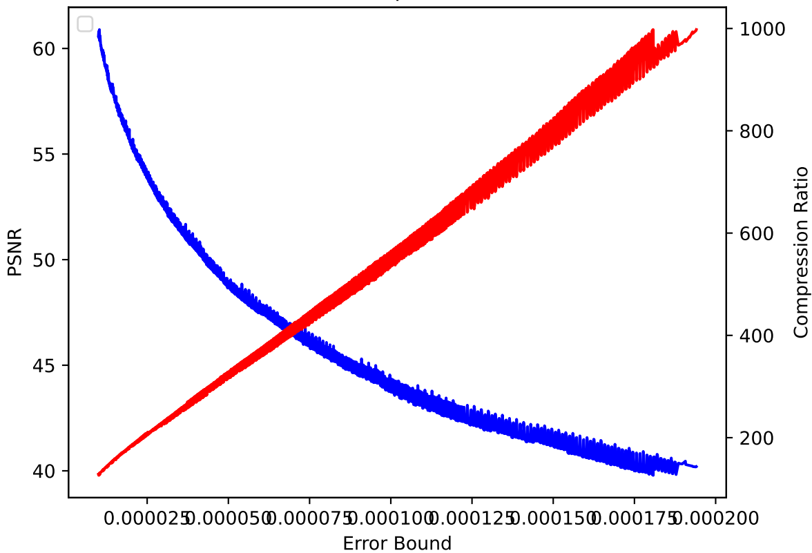
CLOUD 48 pressio:abs
