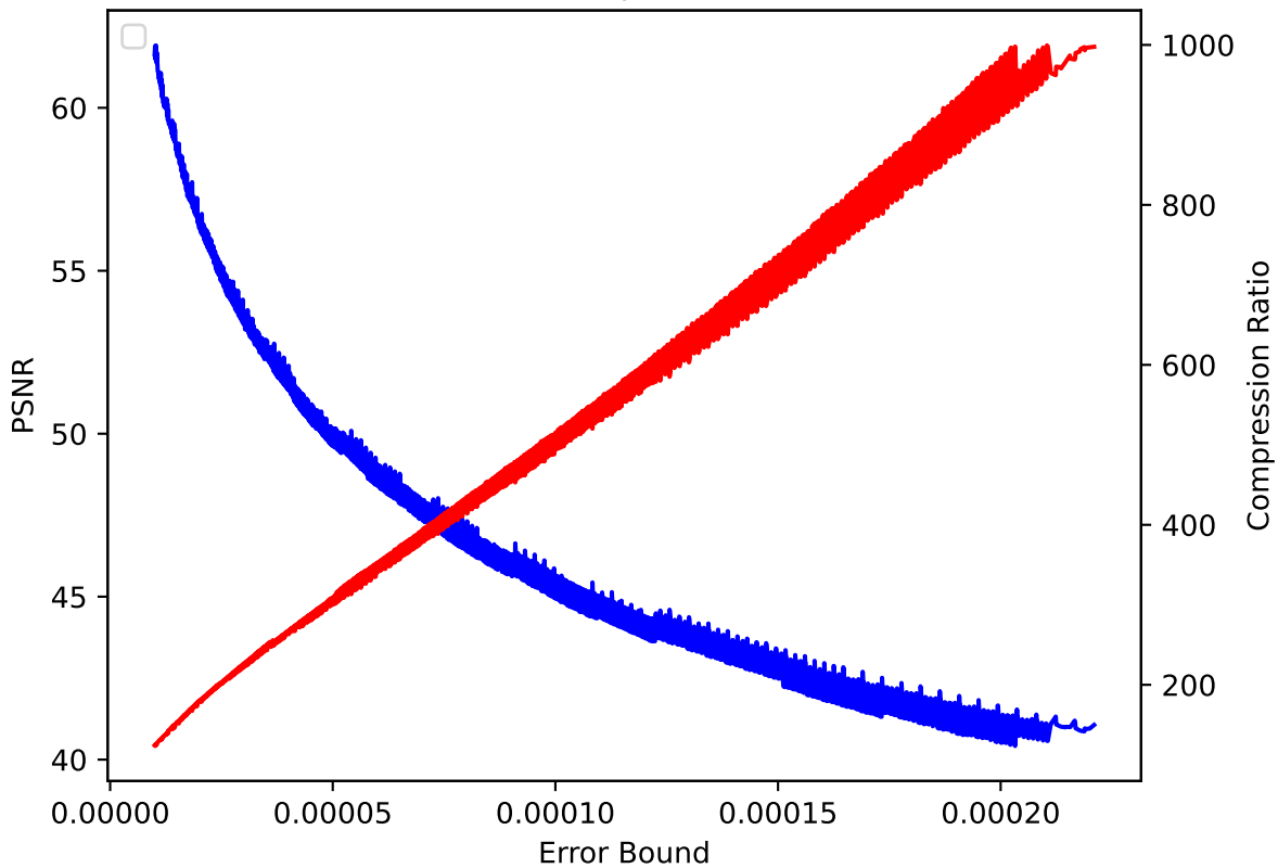
CLOUD 36 pressio:abs
