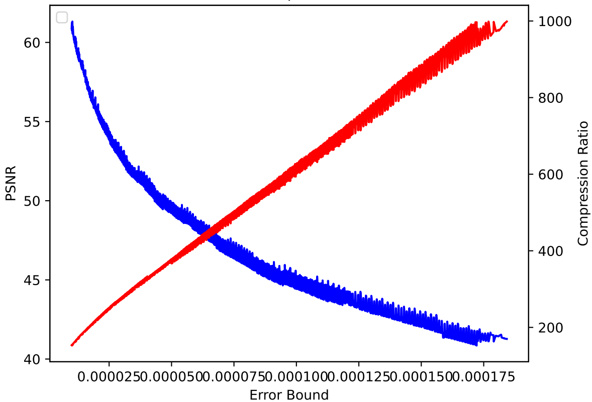
CLOUD 21 pressio:abs
