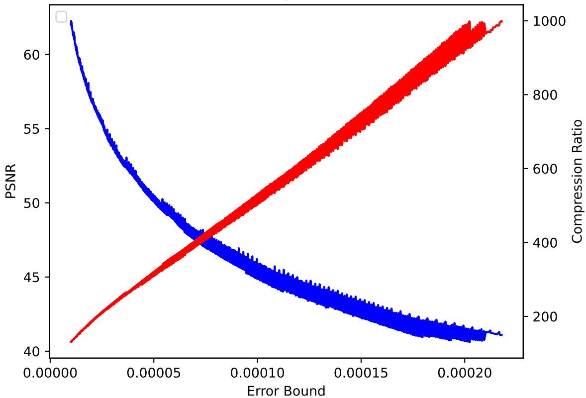
CLOUD 30 pressio:abs
