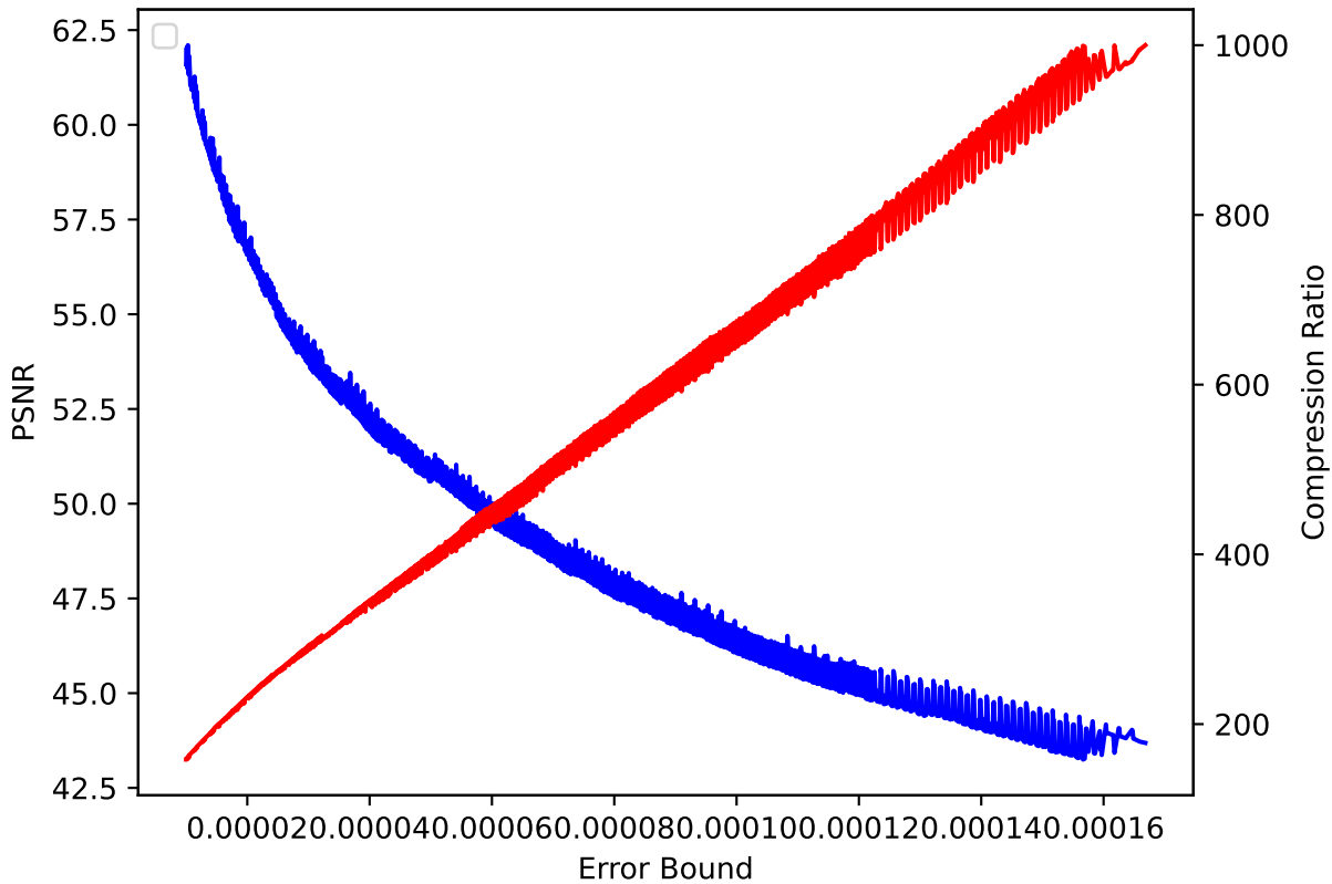
CLOUD 14 pressio:abs
