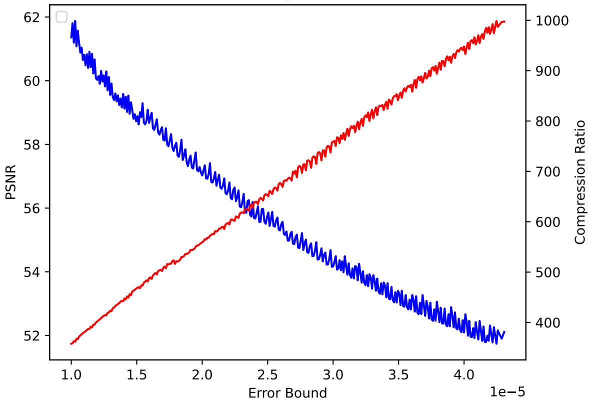
CLOUD 04 pressio:abs
