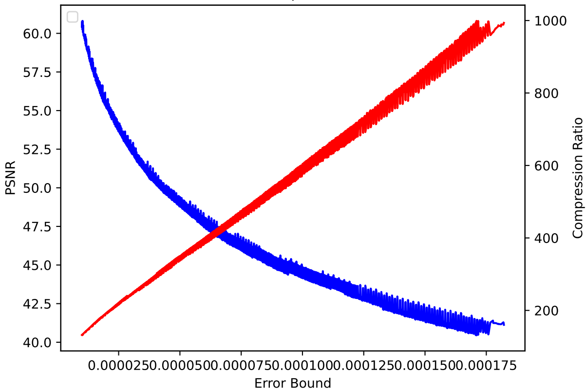
CLOUD 41 pressio:abs
