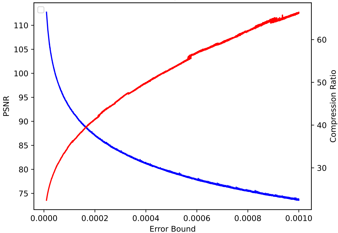
CLOUD 48 pressio:rel
