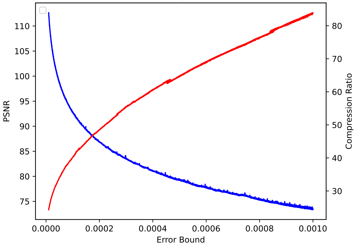
CLOUD 16 pressio:rel
