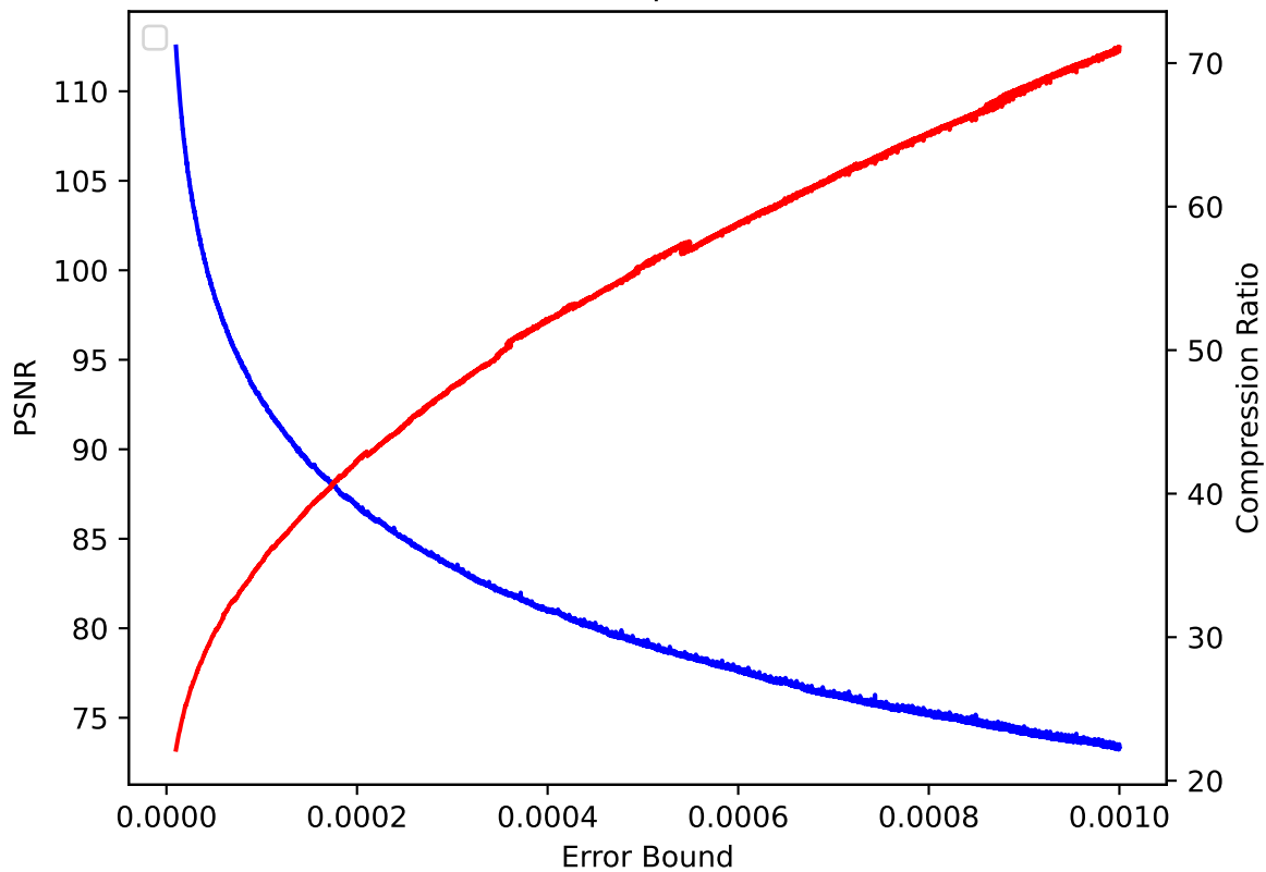
CLOUD 44 pressio:rel
