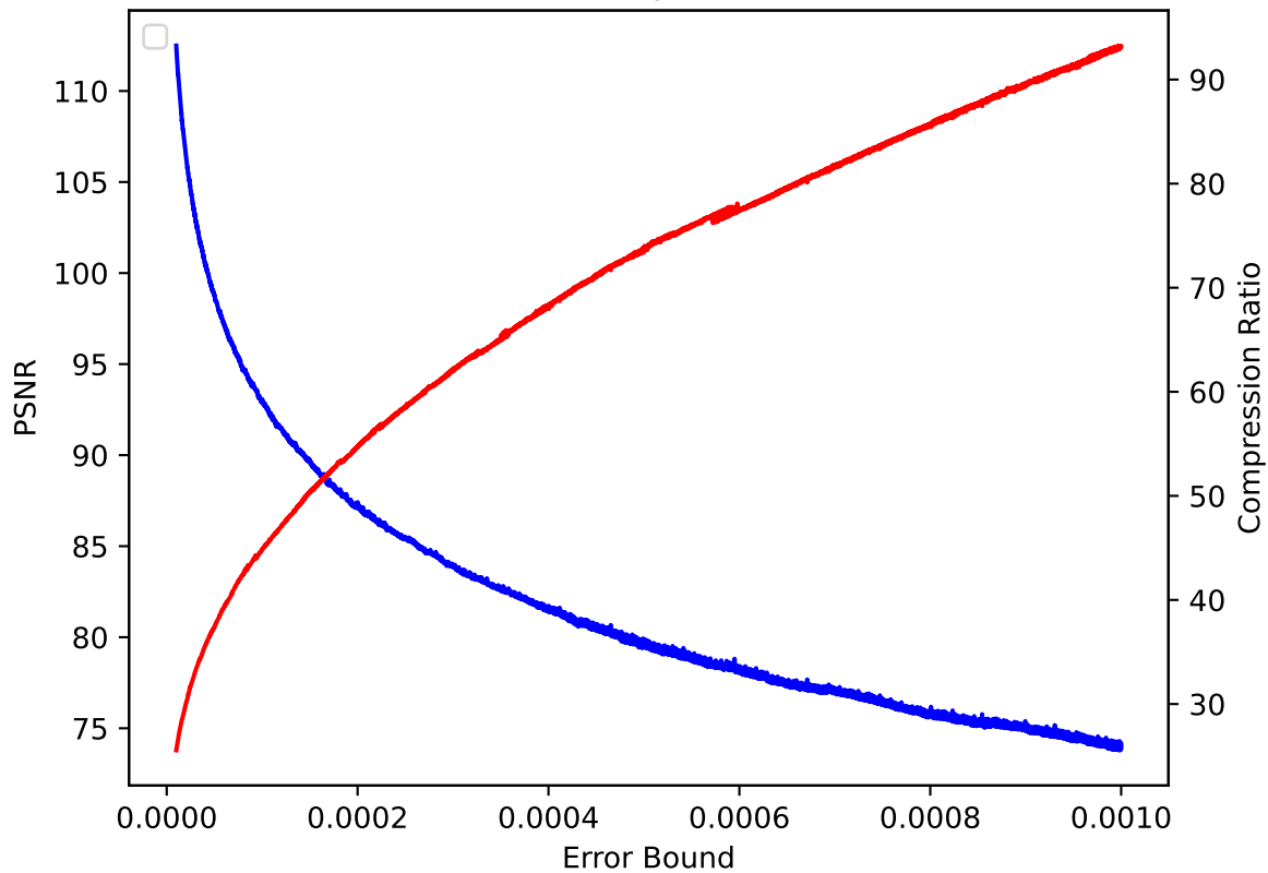
CLOUD 08 pressio:rel
