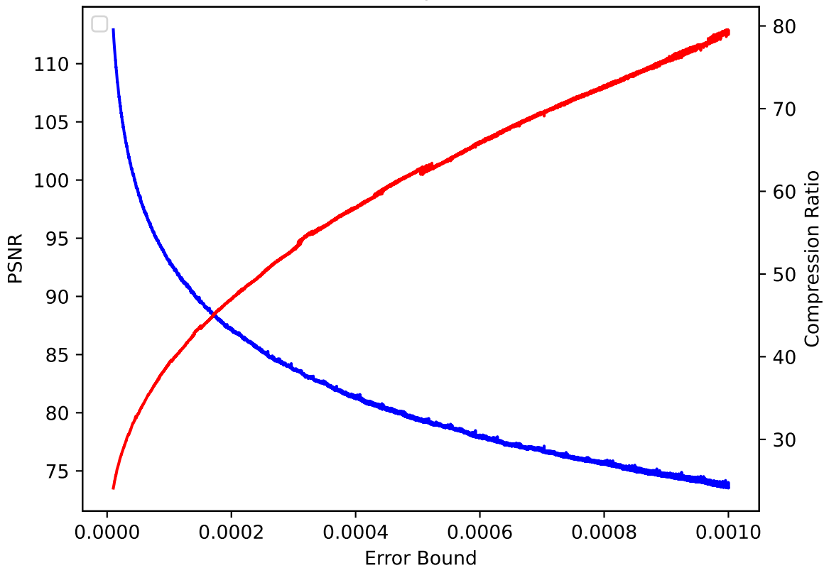
CLOUD 23 pressio:rel
