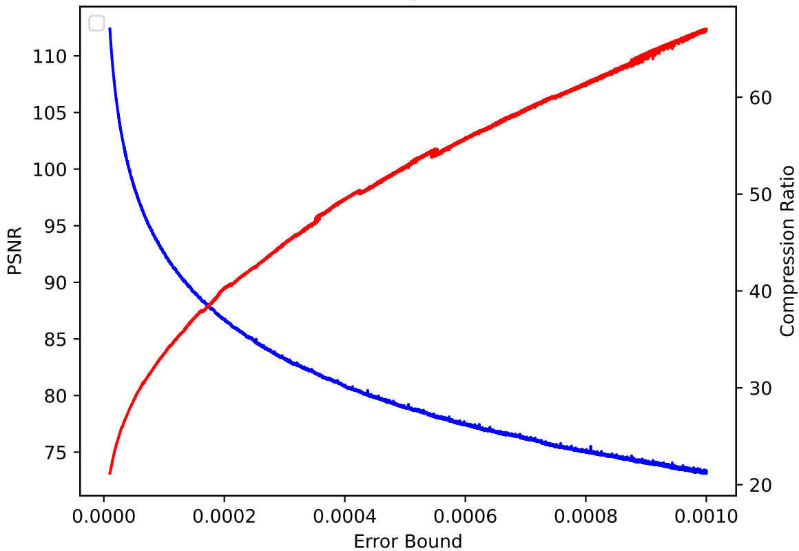
CLOUD 39 pressio:rel
