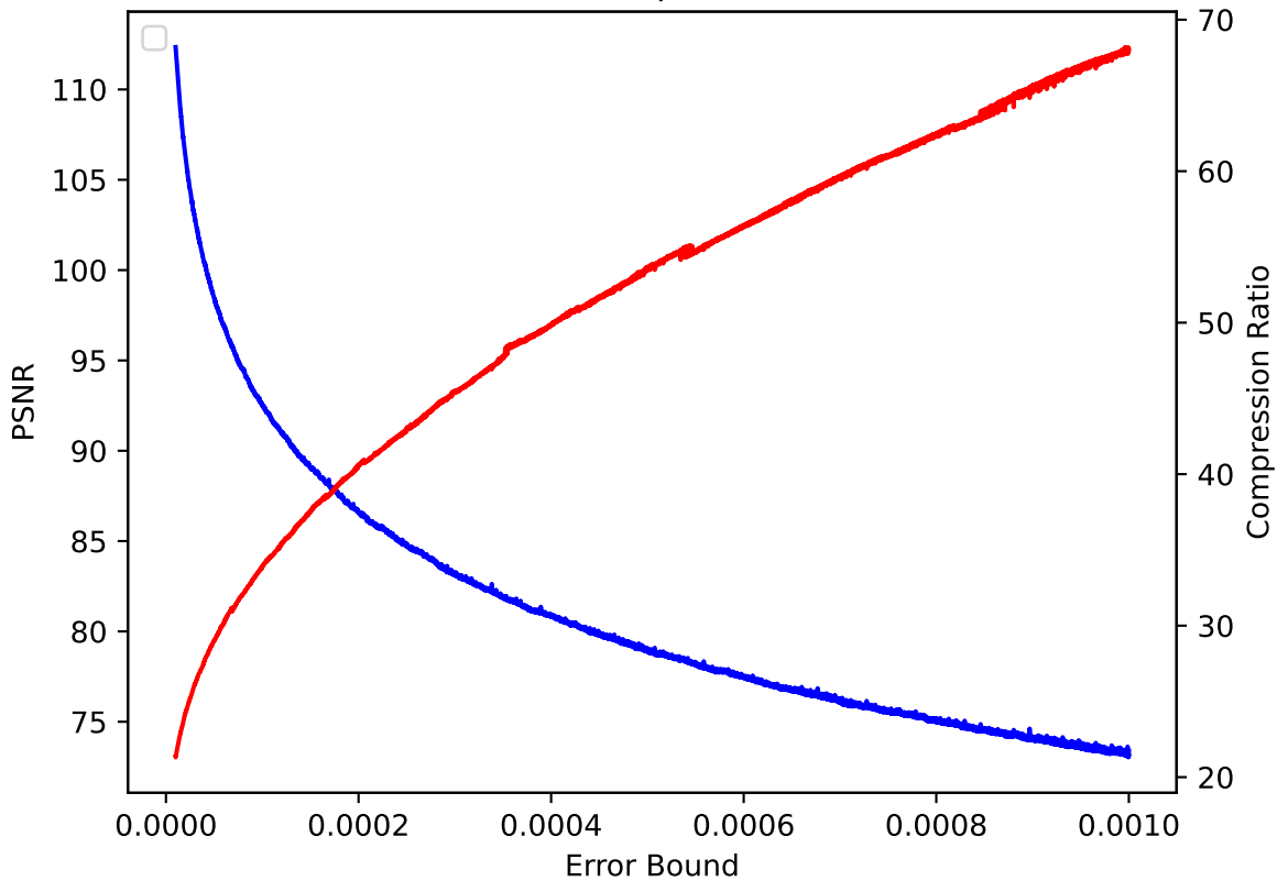
CLOUD 42 pressio:rel
