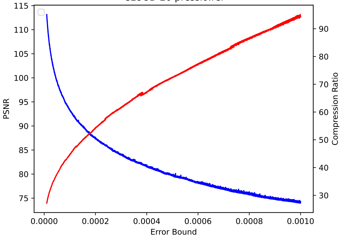
CLOUD 20 pressio:rel
