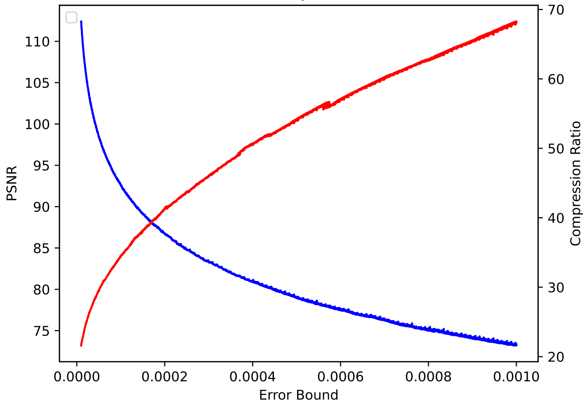
CLOUD 36 pressio:rel
