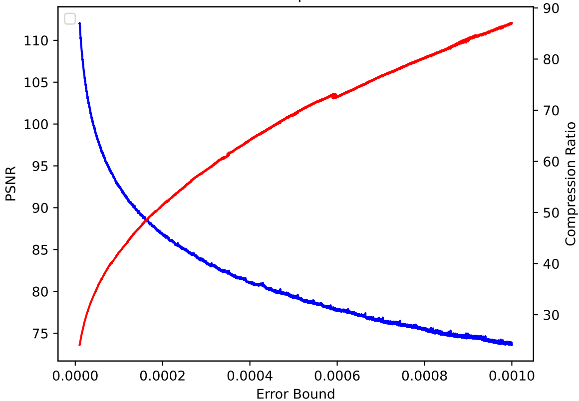
CLOUD 09 pressio:rel
