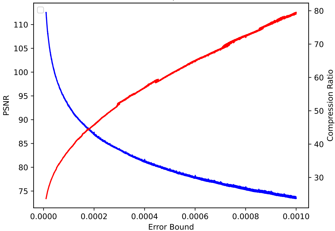
CLOUD 46 pressio:rel
