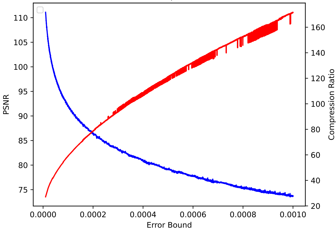
CLOUD 02 pressio:rel
