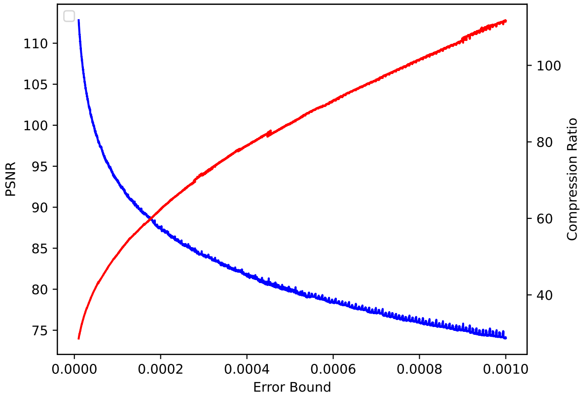
CLOUD 06 pressio:rel
