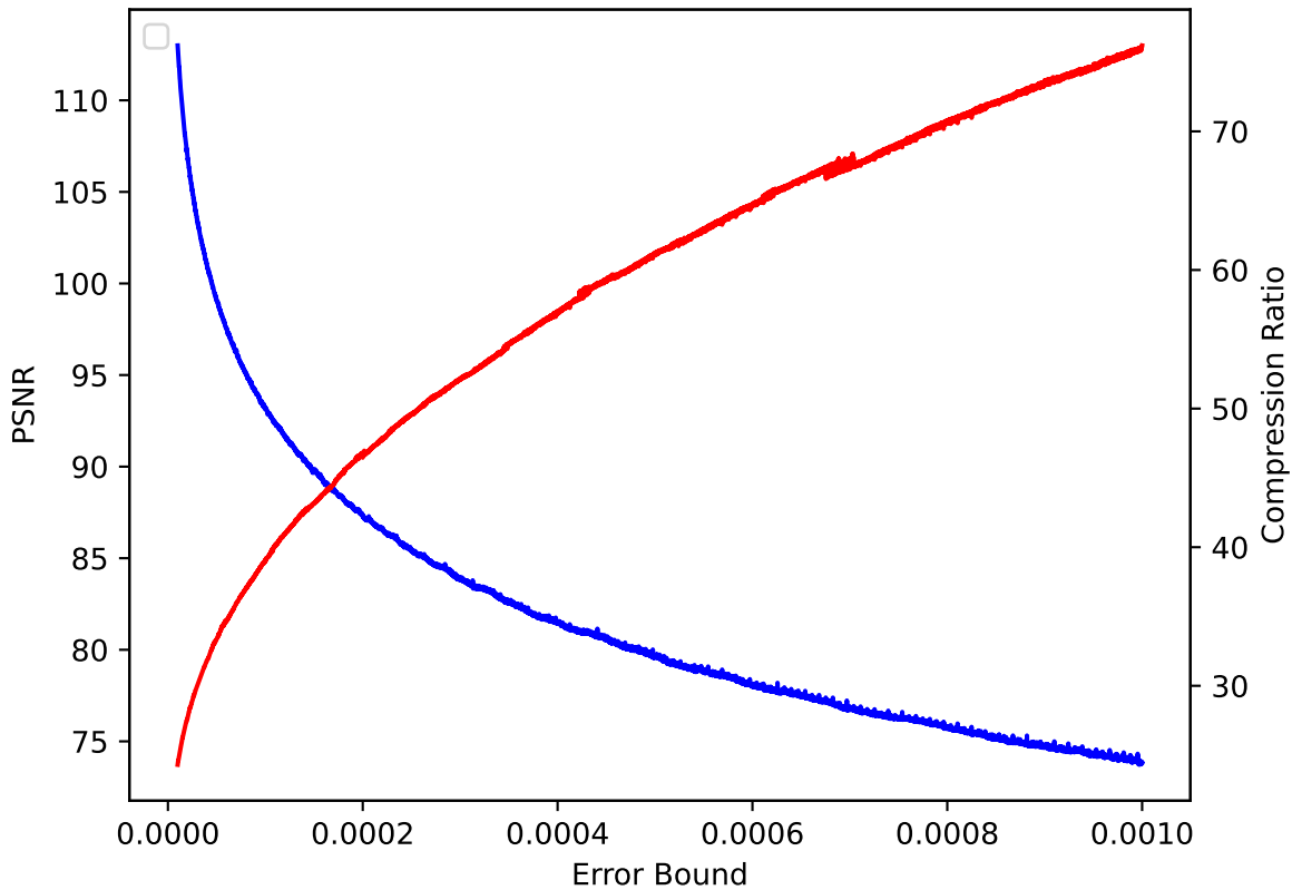
CLOUD 26 pressio:rel
