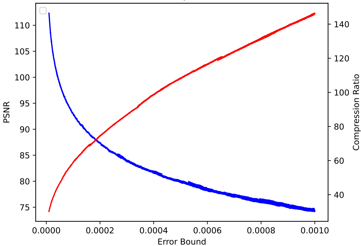
CLOUD 04 pressio:rel
