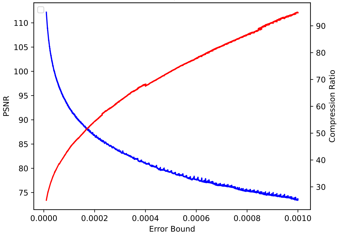
CLOUD 10 pressio:rel
