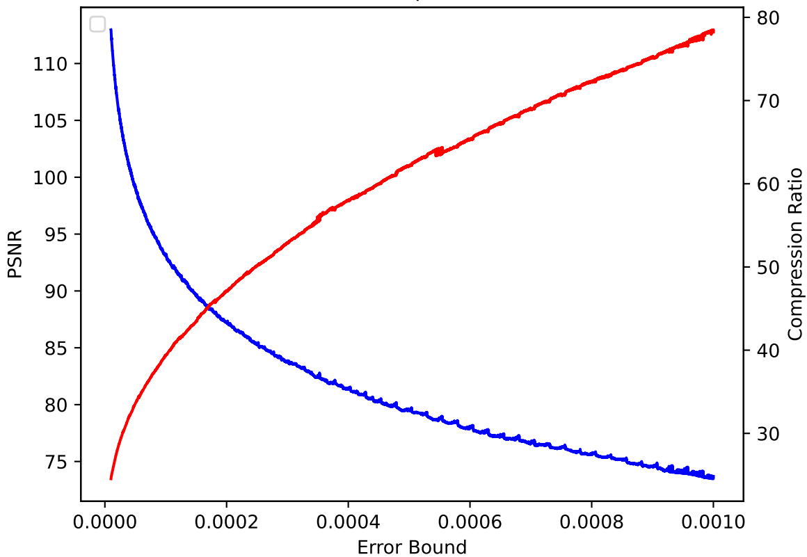
CLOUD 21 pressio:rel
