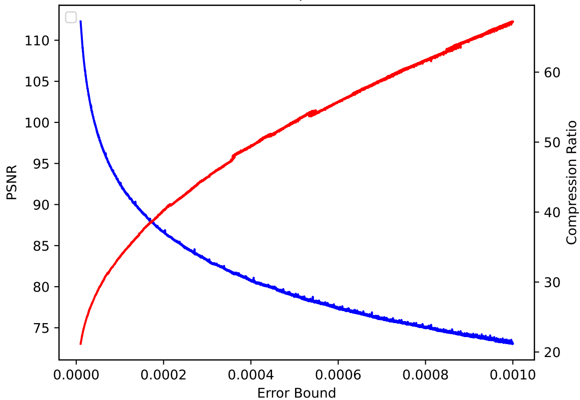
CLOUD 41 pressio:rel
