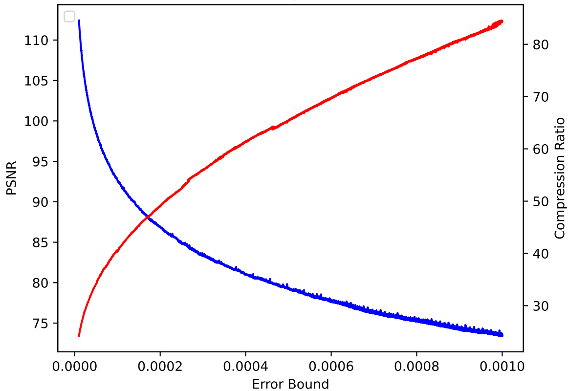
CLOUD 13 pressio:rel
