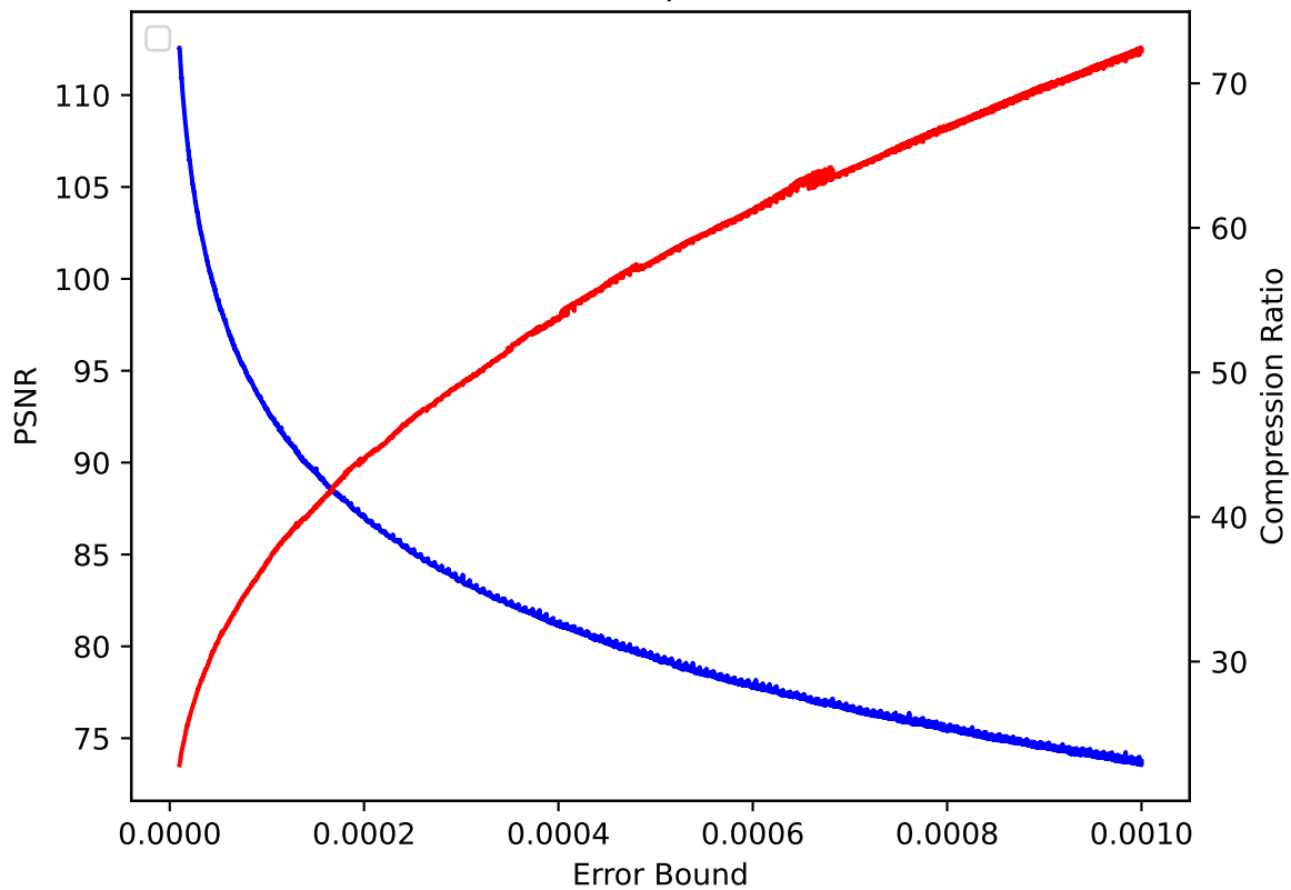
CLOUD 32 pressio:rel
