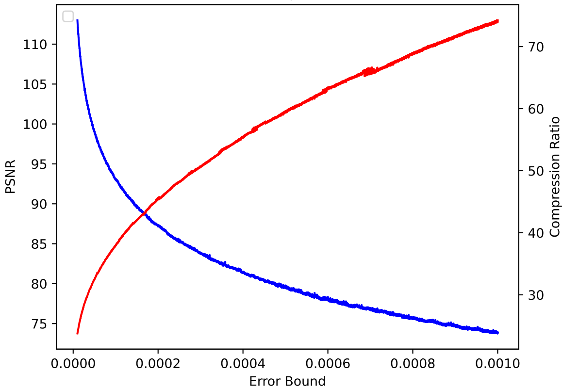
CLOUD 25 pressio:rel
