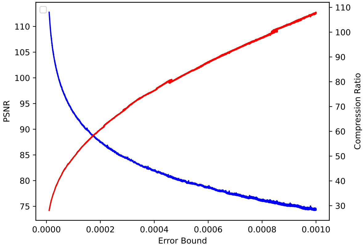
CLOUD 07 pressio:rel
