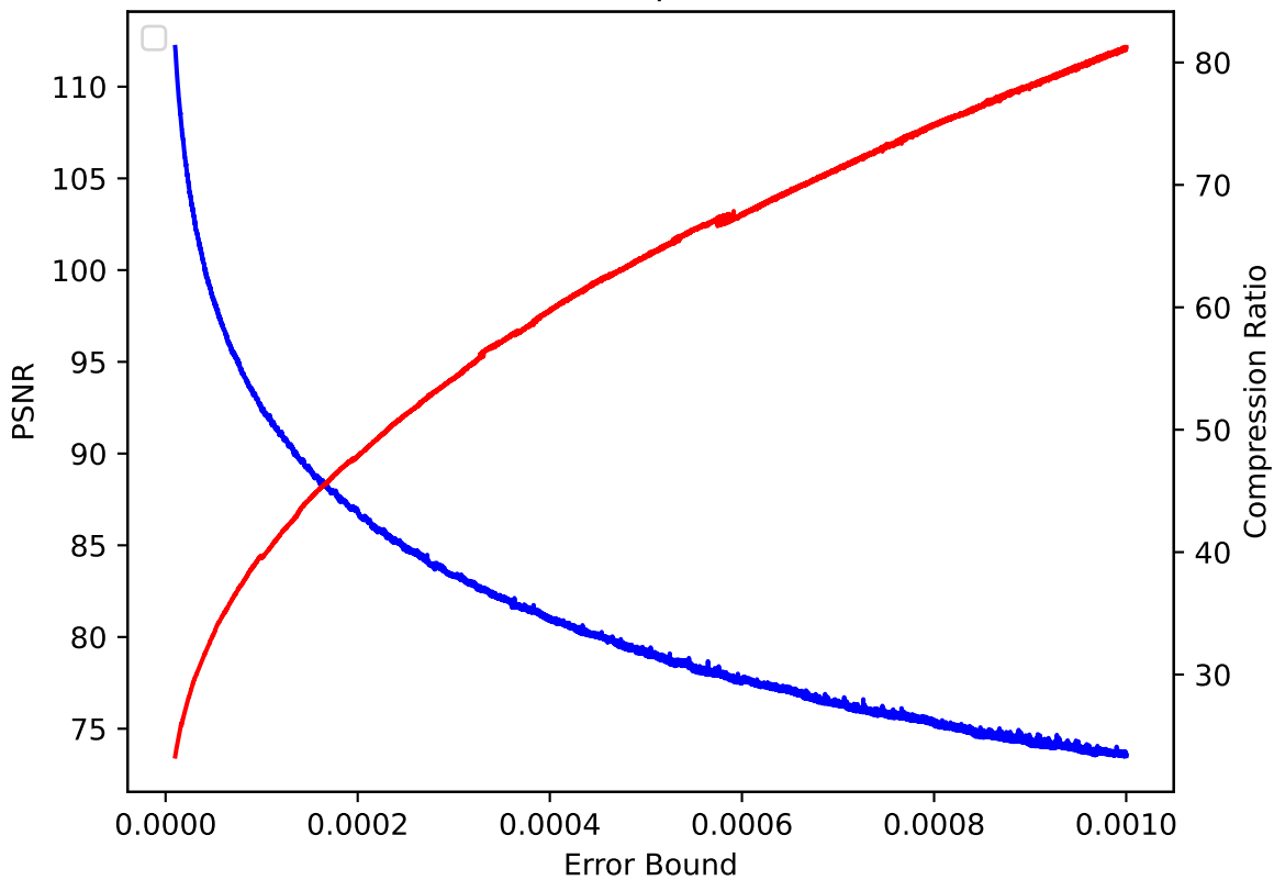
CLOUD 11 pressio:rel
