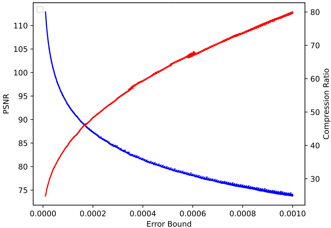
CLOUD 28 pressio:rel
