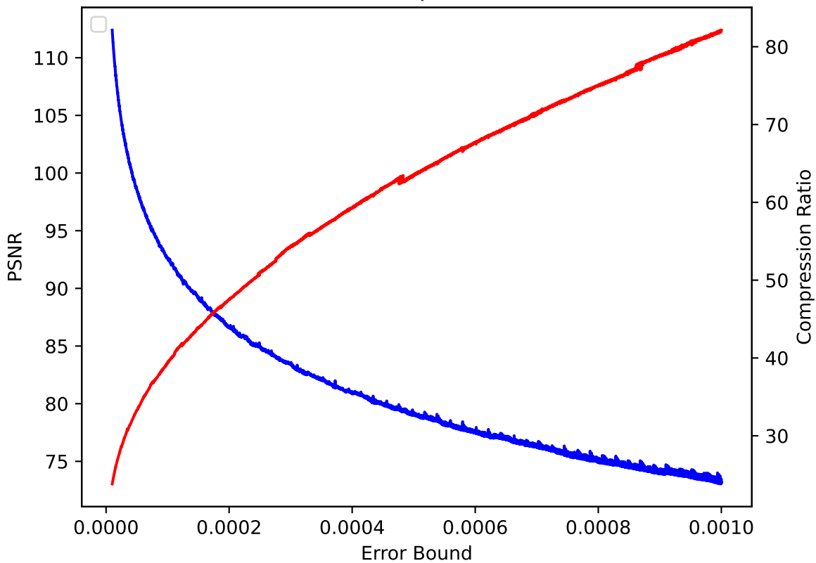
CLOUD 15 pressio:rel
