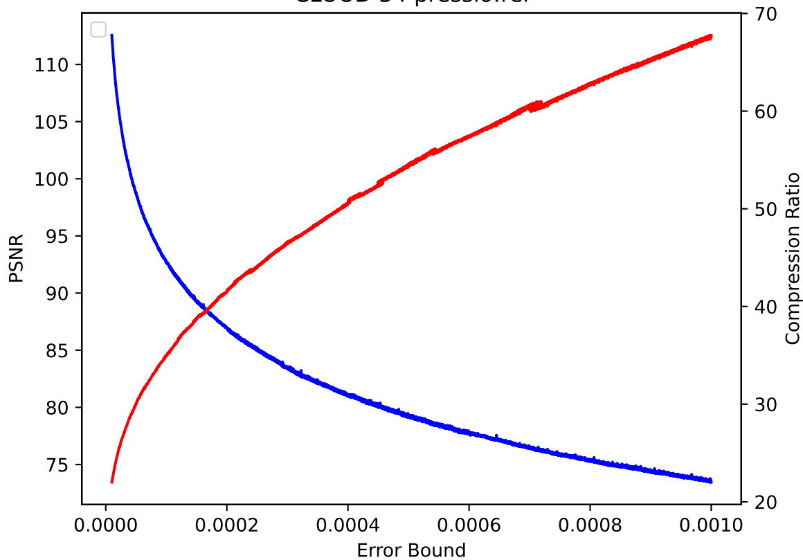
CLOUD 34 pressio:rel
