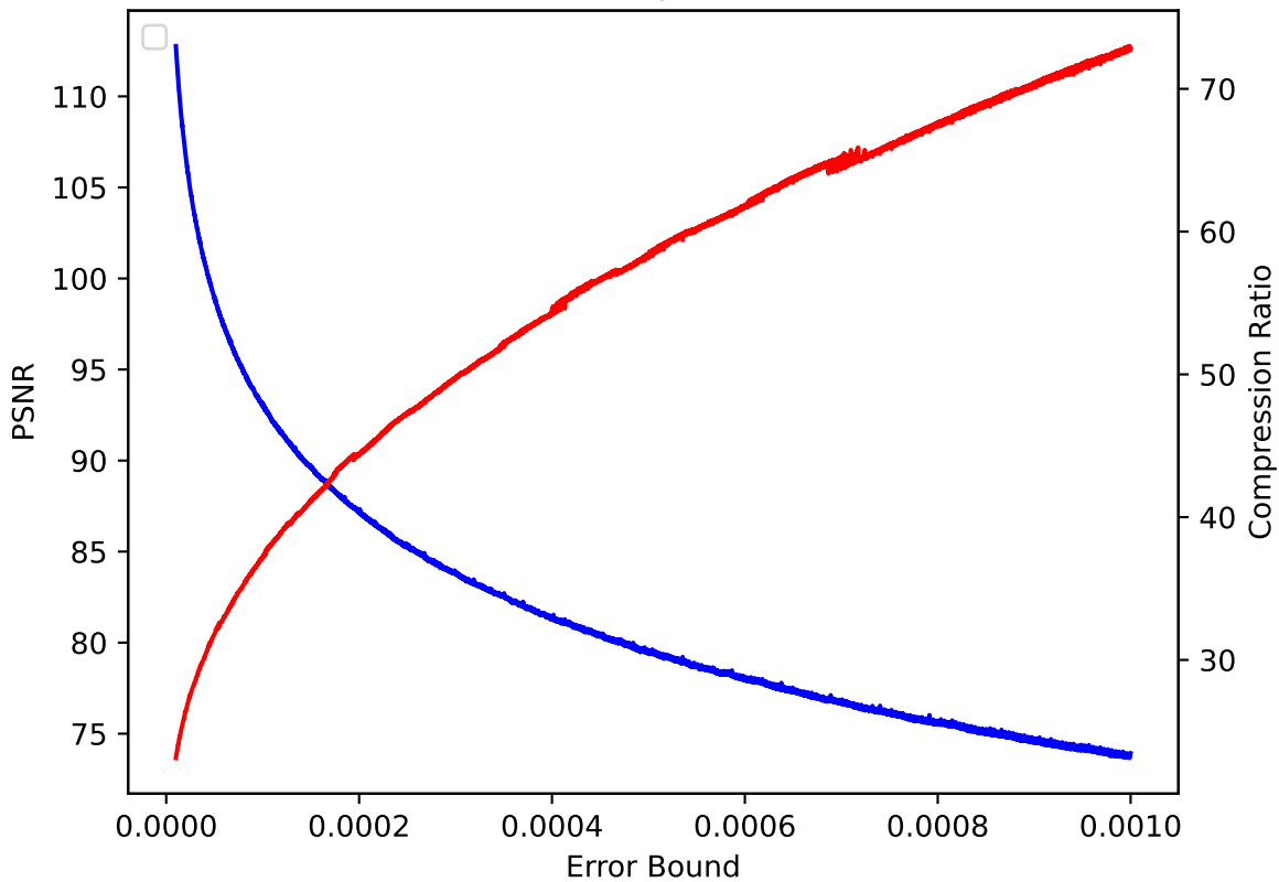
CLOUD 30 pressio:rel
