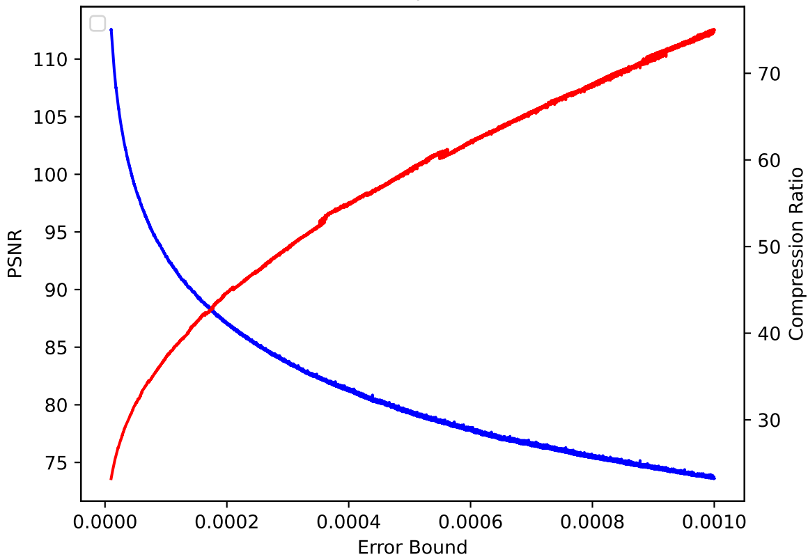
CLOUD 47 pressio:rel
