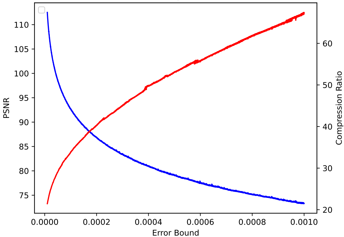
CLOUD 43 pressio:rel
