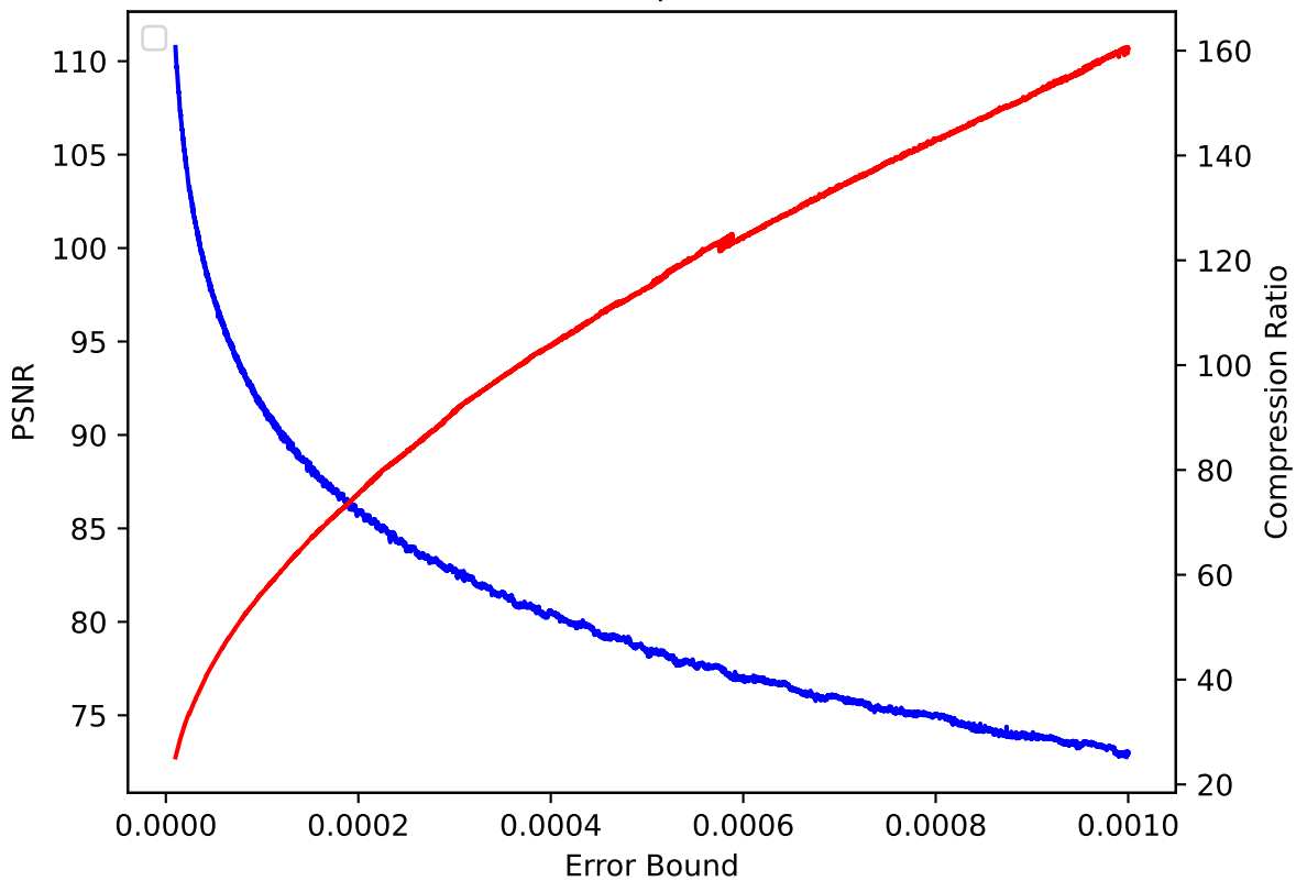
CLOUD 01 pressio:rel
