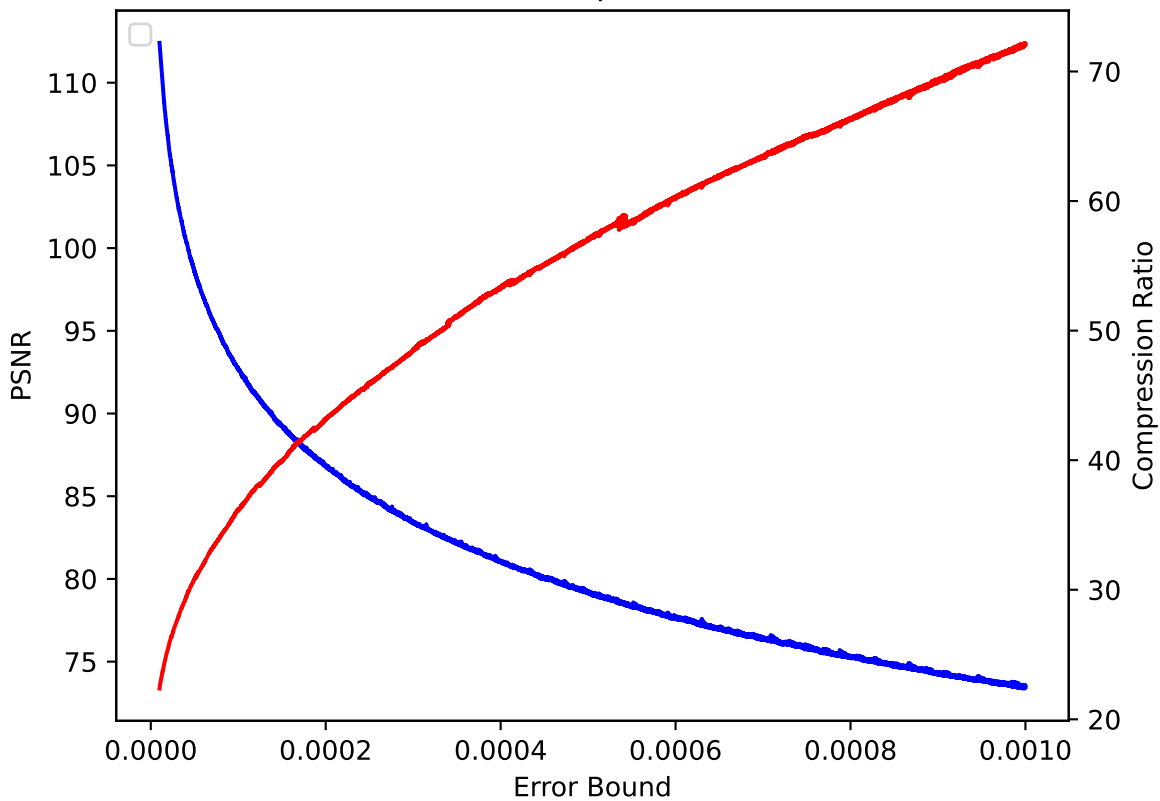
CLOUD 35 pressio:rel
