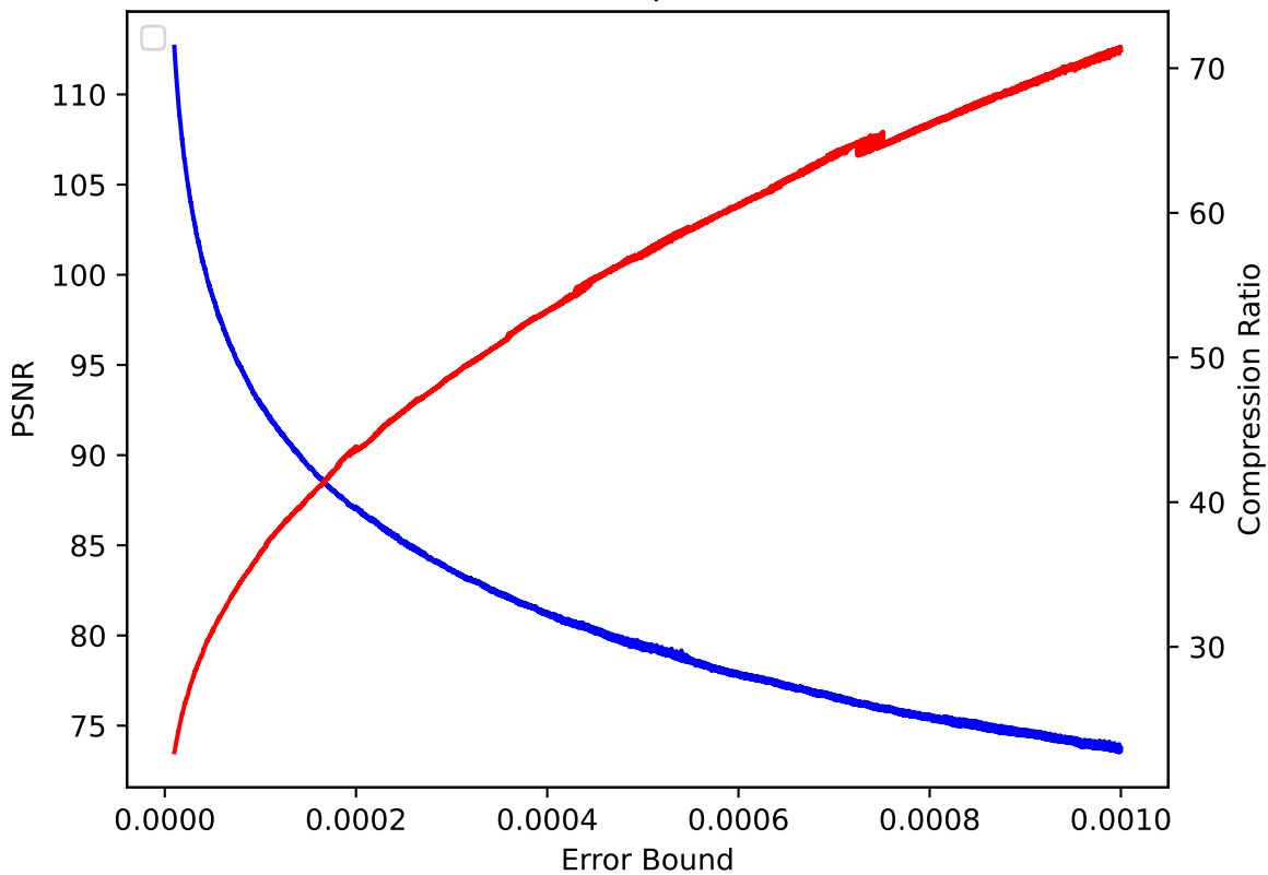
CLOUD 31 pressio:rel
