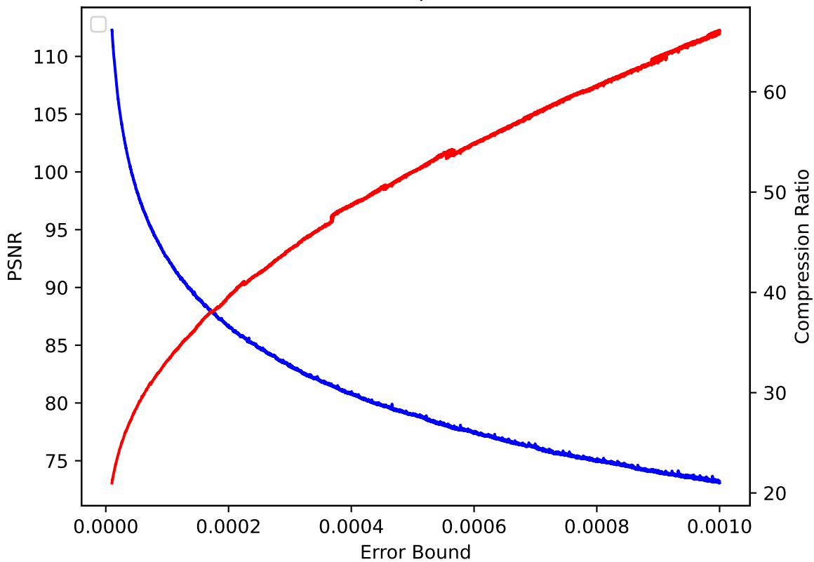
CLOUD 40 pressio:rel
