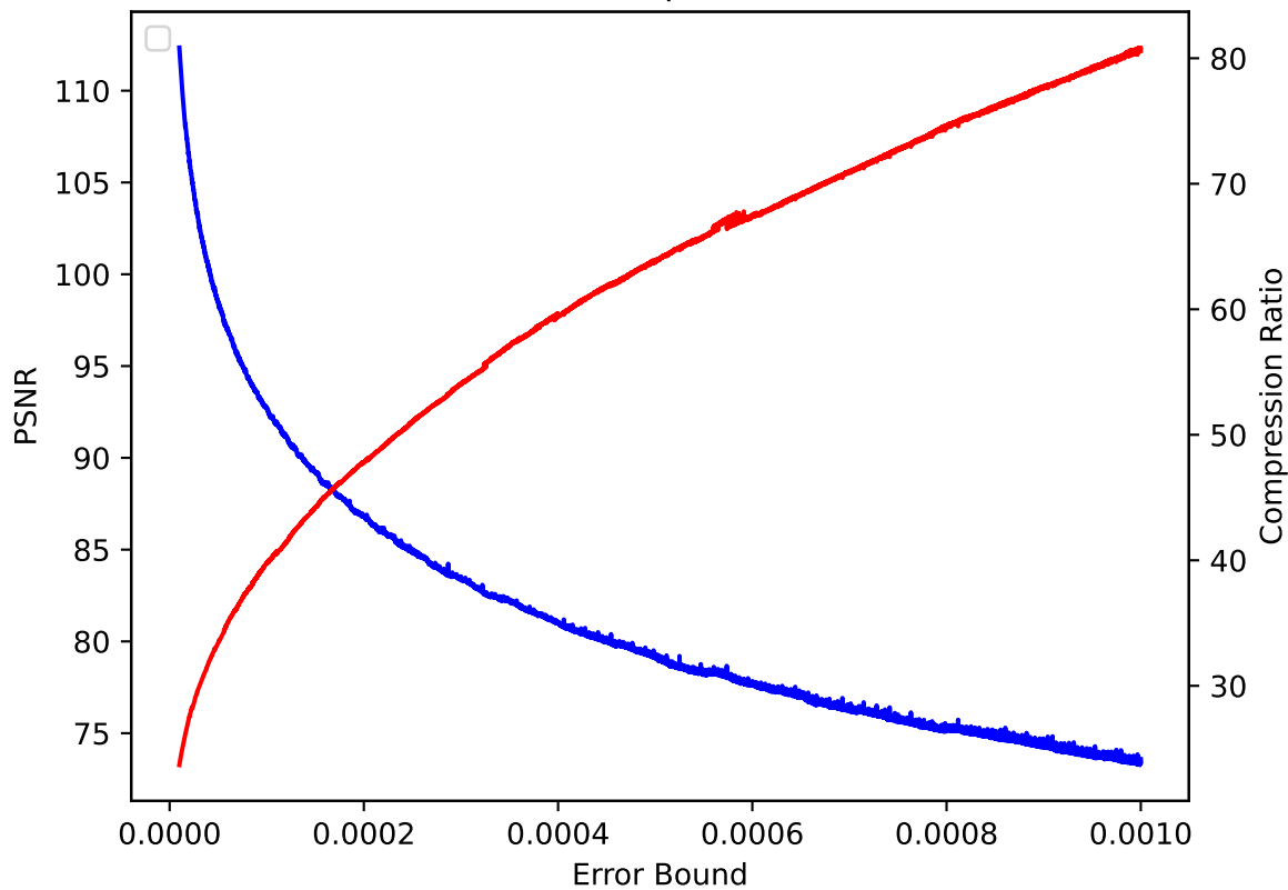
CLOUD 12 pressio:rel
