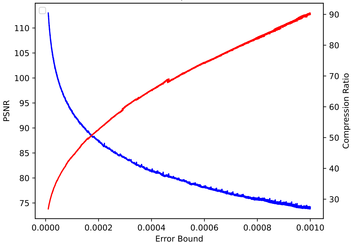
CLOUD 18 pressio:rel
