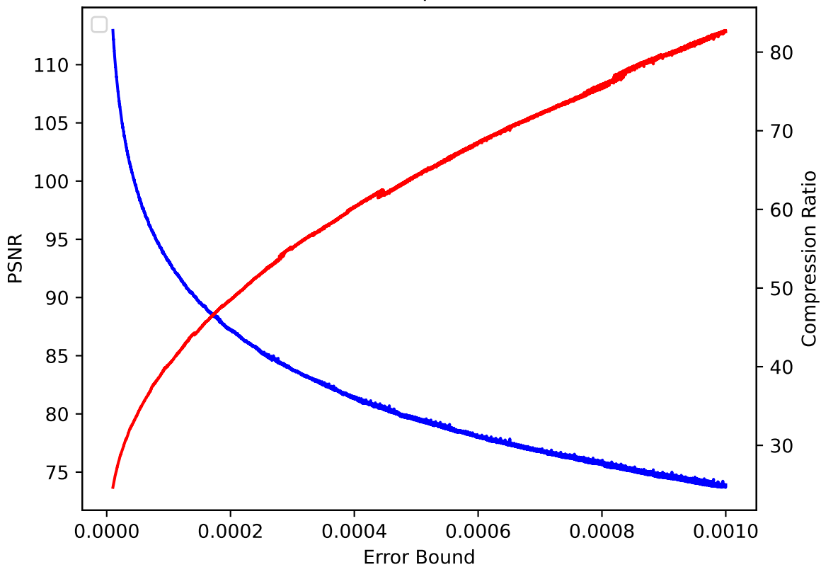
CLOUD 22 pressio:rel
