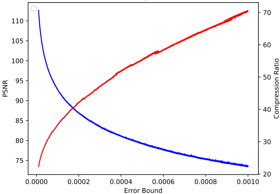
CLOUD 45 pressio:rel
