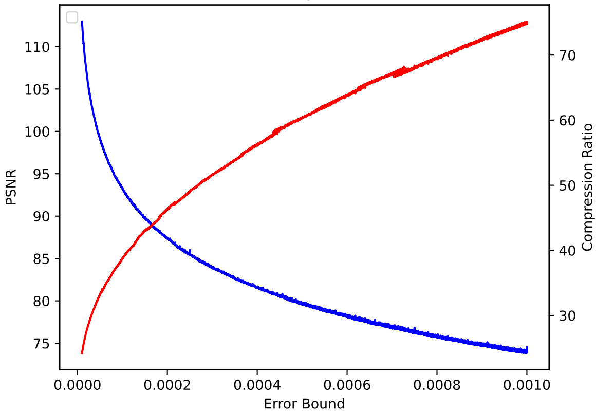
CLOUD 27 pressio:rel
