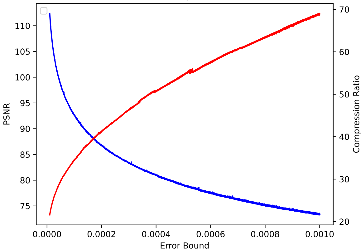
CLOUD 38 pressio:rel
