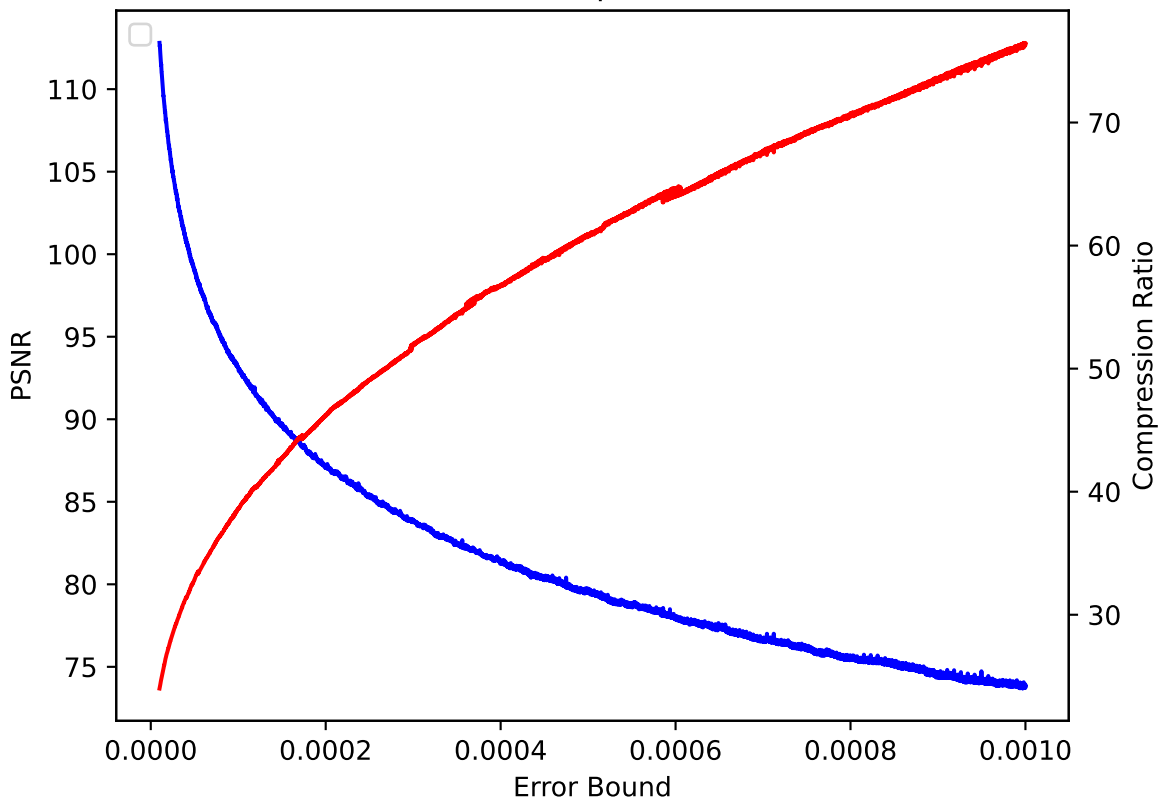
CLOUD 24 pressio:rel
