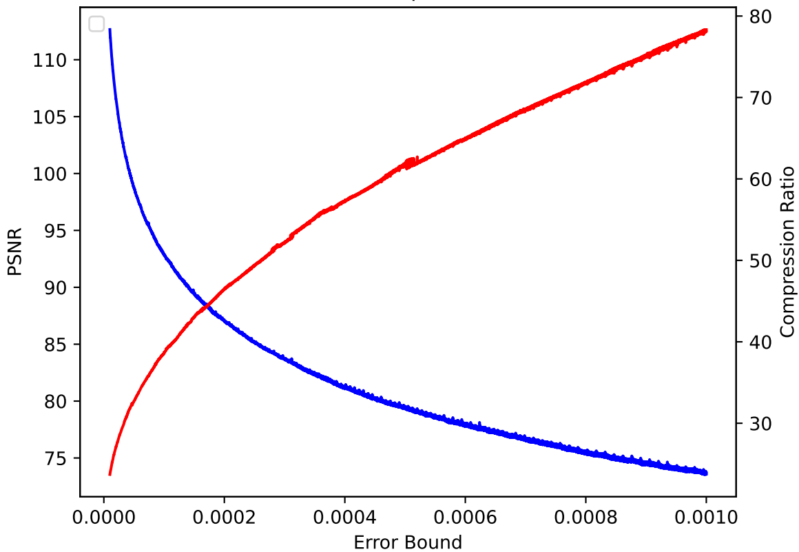
CLOUD 33 pressio:rel
