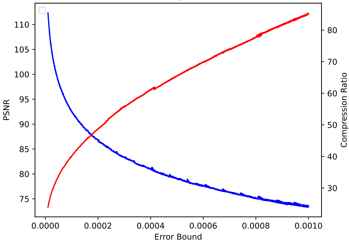
CLOUD 14 pressio:rel
