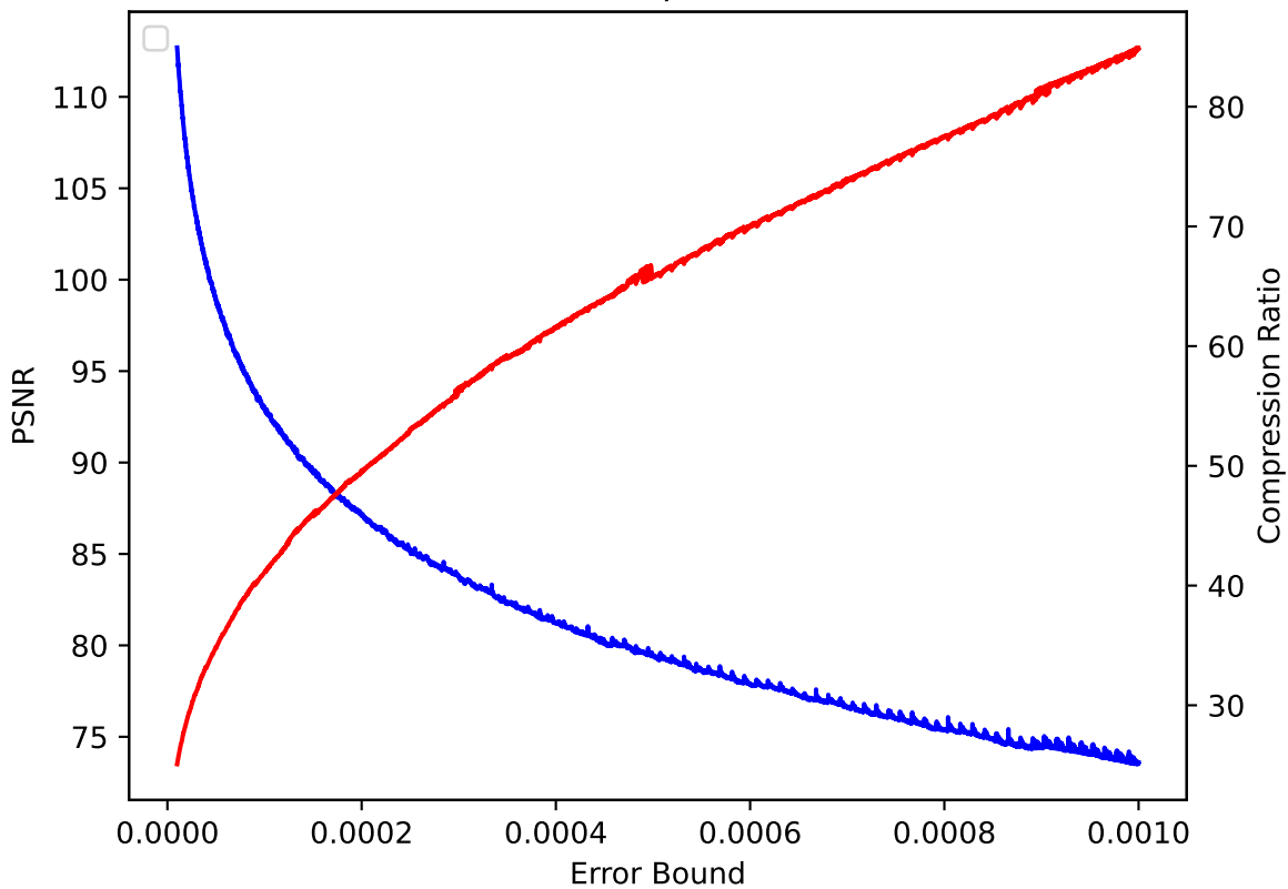
CLOUD 17 pressio:rel
