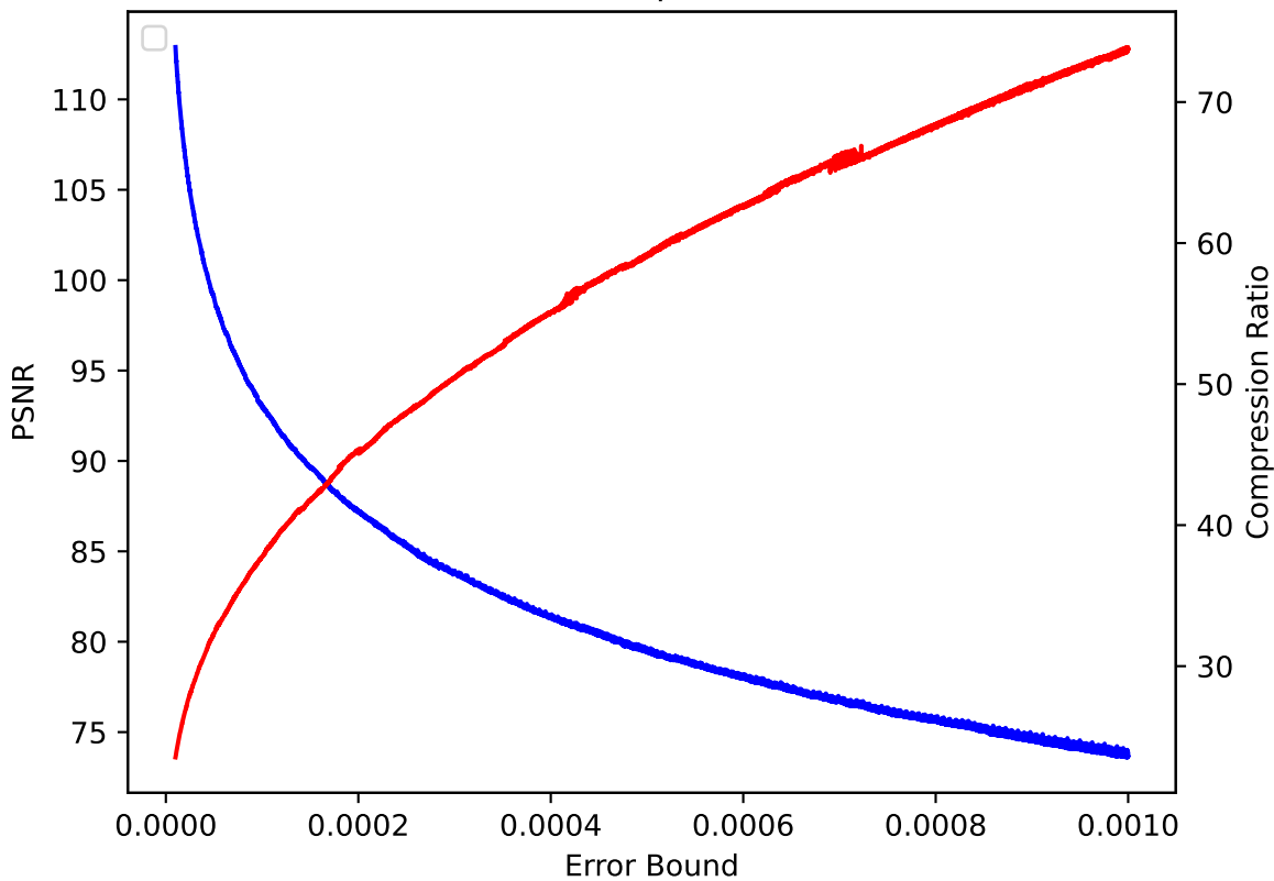
CLOUD 29 pressio:rel
