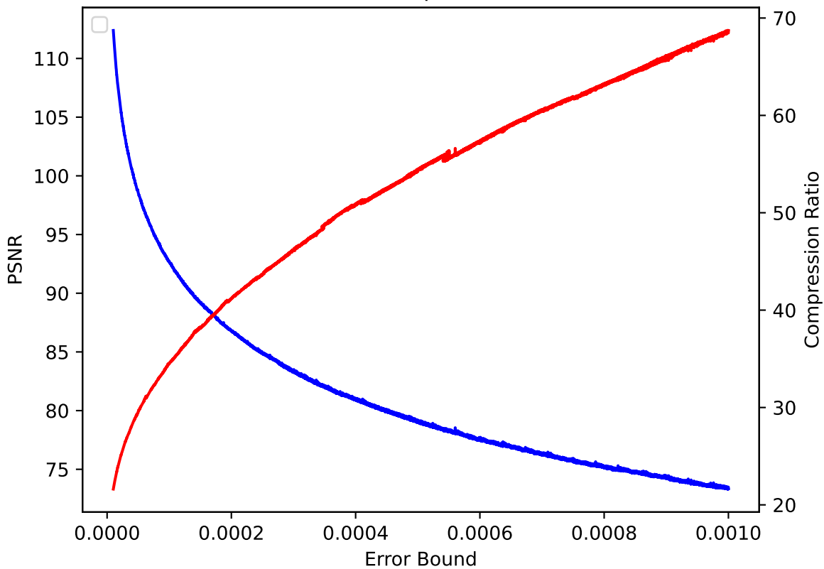
CLOUD 37 pressio:rel
