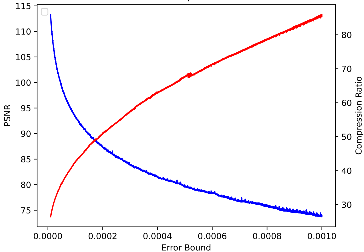
CLOUD 19 pressio:rel
