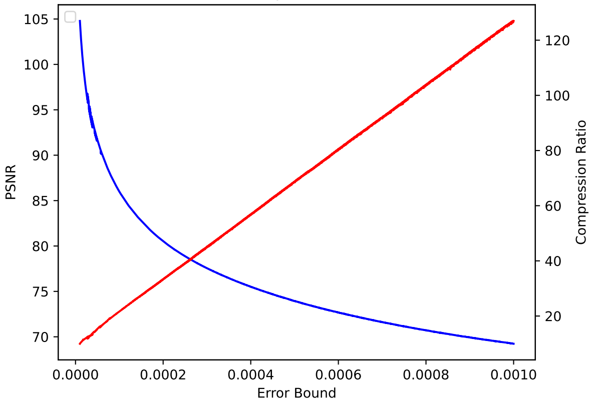
P 18 pressio:rel
