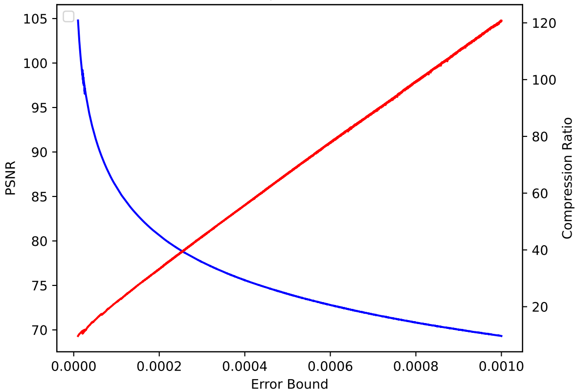
P 46 pressio:rel
