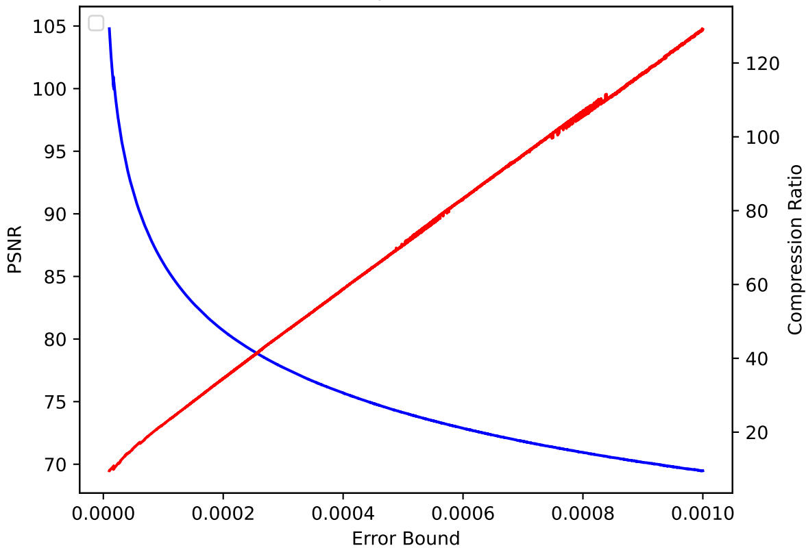
P 35 pressio:rel
