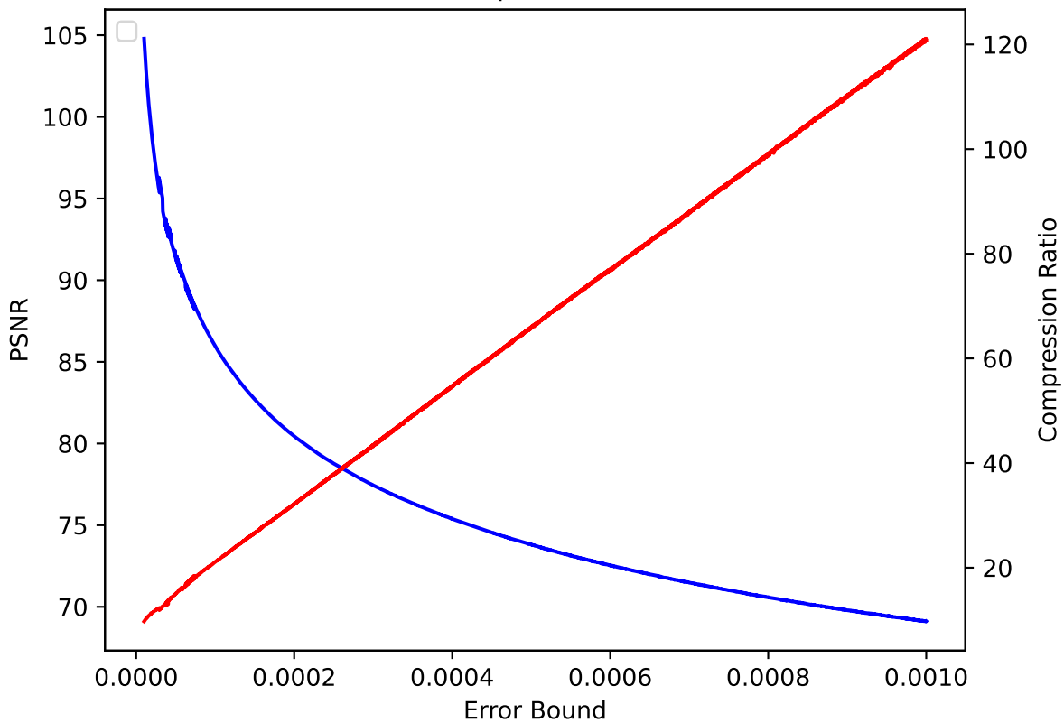
P 13 pressio:rel
