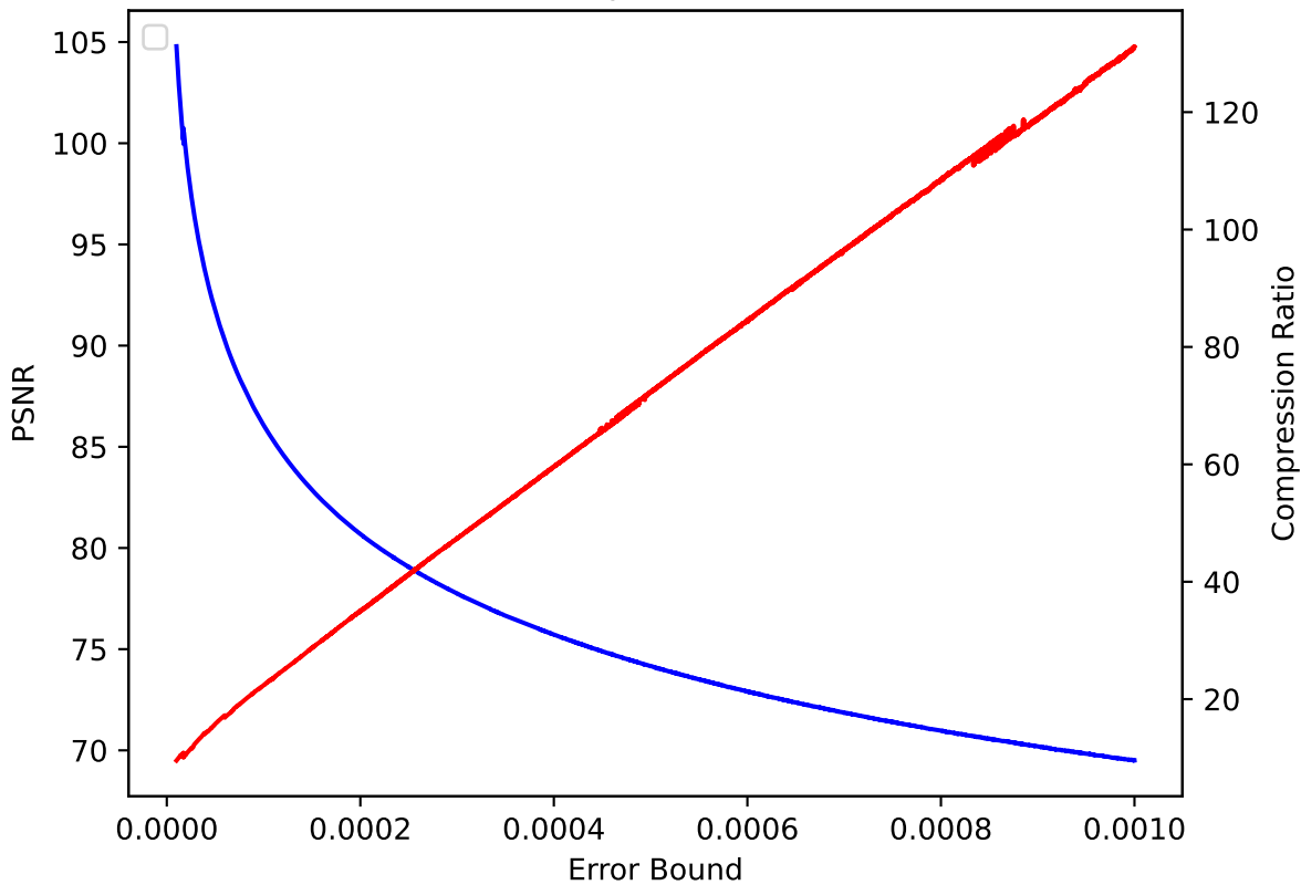
P 36 pressio:rel
