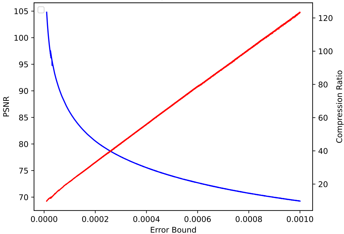
P 21 pressio:rel
