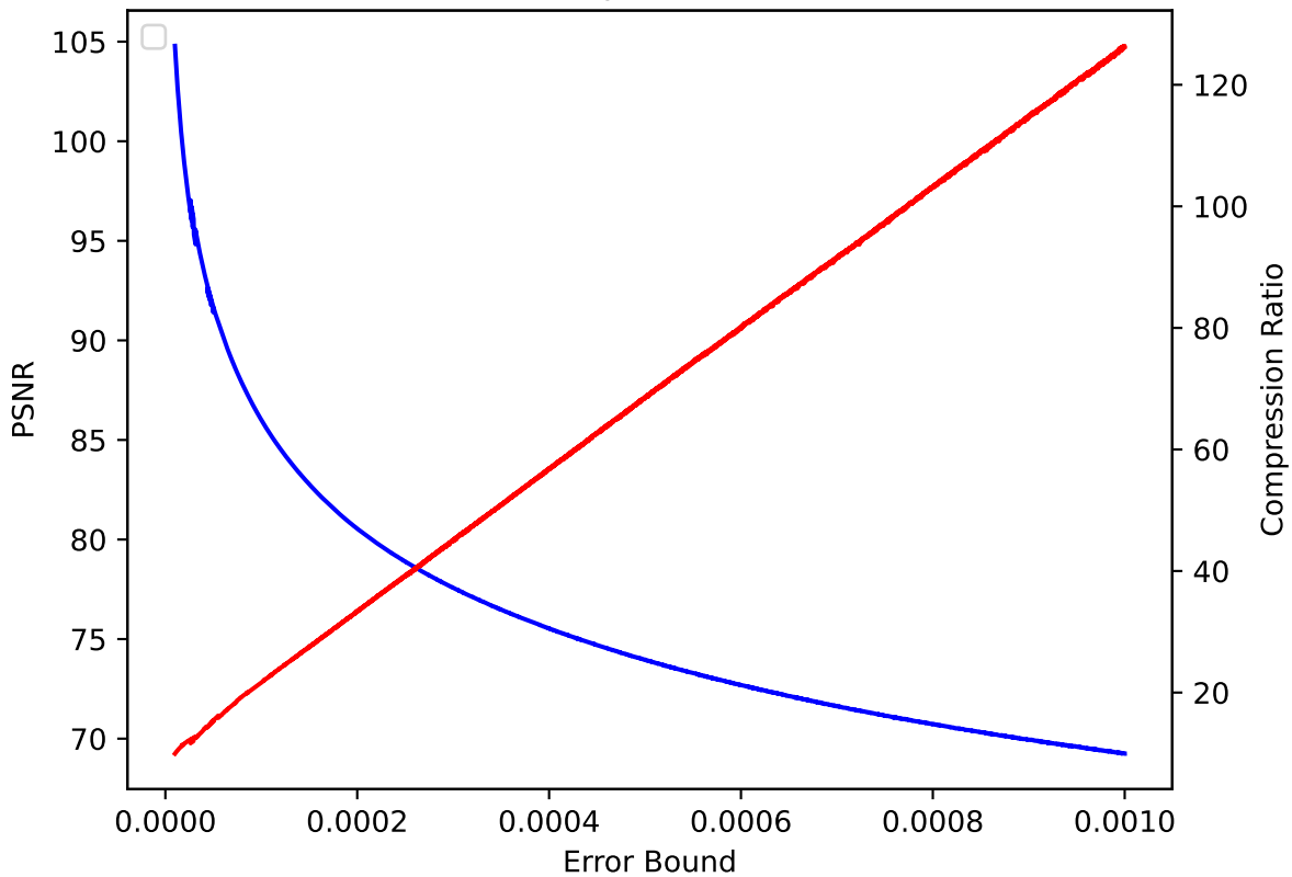
P 19 pressio:rel
