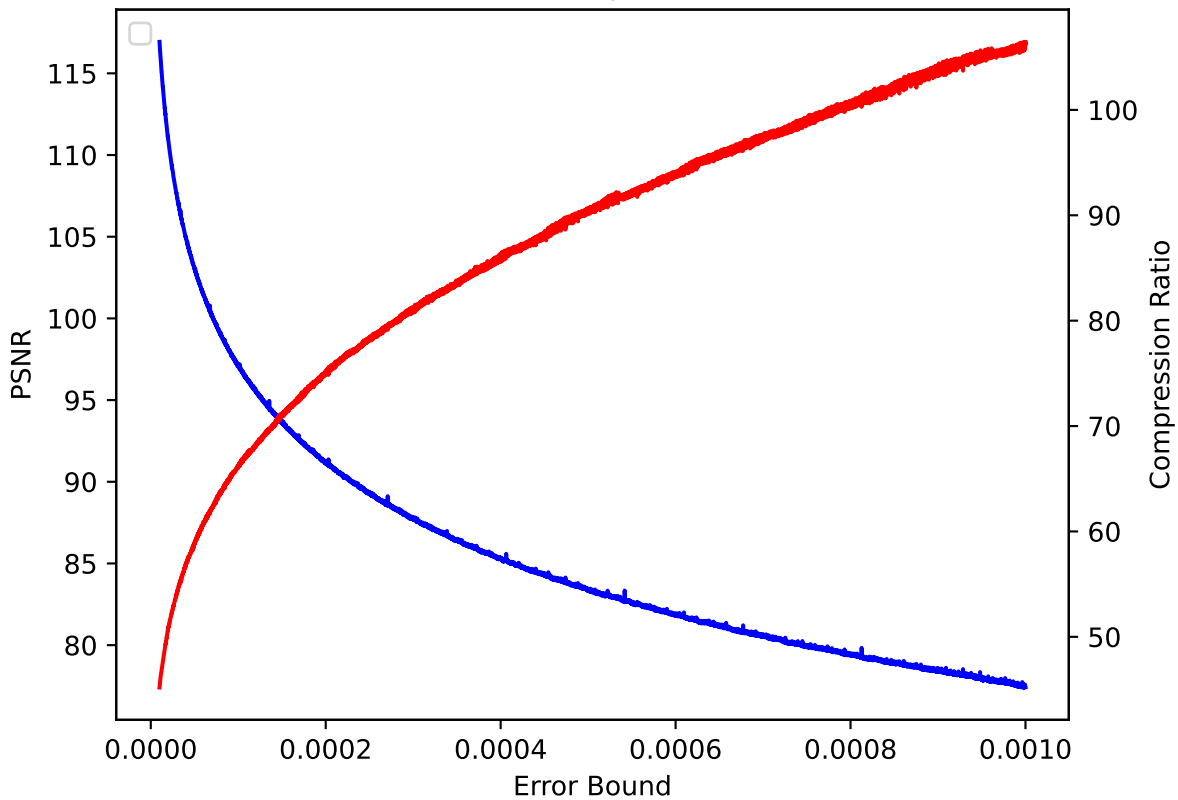
QCLLOUD 41 pressio:rel
