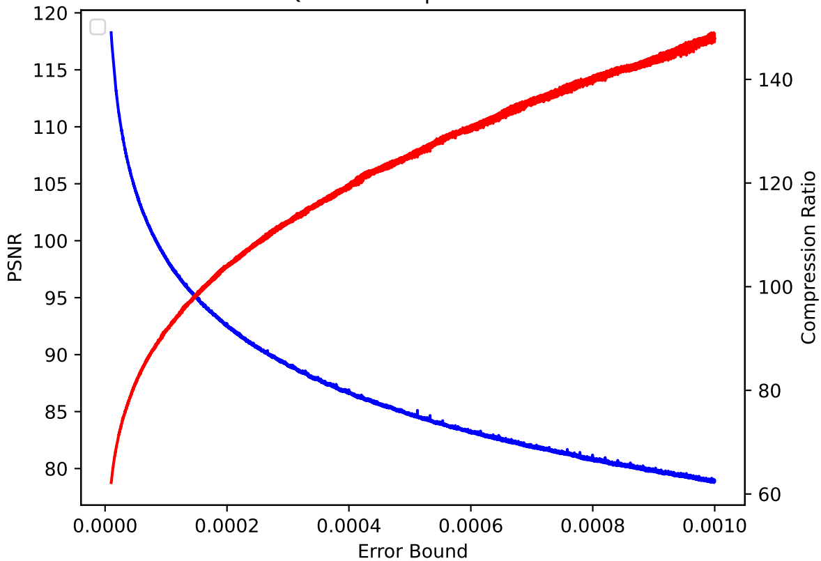
QCLLOUD 20 pressio:rel
