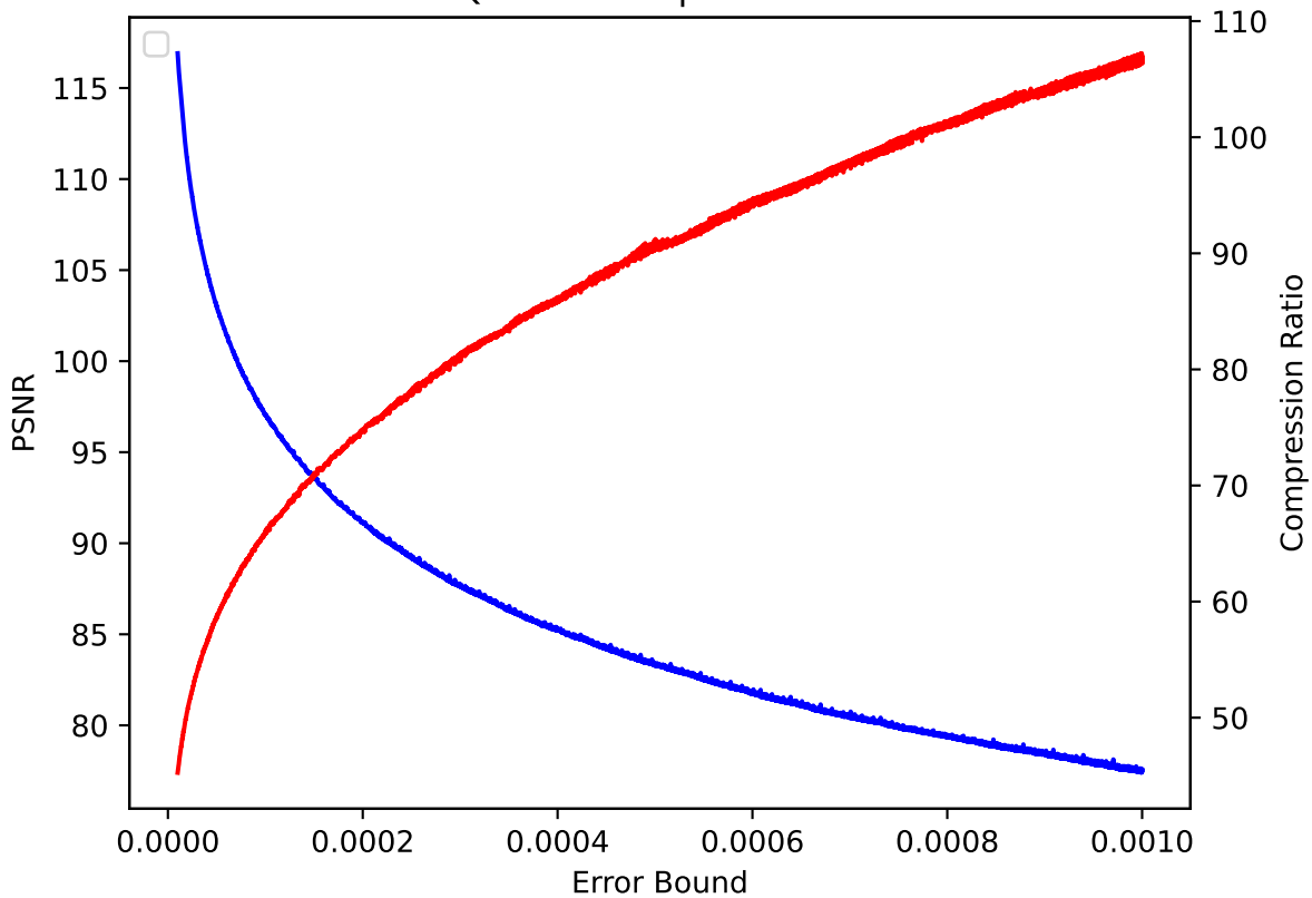
QCLLOUD 45 pressio:rel
