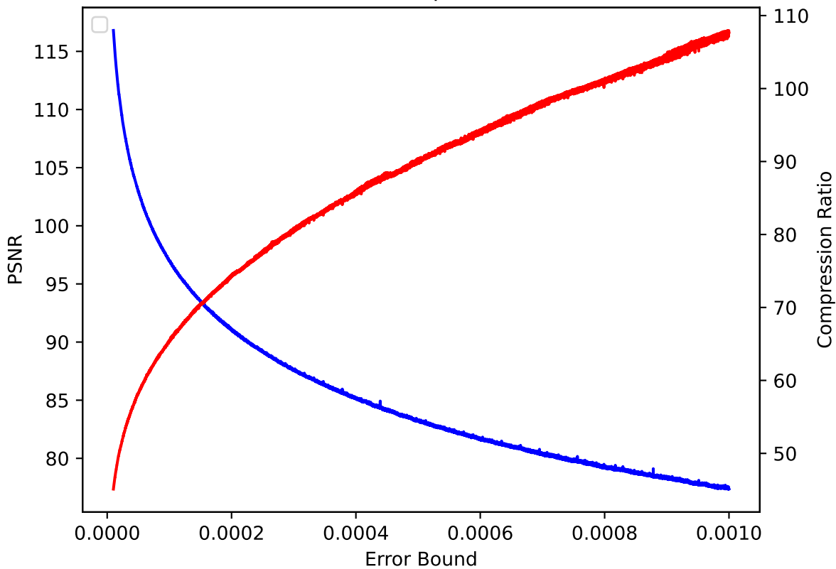
QCLLOUD 47 pressio:rel
