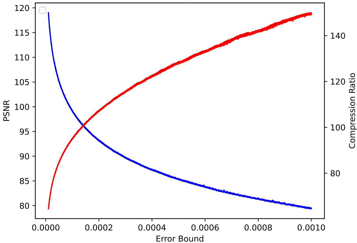
QCLLOUD 08 pressio:rel
