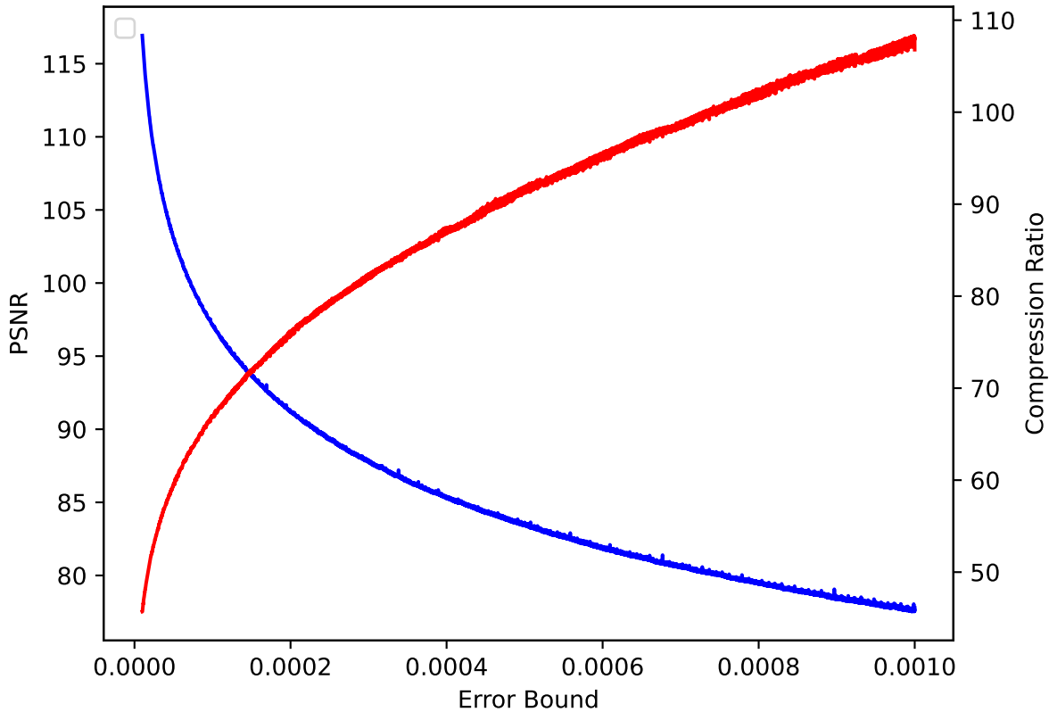
QCLLOUD 42 pressio:rel
