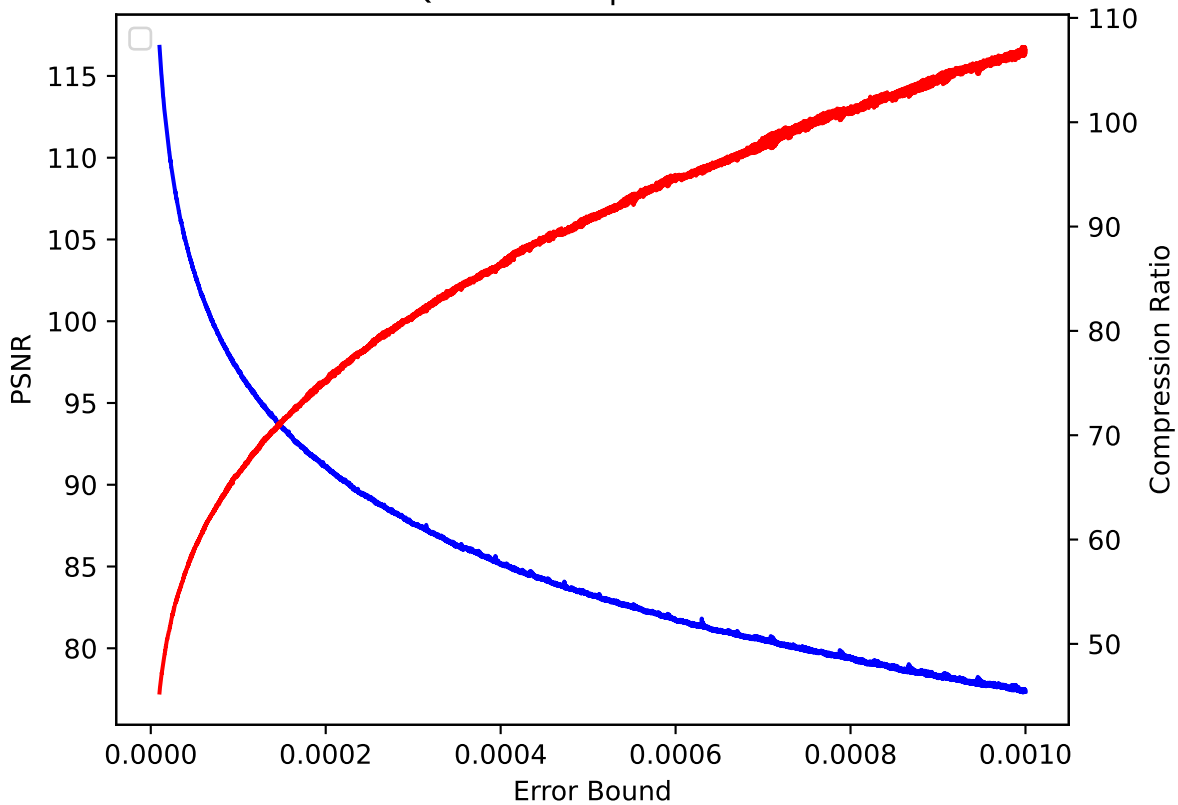
QCLLOUD 35 pressio:rel
