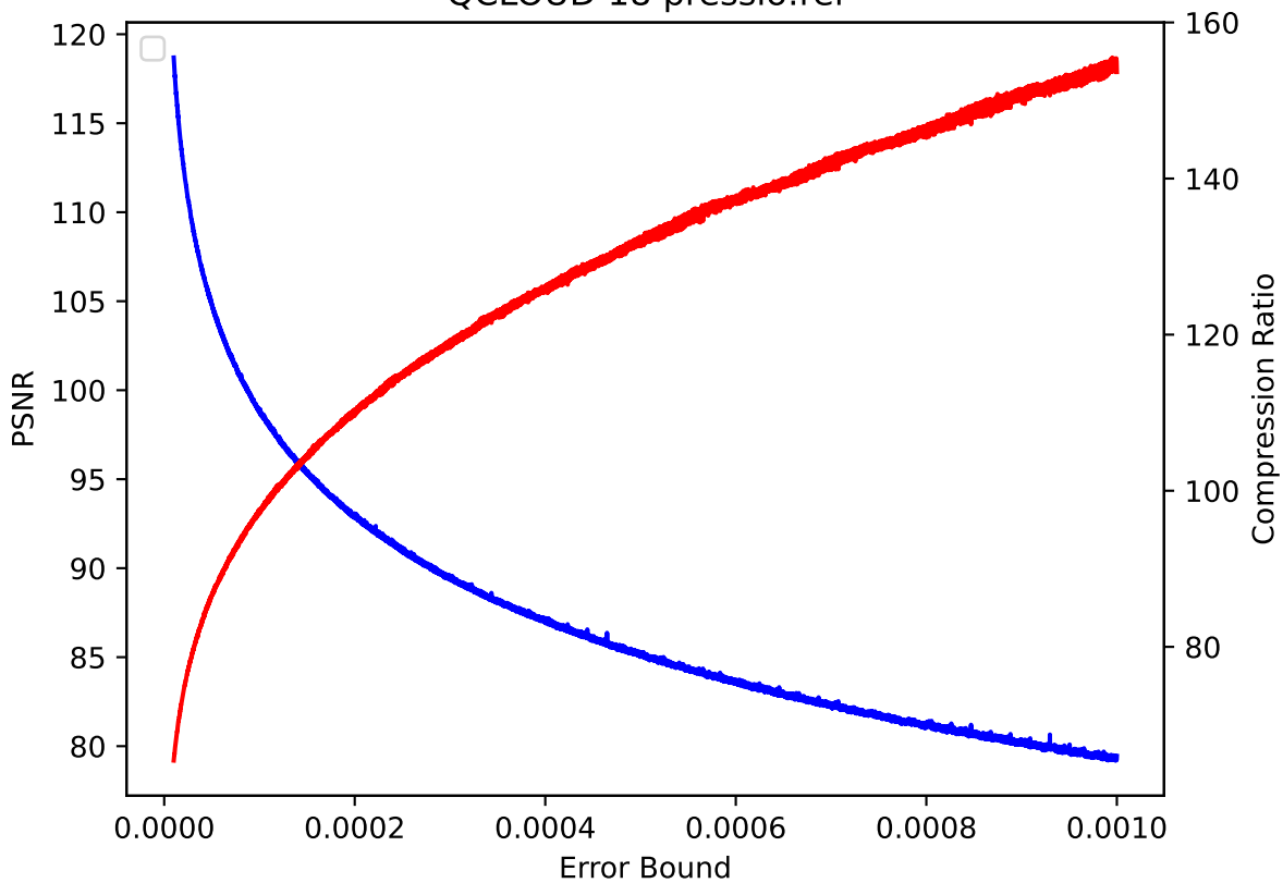
QCLLOUD 18 pressio:rel
