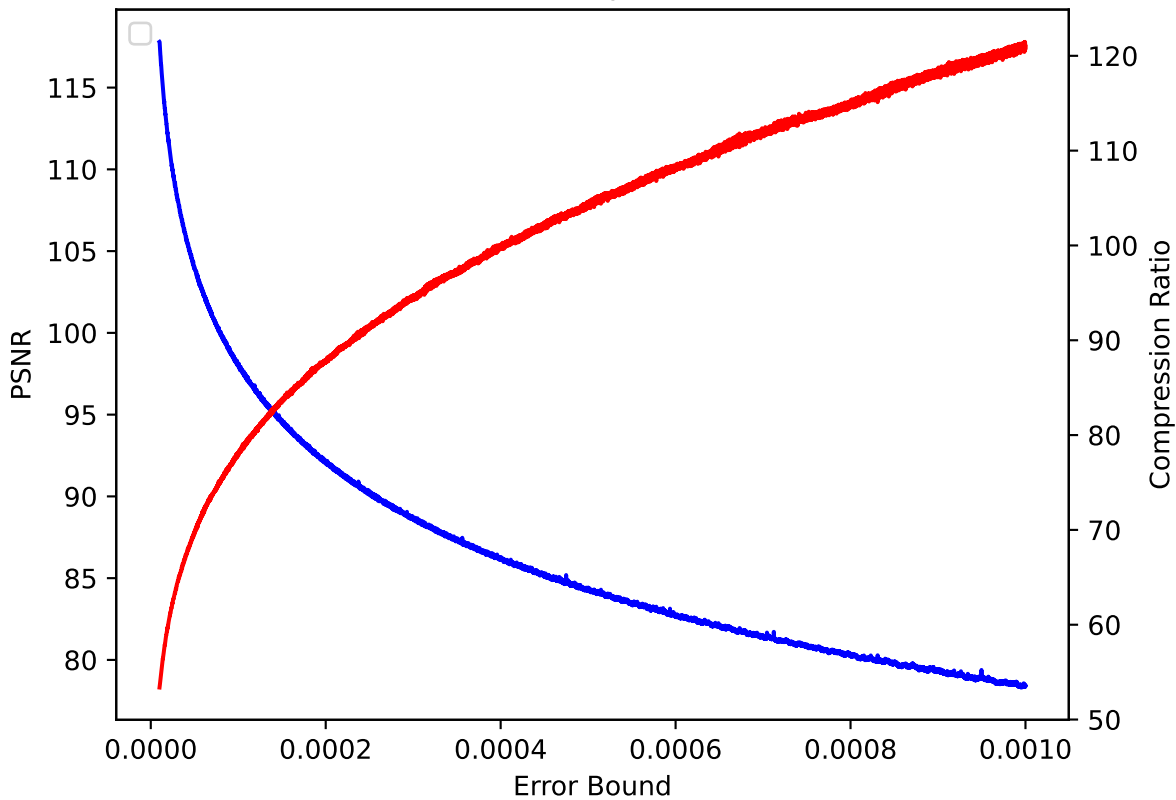
QCLLOUD 24 pressio:rel
