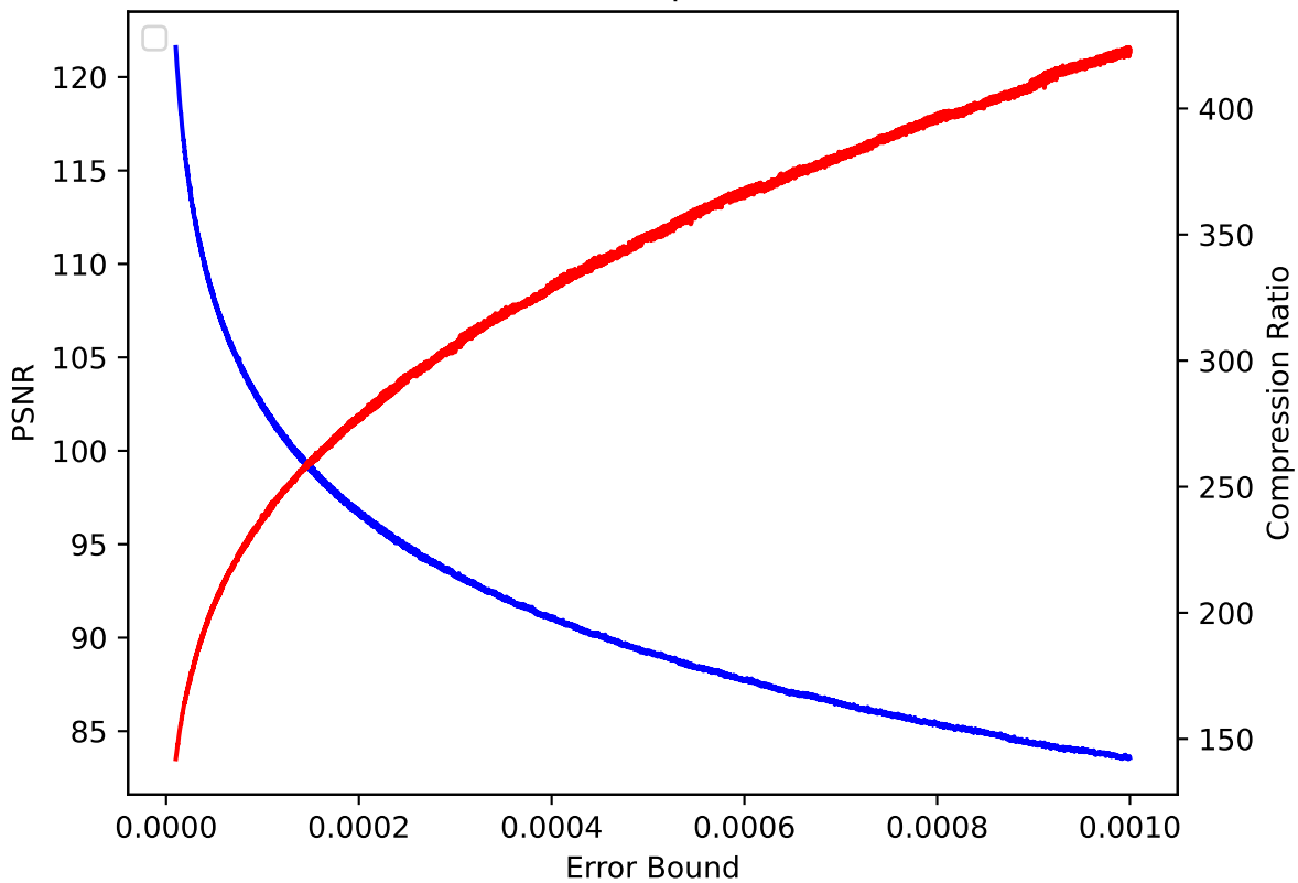
QCLLOUD 03 pressio:rel
