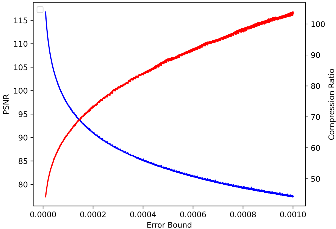
QCLLOUD 36 pressio:rel
