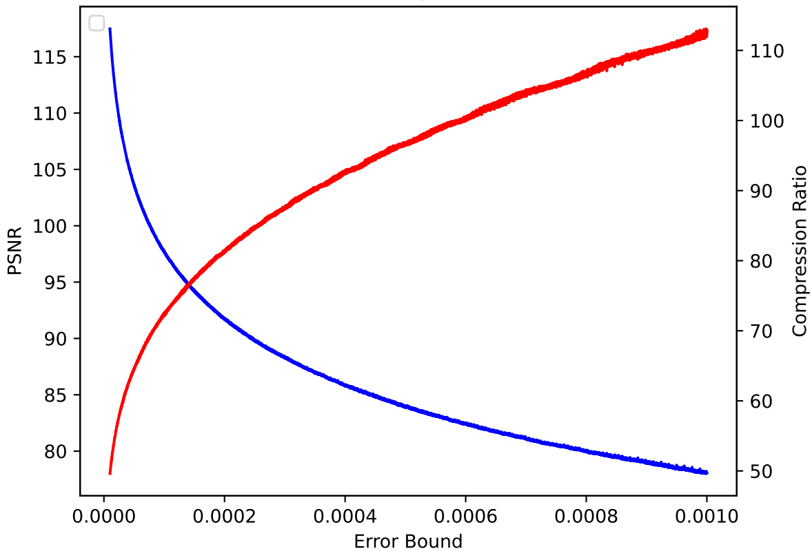
QCLLOUD 29 pressio:rel
