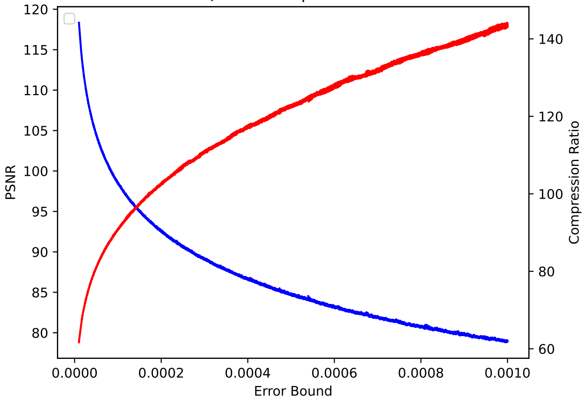
QCLLOUD 14 pressio:rel
