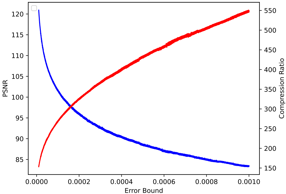
QCLLOUD 01 pressio:rel
