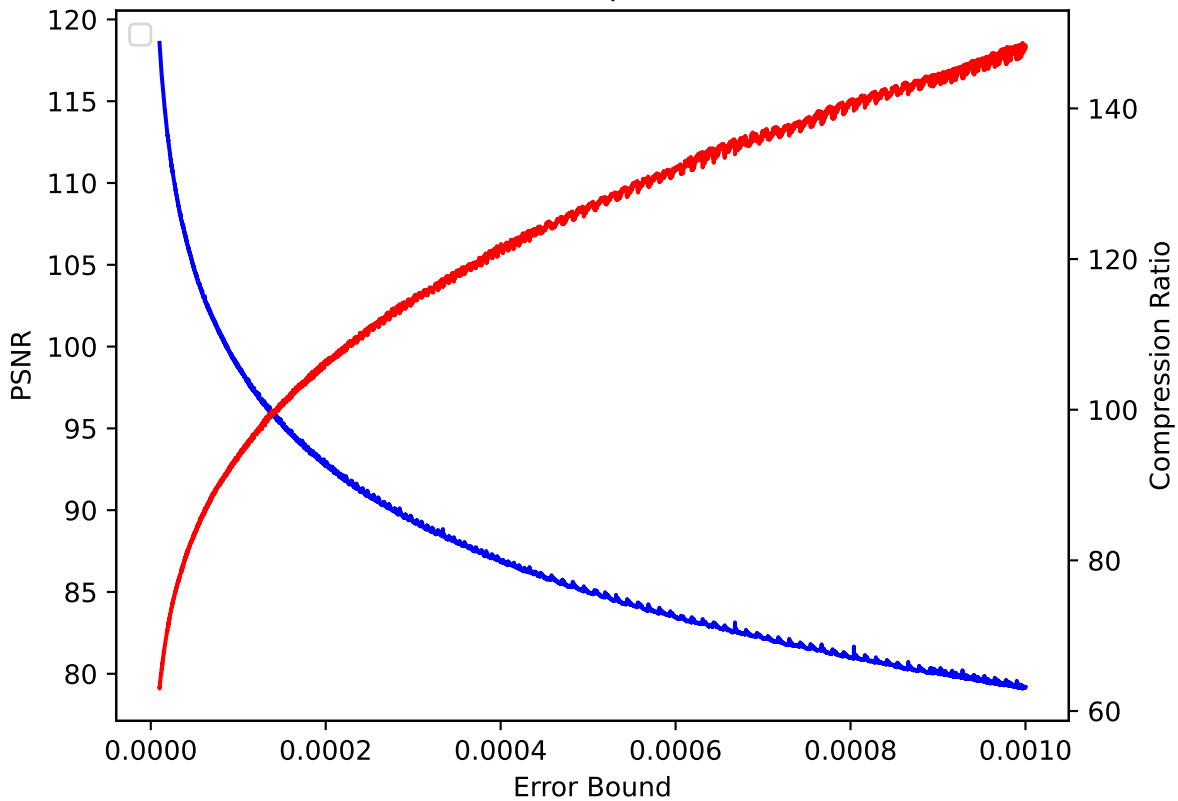
QCLLOUD 17 pressio:rel
