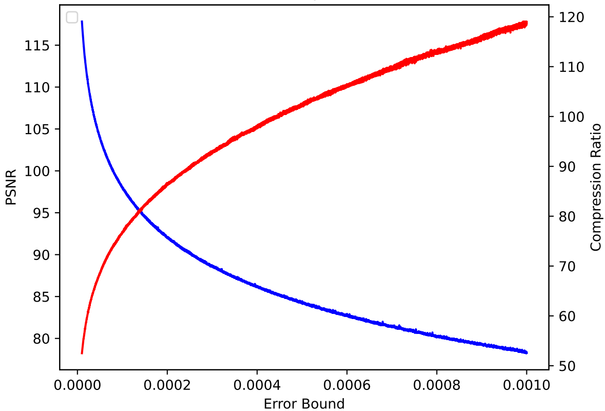
QCLoud 25 pressio:rel
