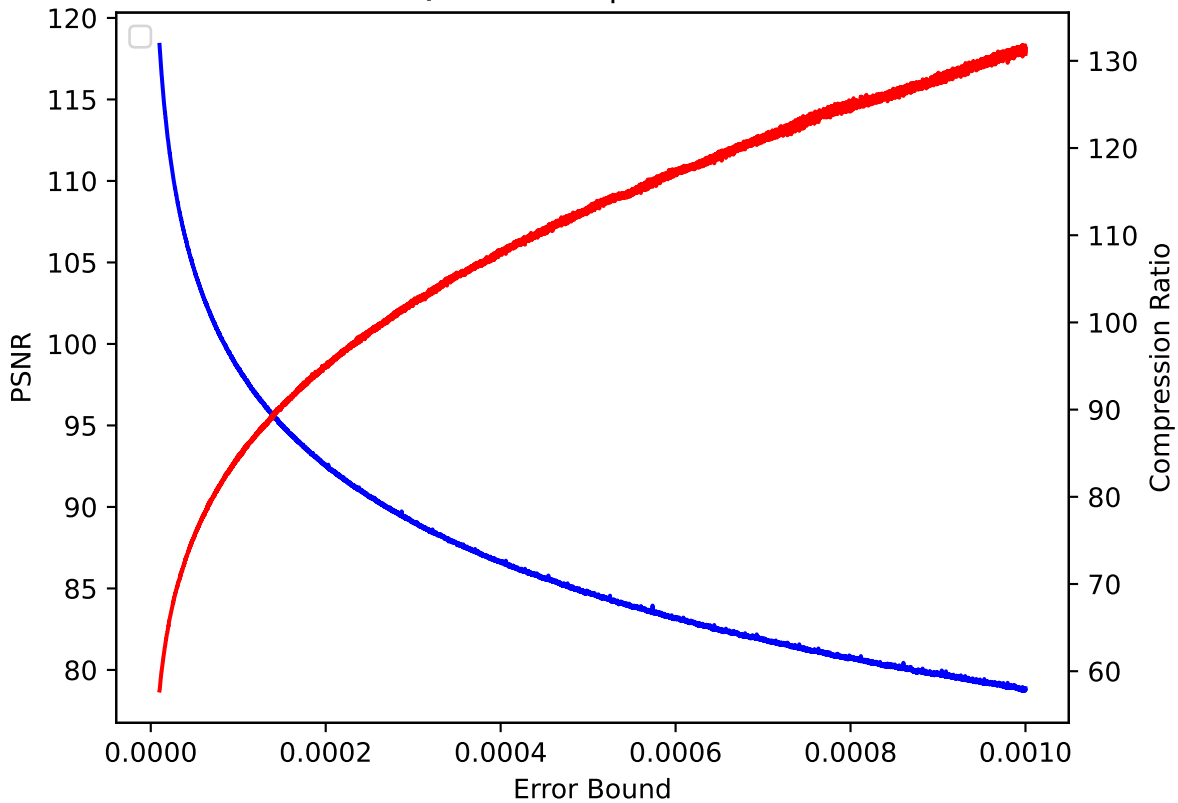
QCLLOUD 12 pressio:rel
