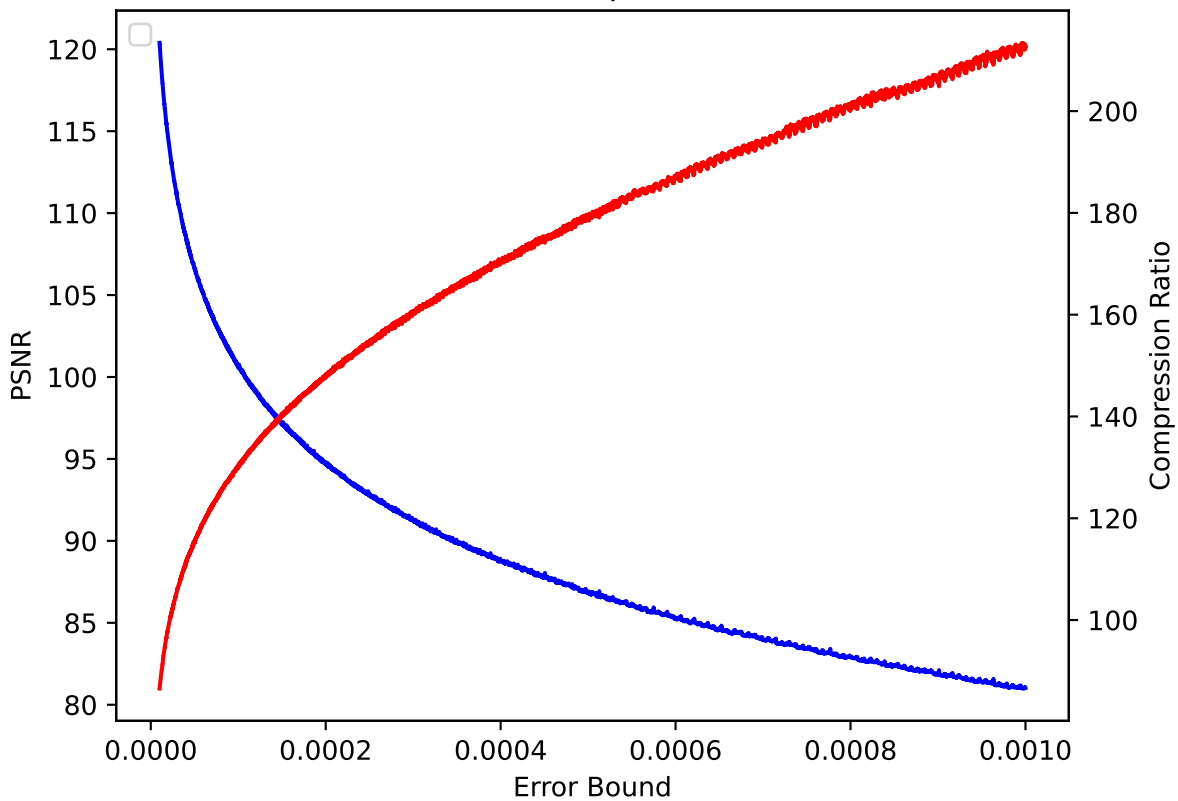
QCLLOUD 06 pressio:rel
