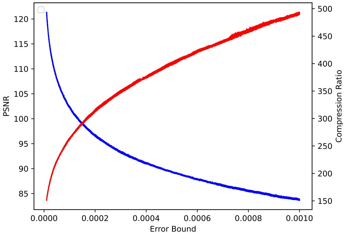
QCLLOUD 02 pressio:rel
