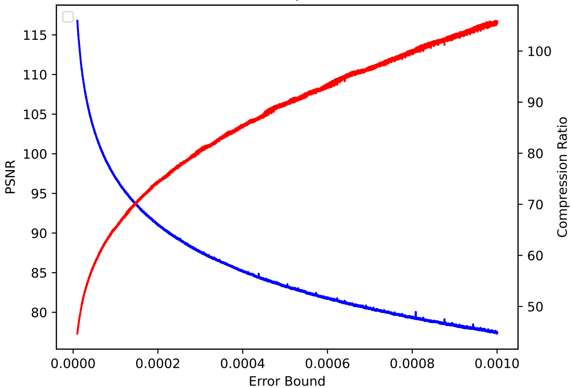
QCLLOUD 39 pressio:rel
