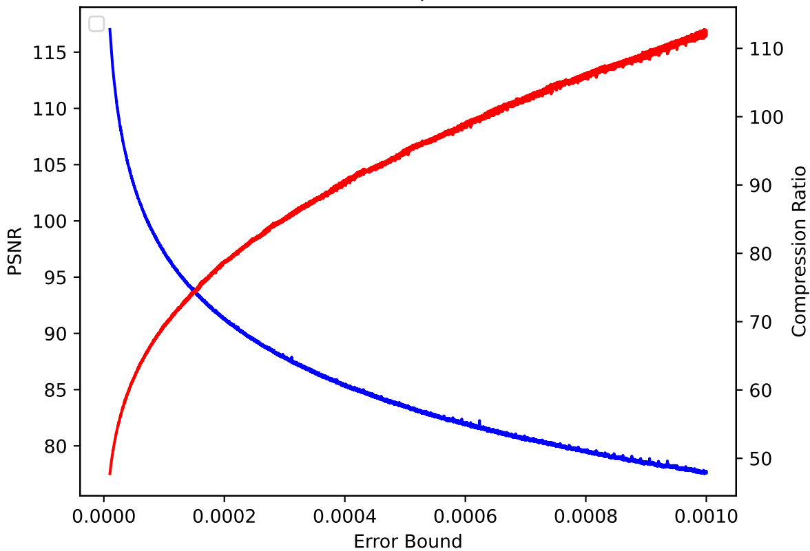
QCLLOUD 33 pressio:rel
