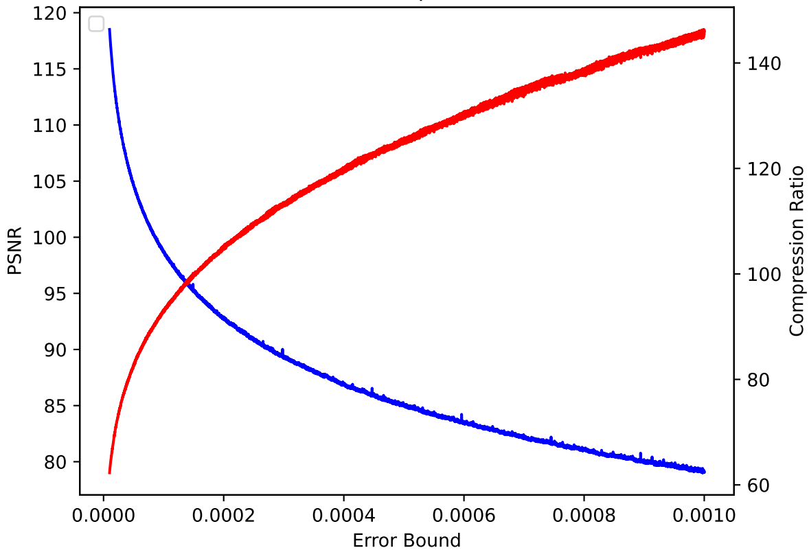
QCLLOUD 16 pressio:rel
