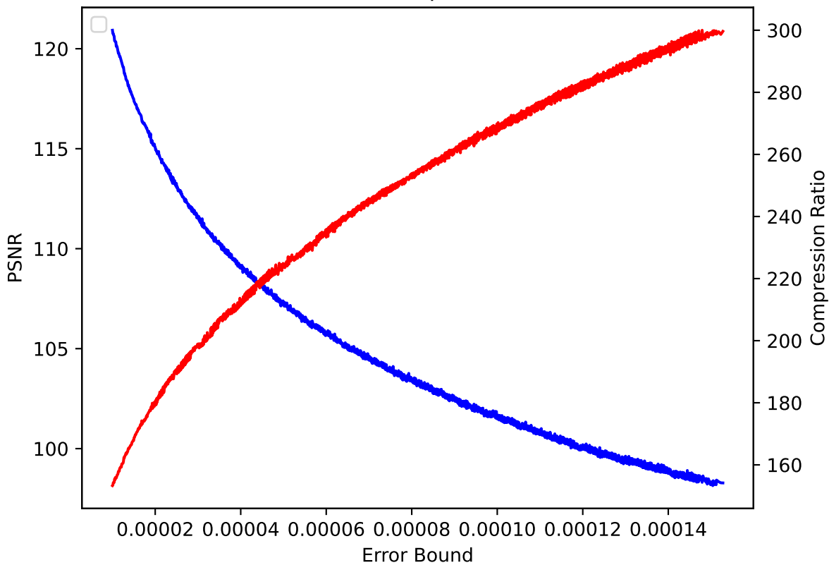
QCLLOUD 01 pressio:rel
