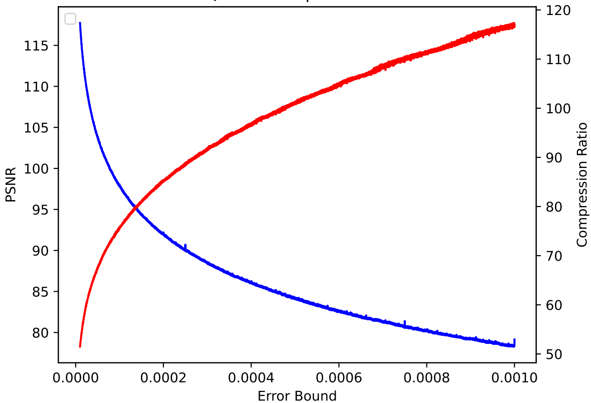
QCLLOUD 27 pressio:rel
