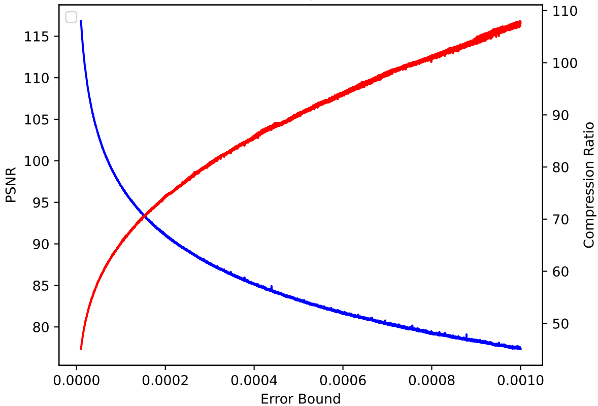
QCLLOUD 47 pressio:rel
