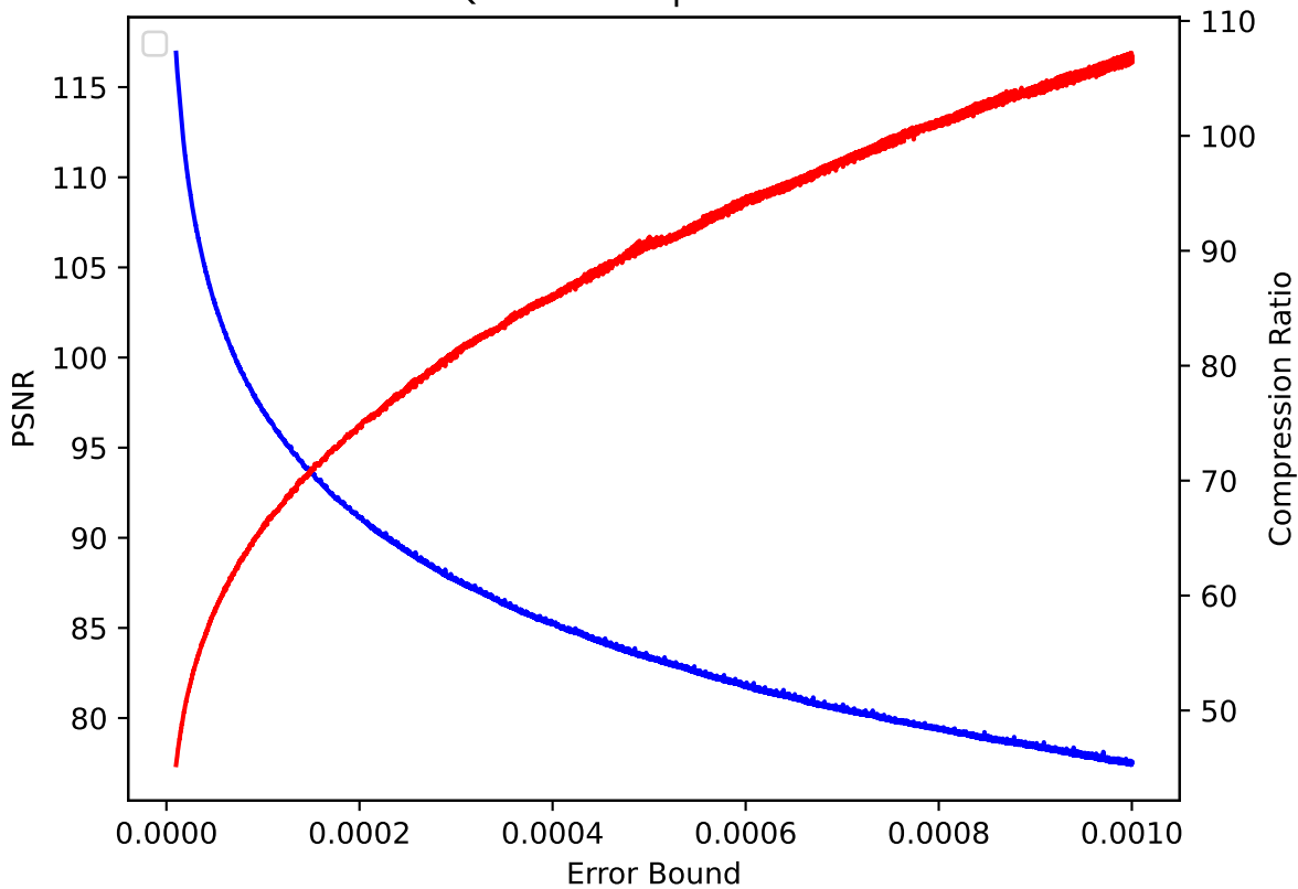
QCLLOUD 45 pressio:rel
