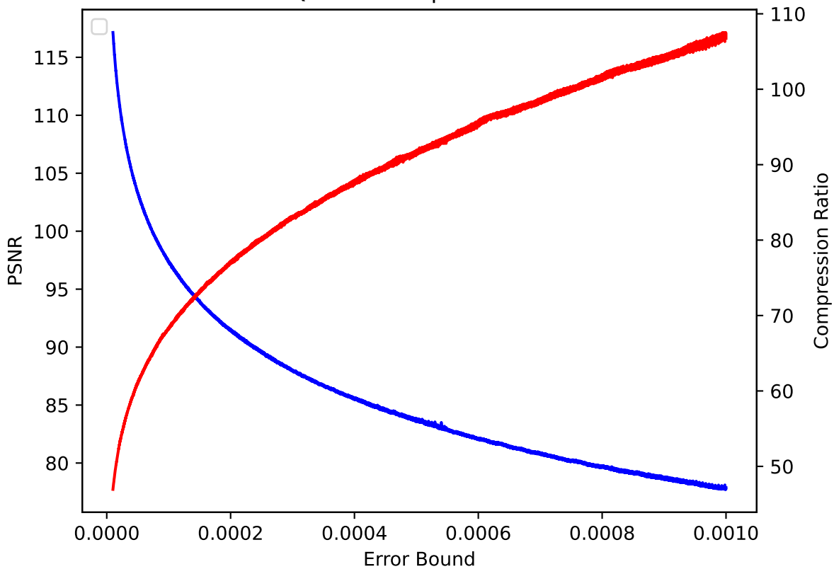
QCLLOUD 31 pressio:rel
