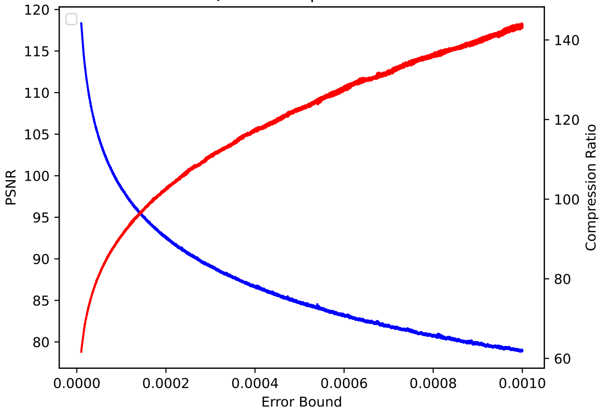
QCLLOUD 14 pressio:rel
