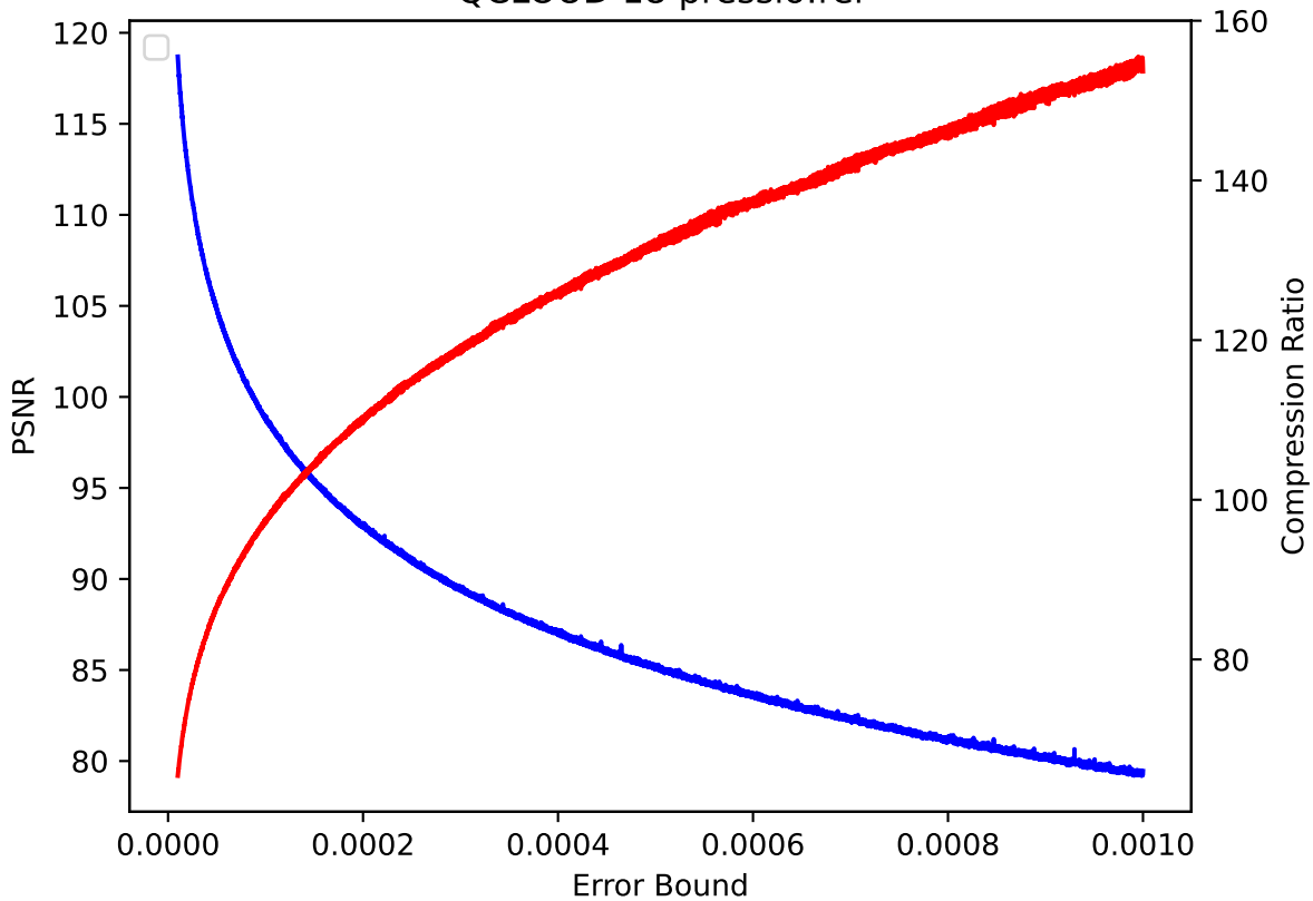
QCLLOUD 18 pressio:rel
