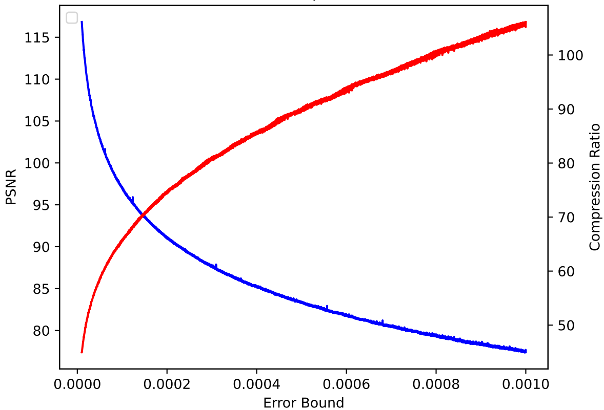
QCLLOUD 38 pressio:rel
