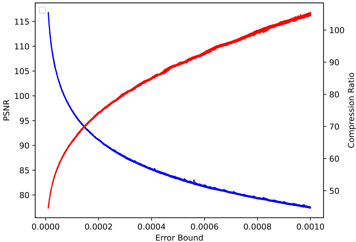
QCLLOUD 37 pressio:rel
