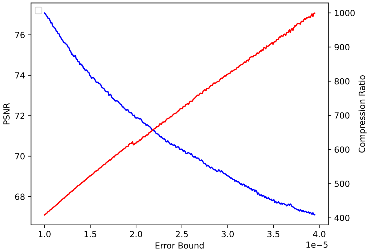
QGRAUP 37 pressio:abs
