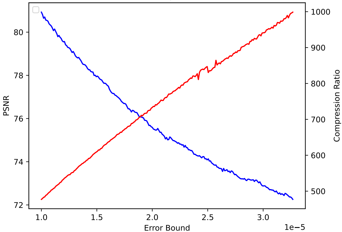
QGRAUP 33 pressio:abs
