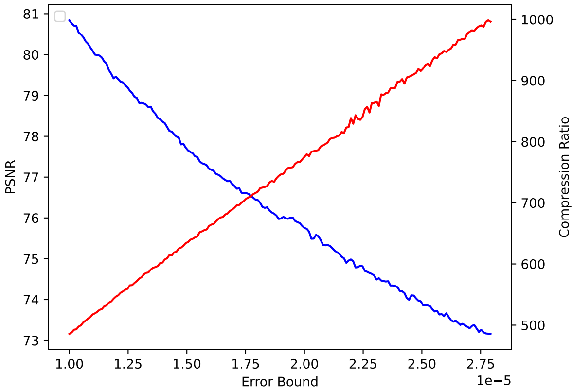
QGRAUP 44 pressio:abs
