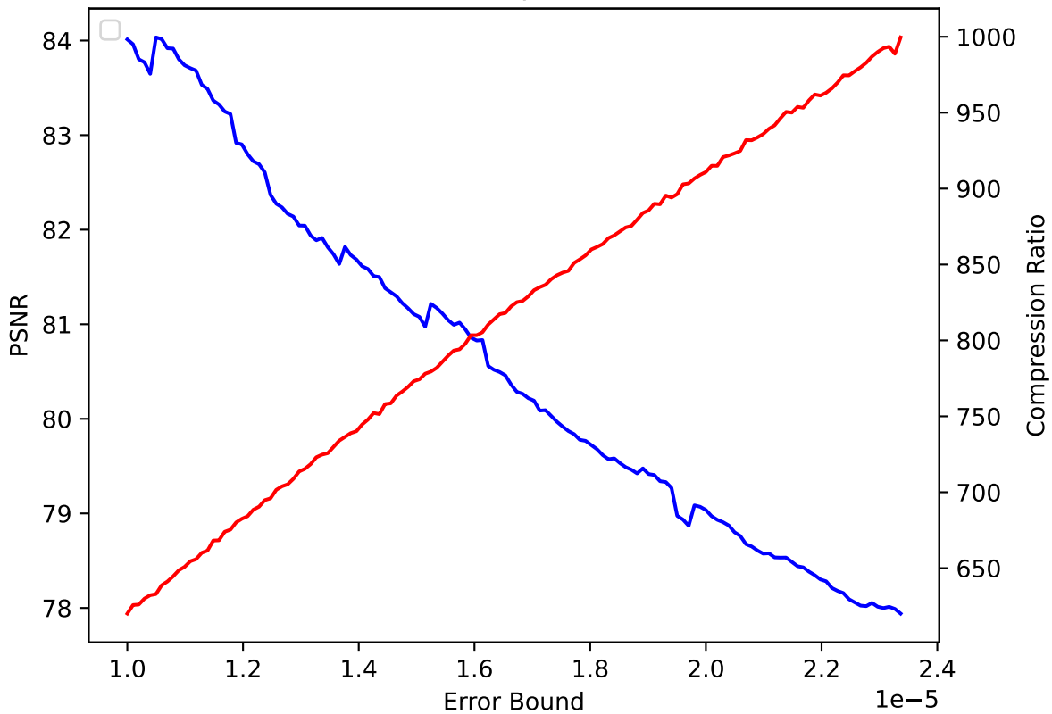
QGRAUP 07 pressio:abs
