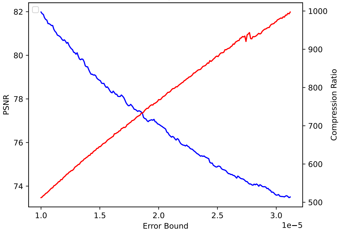
QGRAUP 20 pressio:abs
