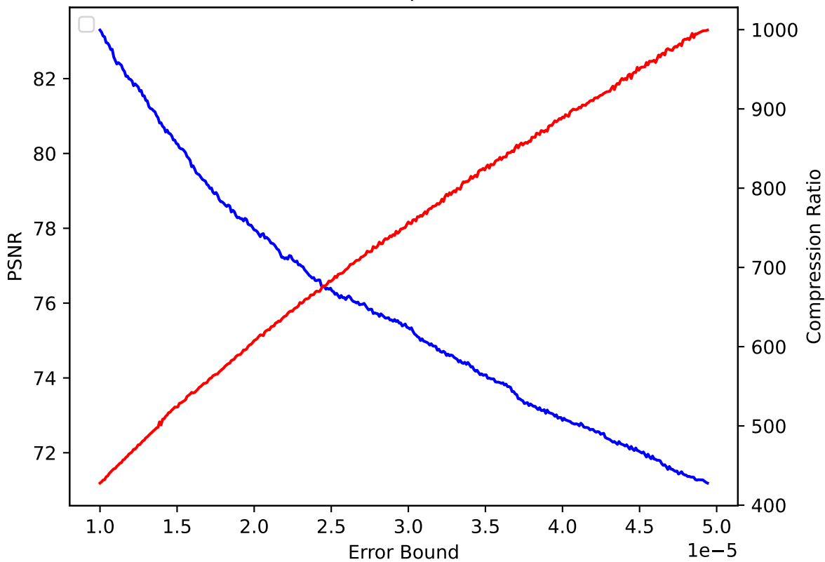
QGRAUP 09 pressio:abs
