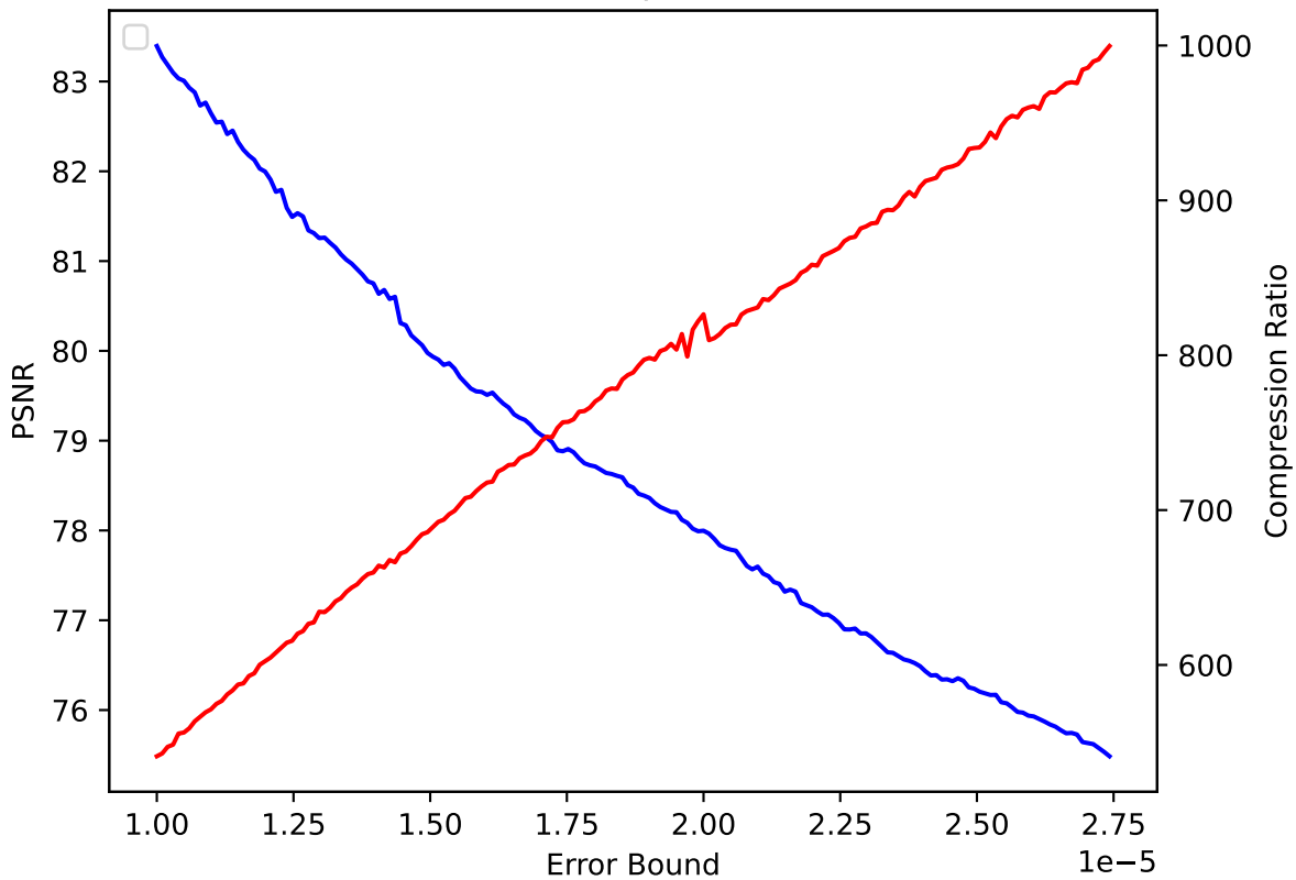
QGRAUP 28 pressio:abs
