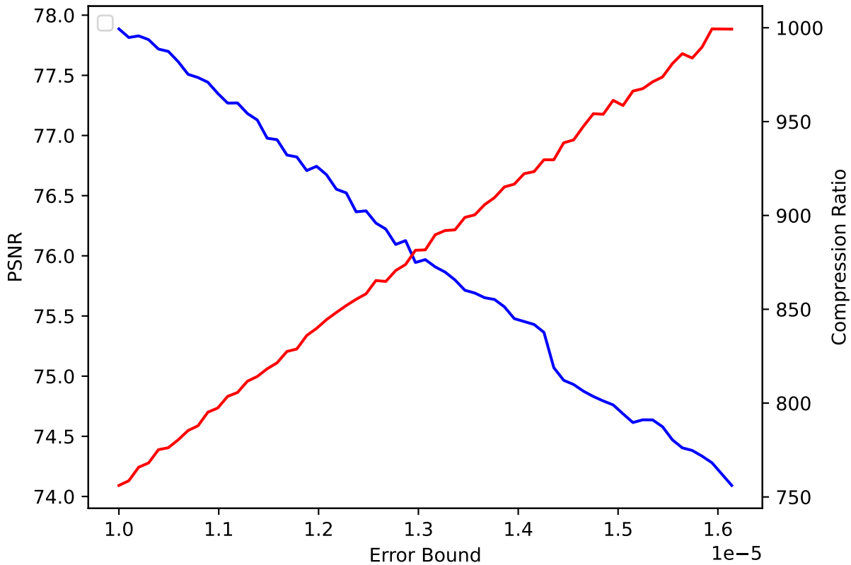
QGRAUP 05 pressio:abs
