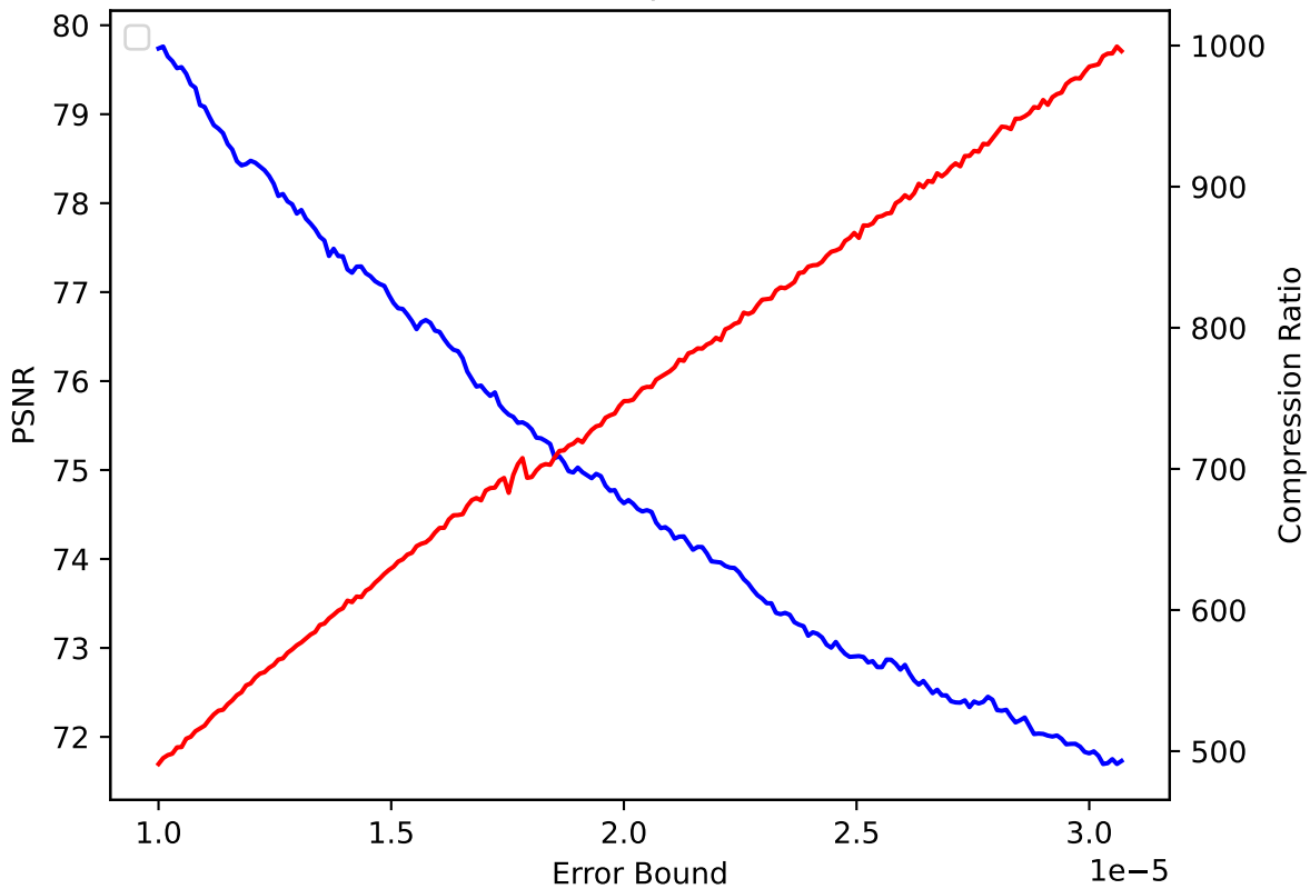
QGRAUP 32 pressio:abs
