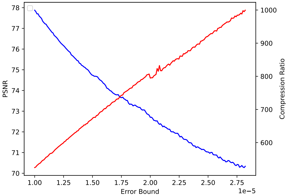
QGRAUP 31 pressio:abs
