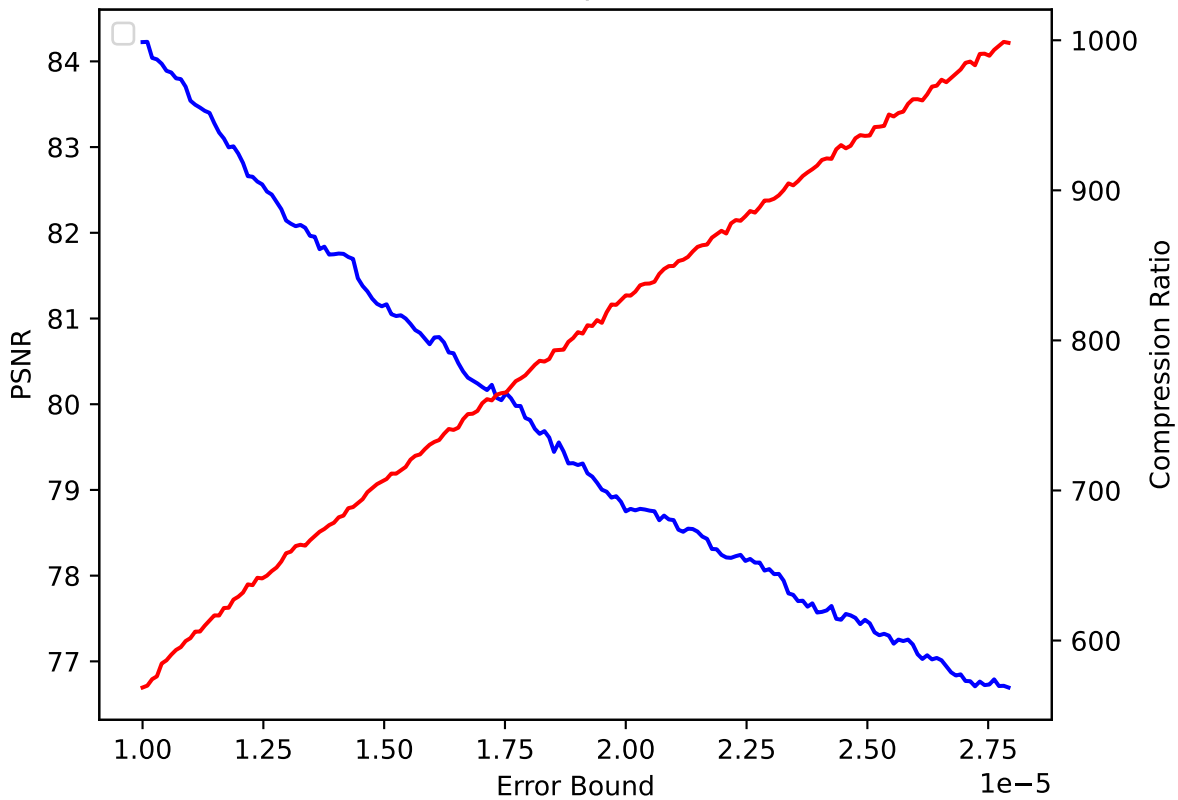
QGRAUP 08 pressio:abs
