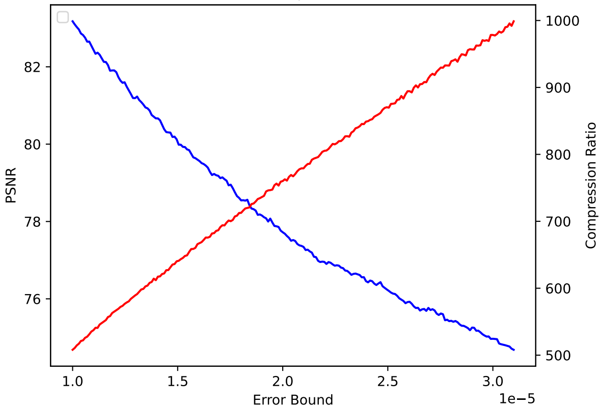
QGRAUP 22 pressio:abs
