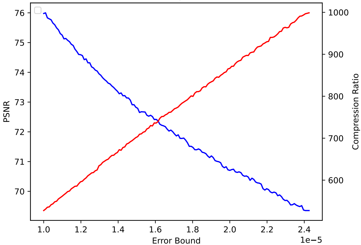
QGRAUP 48 pressio:abs
