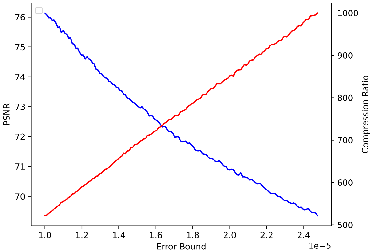
QGRAUP 47 pressio:abs
