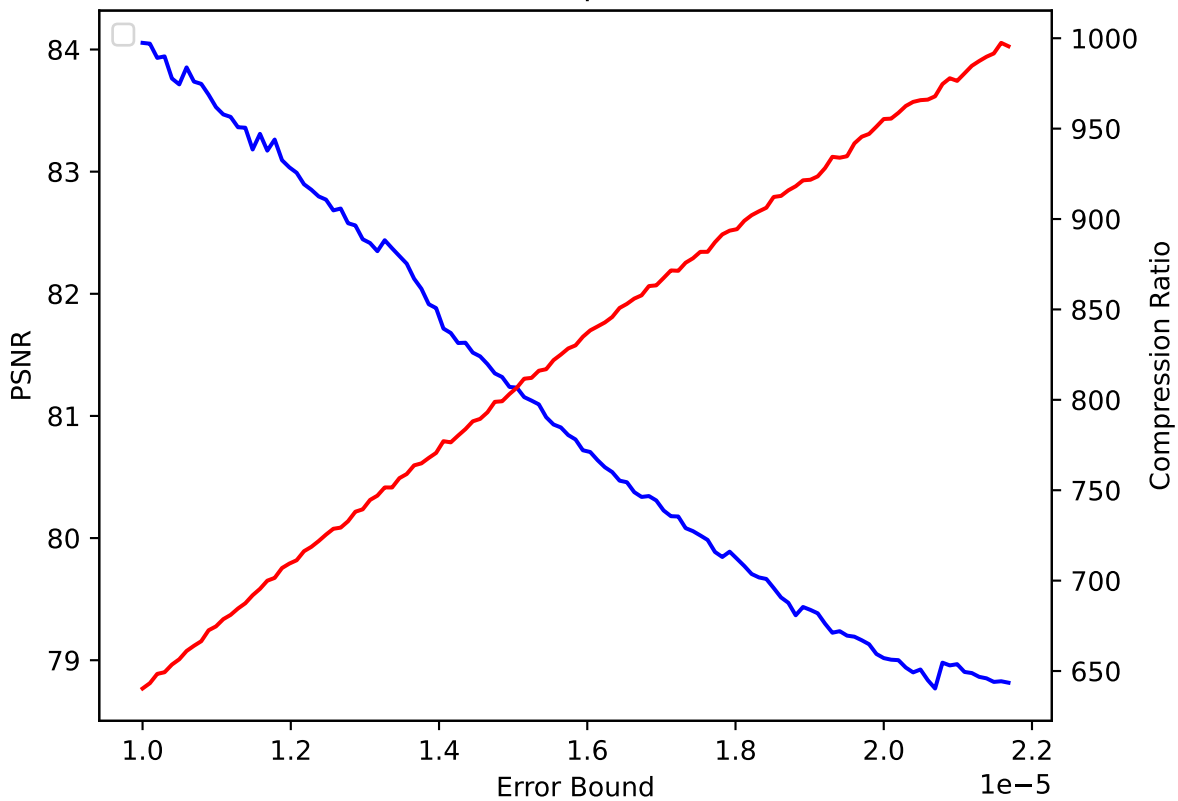
QGRAUP 06 pressio:abs
