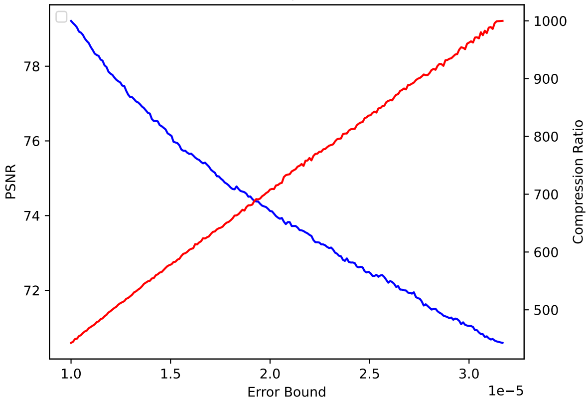
QGRAUP 41 pressio:abs
