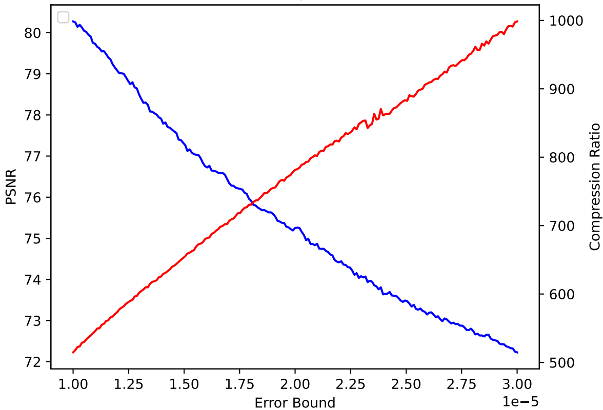
QGRAUP 15 pressio:abs
