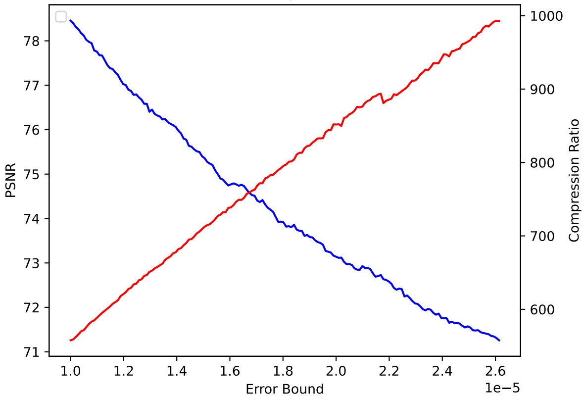
QGRAUP 16 pressio:abs
