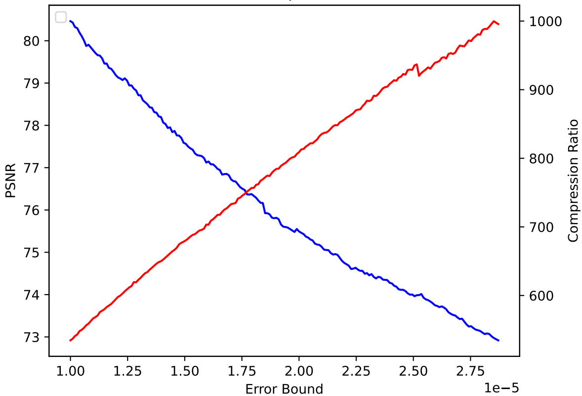
QGRAUP 17 pressio:abs
