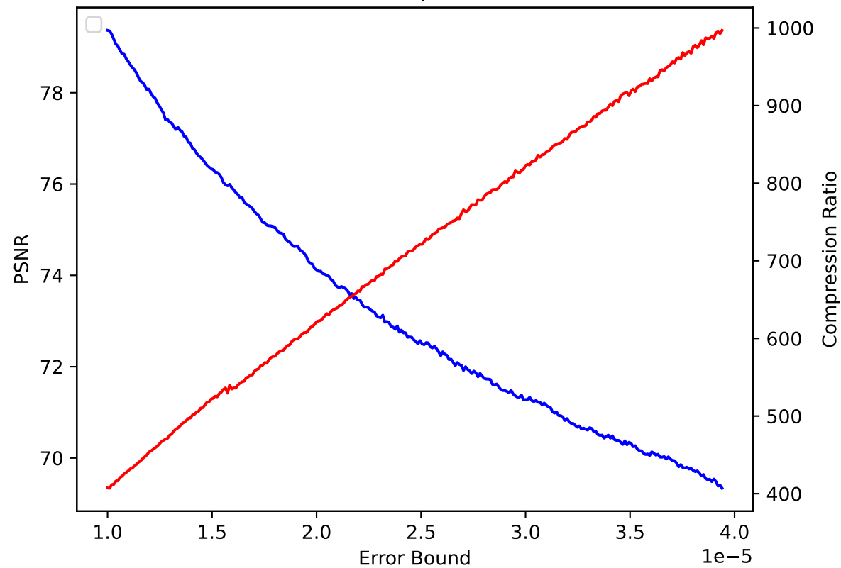
QGRAUP 38 pressio:abs
