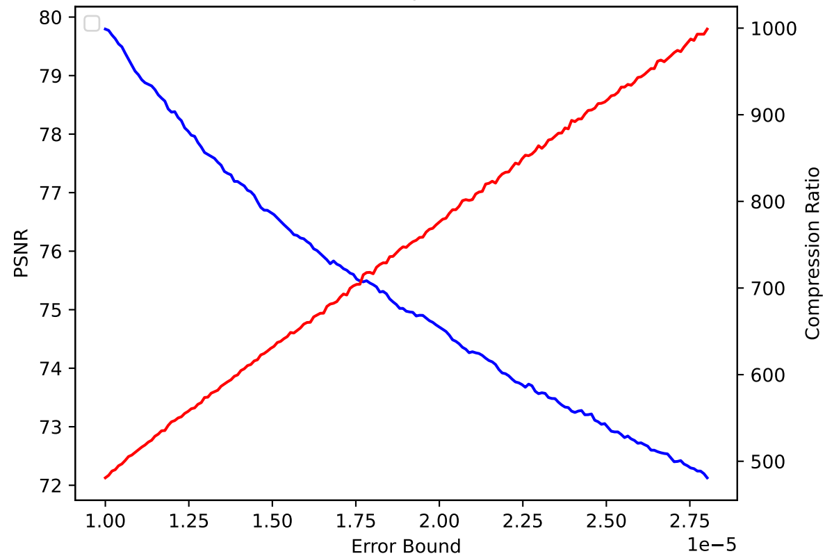
QGRAUP 45 pressio:abs
