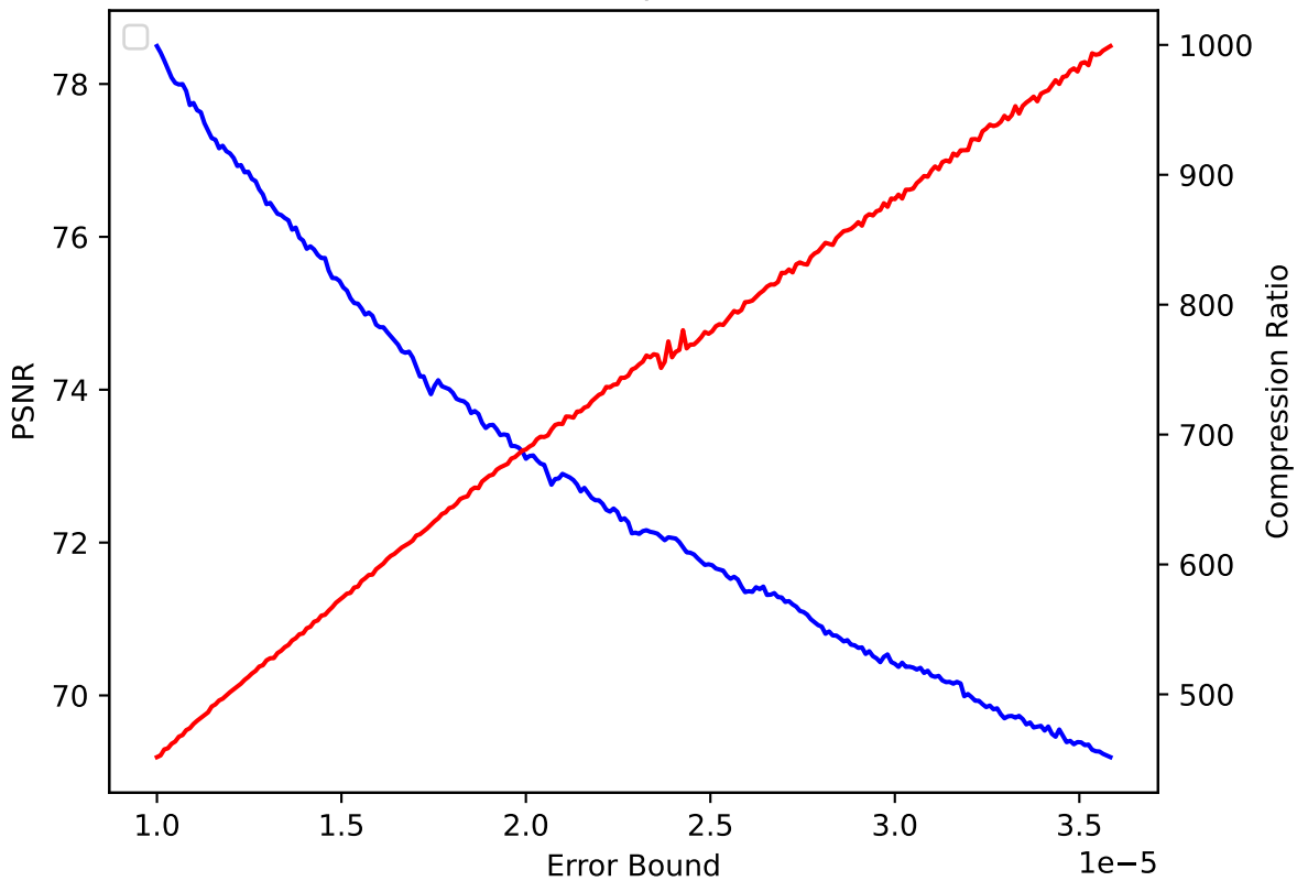
QGRAUP 34 pressio:abs
