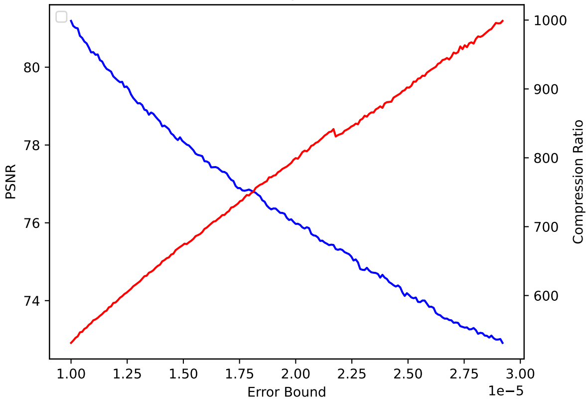
QGRAUP 19 pressio:abs
