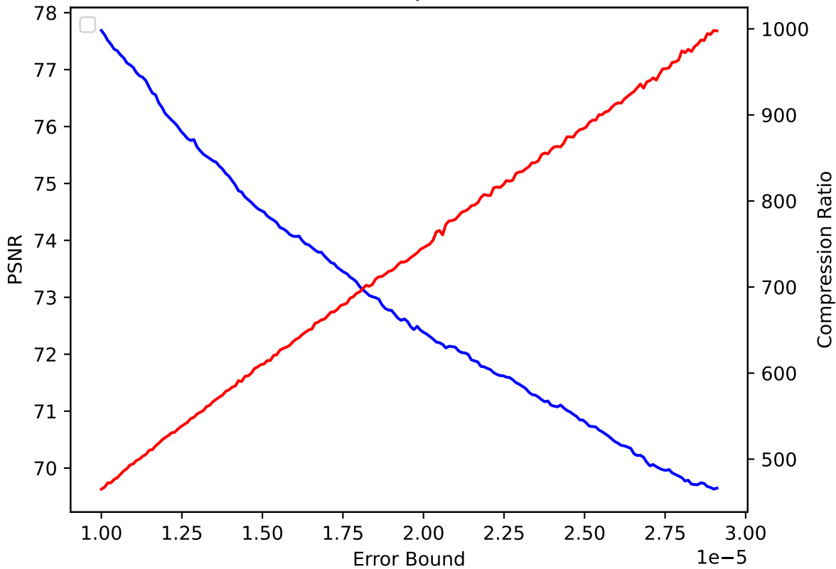
QGRAUP 42 pressio:abs
