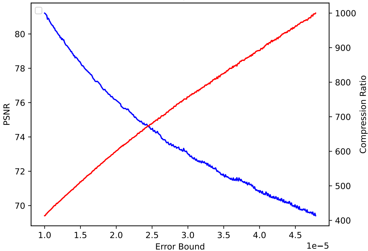
QGRAUP 13 pressio:abs
