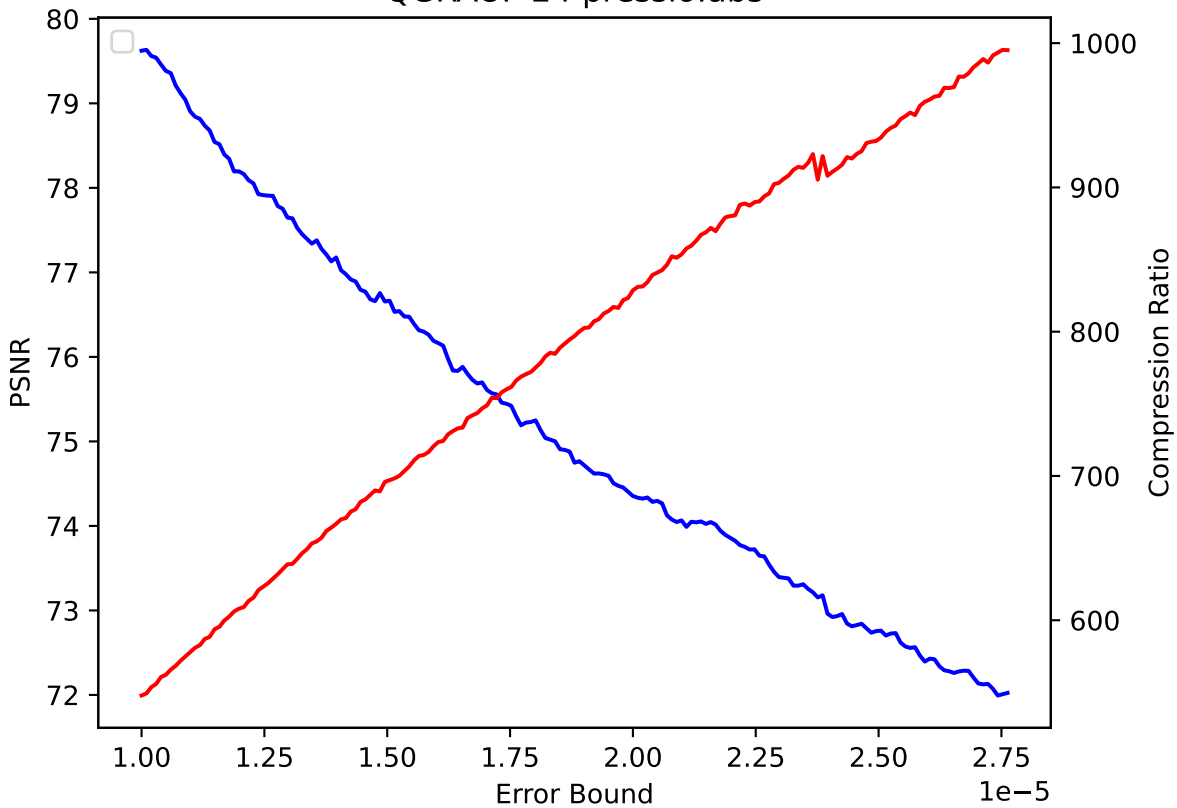
QGRAUP 24 pressio:abs
