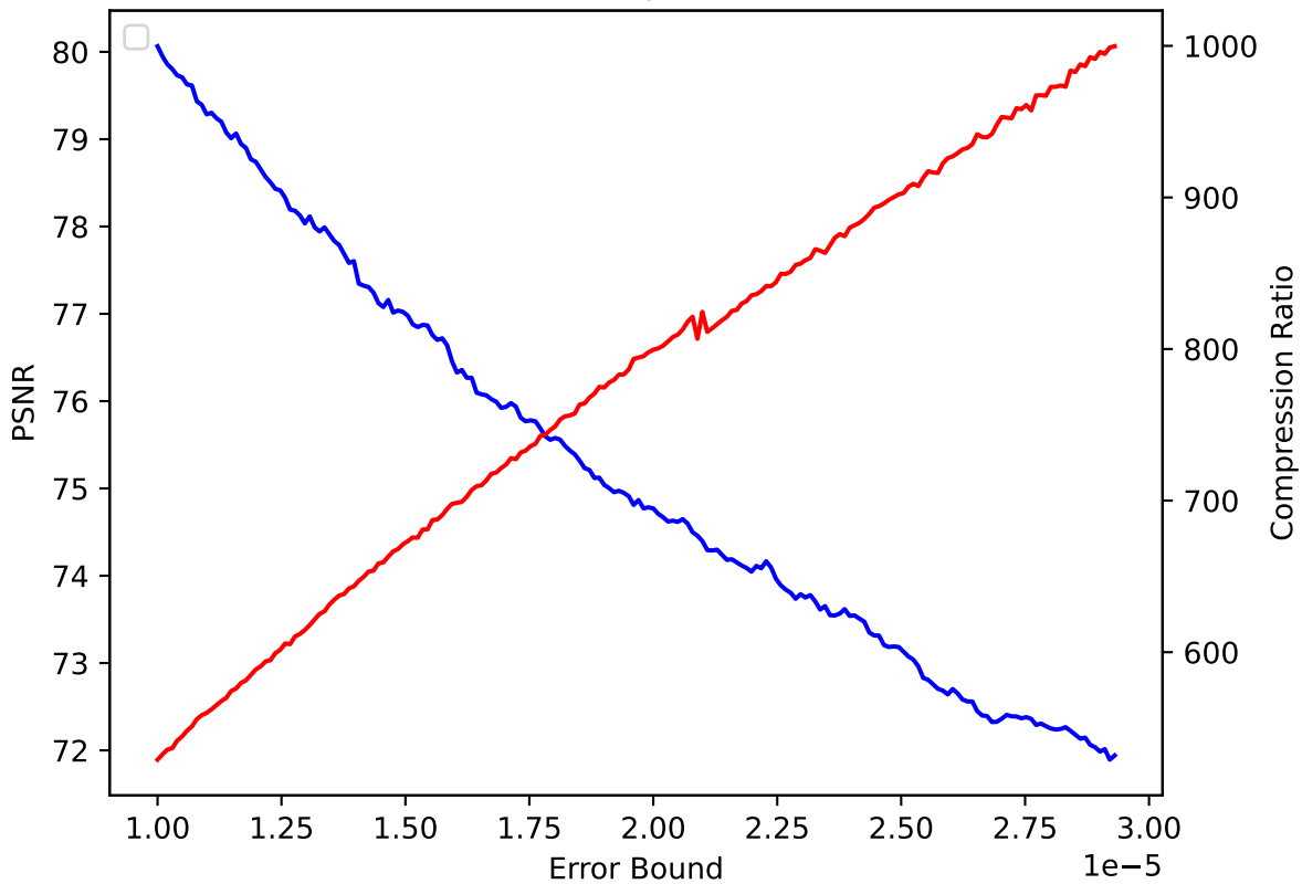
QGRAUP 27 pressio:abs
