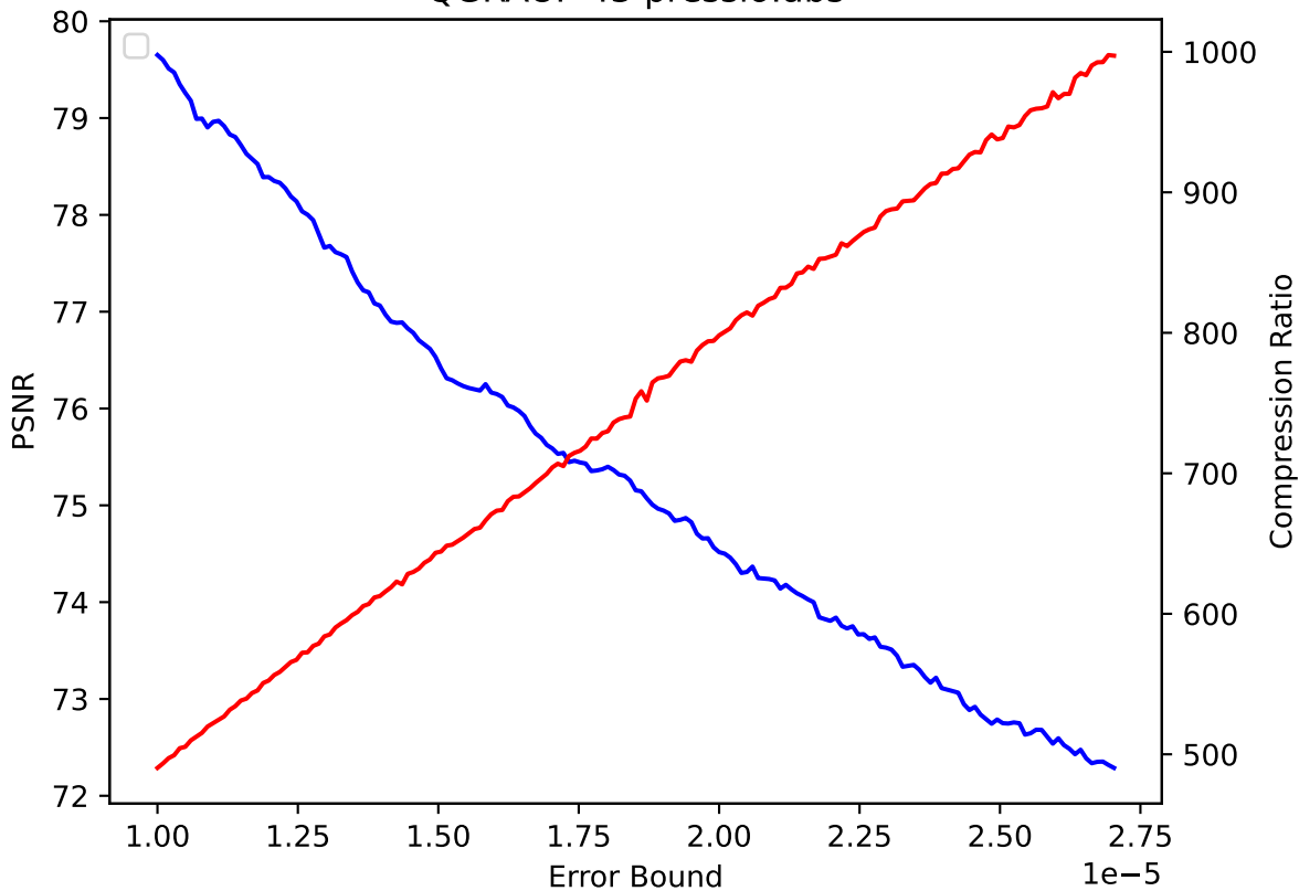
QGRAUP 43 pressio:abs
