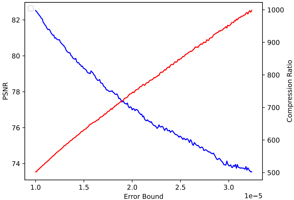
QGRAUP 21 pressio:abs
