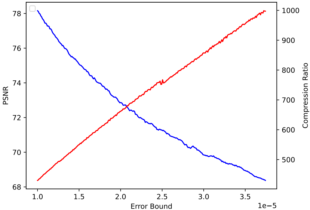
QGRAUP 35 pressio:abs
