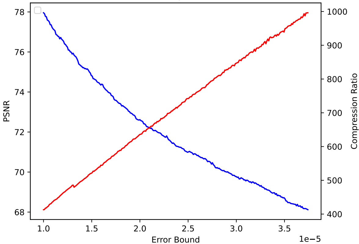
QGRAUP 39 pressio:abs
