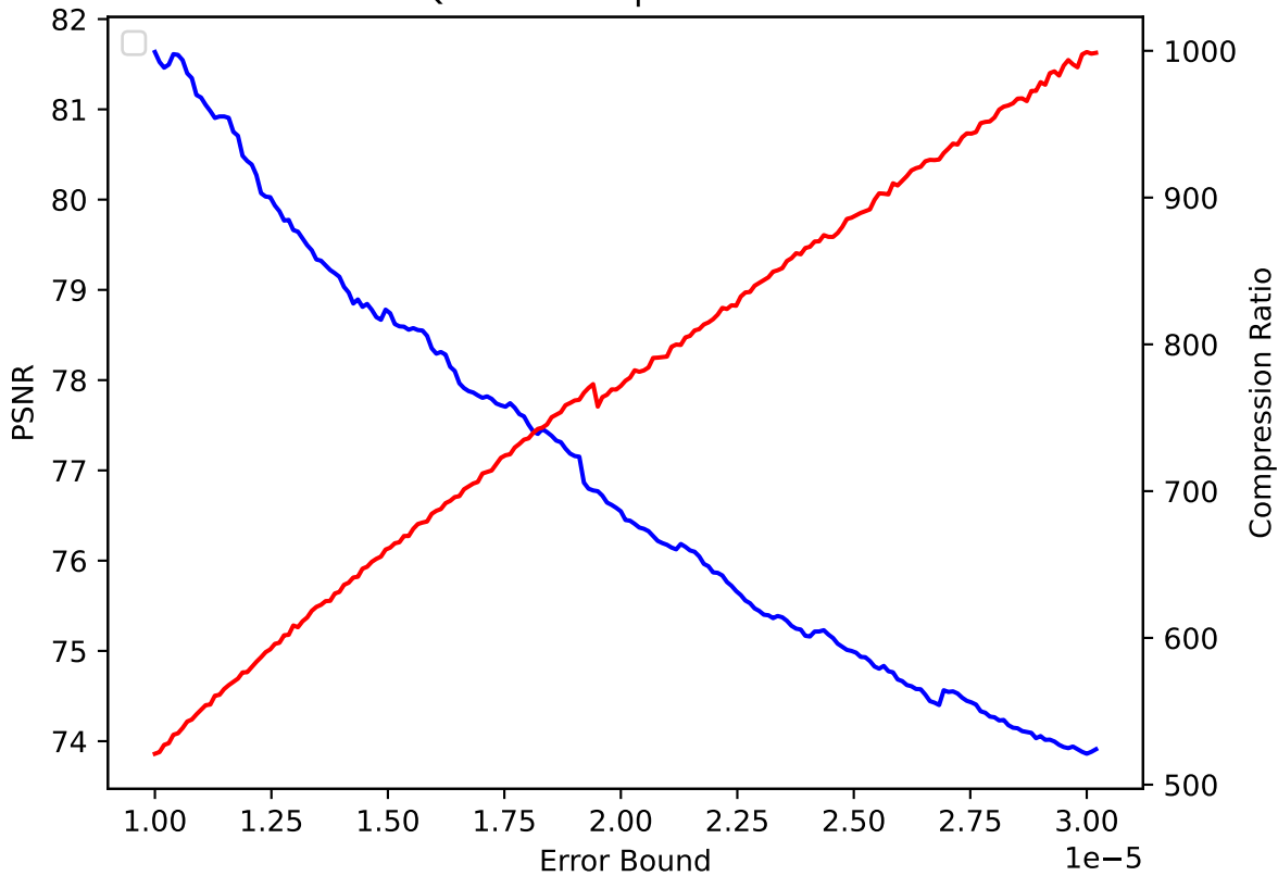
QGRAUP 29 pressio:abs
