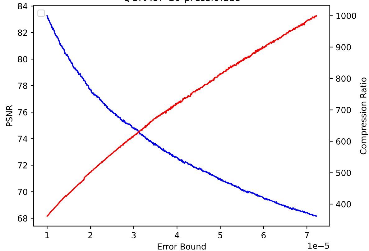
QGRAUP 10 pressio:abs
