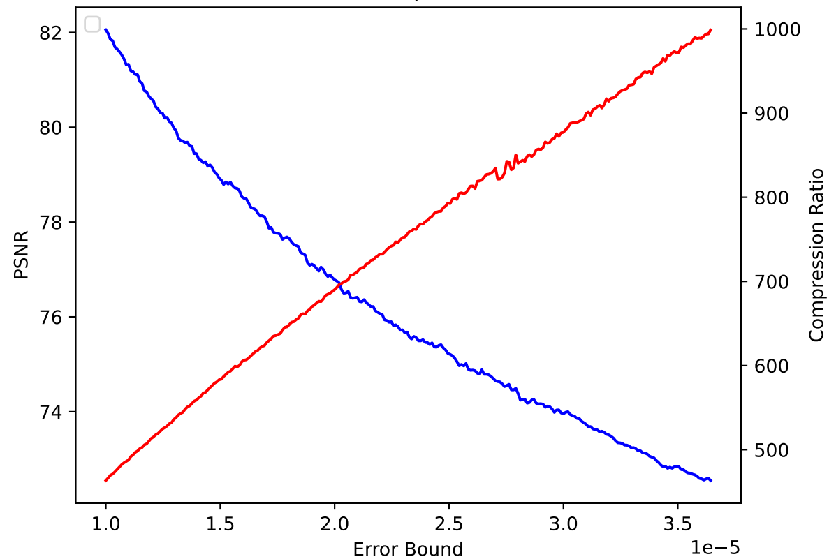
QGRAUP 14 pressio:abs
