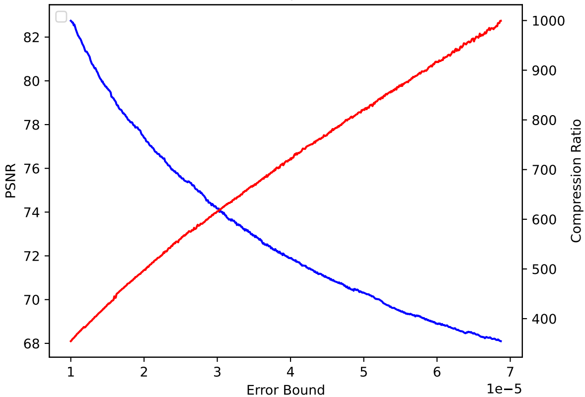
QGRAUP 11 pressio:abs
