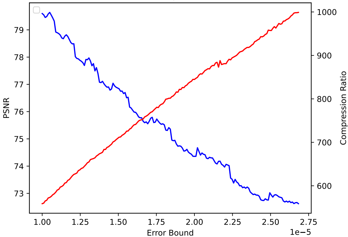
QGRAUP 25 pressio:abs
