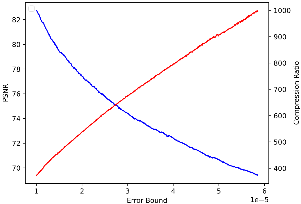
QGRAUP 12 pressio:abs
