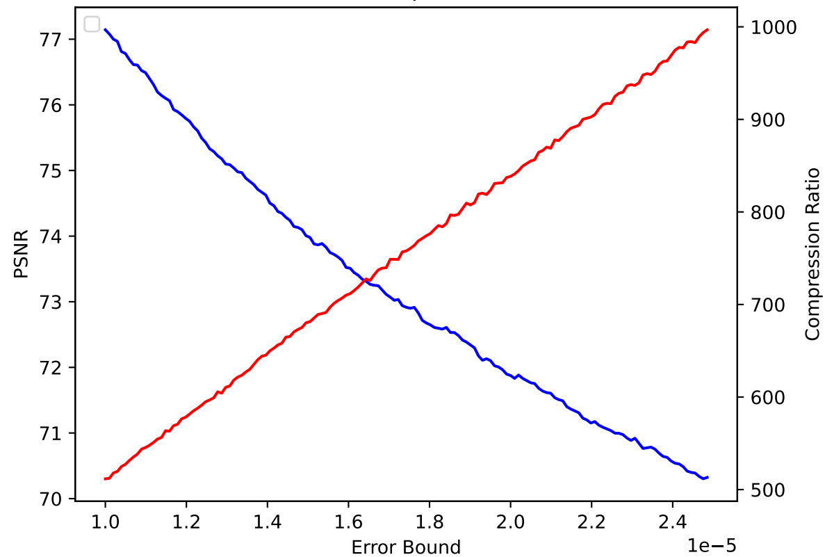
QGRAUP 46 pressio:abs
