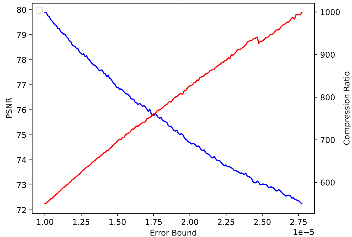
QGRAUP 26 pressio:abs
