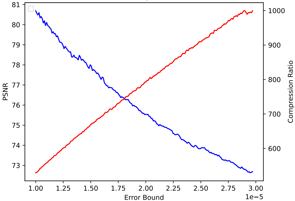
QGRAUP 23 pressio:abs
