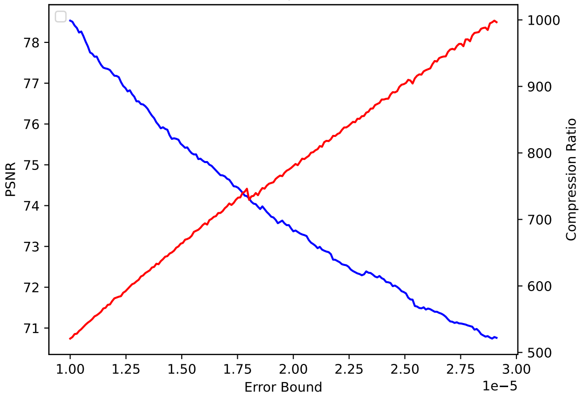
QGRAUP 30 pressio:abs
