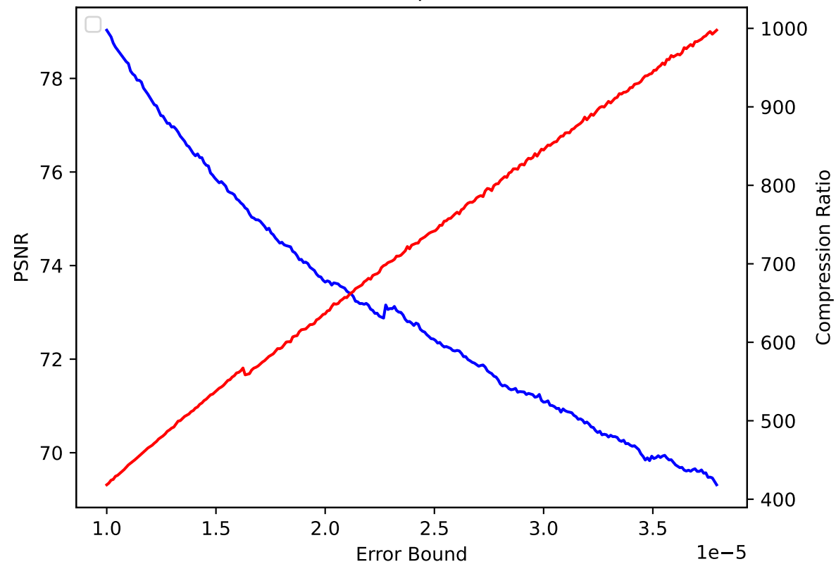
QGRAUP 36 pressio:abs
