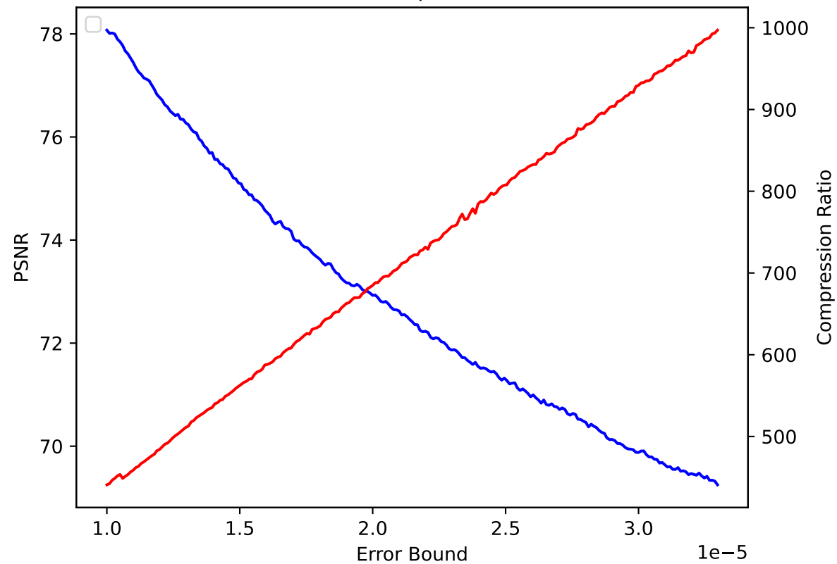
QGRAUP 40 pressio:abs
