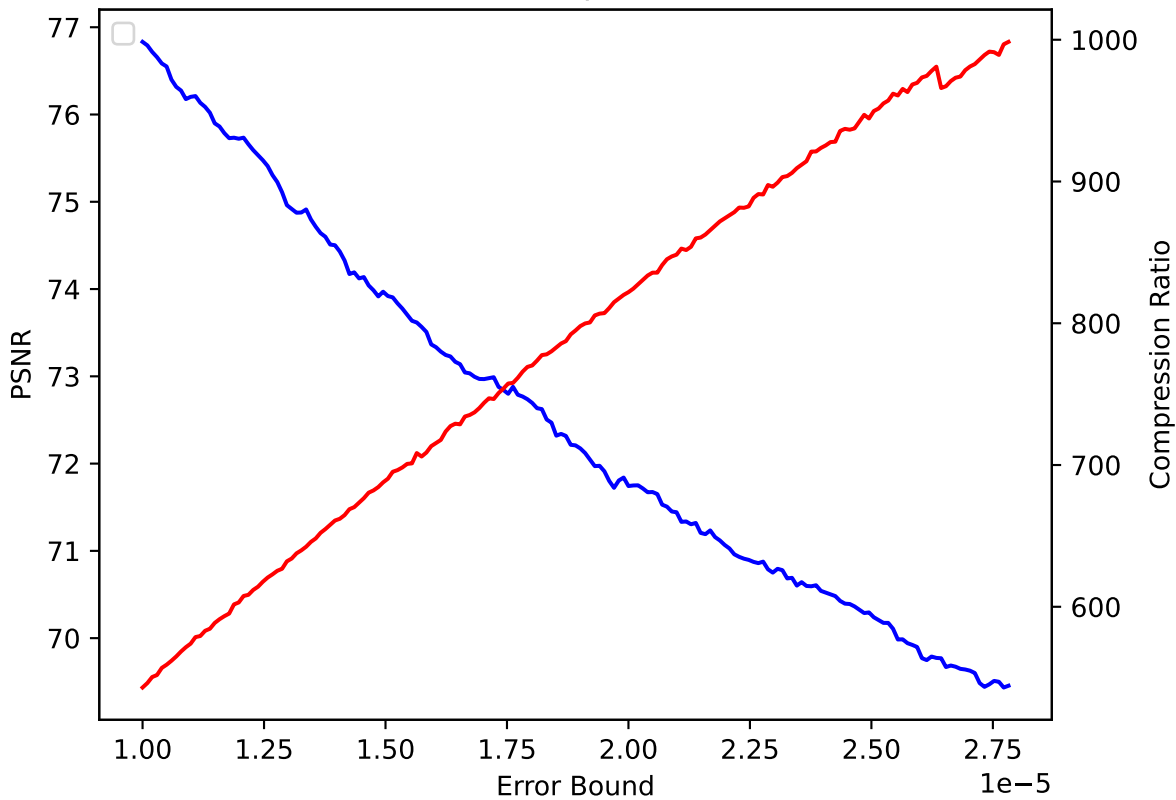
QGRAUP 18 pressio:abs
