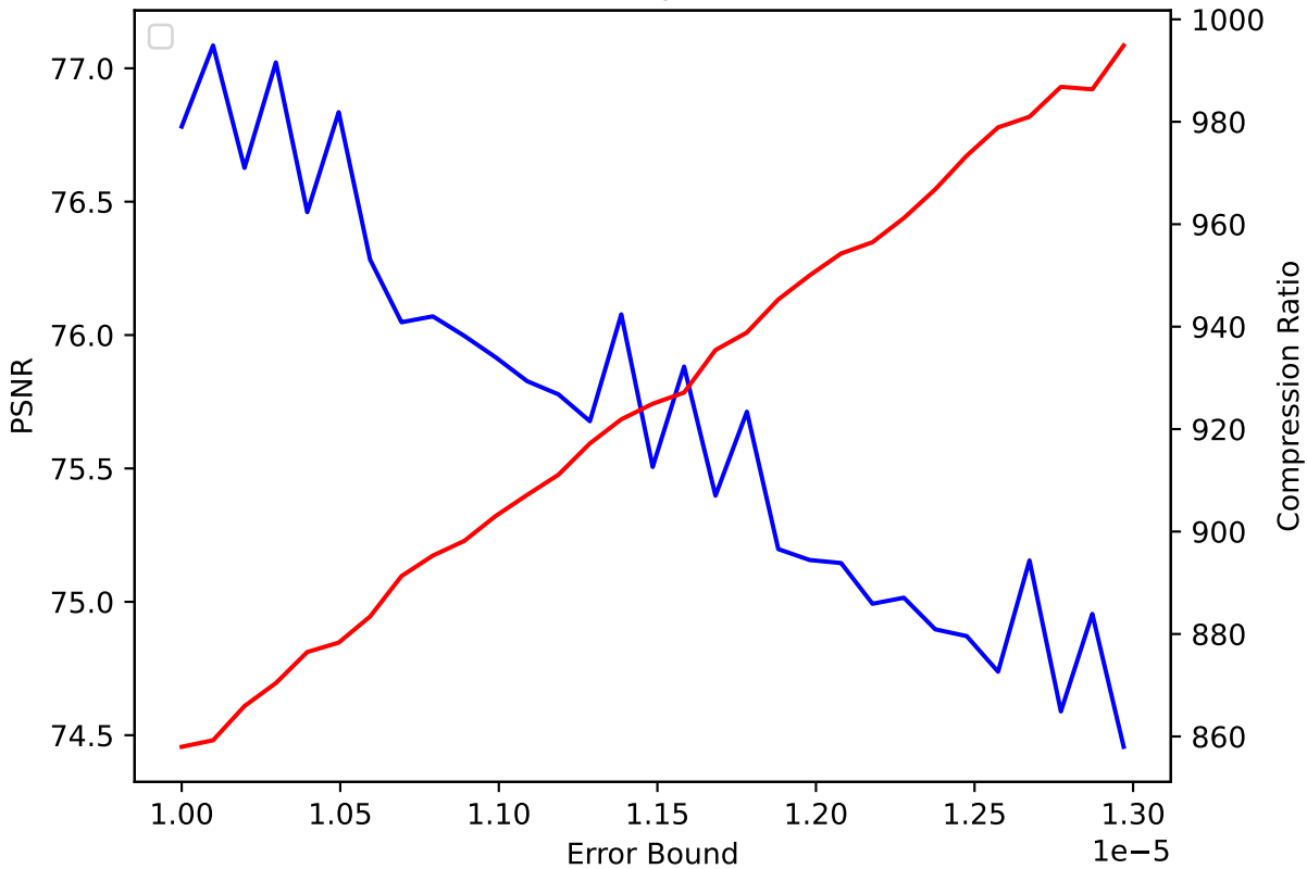
QGRAUP 04 pressio:abs
