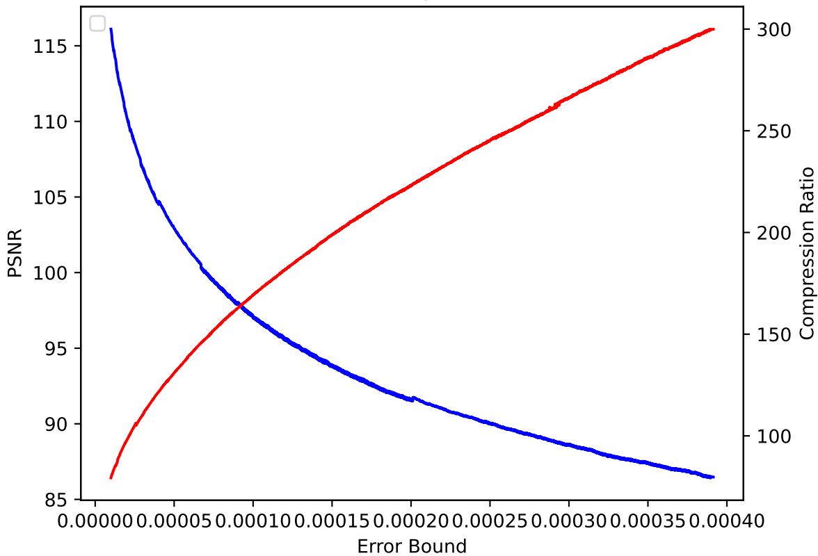
QGRAUP 12 pressio:rel
