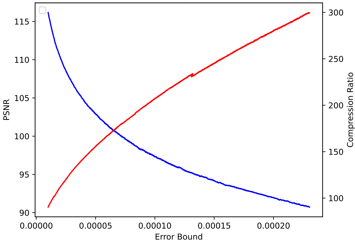
QGRAUP 22 pressio:rel
