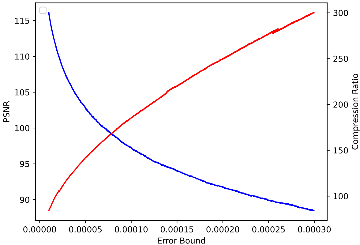
QGRAUP 14 pressio:rel
