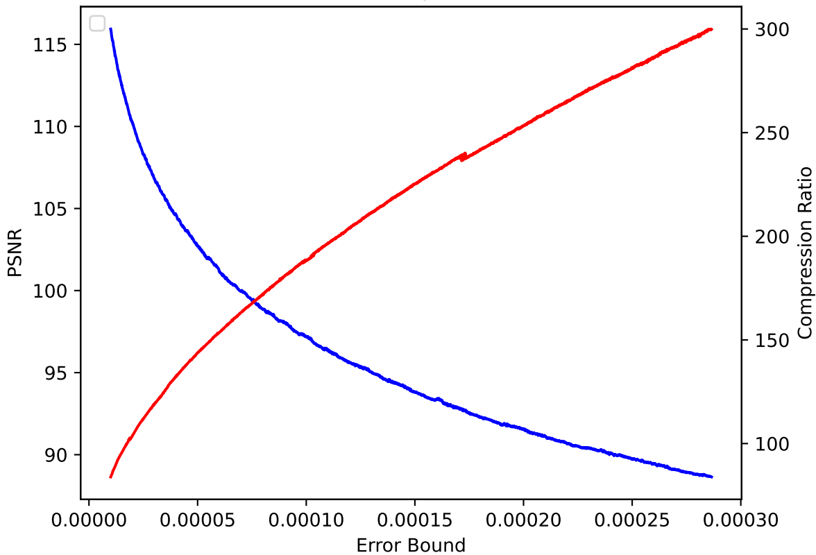
QGRAUP 23 pressio:rel
