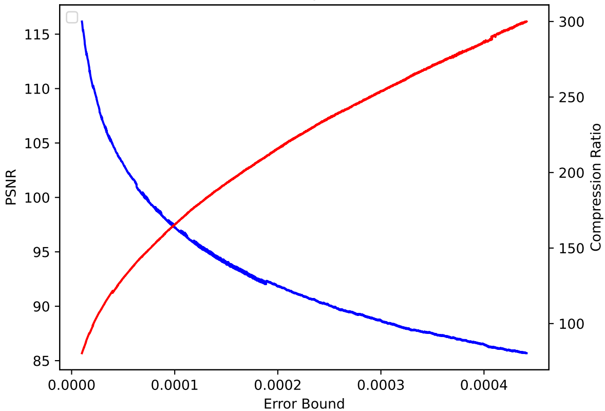
QGRAUP 11 pressio:rel
