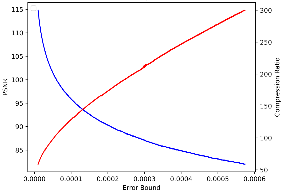
QGRAUP 39 pressio:rel
