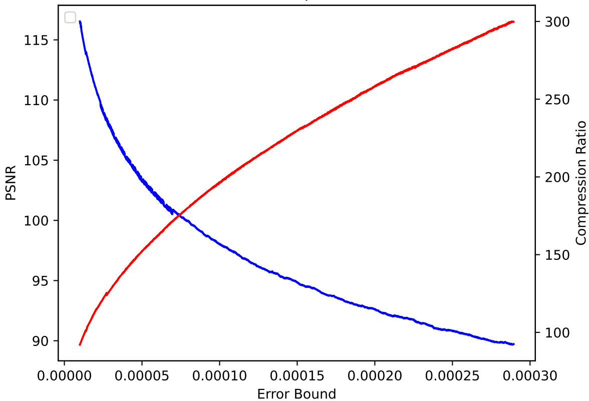
QGRAUP 09 pressio:rel
