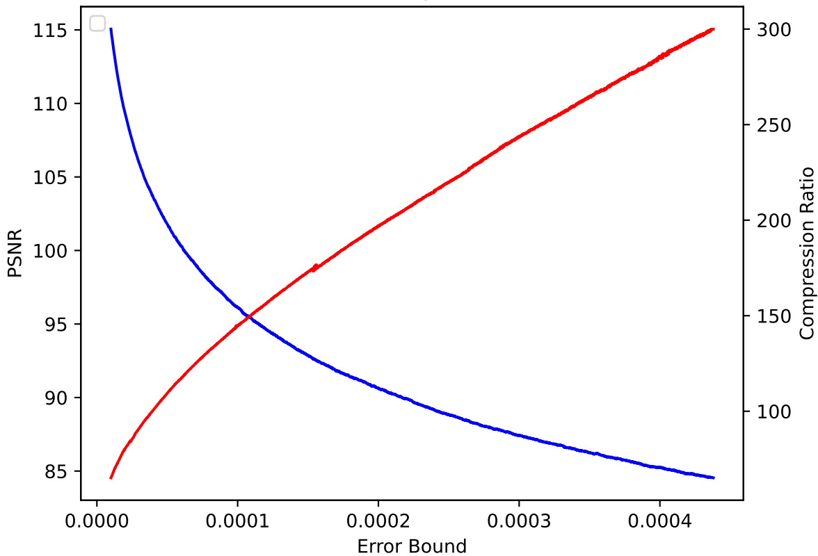
QGRAUP 41 pressio:rel
