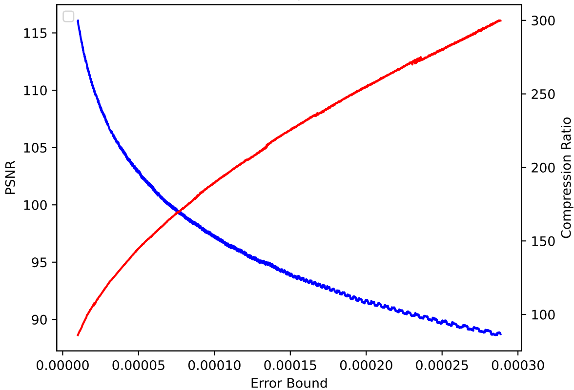
QGRAUP 25 pressio:rel
