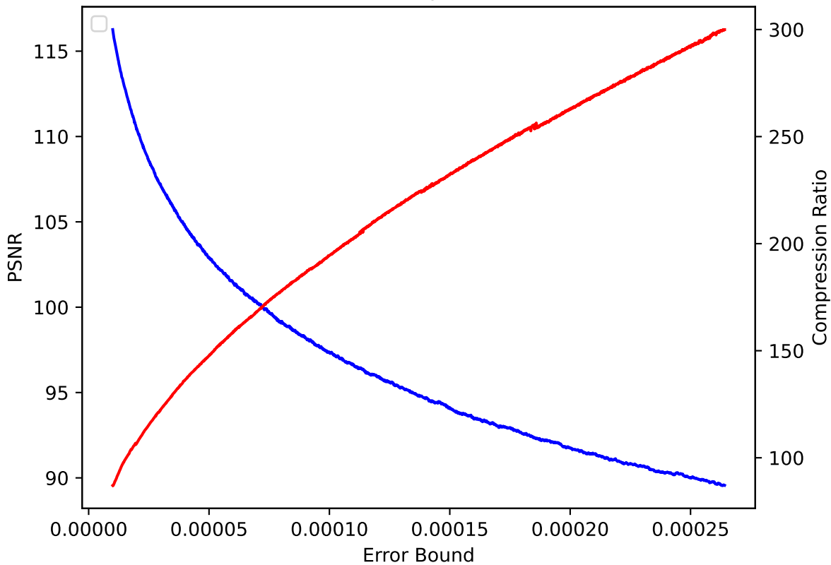
QGRAUP 20 pressio:rel
