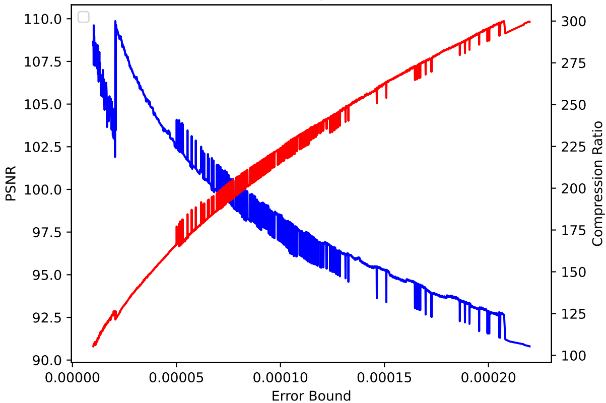
QGRAUP 05 pressio:rel
