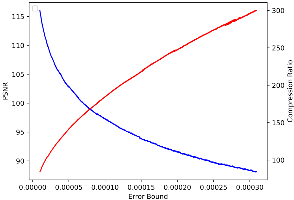
QGRAUP 24 pressio:rel
