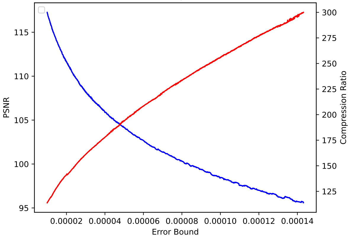
QGRAUP 07 pressio:rel
