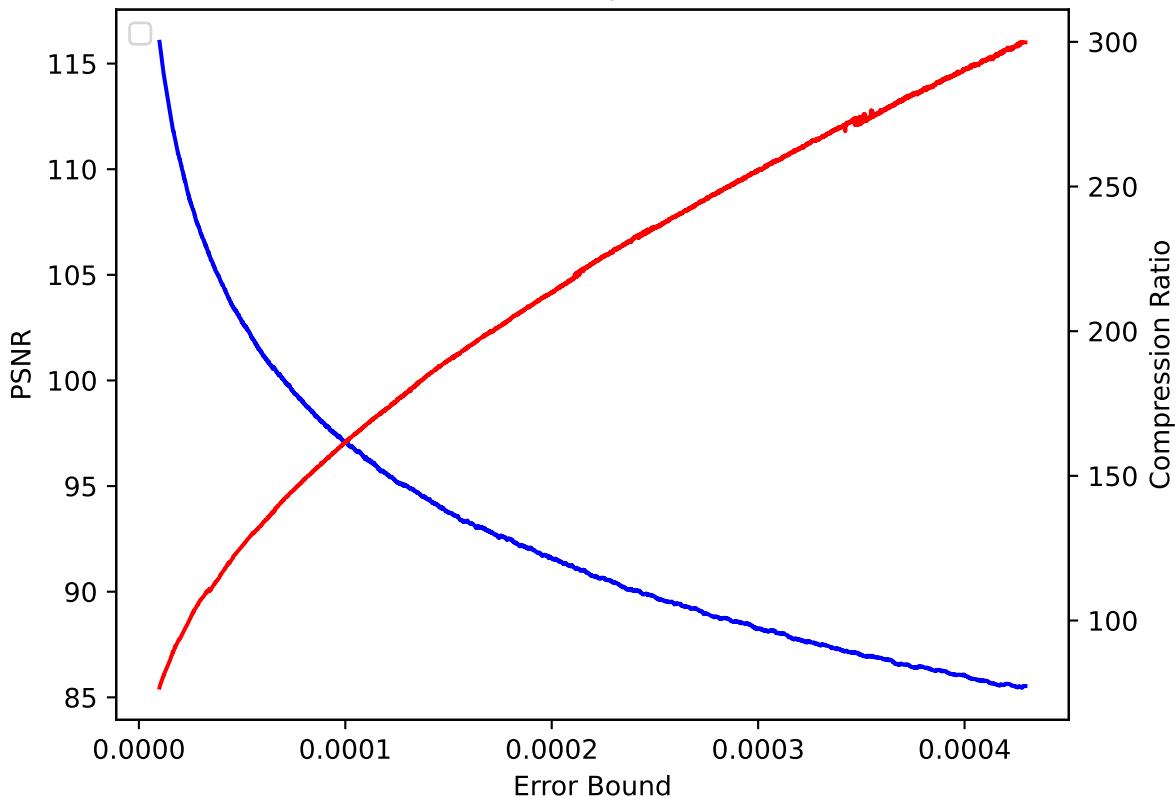
QGRAUP 18 pressio:rel
