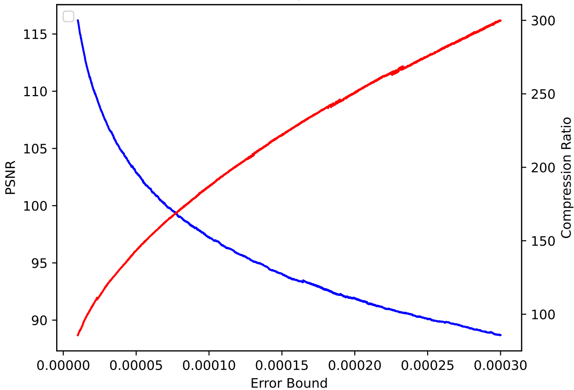
QGRAUP 26 pressio:rel
