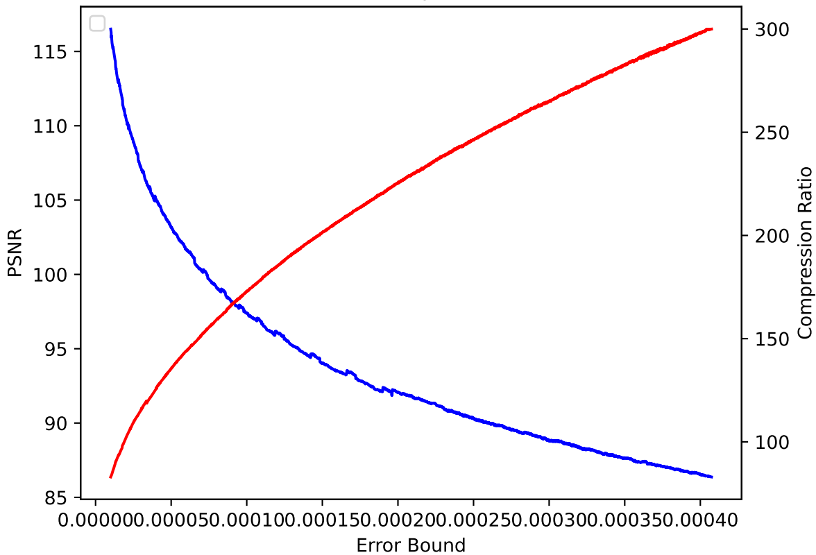
QGRAUP 10 pressio:rel
