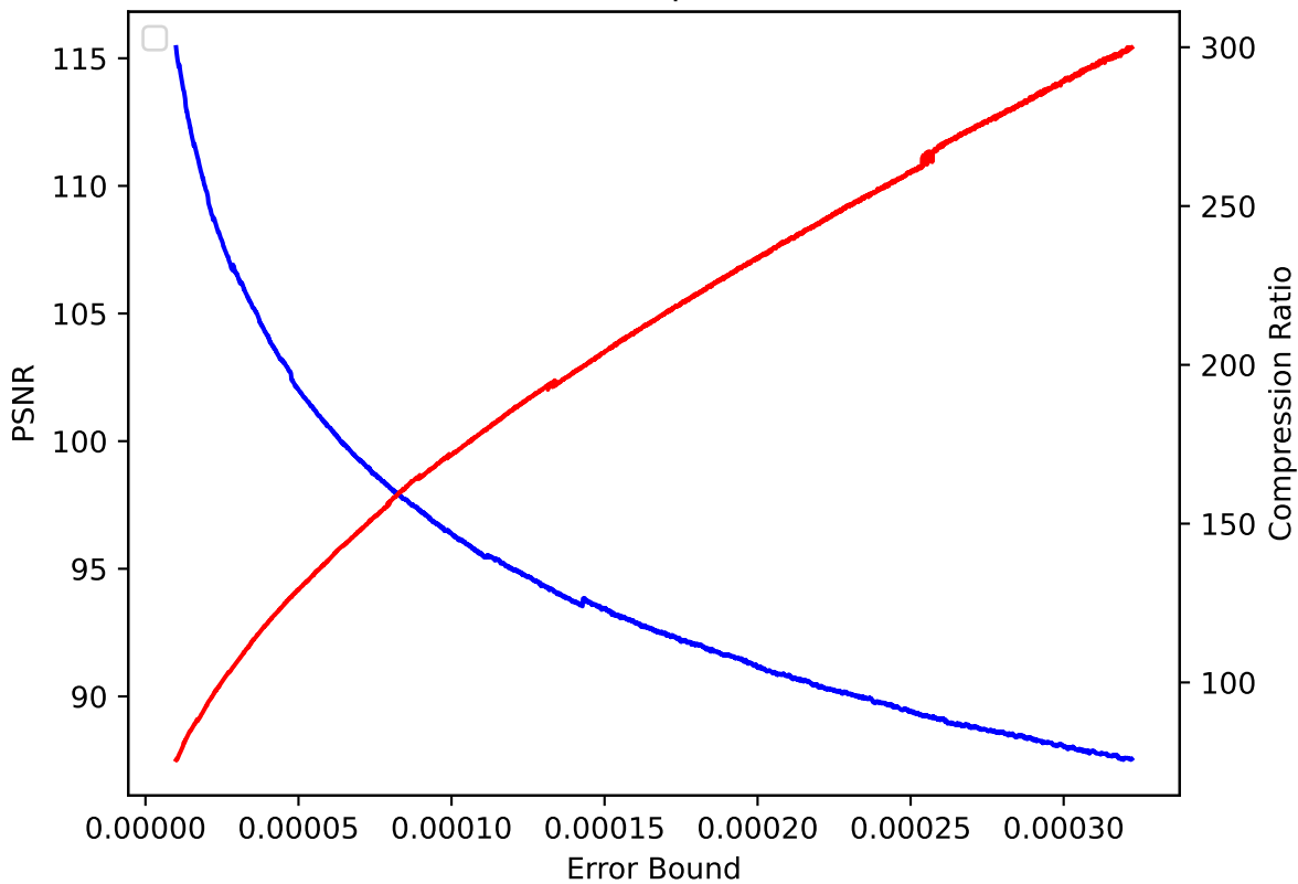
QGRAUP 33 pressio:rel
