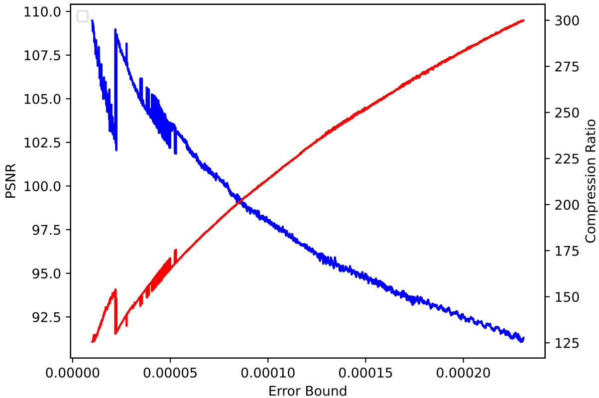
QGRAUP 02 pressio:rel
