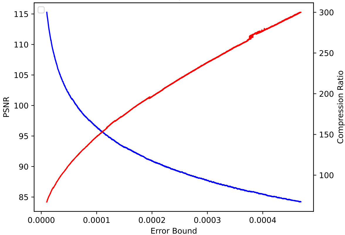
QGRAUP 34 pressio:rel
