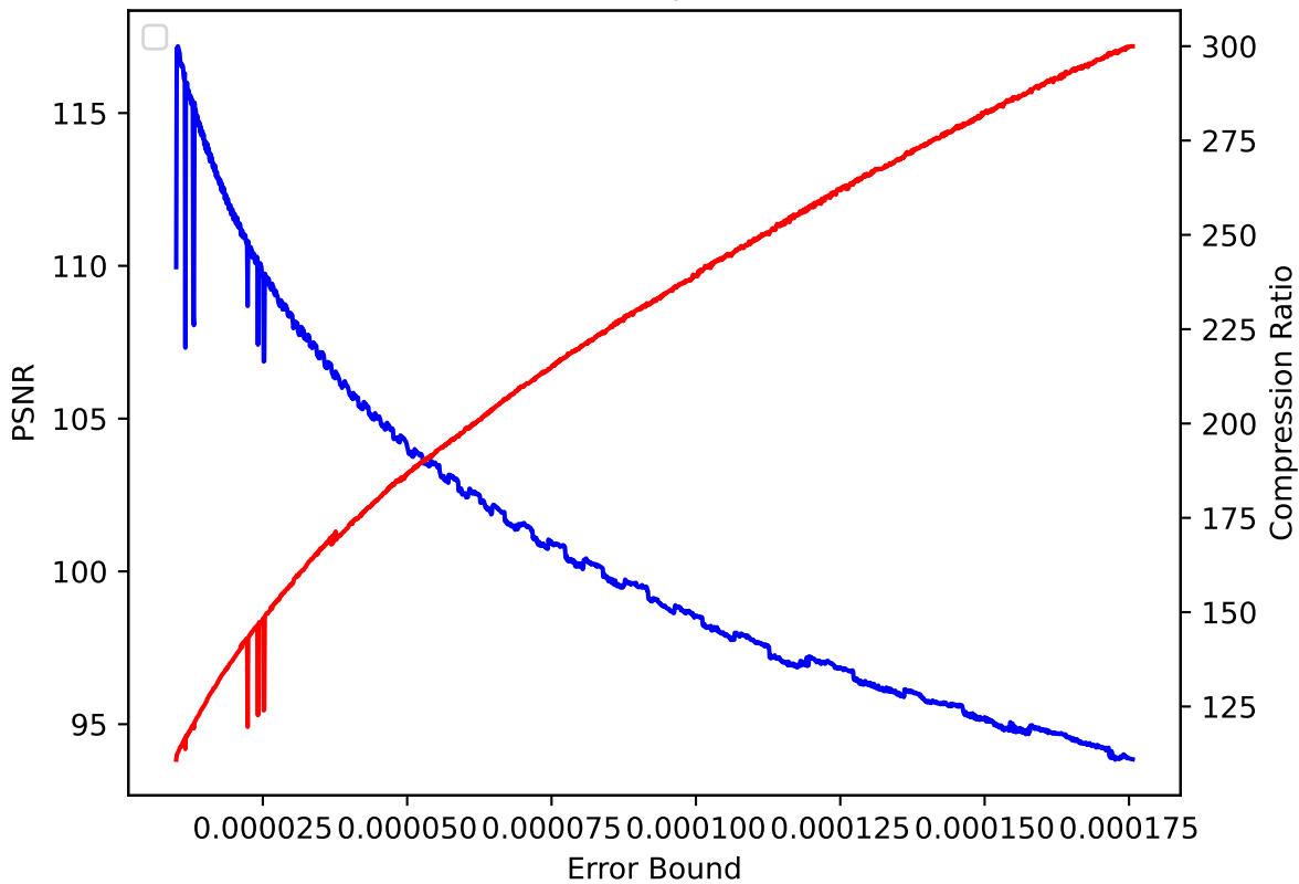
QGRAUP 04 pressio:rel
