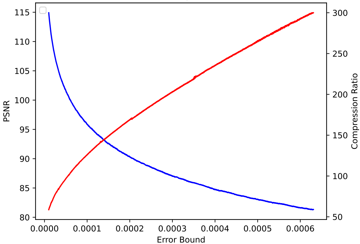
QGRAUP 37 pressio:rel
