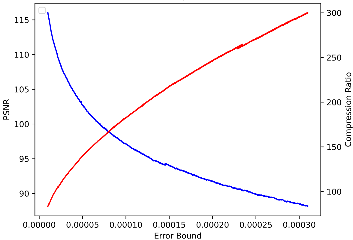
QGRAUP 27 pressio:rel
