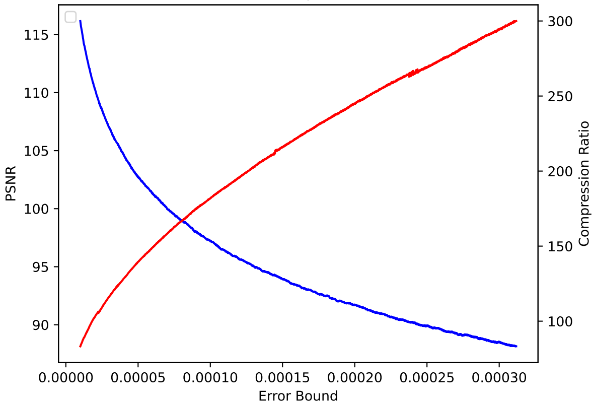
QGRAUP 15 pressio:rel
