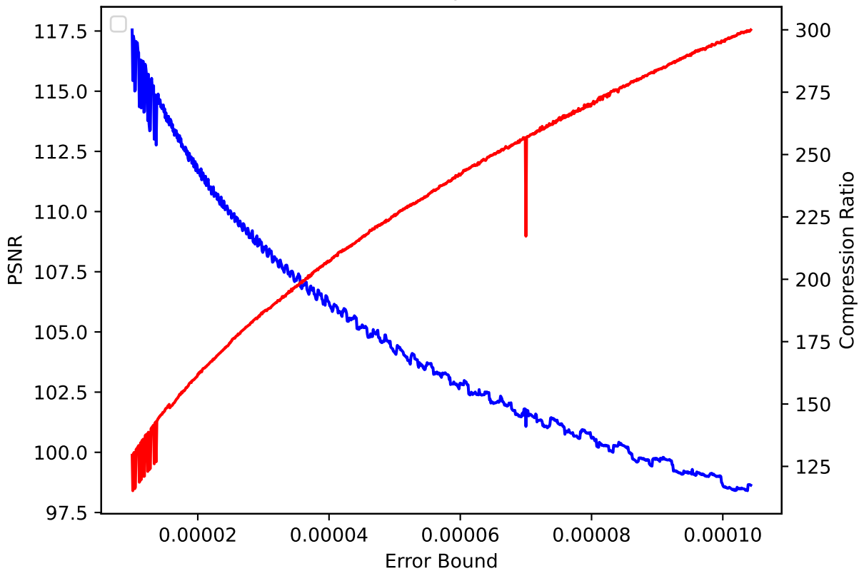
QGRAUP 03 pressio:rel
