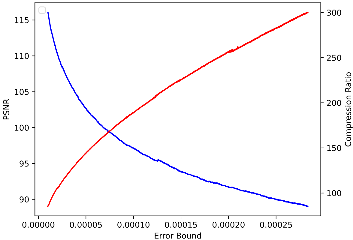
QGRAUP 17 pressio:rel
