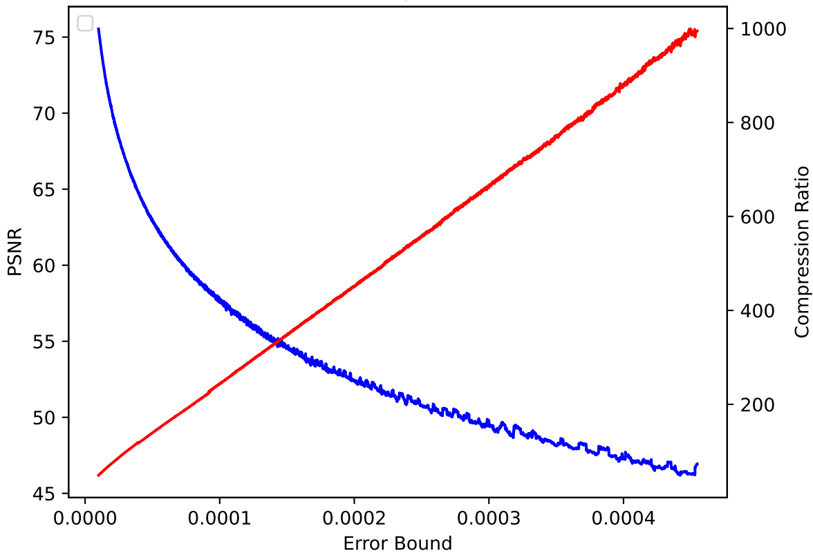
QVAPOR 05 pressio:abs
