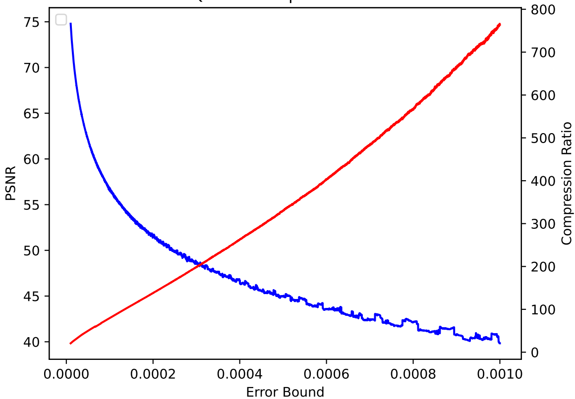
QVAPOR 38 pressio:abs
