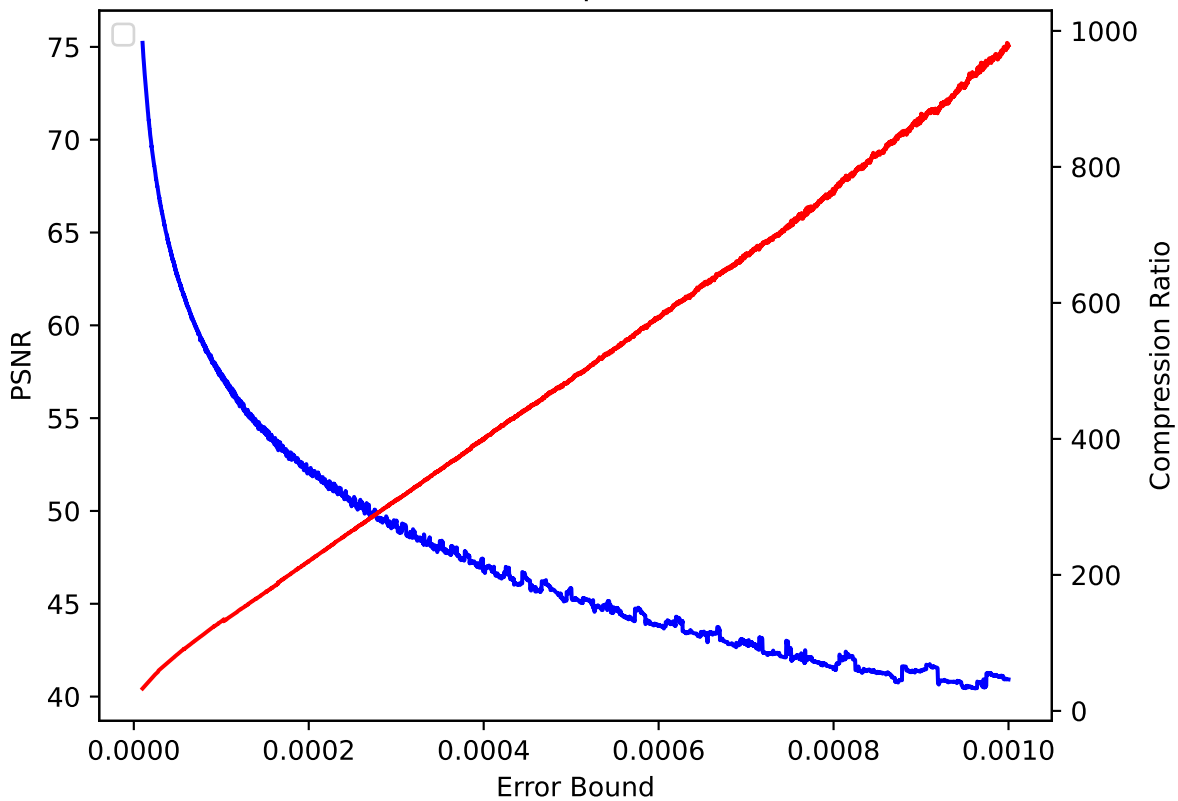
QVAPOR 08 pressio:abs
