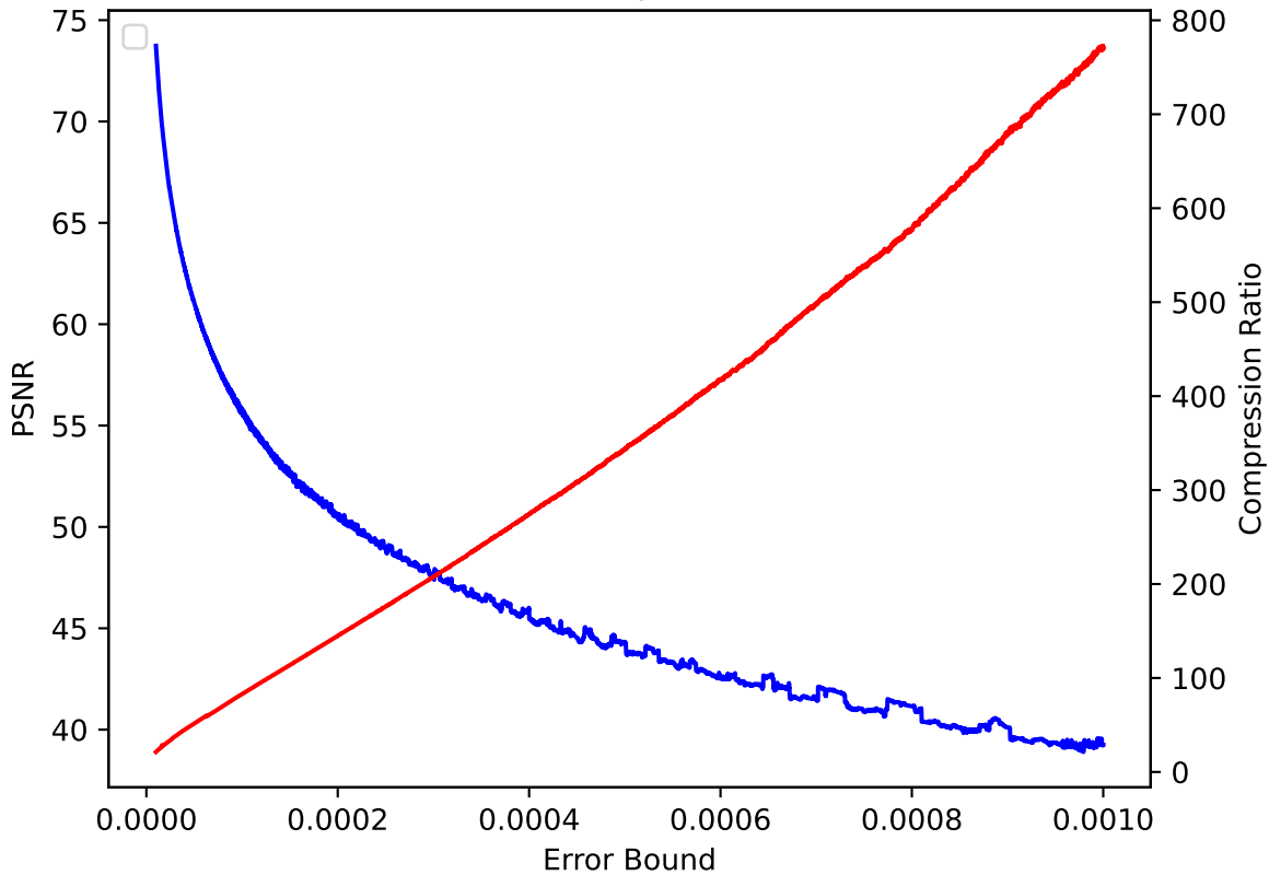
QVAPOR 47 pressio:abs
