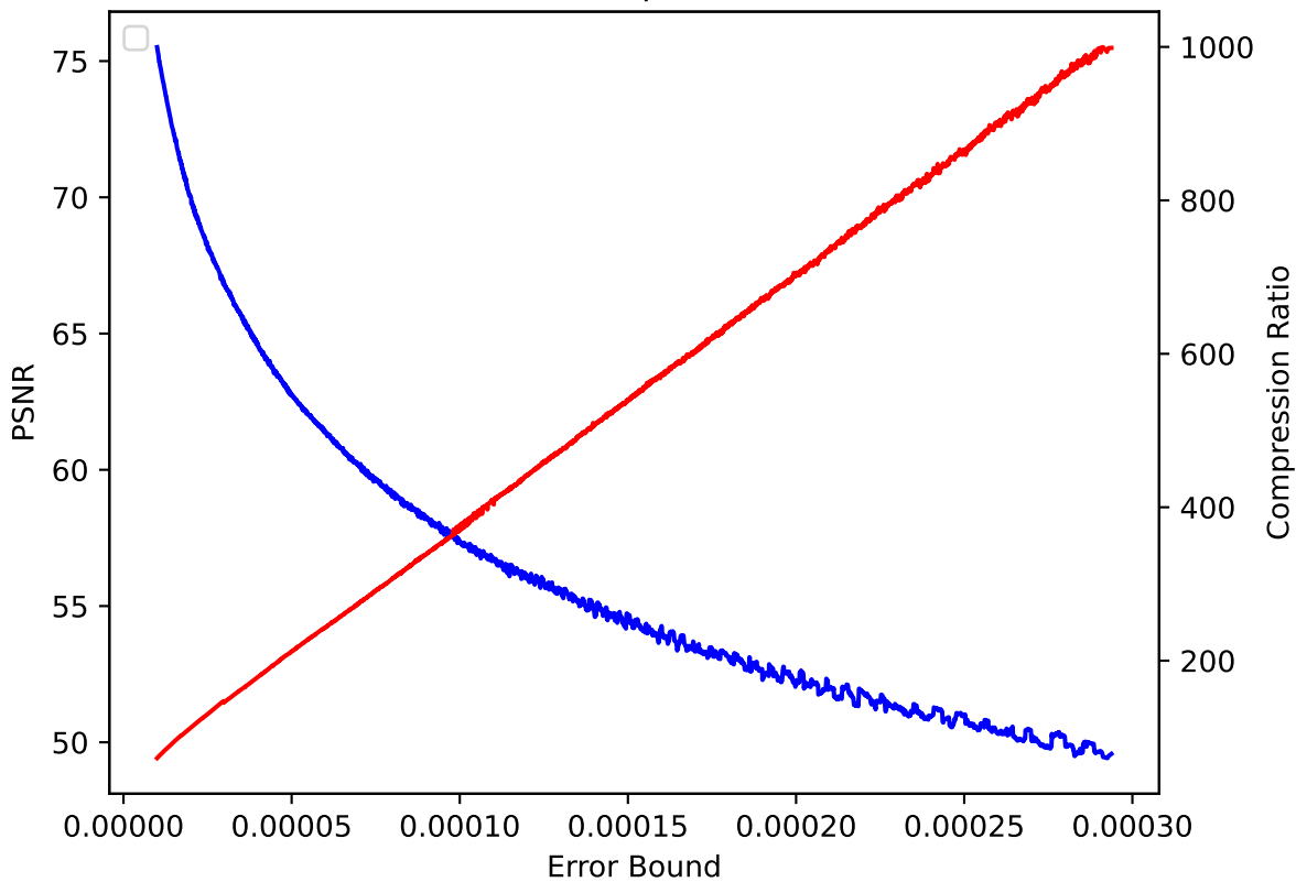
QVAPOR 02 pressio:abs
