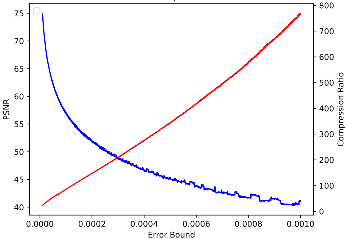
QVAPOR 21 pressio:abs
