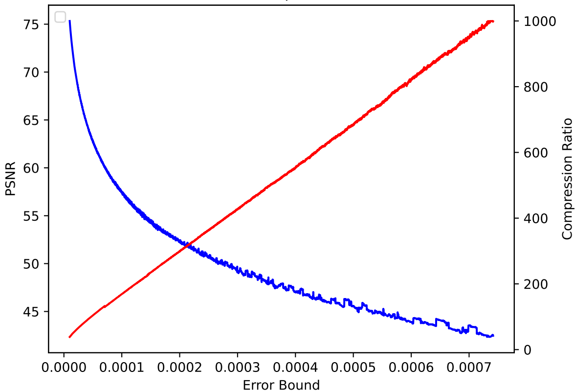
QVAPOR 07 pressio:abs
