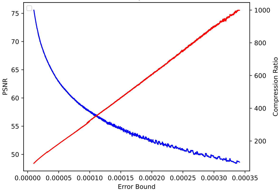
QVAPOR 03 pressio:abs
