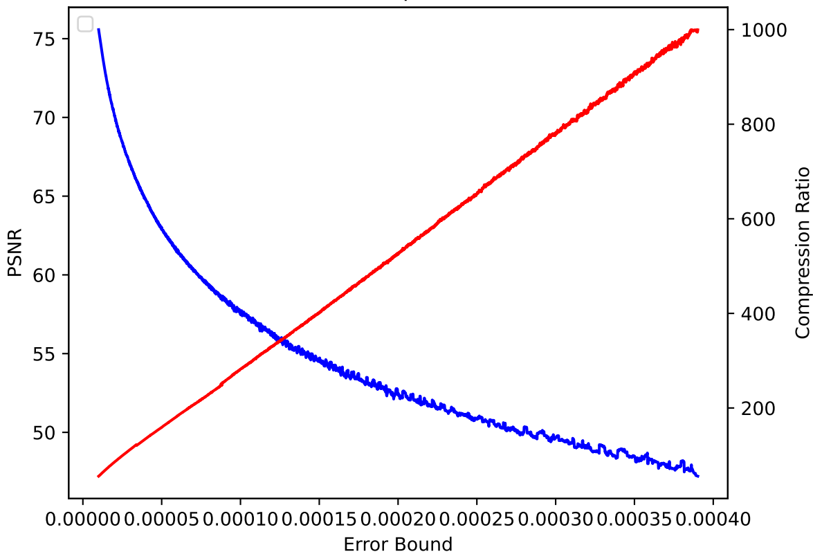
QVAPOR 04 pressio:abs
