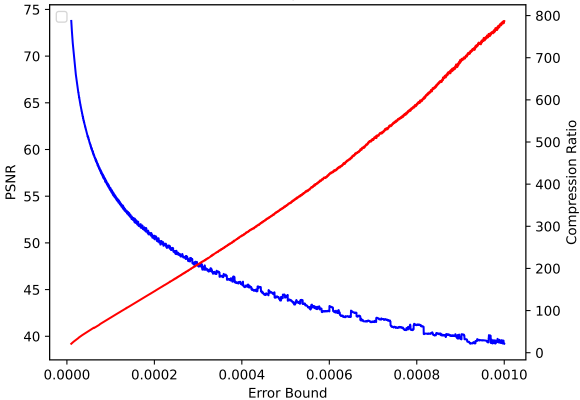
QVAPOR 46 pressio:abs
