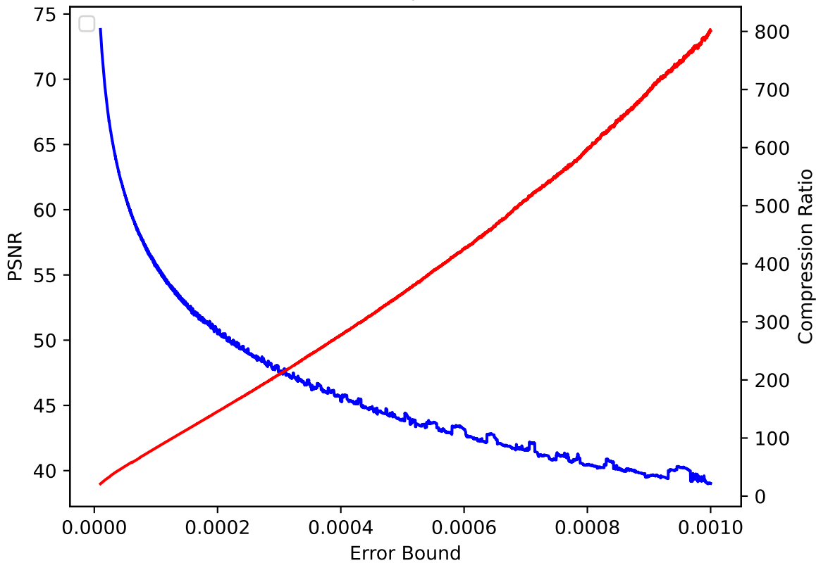
QVAPOR 45 pressio:abs
