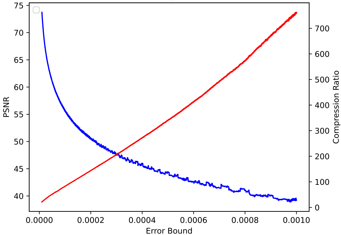
QVAPOR 48 pressio:abs
