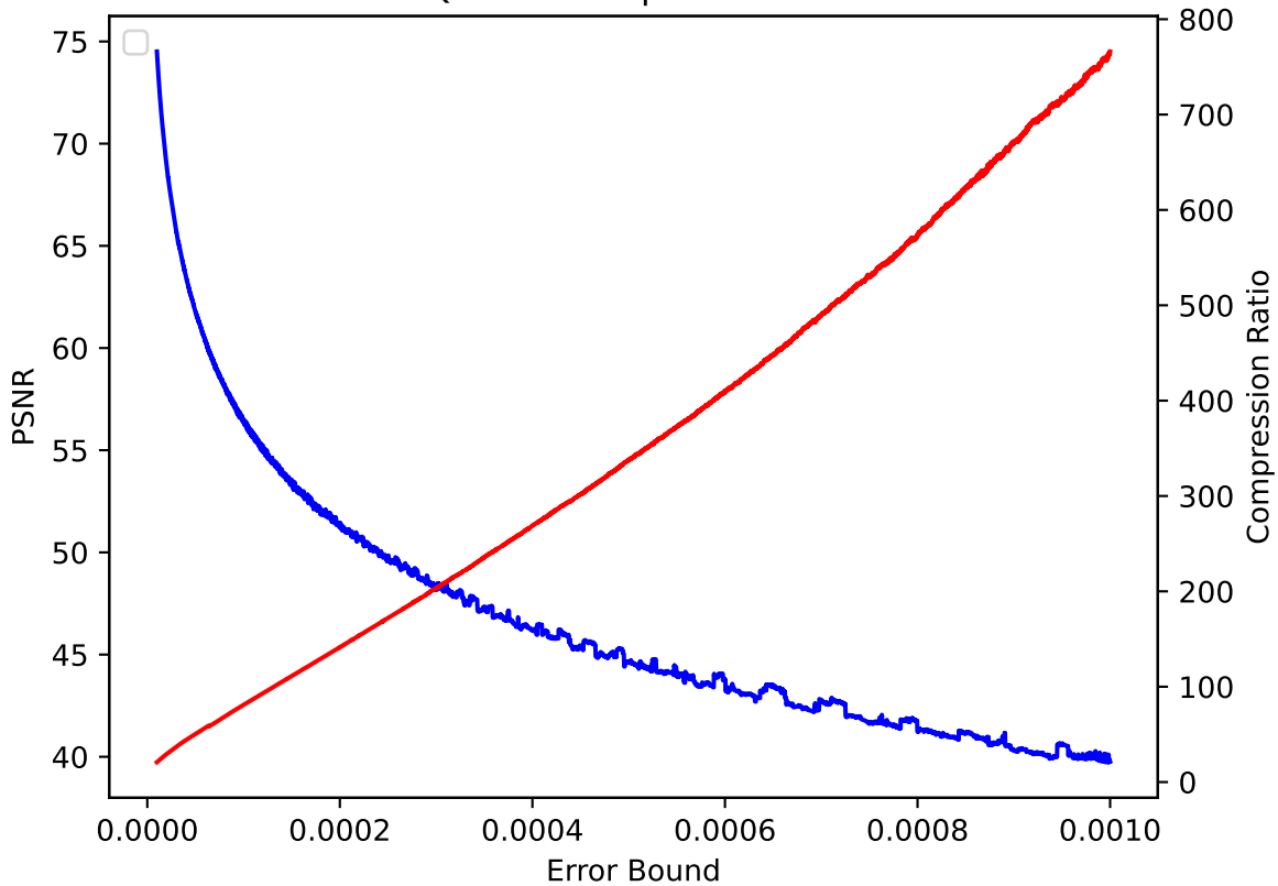
QVAPOR 43 pressio:abs
