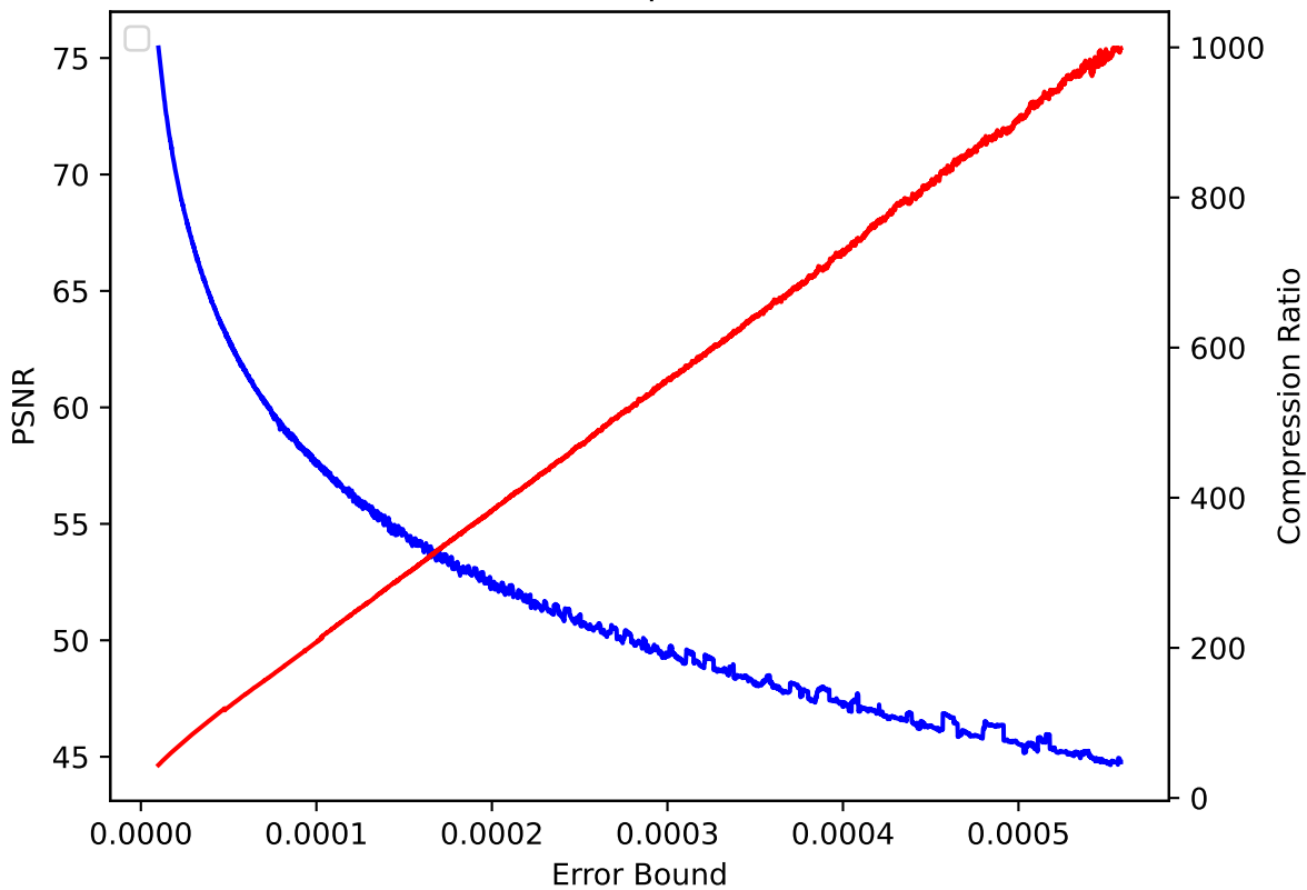
QVAPOR 06 pressio:abs
