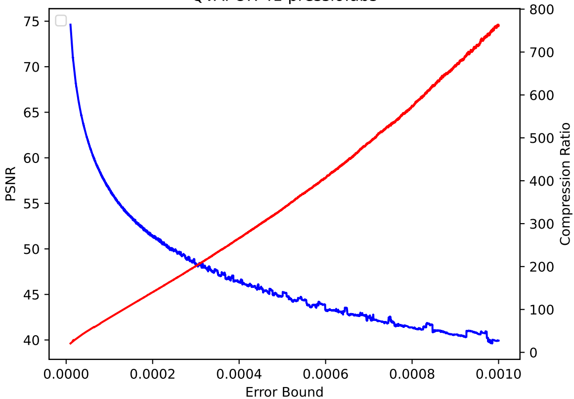
QVAPOR 41 pressio:abs
