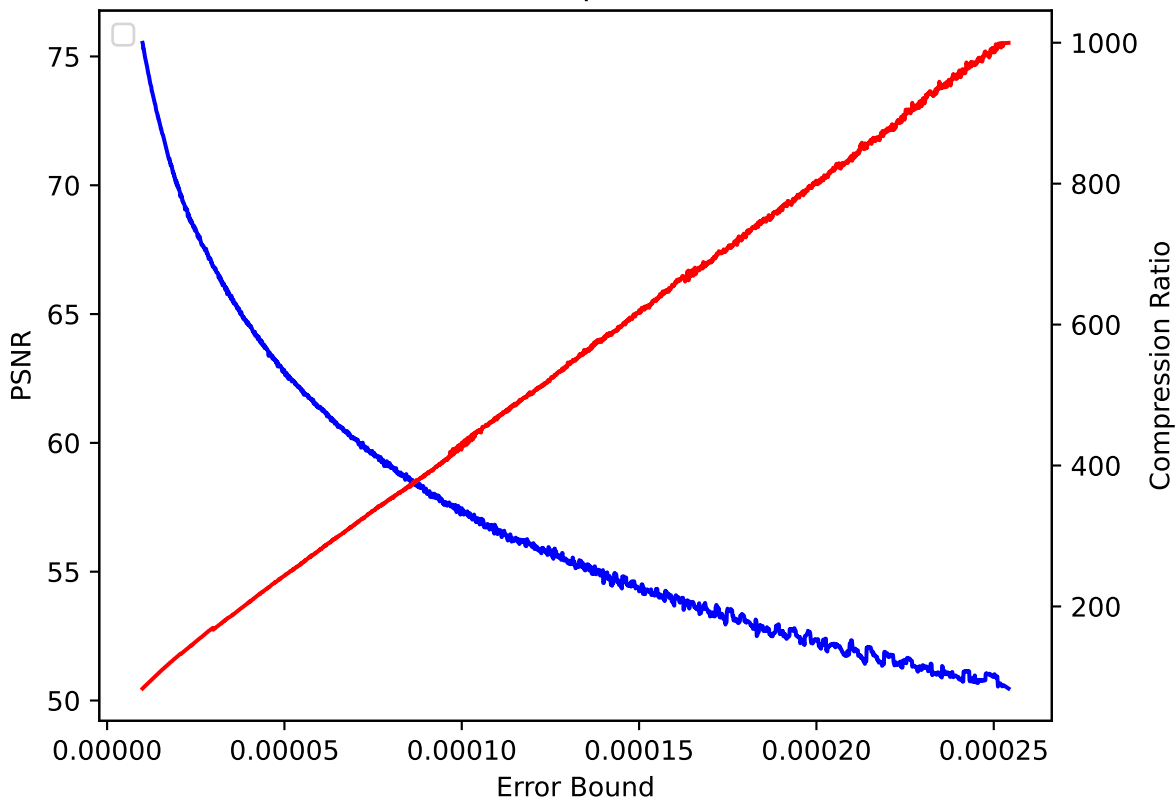
QVAPOR 01 pressio:abs
