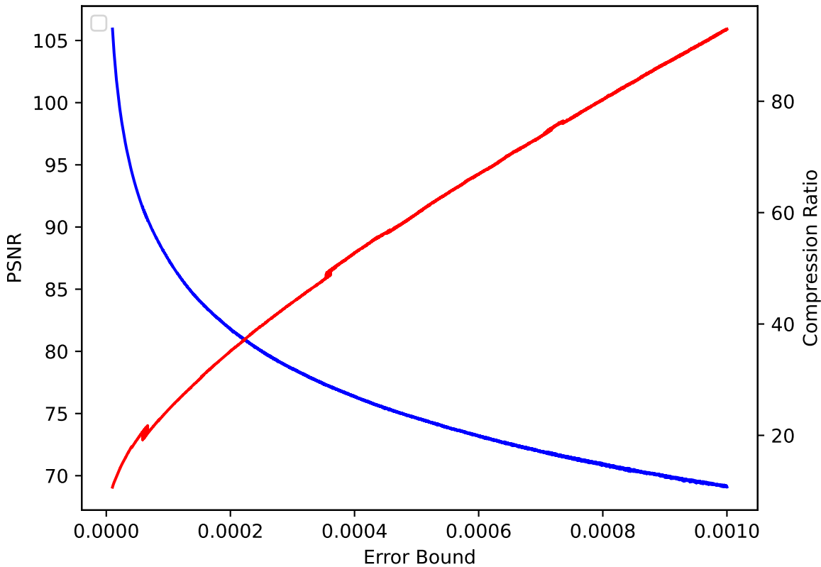
QVAPOR 04 pressio:rel
