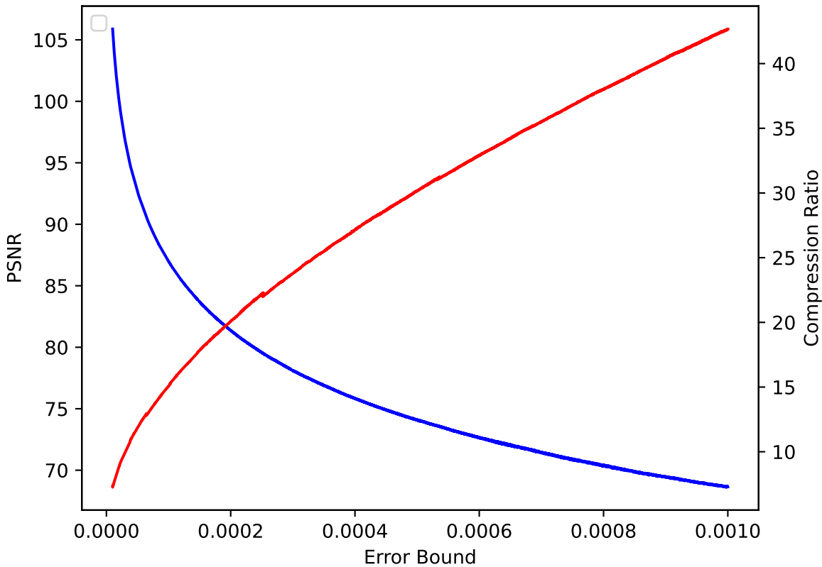
QVAPOR 09 pressio:rel
