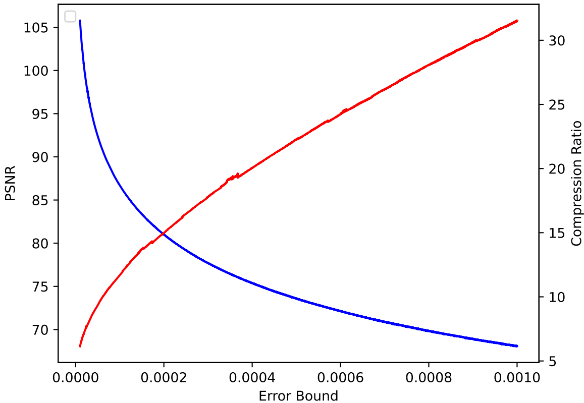
QVAPOR 38 pressio:rel
