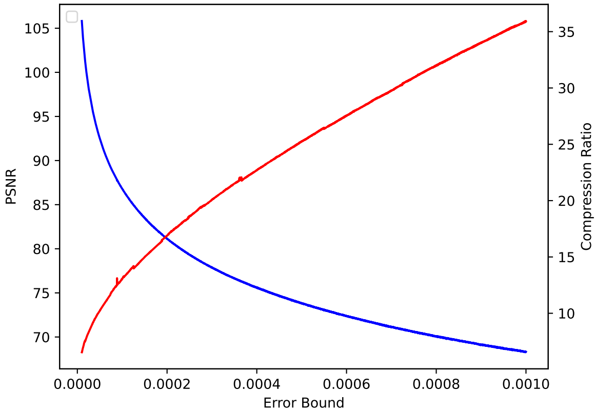
QVAPOR 17 pressio:rel
