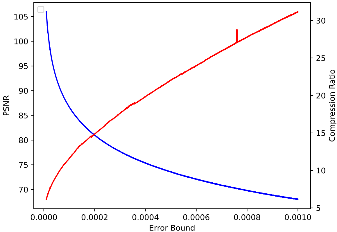
QVAPOR 43 pressio:rel
