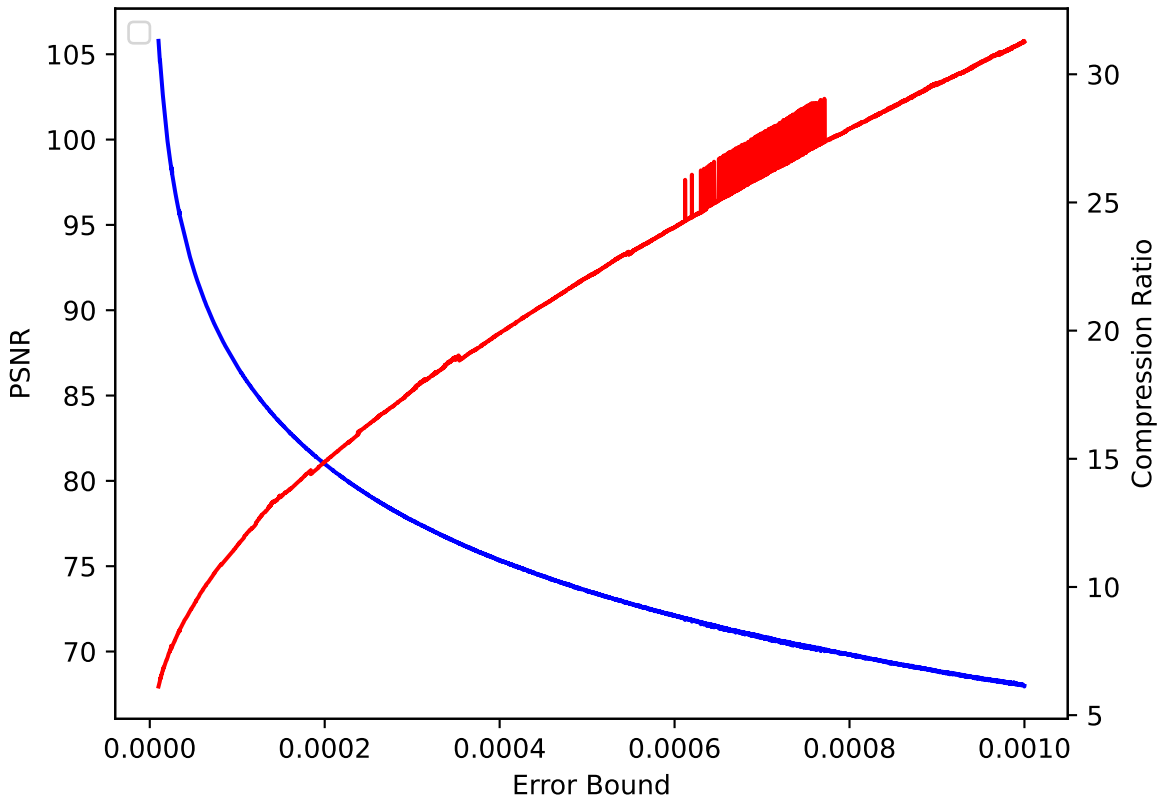
QVAPOR 41 pressio:rel
