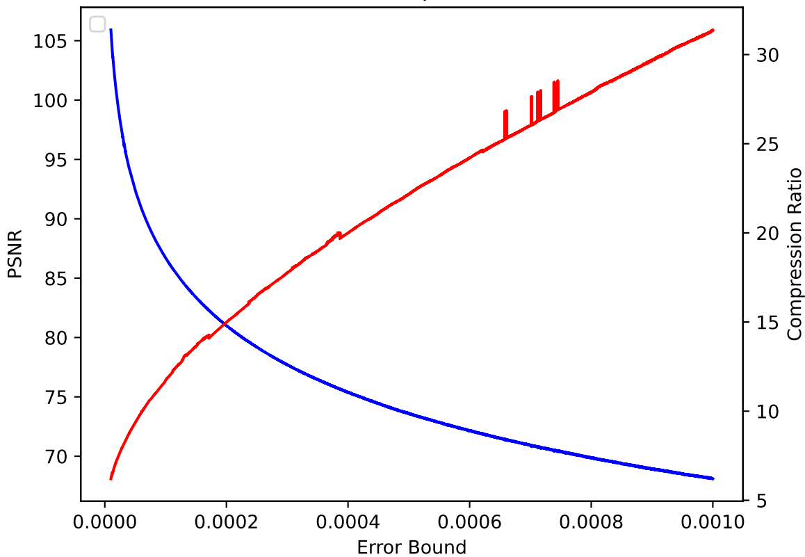
QVAPOR 34 pressio:rel
