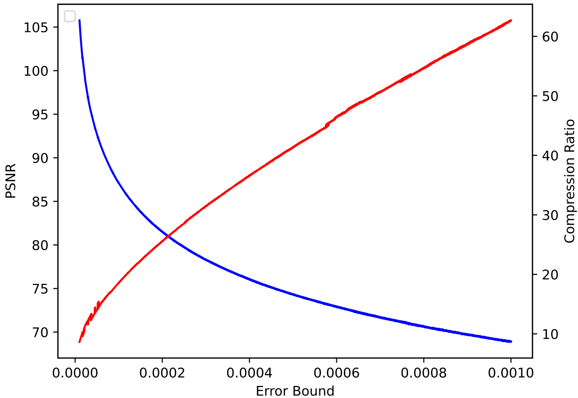
QVAPOR 07 pressio:rel
