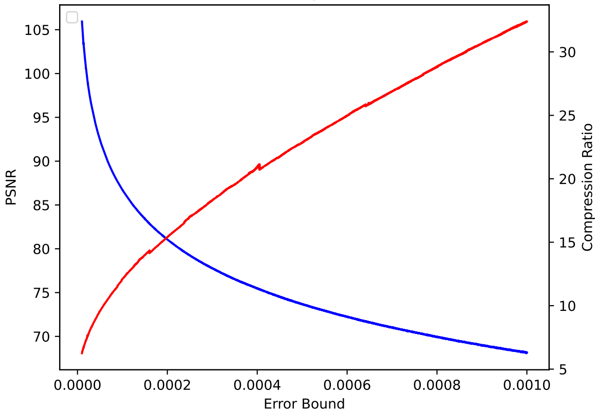
QVAPOR 26 pressio:rel
