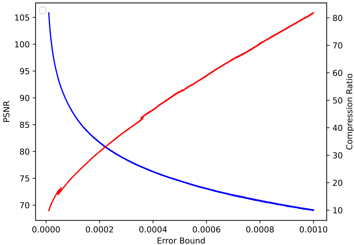
QVAPOR 05 pressio:rel
