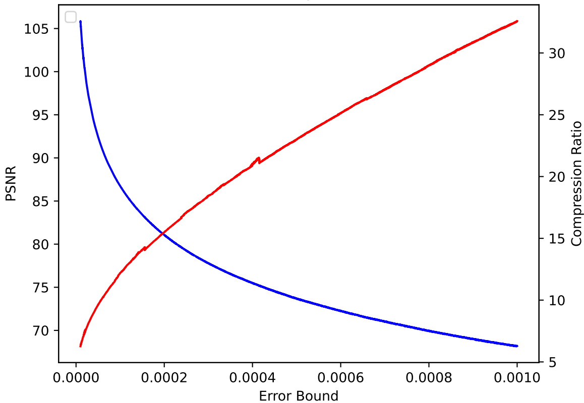
QVAPOR 25 pressio:rel
