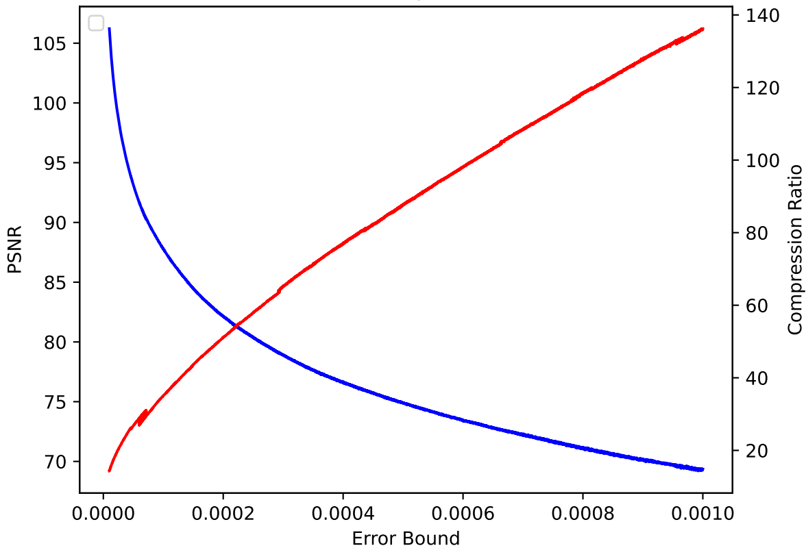
QVAPOR 01 pressio:rel
