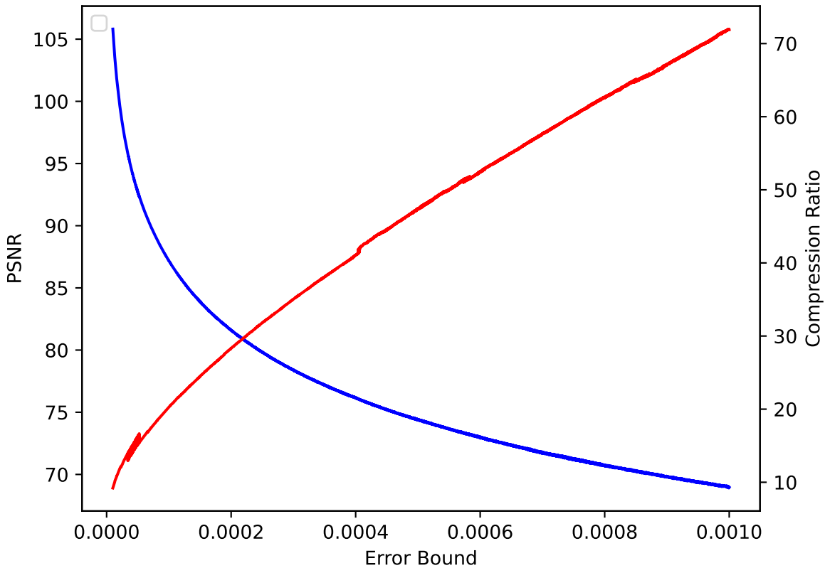
QVAPOR 06 pressio:rel
