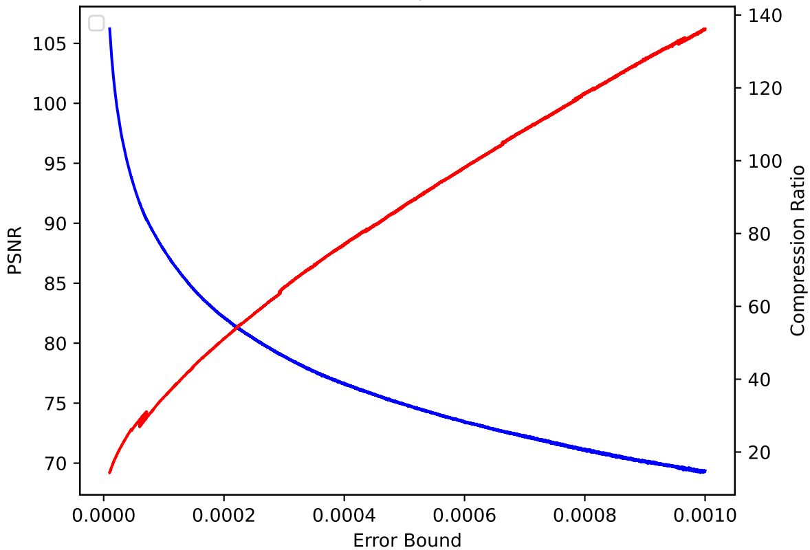
QVAPOR 01 pressio:rel
