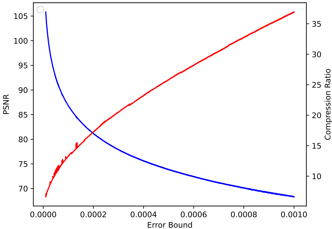
QVAPOR 15 pressio:rel
