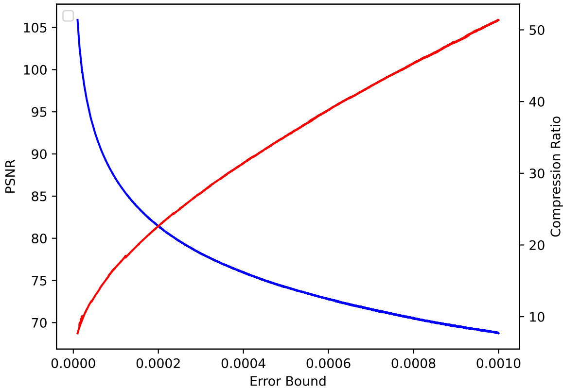
QVAPOR 08 pressio:rel
