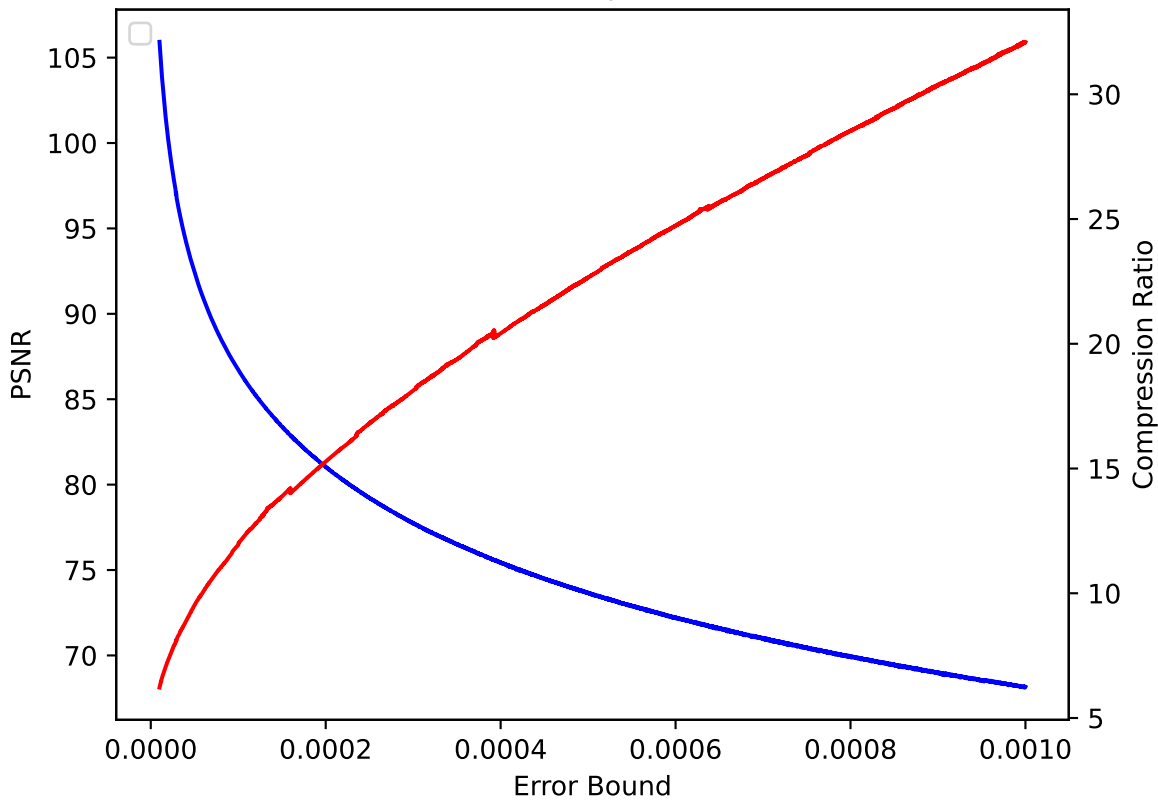
QVAPOR 28 pressio:rel
