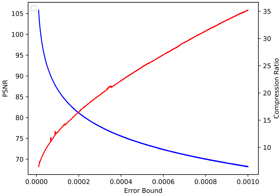
QVAPOR 20 pressio:rel
