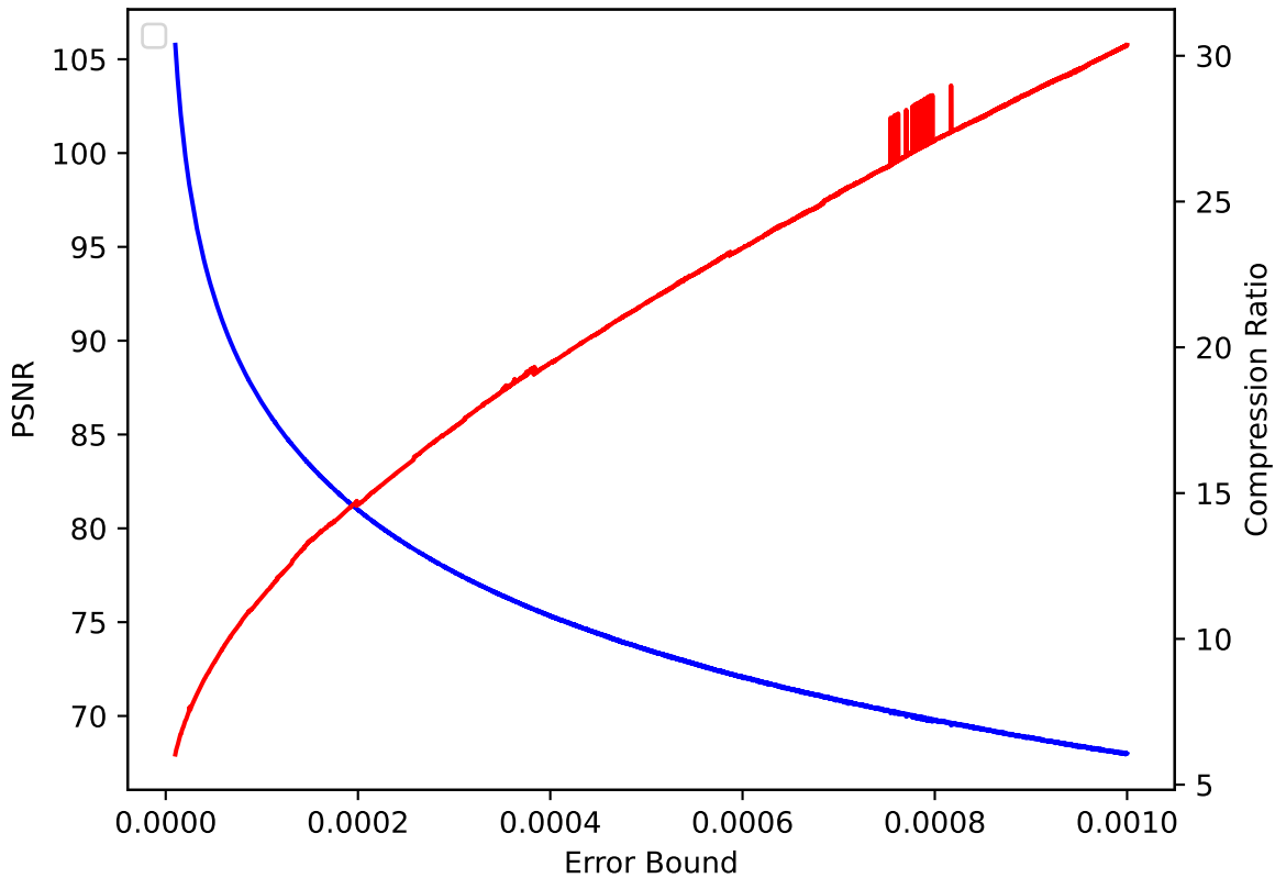
QVAPOR 47 pressio:rel
