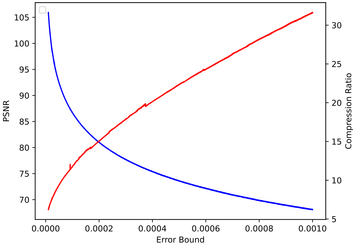
QVAPOR 36 pressio:rel
