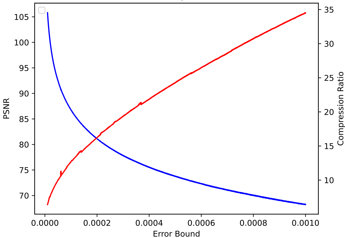
QVAPOR 21 pressio:rel
