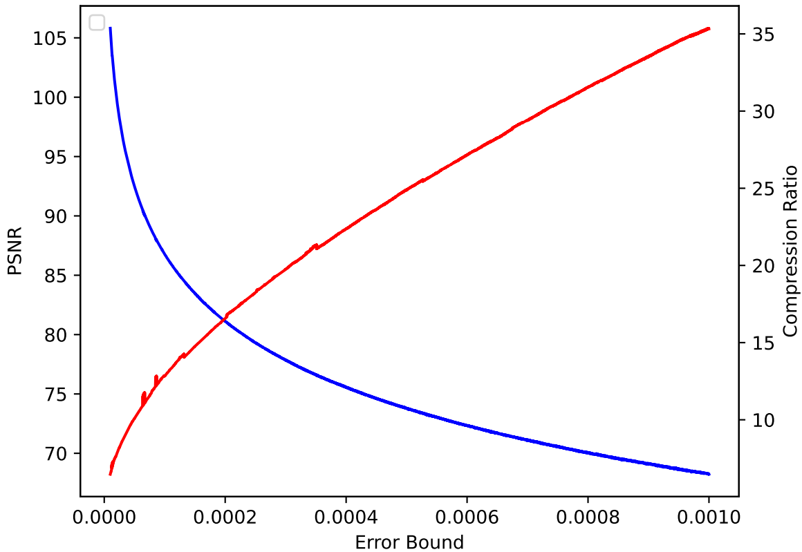
QVAPOR 19 pressio:rel
