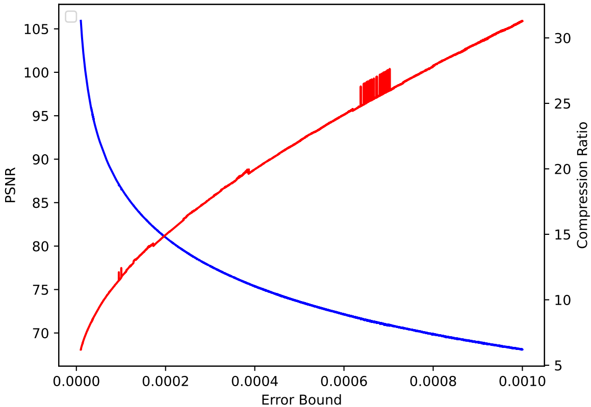
QVAPOR 35 pressio:rel
