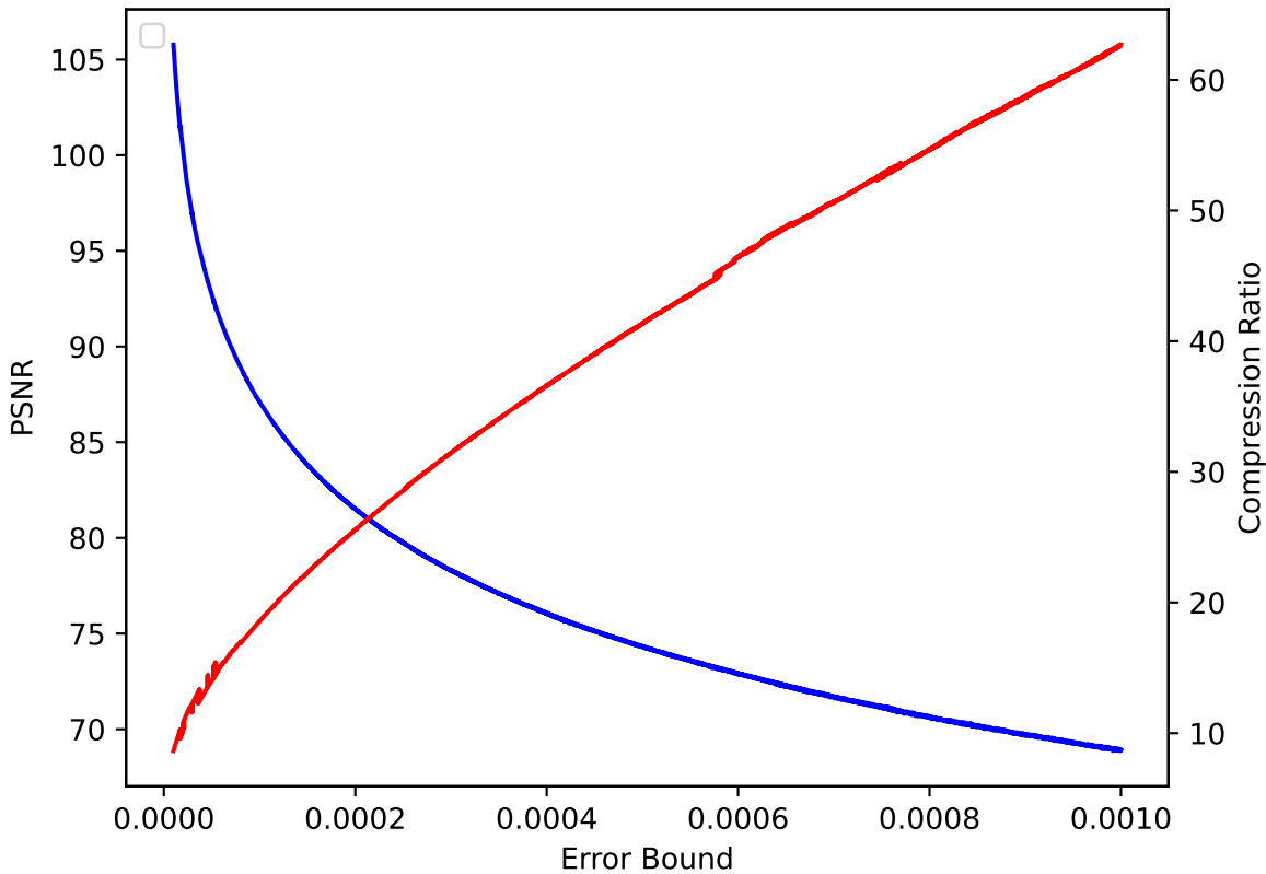
QVAPOR 07 pressio:rel
