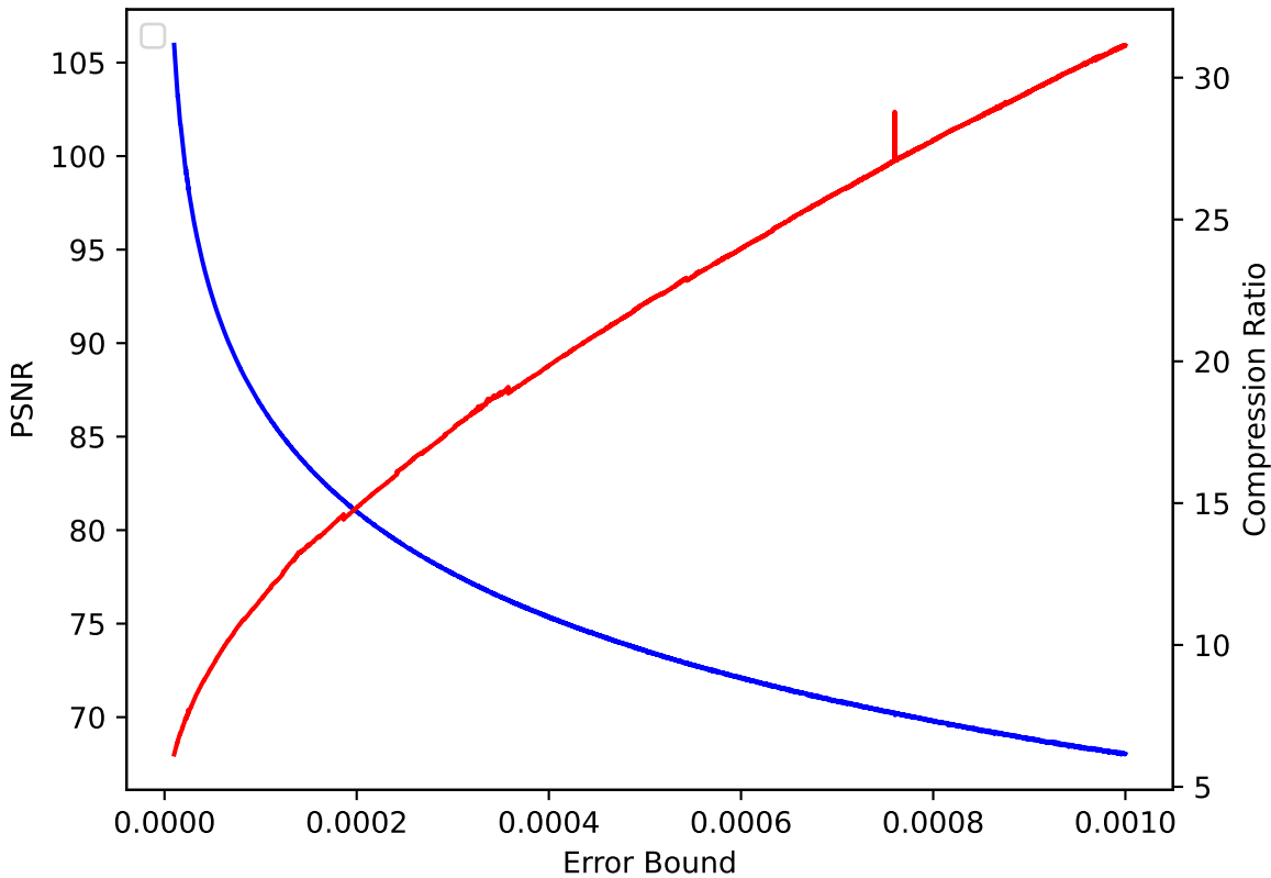
QVAPOR 43 pressio:rel
