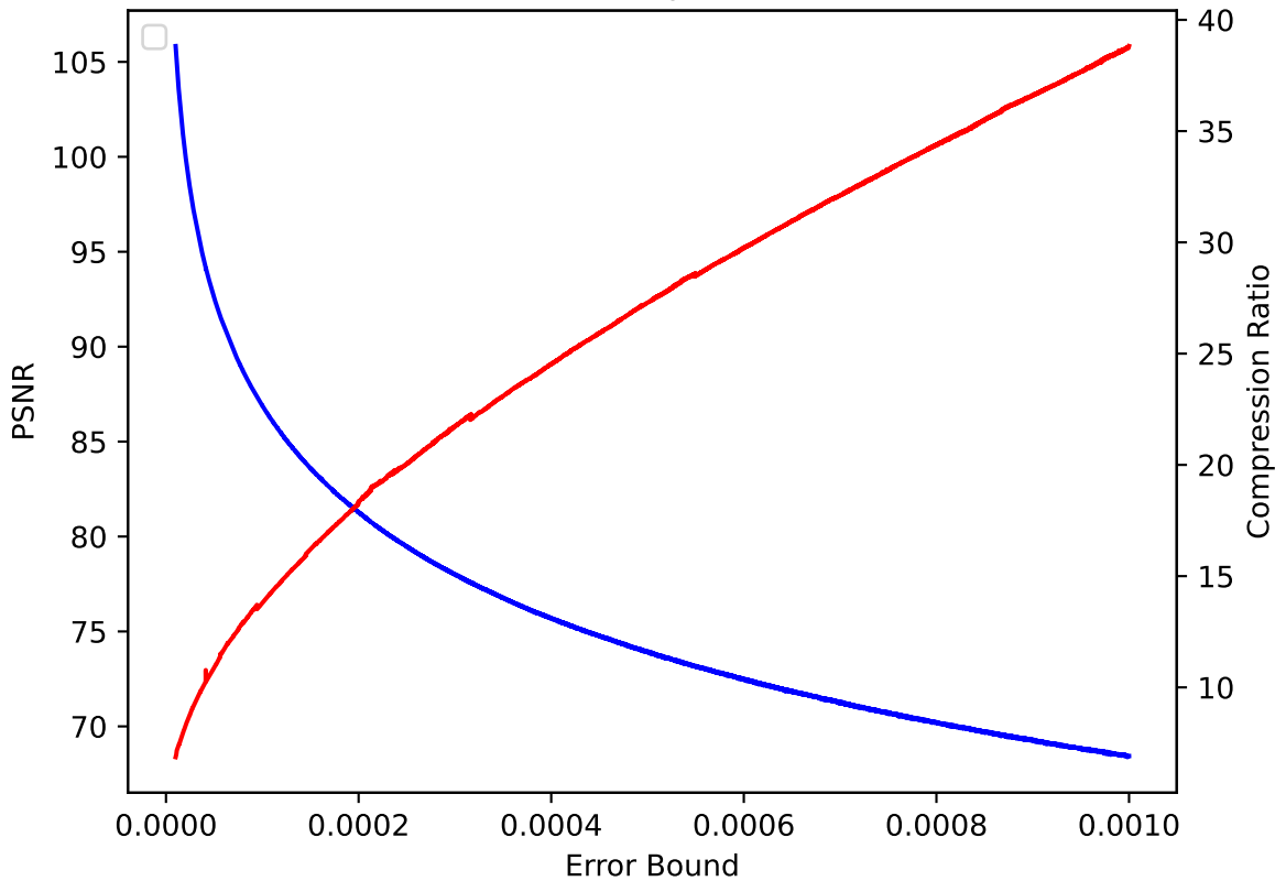
QVAPOR 11 pressio:rel
