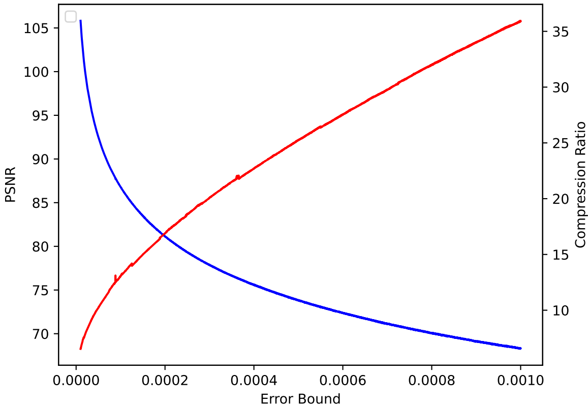
QVAPOR 17 pressio:rel
