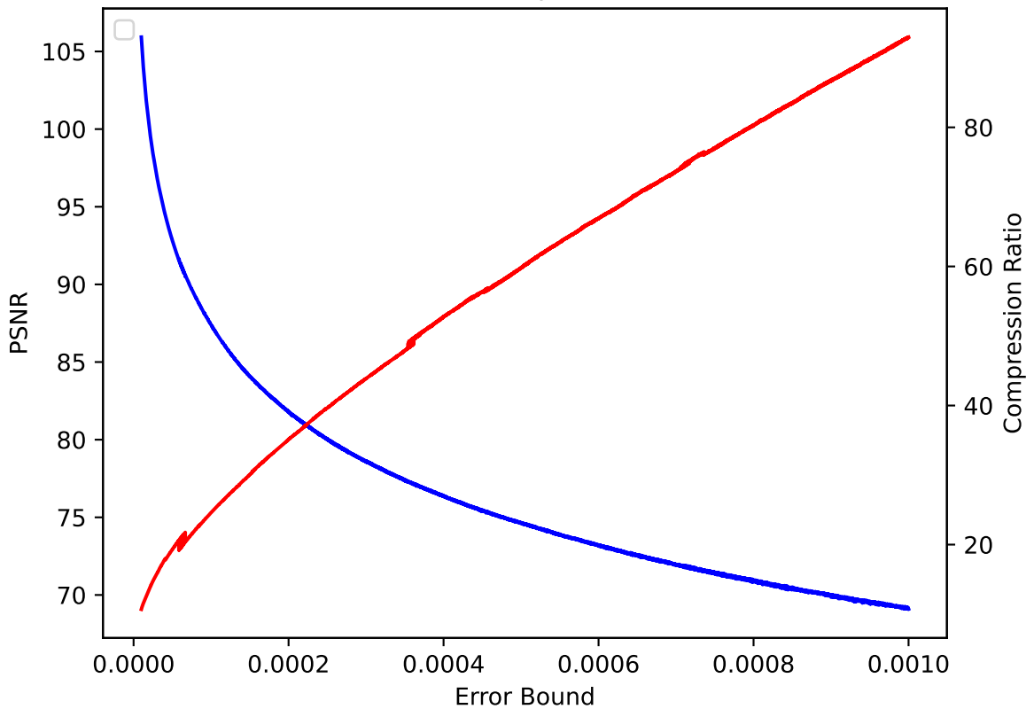
QVAPOR 04 pressio:rel
