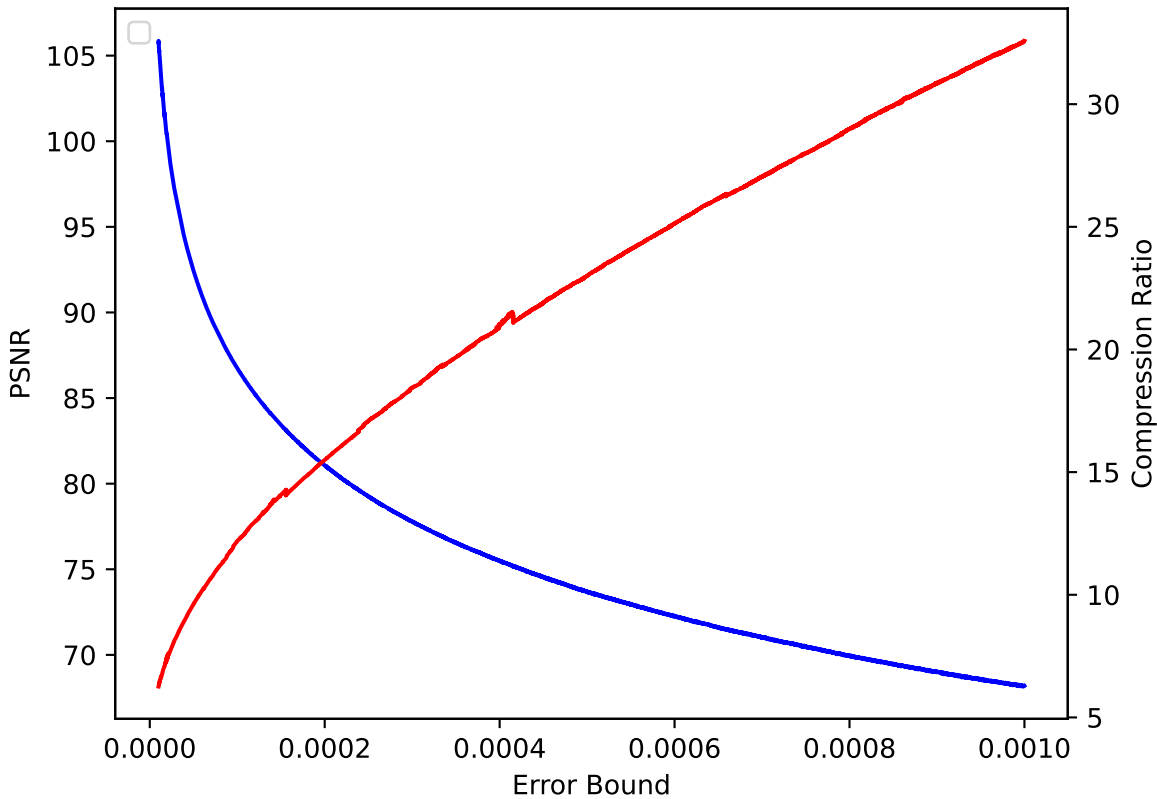
QVAPOR 25 pressio:rel
