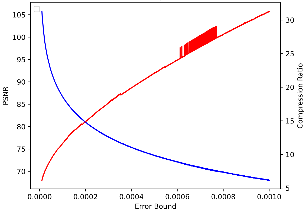
QVAPOR 41 pressio:rel
