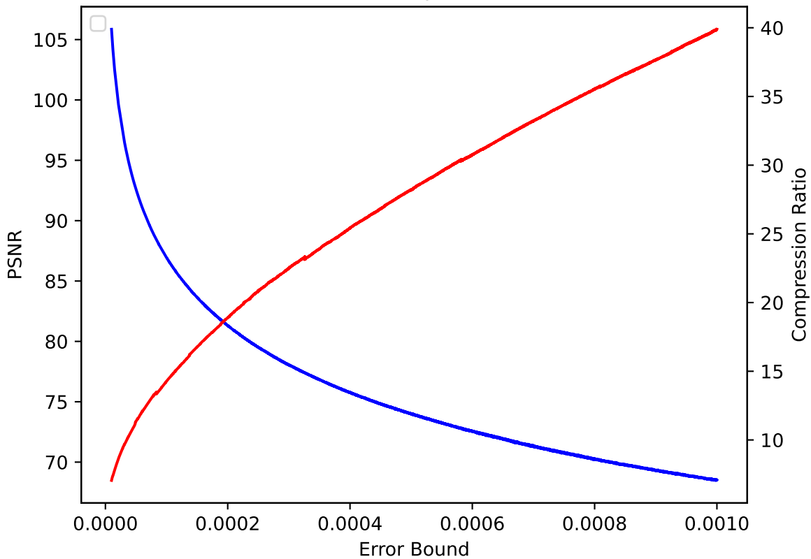
QVAPOR 10 pressio:rel
