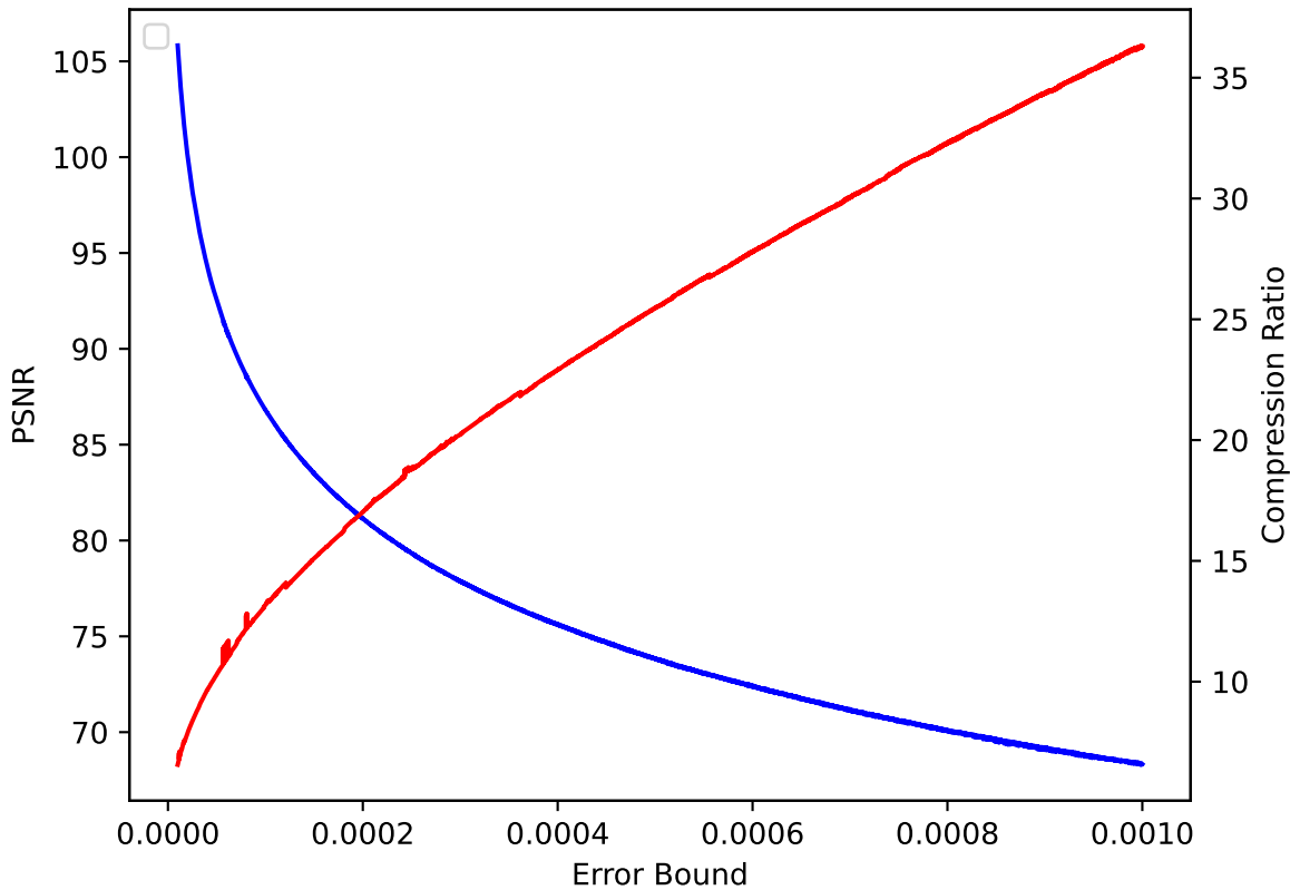
QVAPOR 16 pressio:rel
