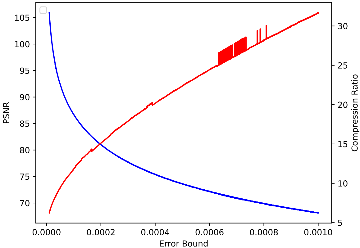
QVAPOR 33 pressio:rel
