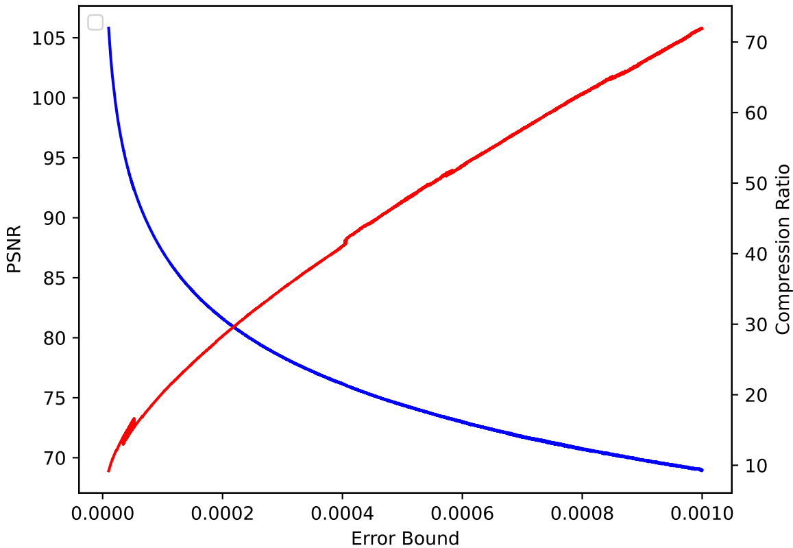
QVAPOR 06 pressio:rel
