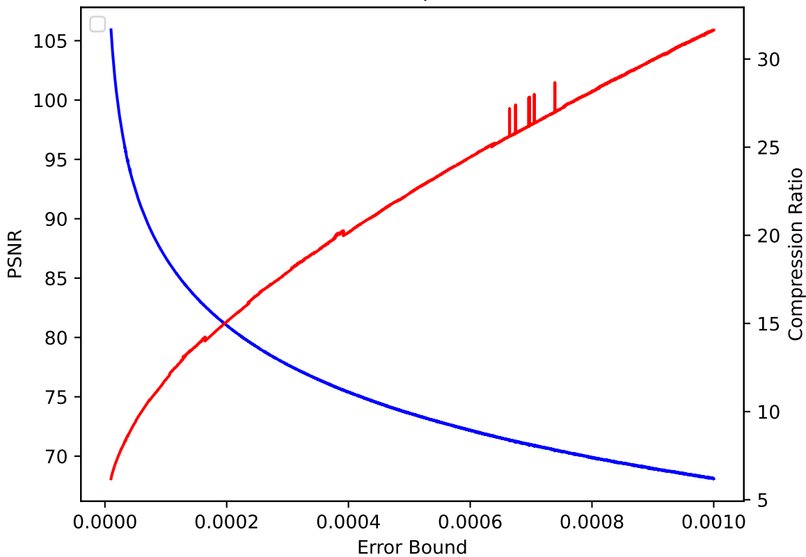
QVAPOR 32 pressio:rel
