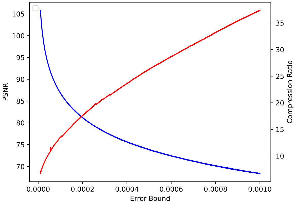
QVAPOR 13 pressio:rel
