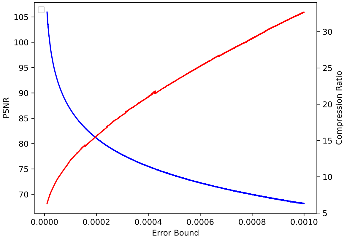
QVAPOR 24 pressio:rel
