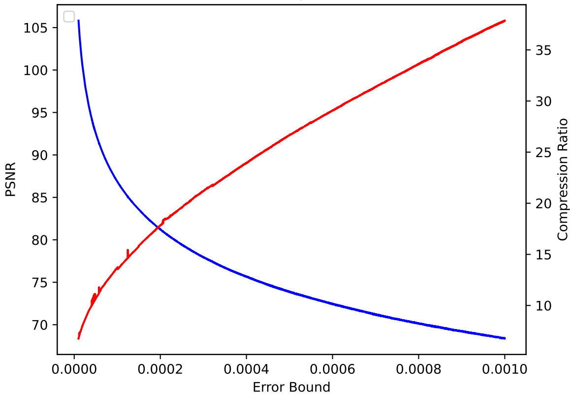
QVAPOR 12 pressio:rel
