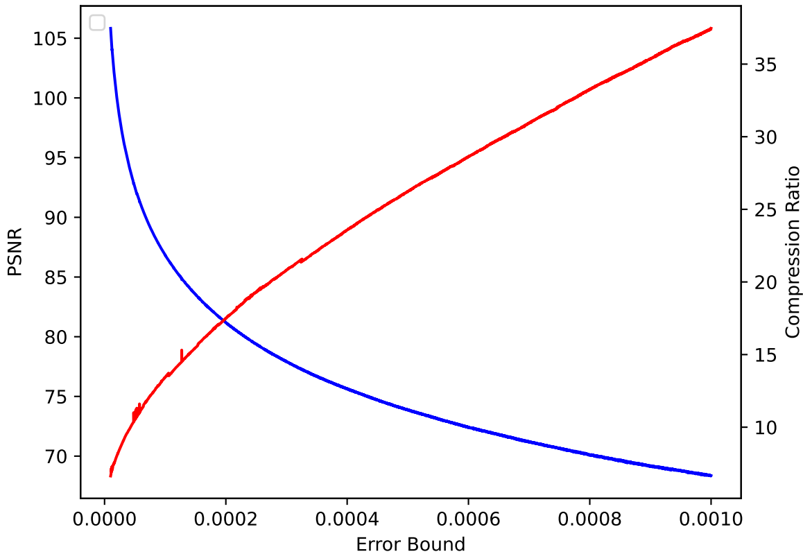
QVAPOR 14 pressio:rel
