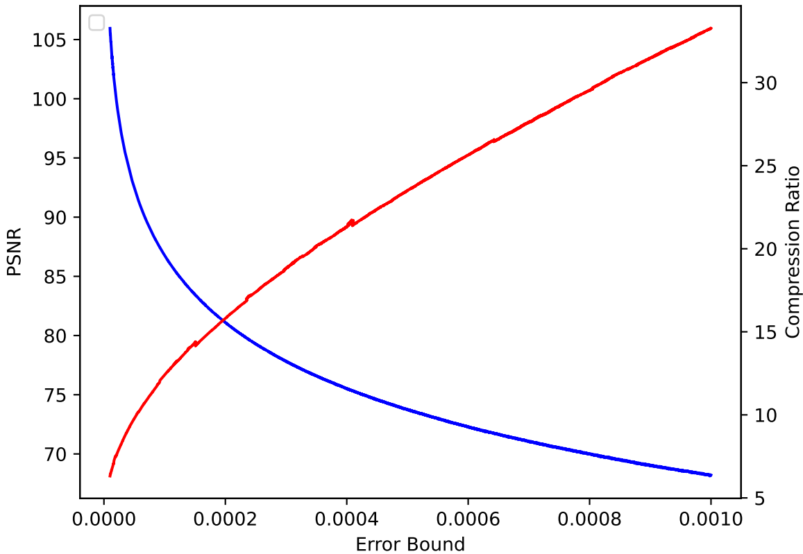
QVAPOR 23 pressio:rel
