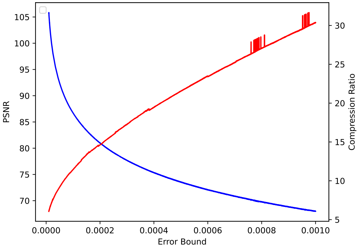
QVAPOR 48 pressio:rel
