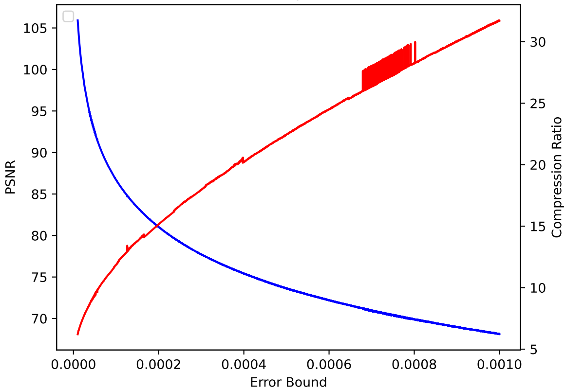
QVAPOR 30 pressio:rel
