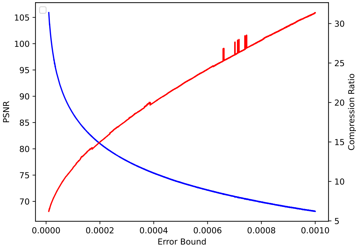
QVAPOR 34 pressio:rel
