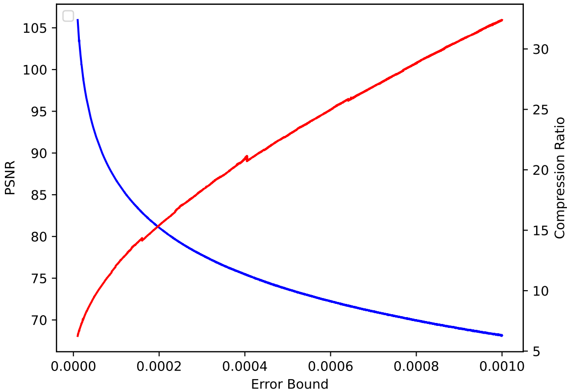
QVAPOR 26 pressio:rel
