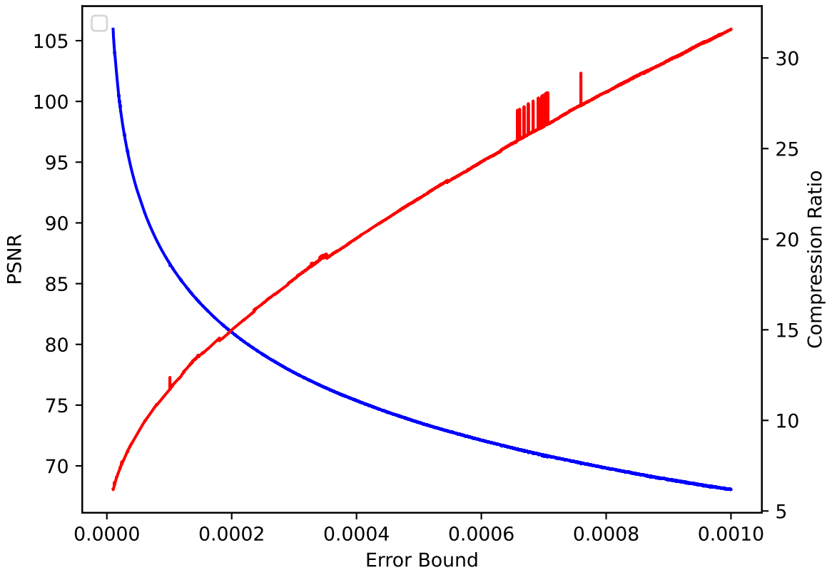
QVAPOR 40 pressio:rel
