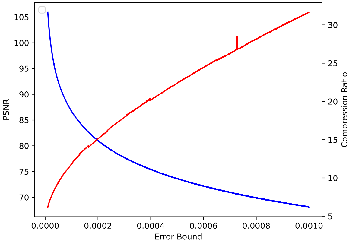
QVAPOR 31 pressio:rel
