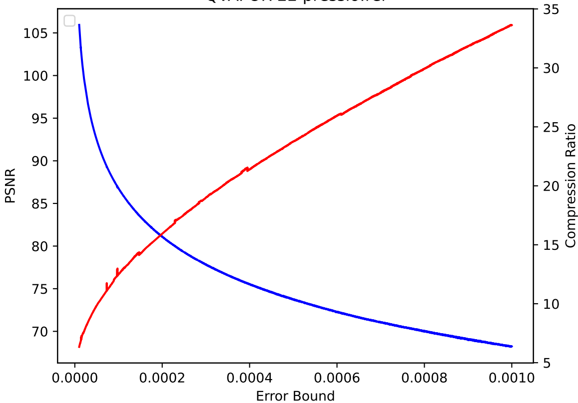
QVAPOR 22 pressio:rel
