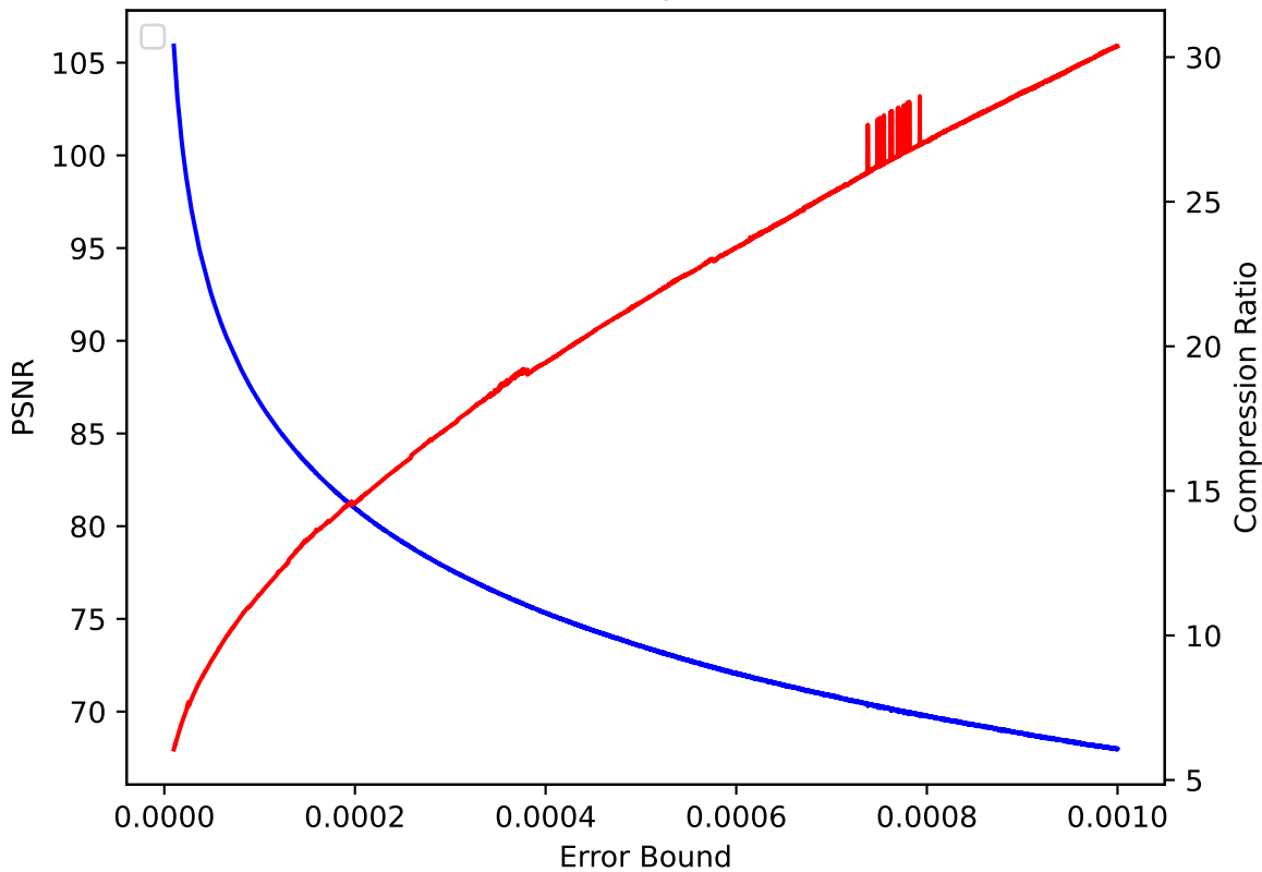
QVAPOR 46 pressio:rel
