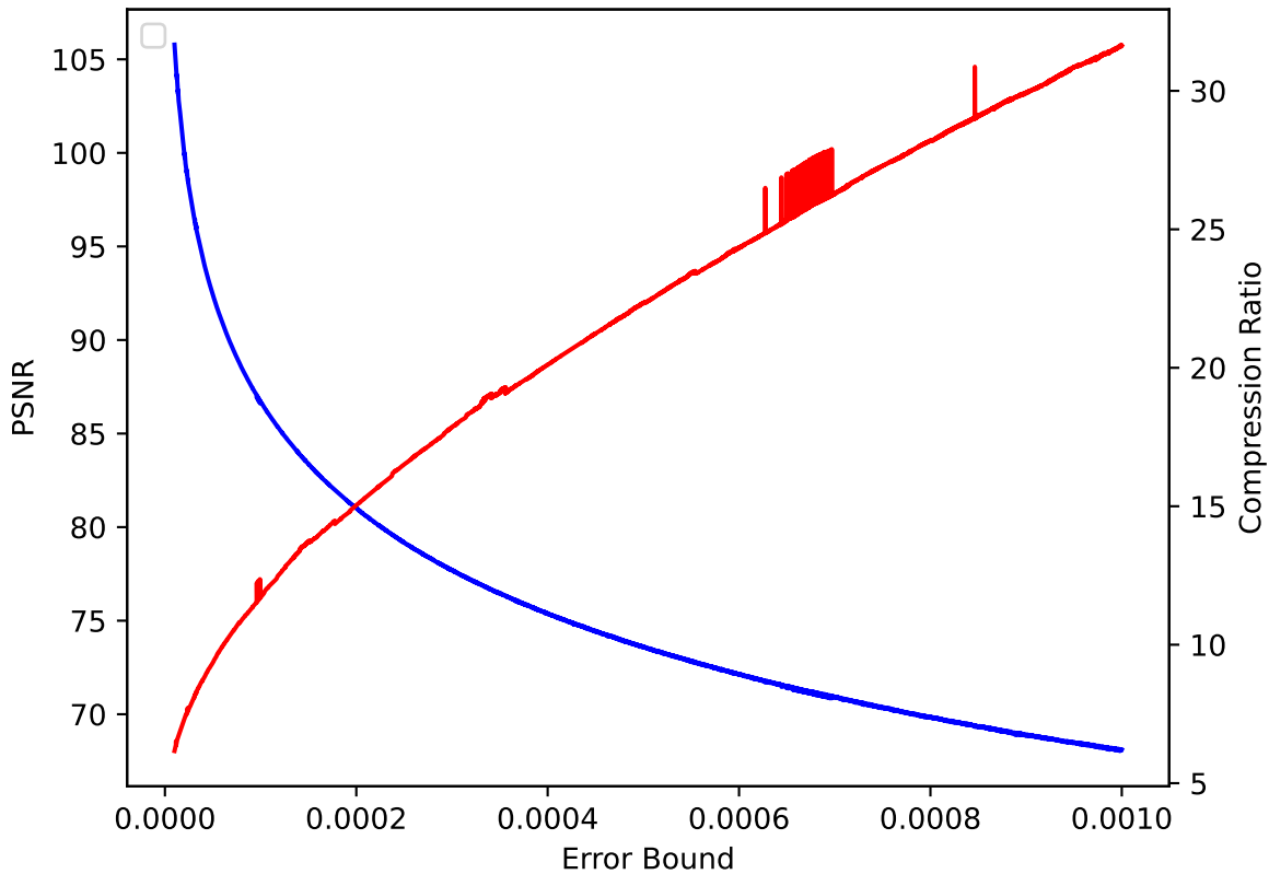
QVAPOR 39 pressio:rel
