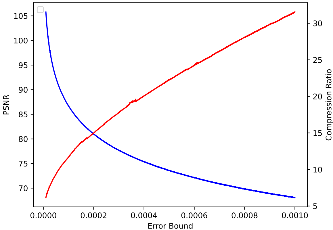
QVAPOR 38 pressio:rel
