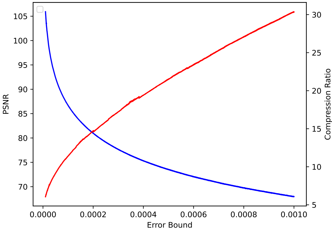
QVAPOR 45 pressio:rel
