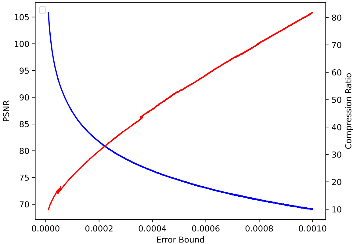
QVAPOR 05 pressio:rel
