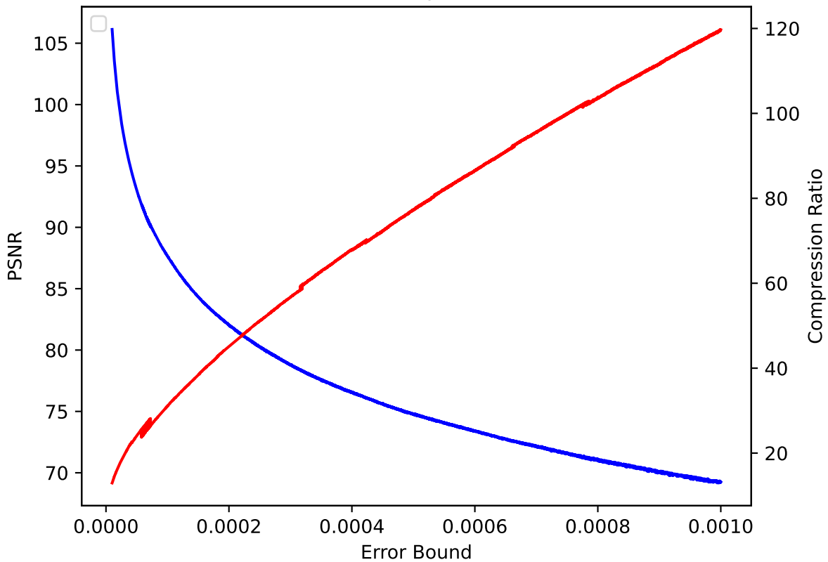
QVAPOR 02 pressio:rel
