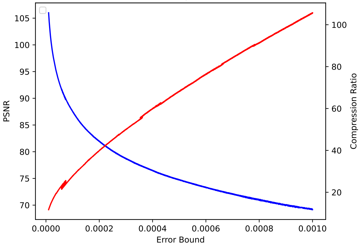
QVAPOR 03 pressio:rel
