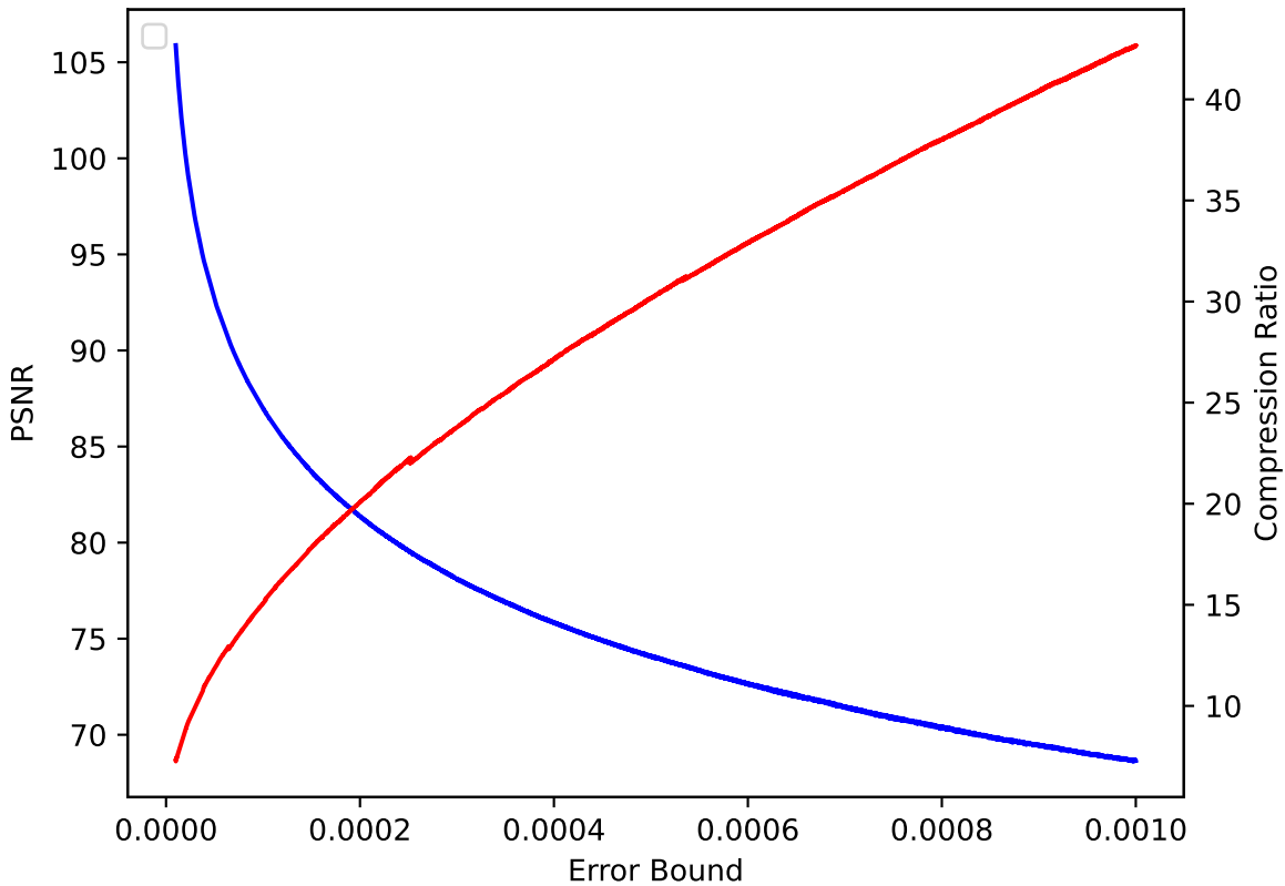
QVAPOR 09 pressio:rel
