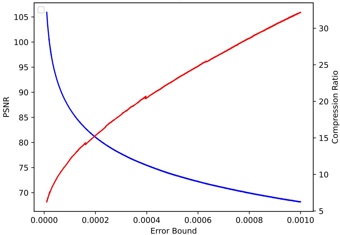
QVAPOR 27 pressio:rel
