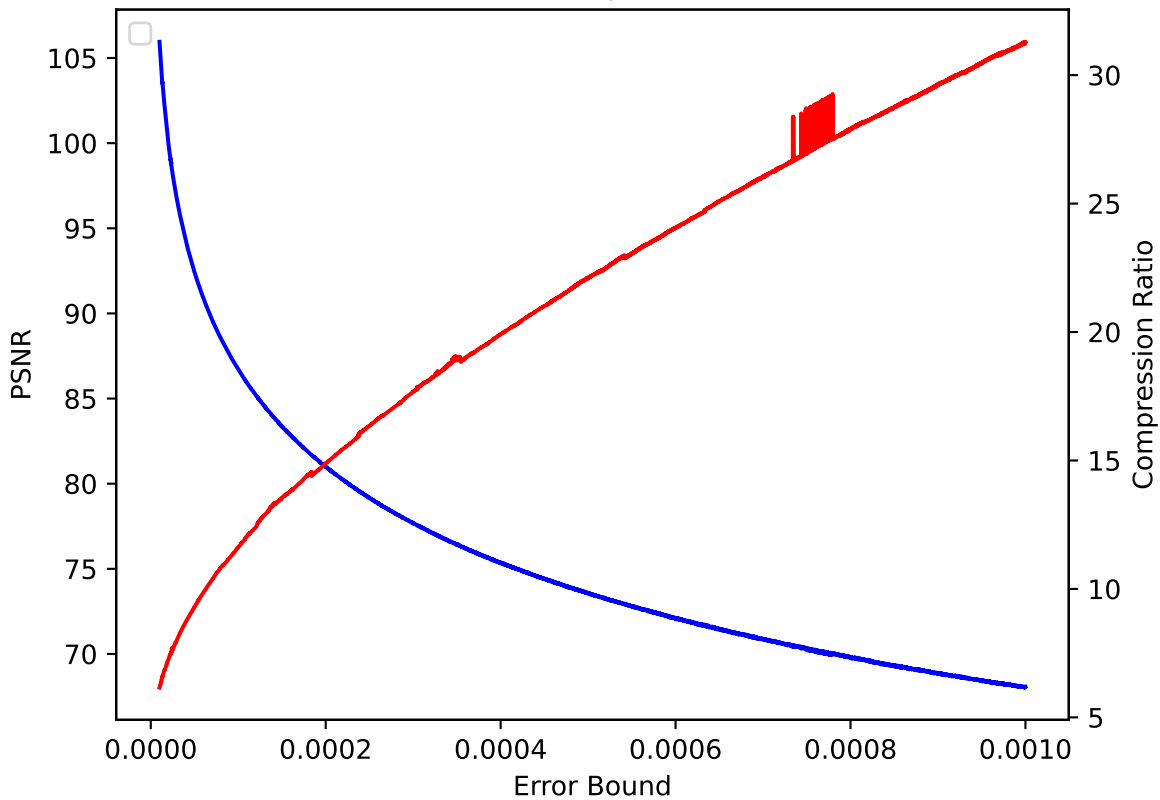
QVAPOR 42 pressio:rel
