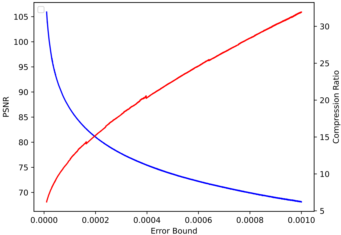
QVAPOR 29 pressio:rel
