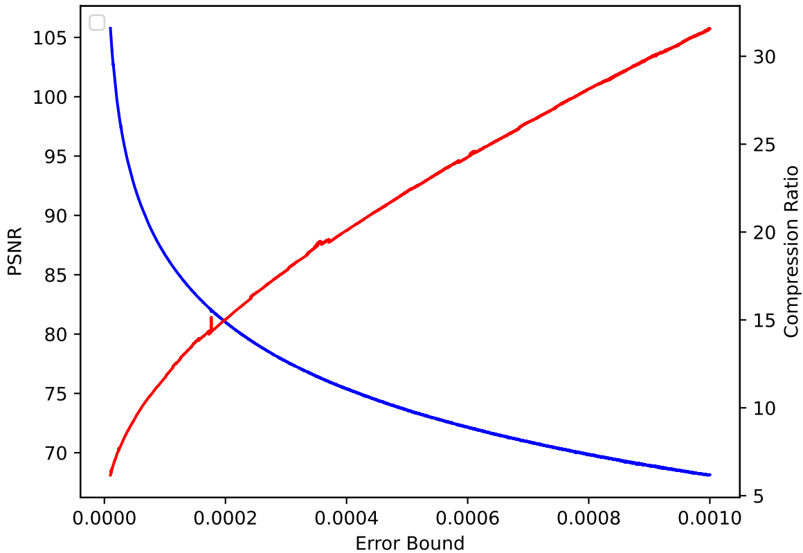
QVAPOR 37 pressio:rel
