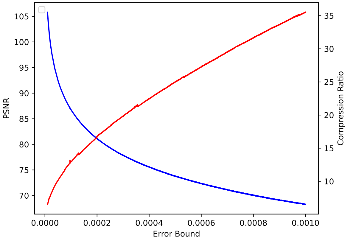
QVAPOR 18 pressio:rel
