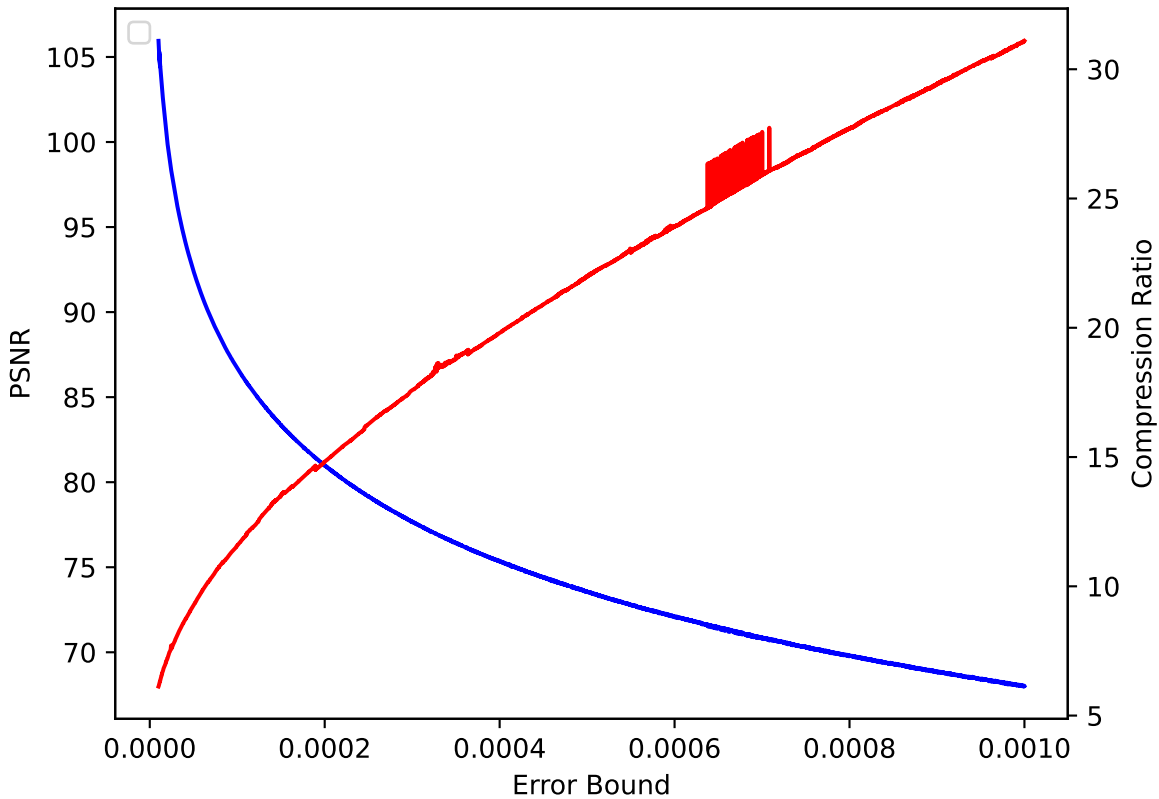
QVAPOR 44 pressio:rel
