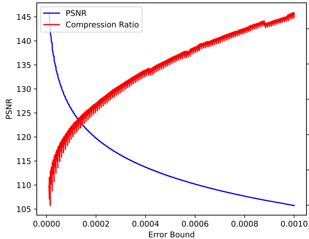
pressio:abs
