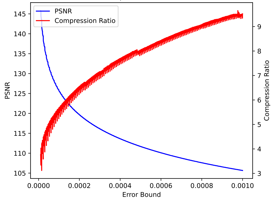
pressio:abs
