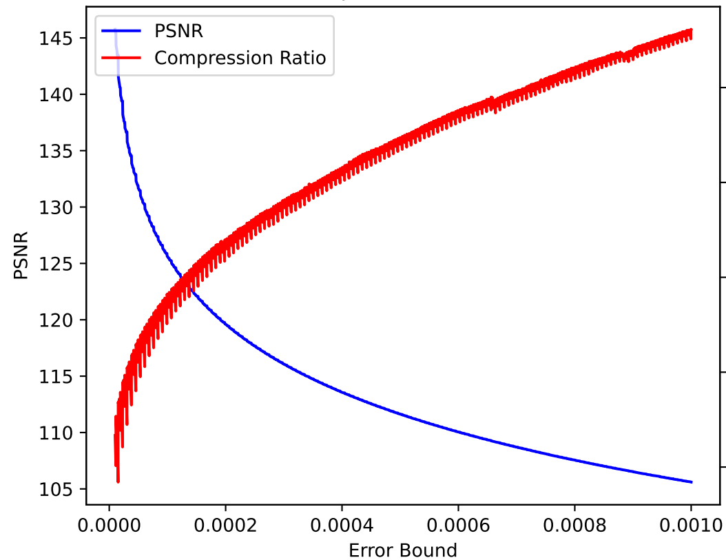
pressio:abs
