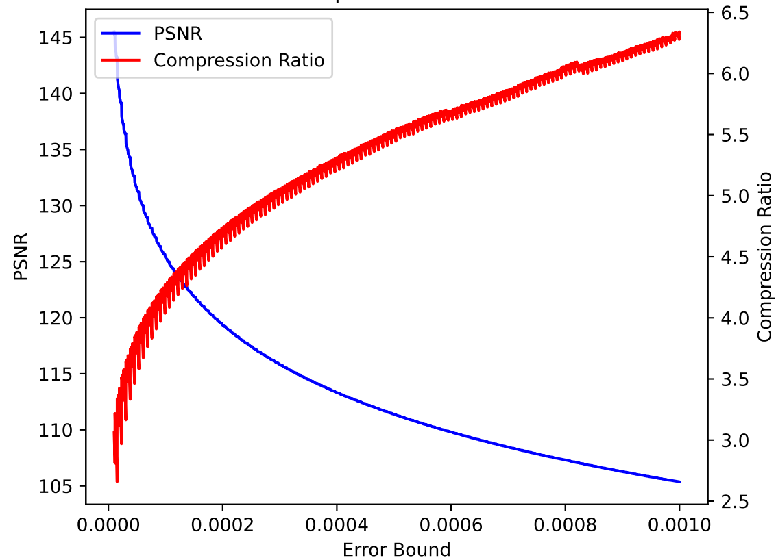
pressio:abs
