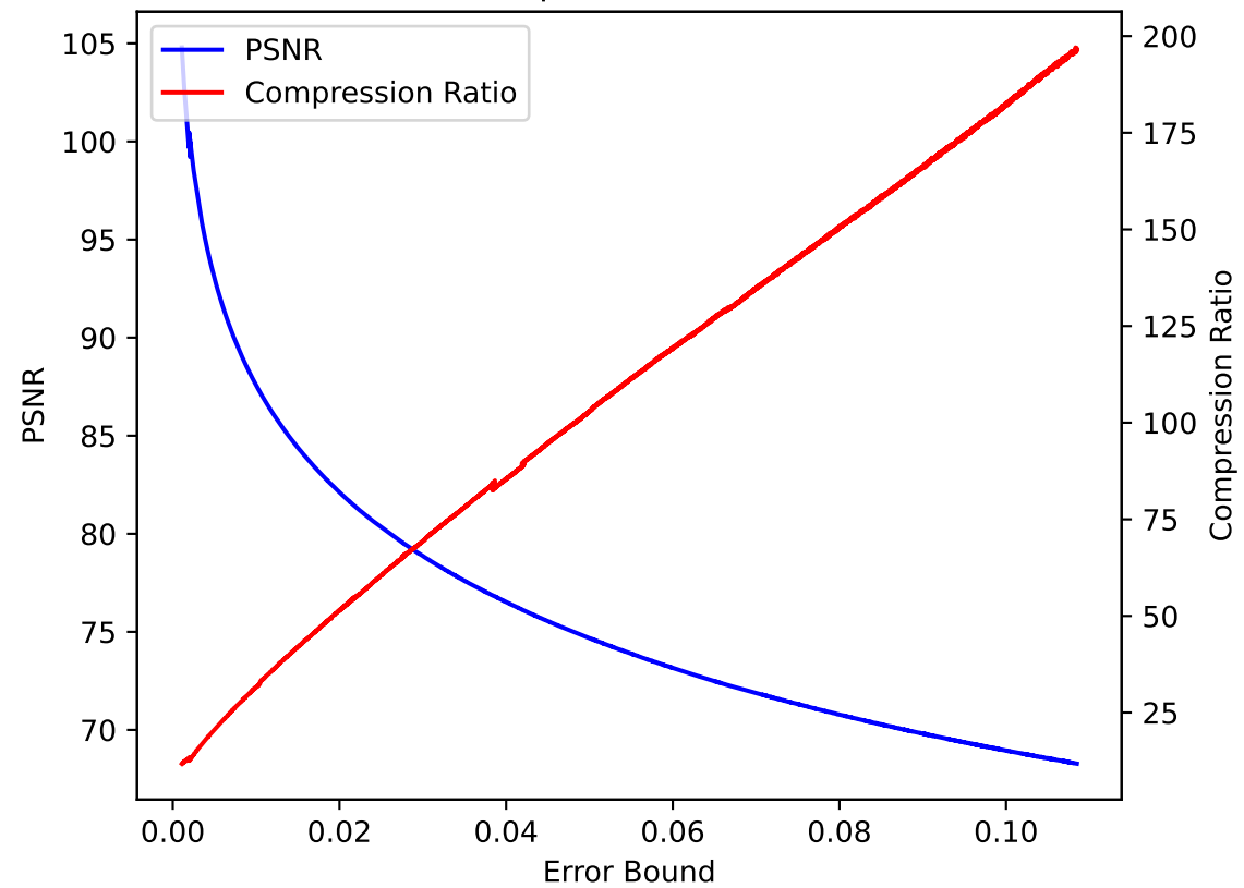
pressio:rel
