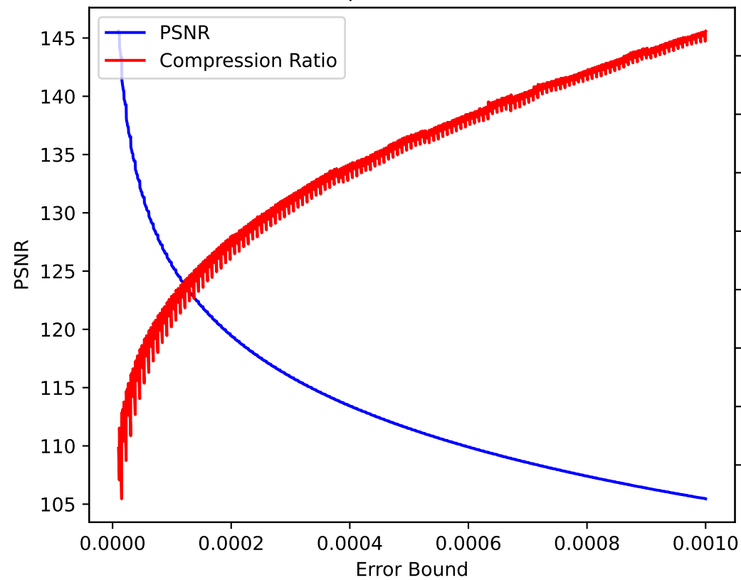
pressio:abs
