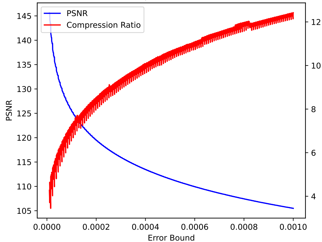
pressio:abs
