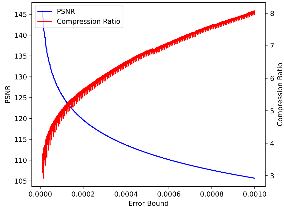
pressio:abs
