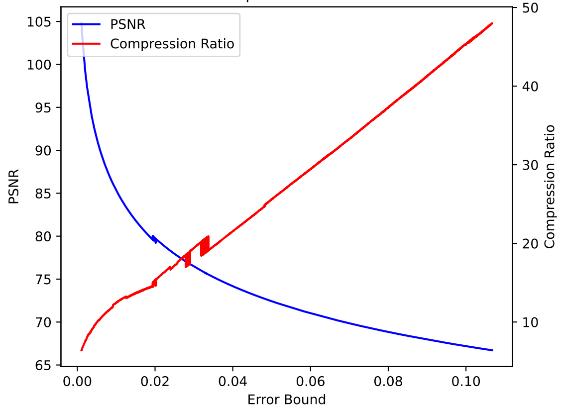
pressio:rel
