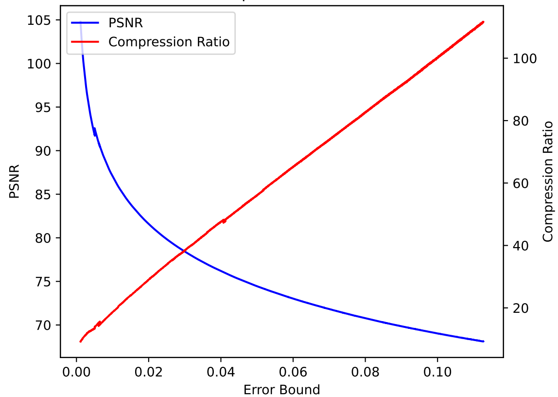
pressio:rel
