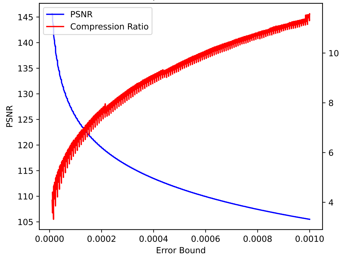
pressio:abs
