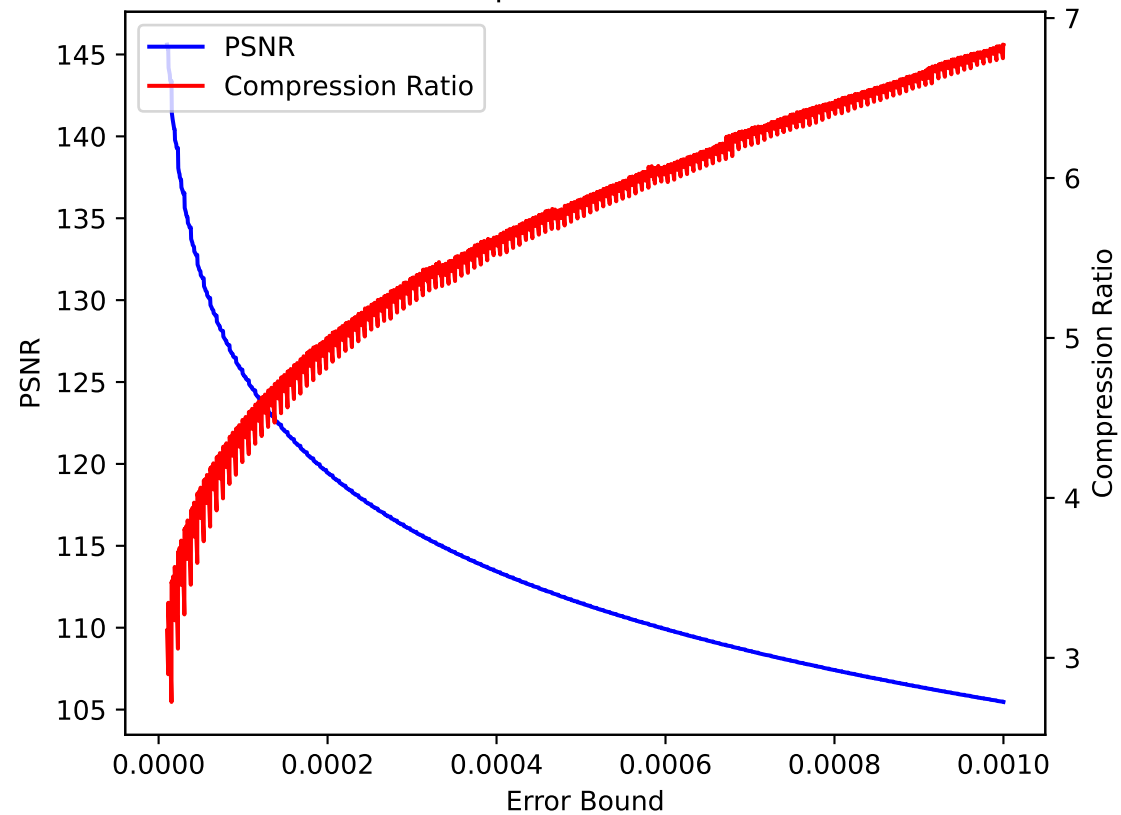
pressio:abs
