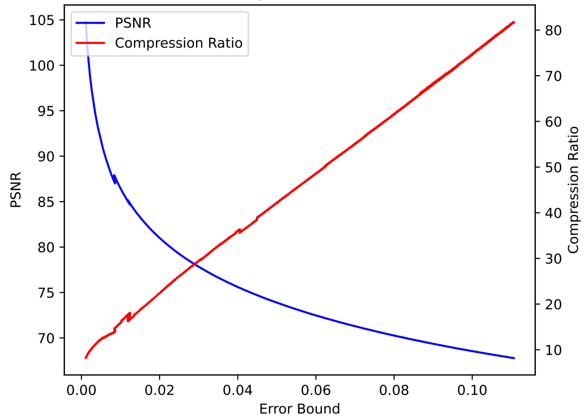
pressio:rel
