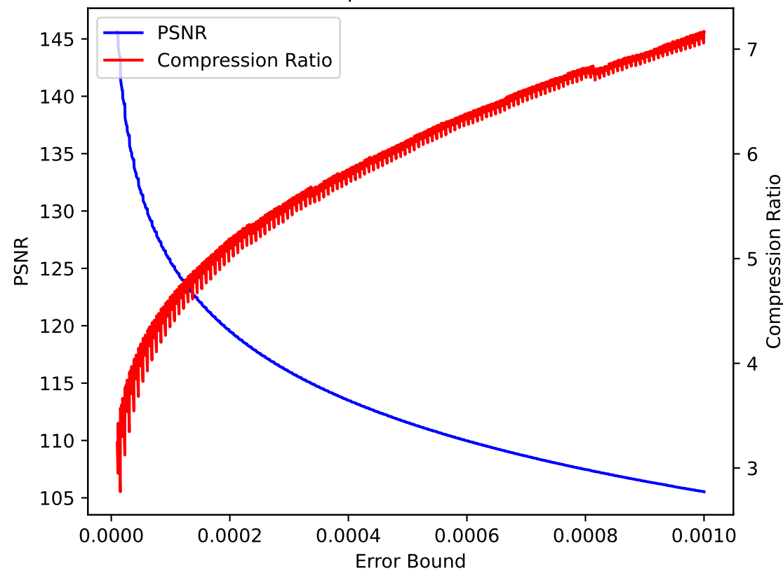
pressio:abs
