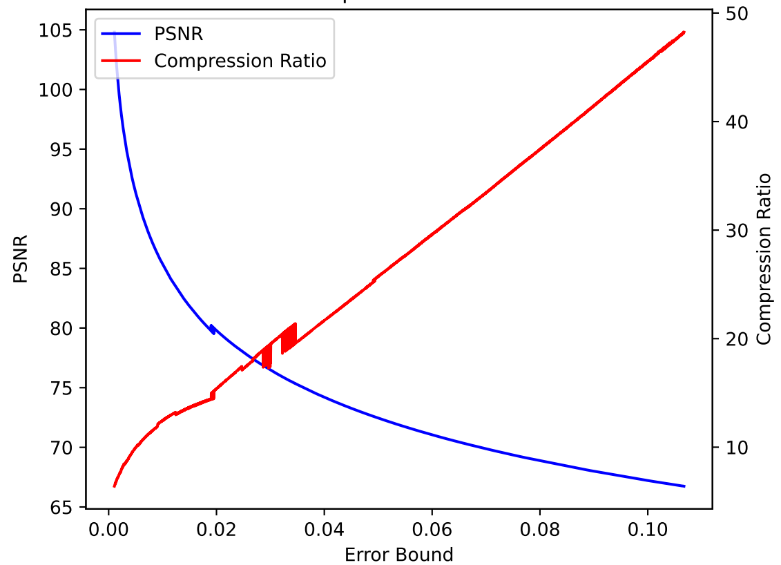
pressio:rel
