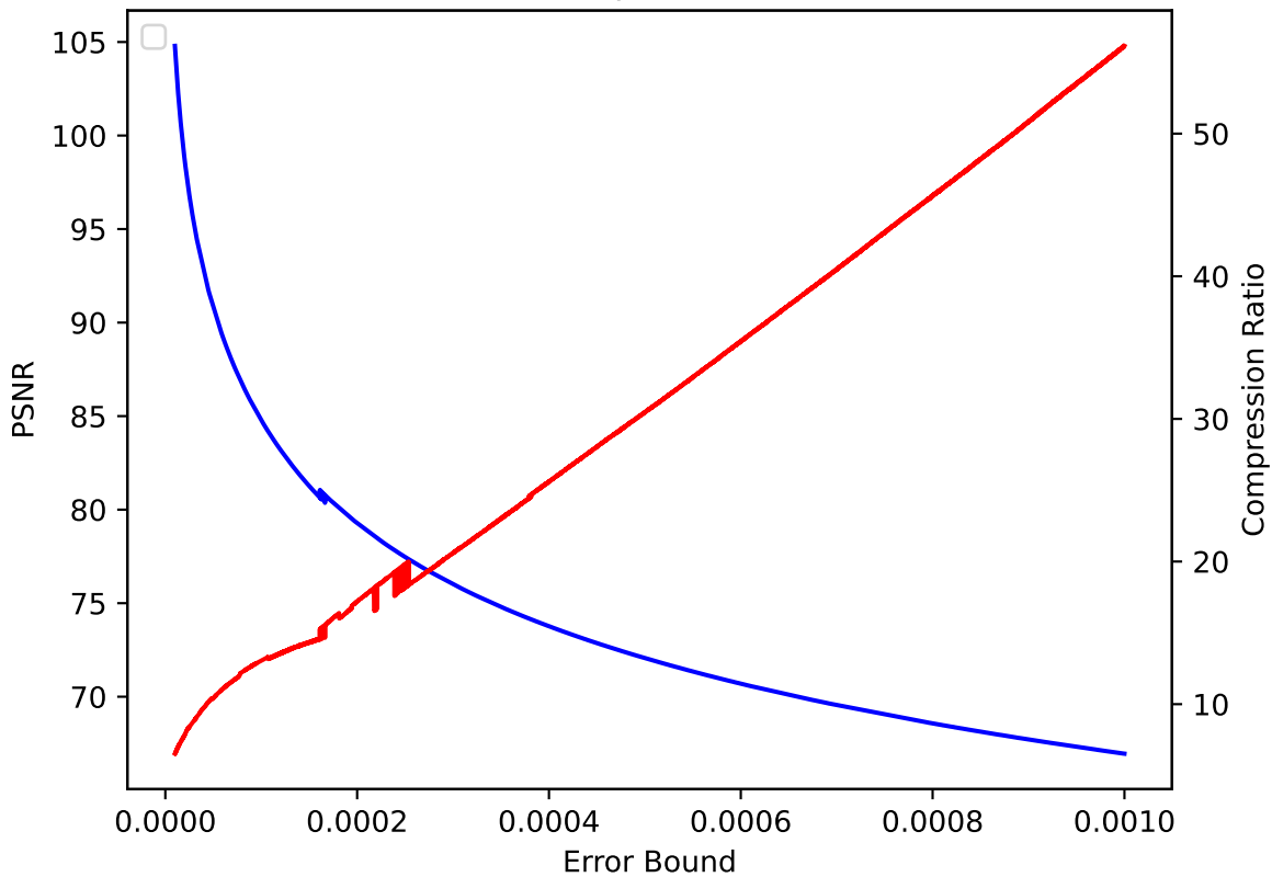
TC 46 pressio:rel
