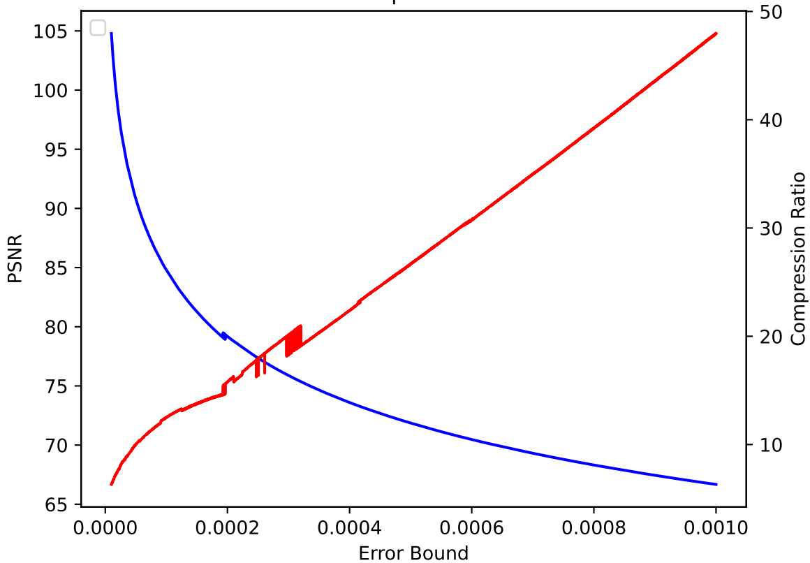
TC 36 pressio:rel
