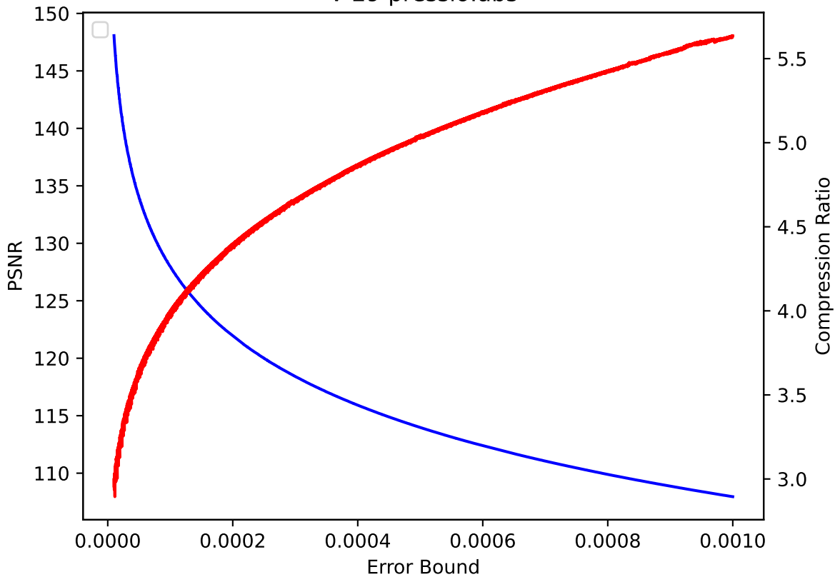
V 29 pressio:abs
