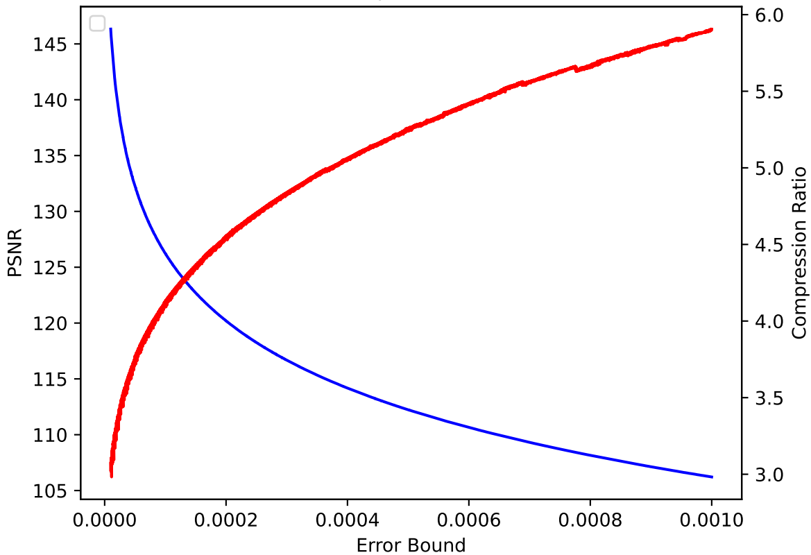
V 14 pressio:abs
