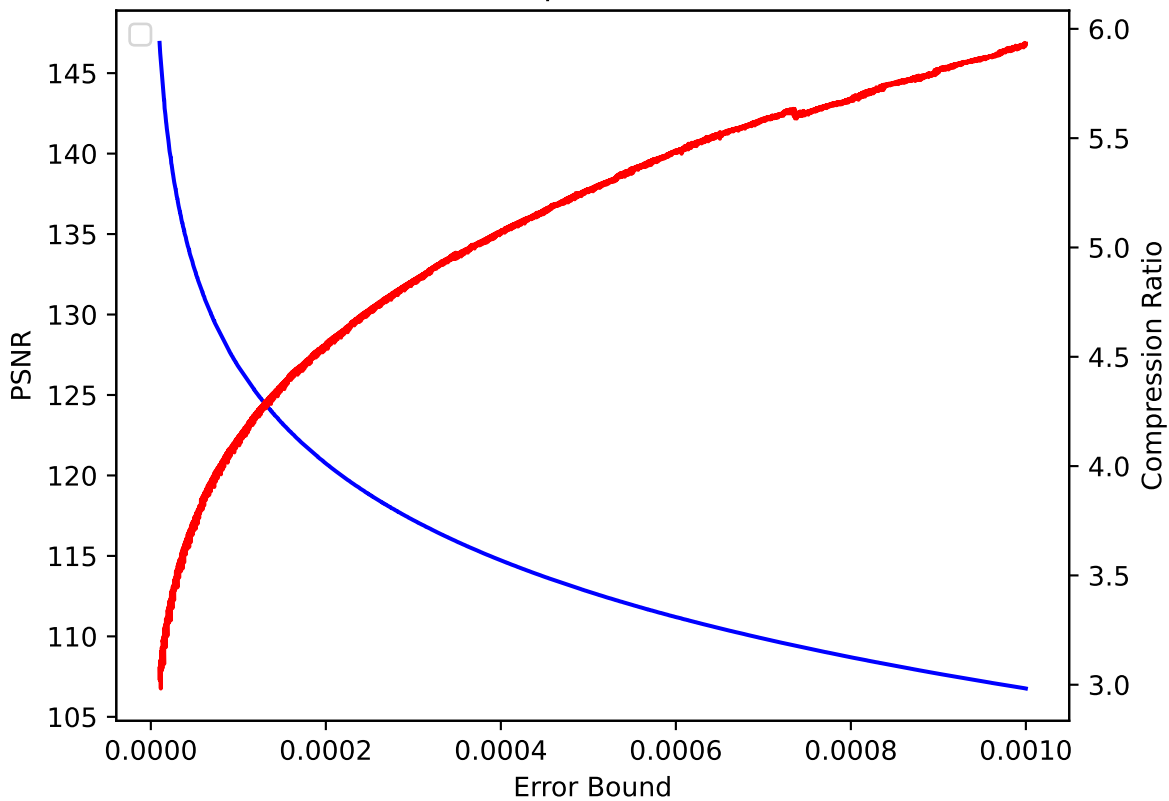
V 13 pressio:abs
