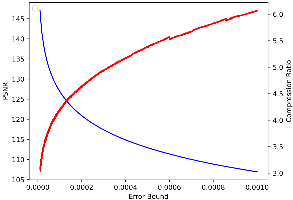
V 11 pressio:abs
