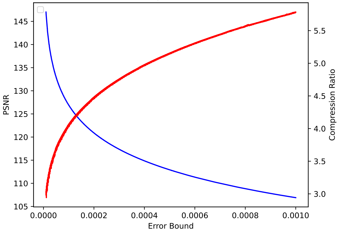
V 21 pressio:abs
