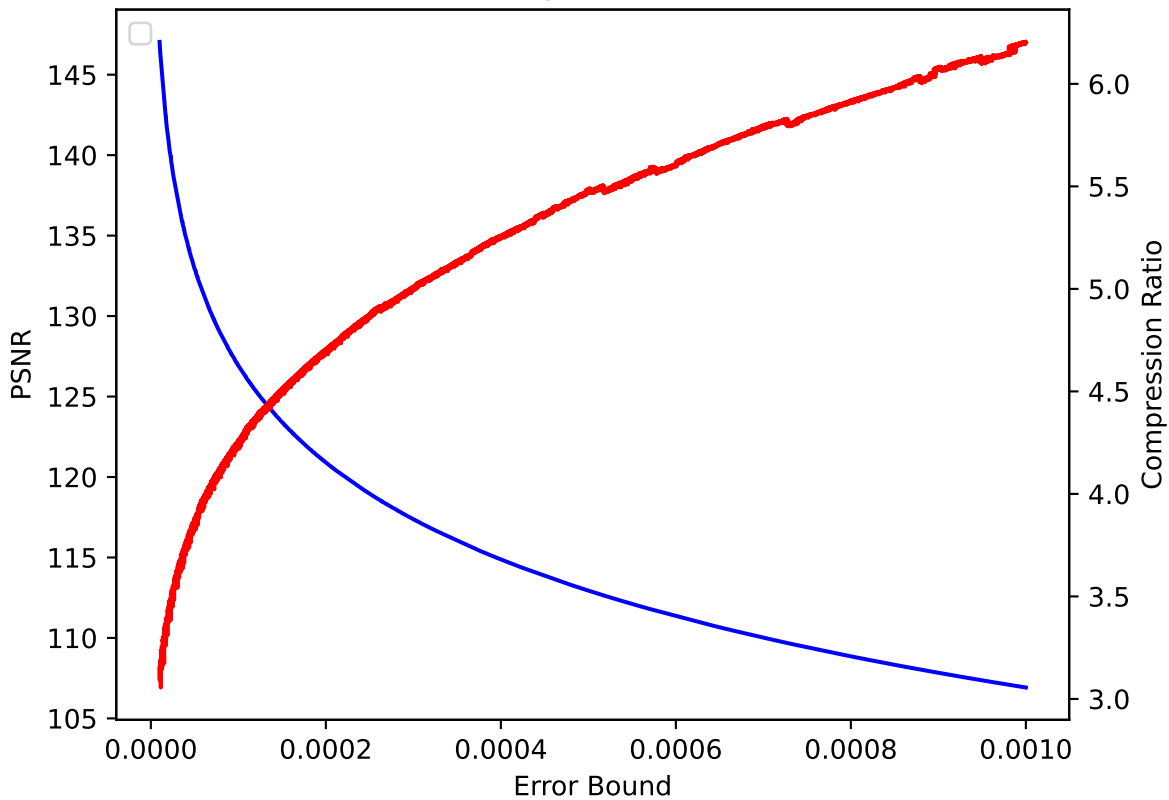
V 10 pressio:abs
