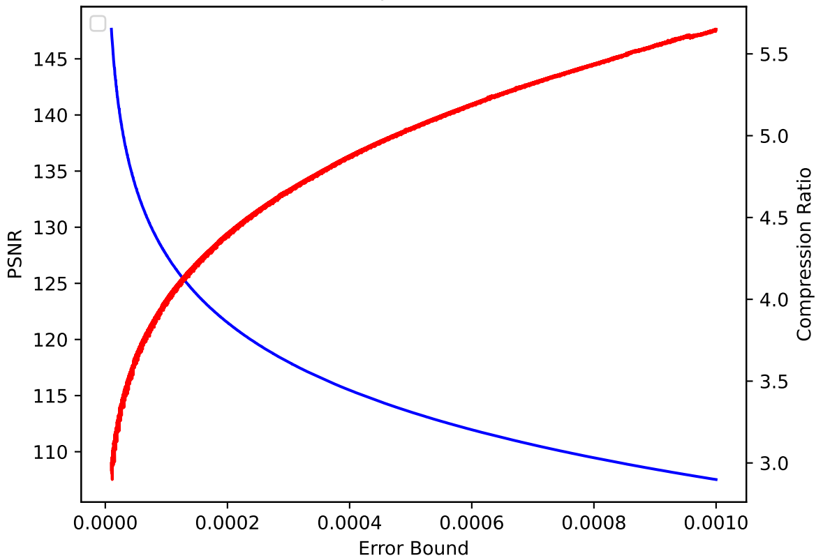
V 28 pressio:abs
