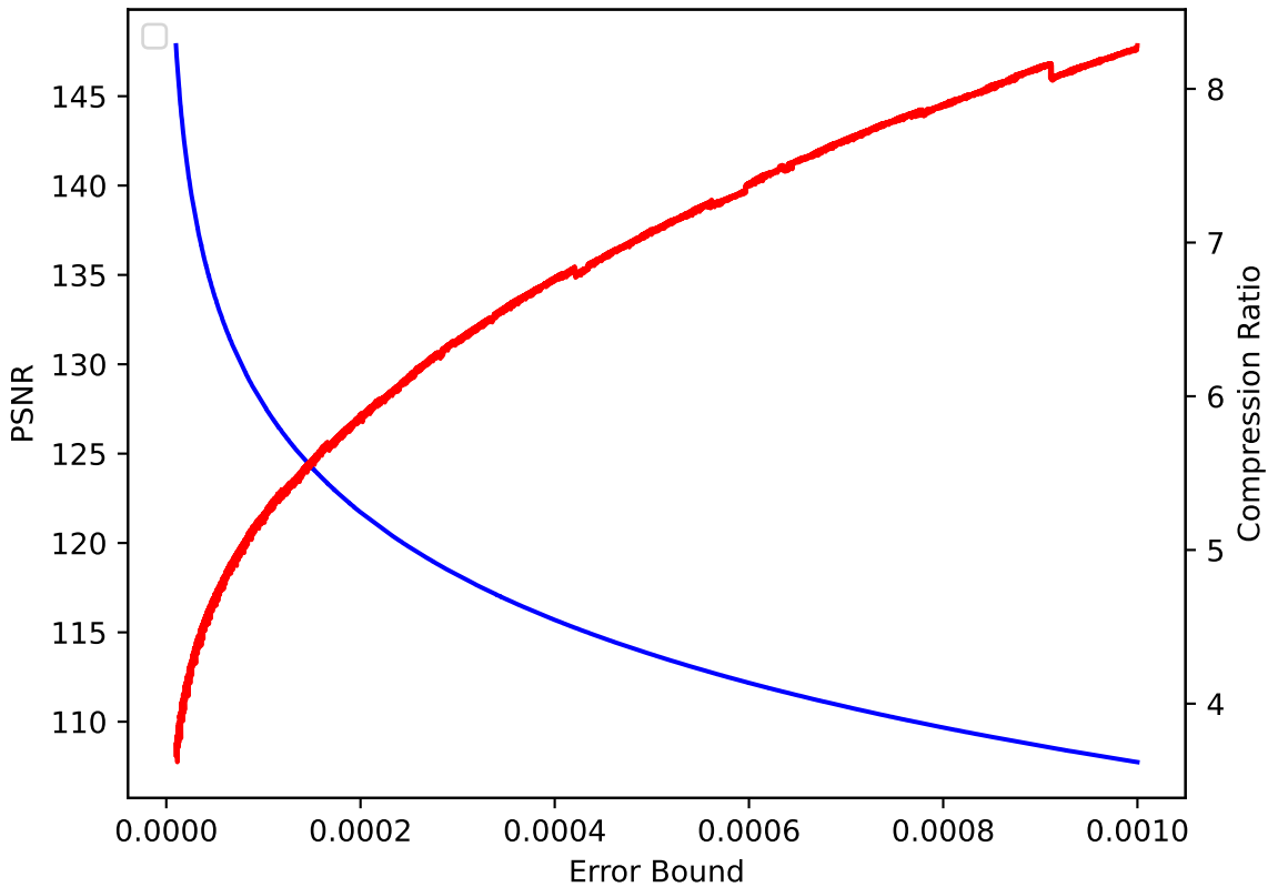
V 04 pressio:abs
