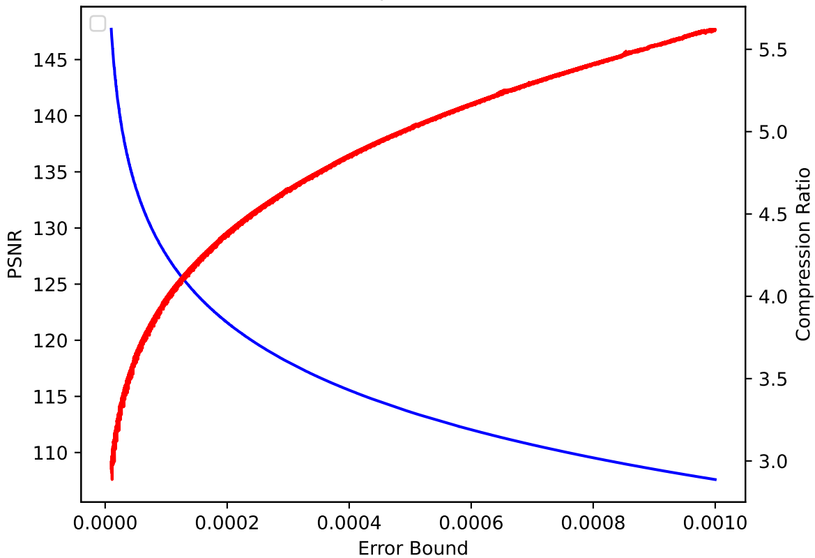
V 31 pressio:abs
