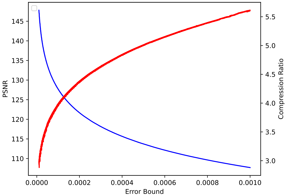
V 37 pressio:abs
