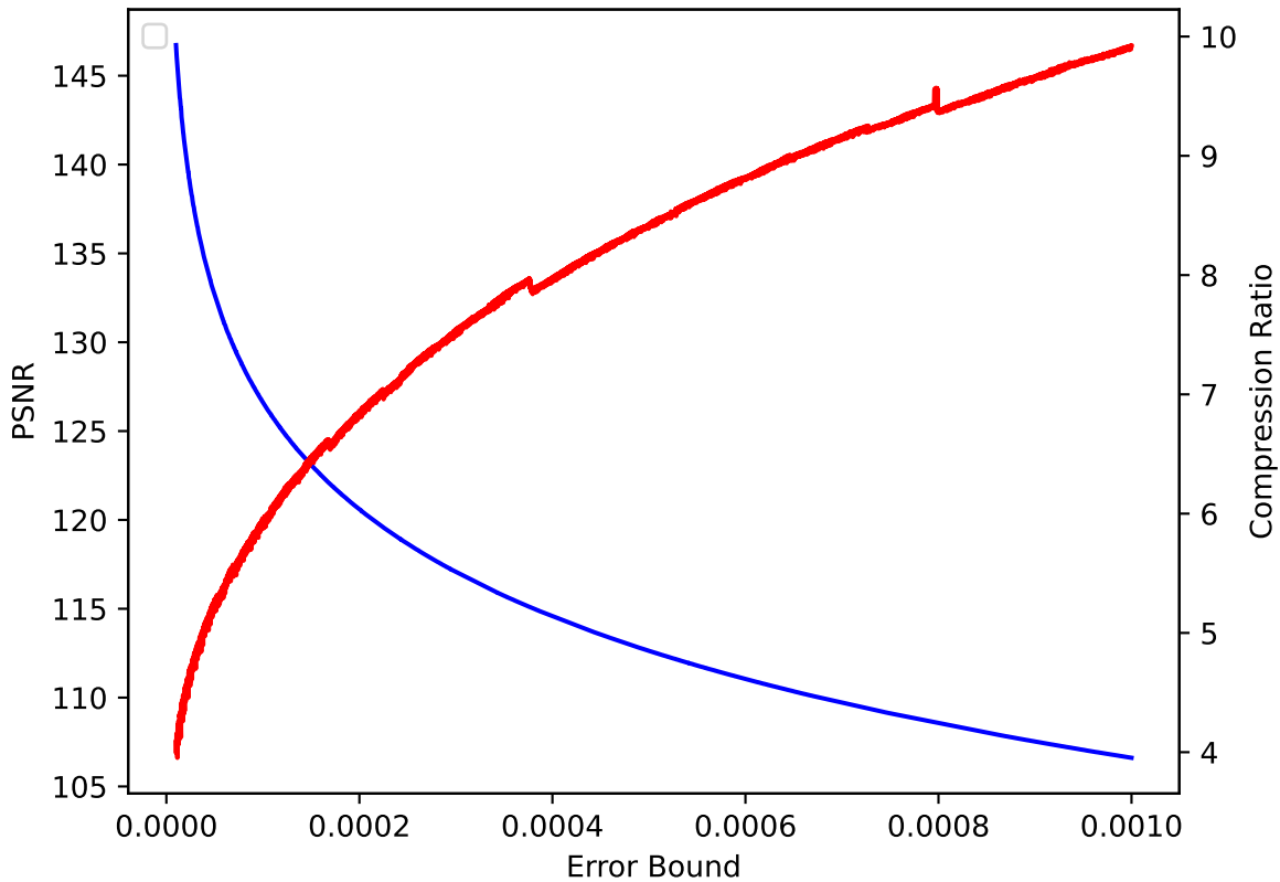
V 02 pressio:abs
