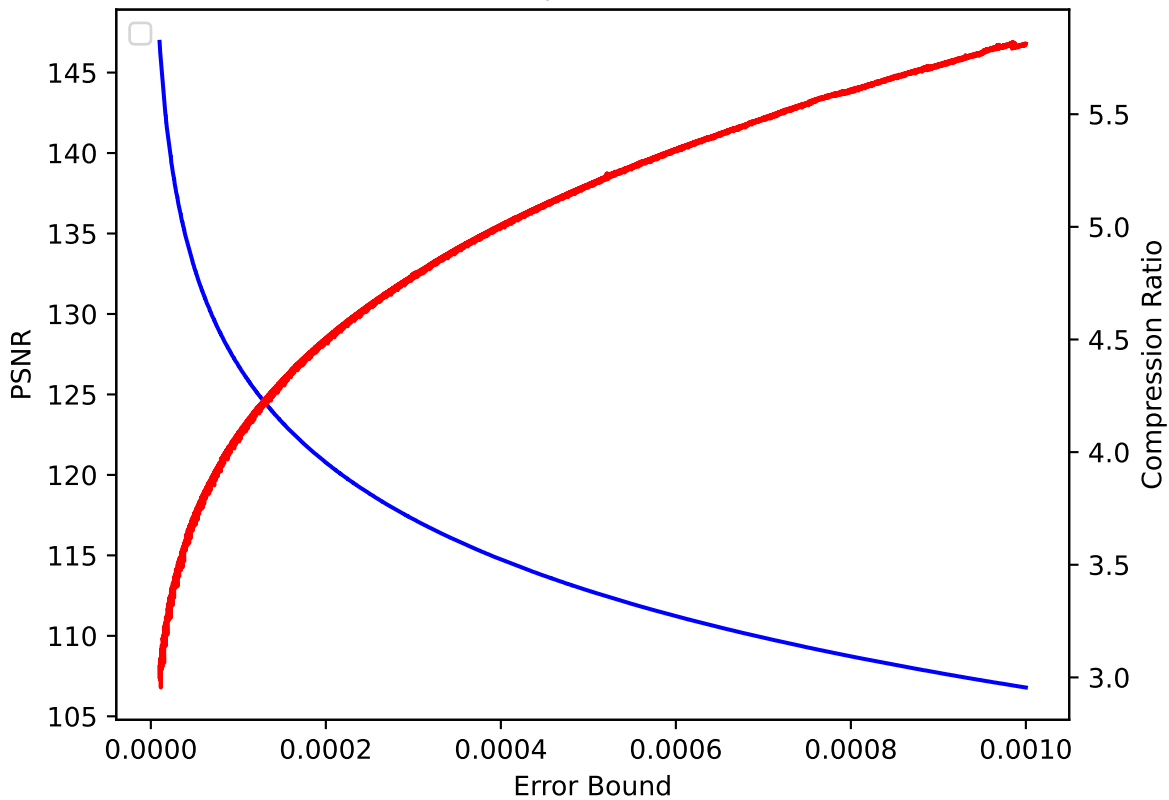
V 19 pressio:abs
