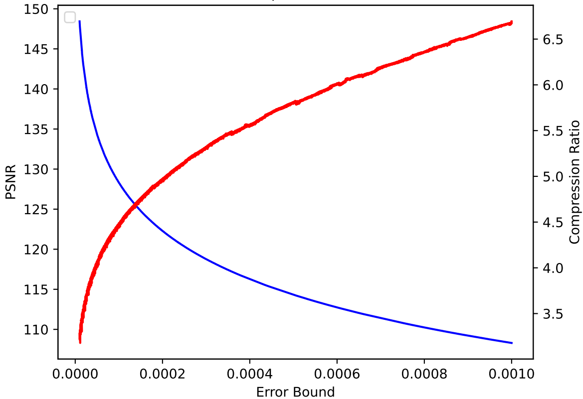
V 08 pressio:abs
