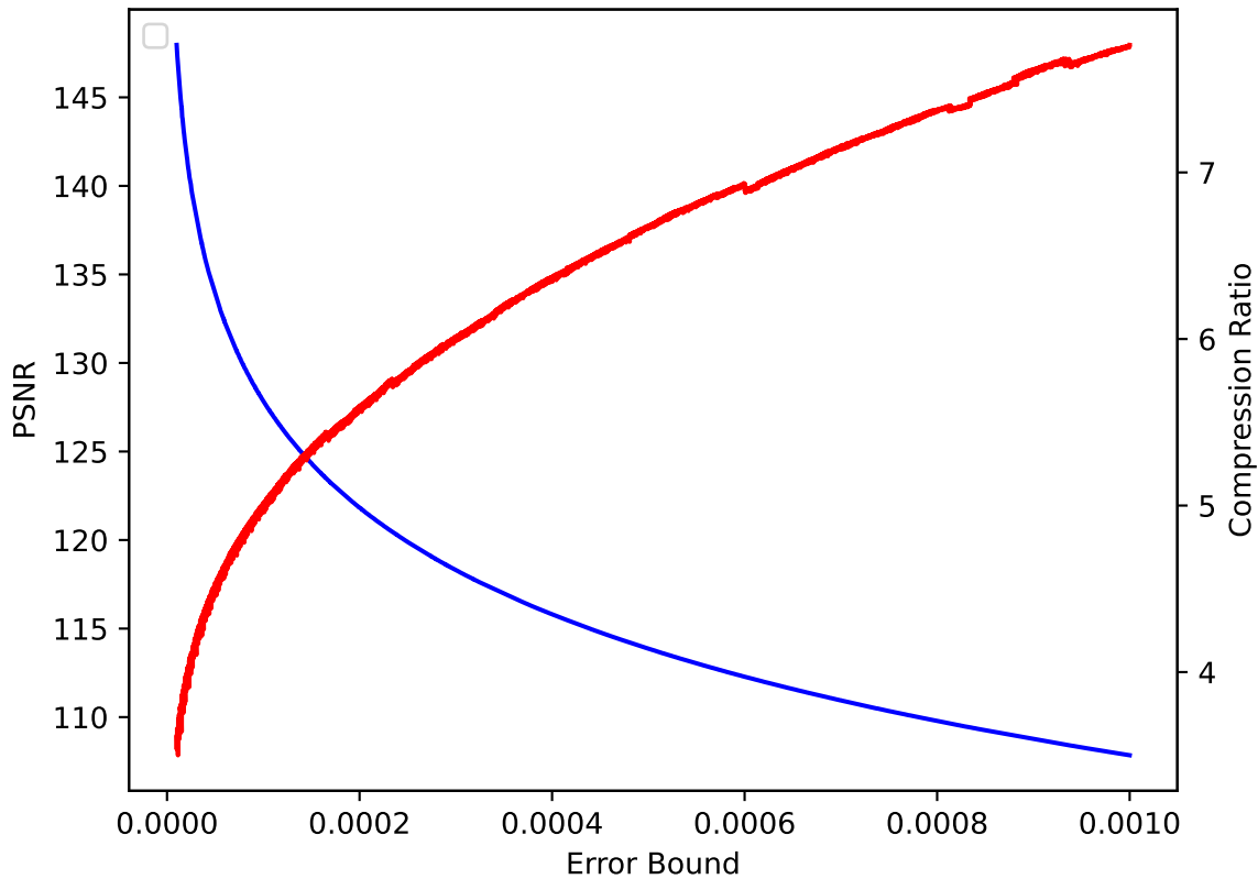
V 05 pressio:abs
