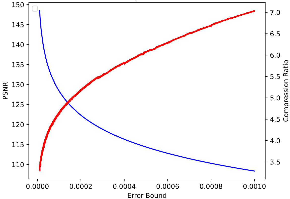
V 07 pressio:abs
