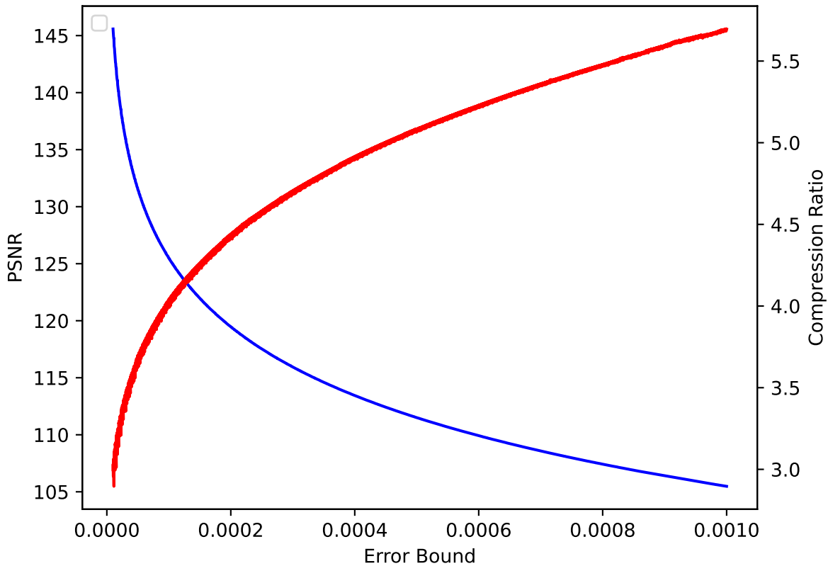
V 45 pressio:abs
