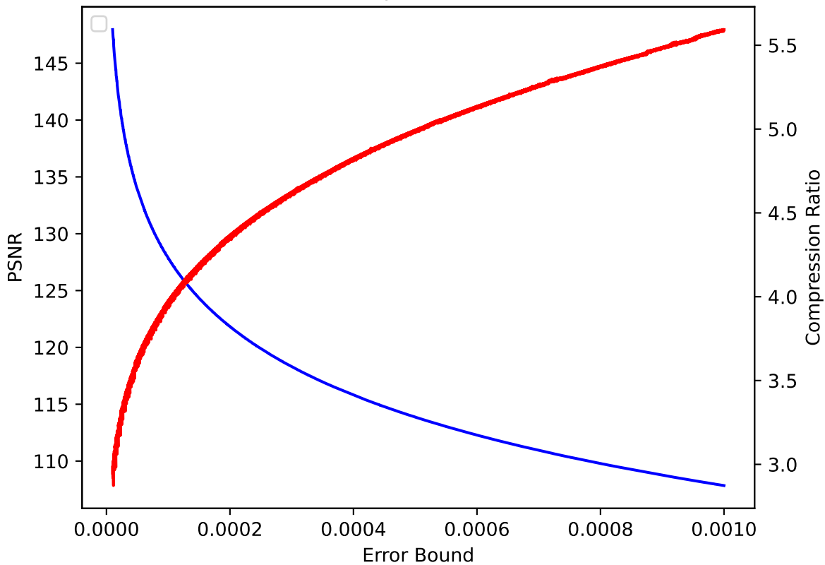
V 35 pressio:abs
