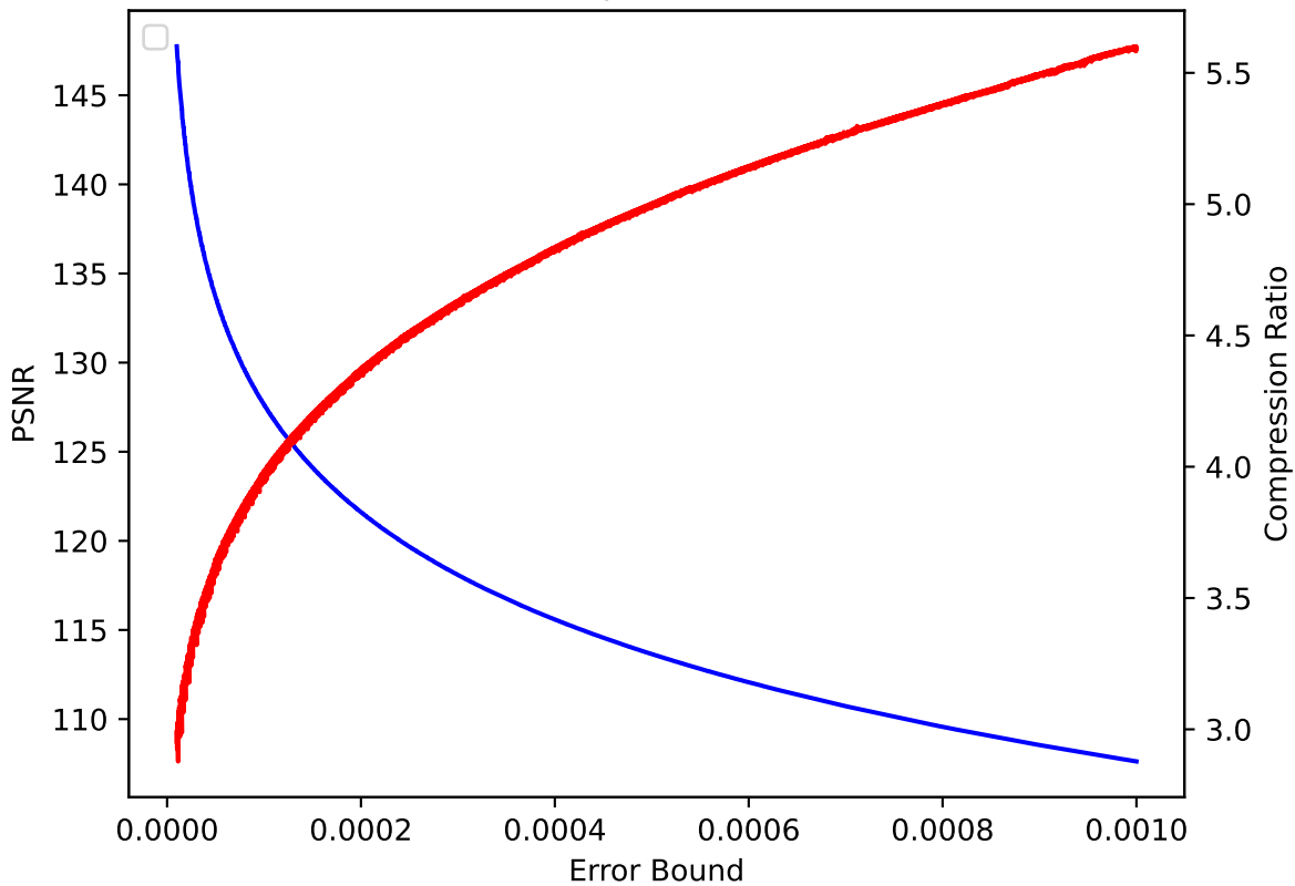
V 36 pressio:abs
