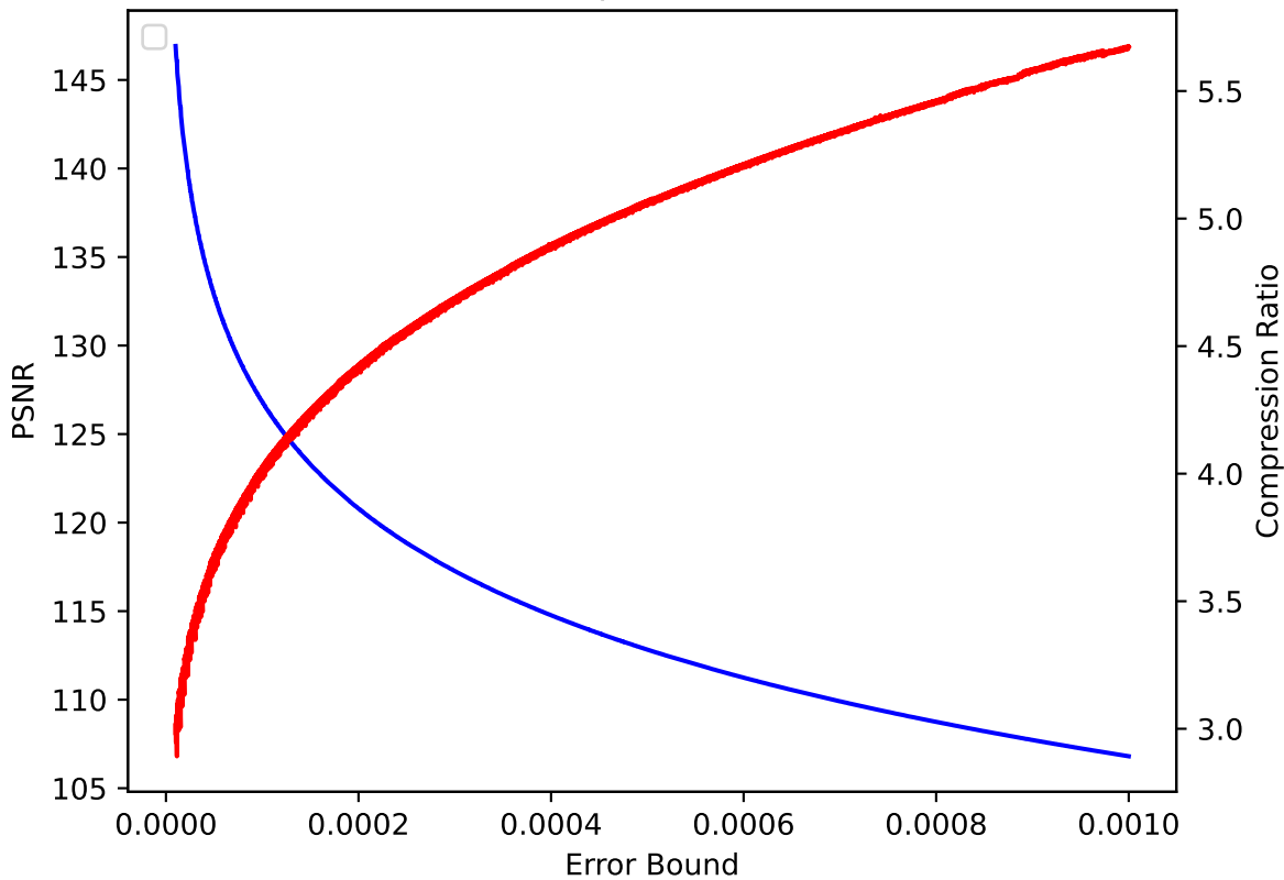
V 41 pressio:abs
