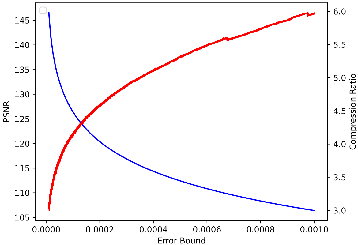
V 12 pressio:abs
