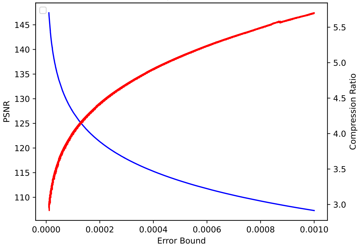
V 23 pressio:abs
