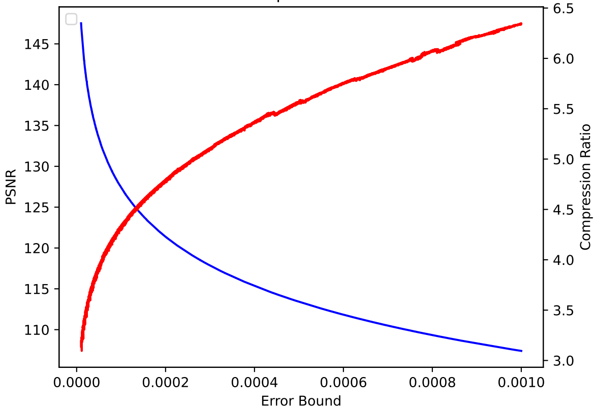
V 09 pressio:abs
