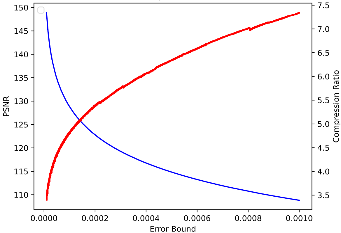
V 06 pressio:abs
