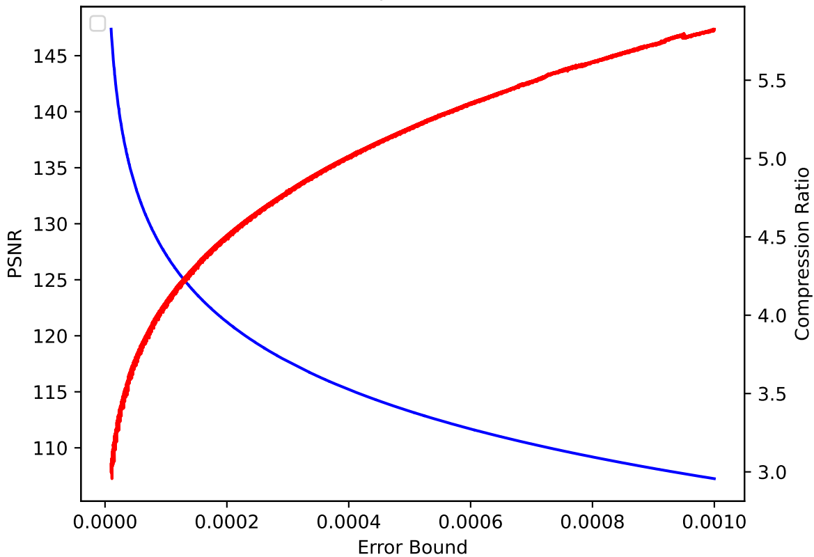
V 18 pressio:abs
