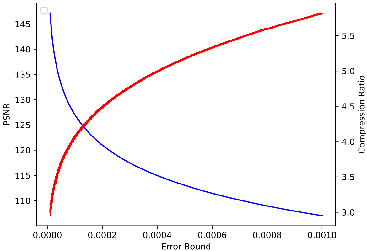
V 20 pressio:abs
