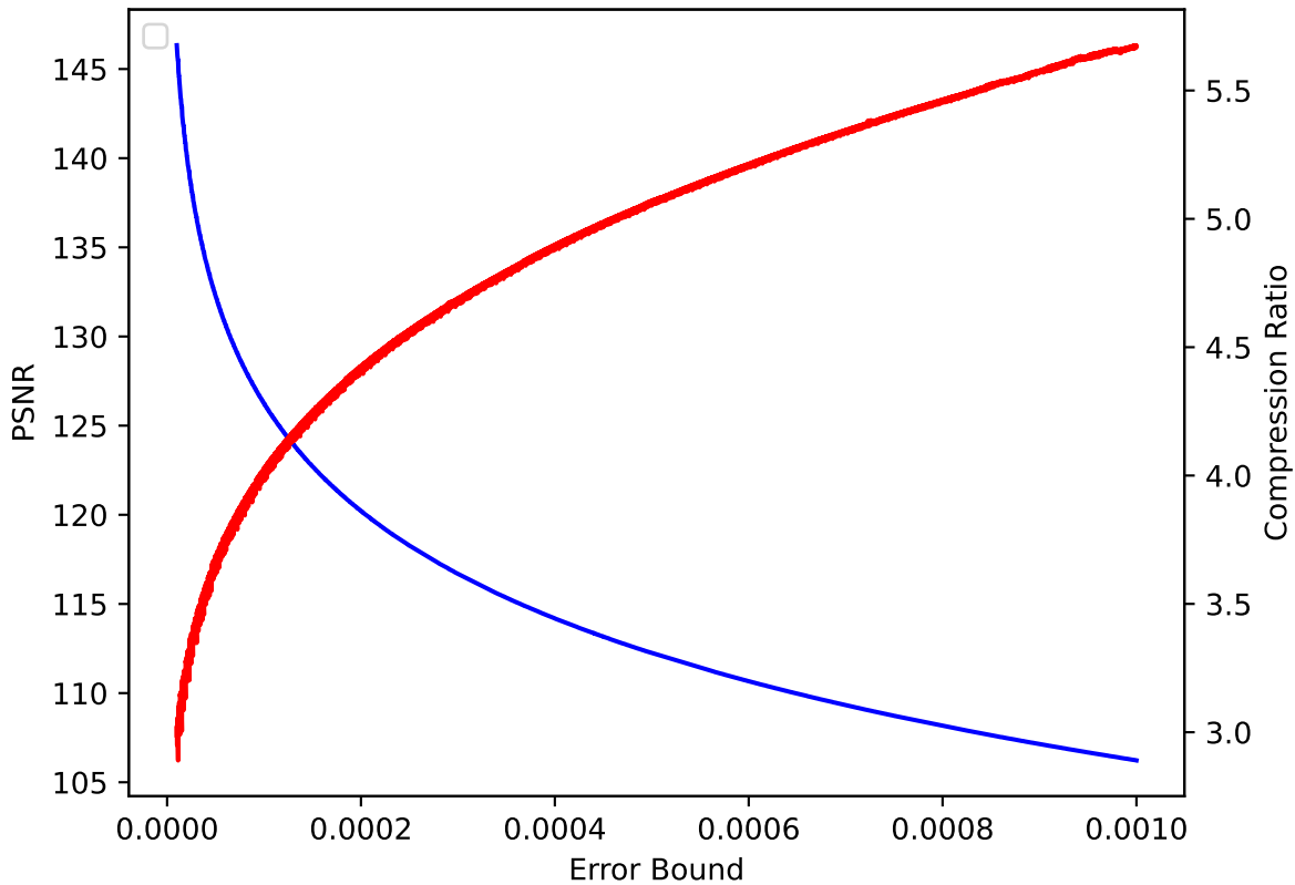
V 43 pressio:abs
