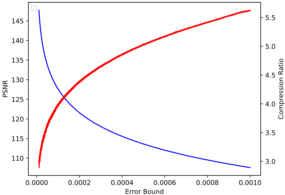
V 30 pressio:abs
