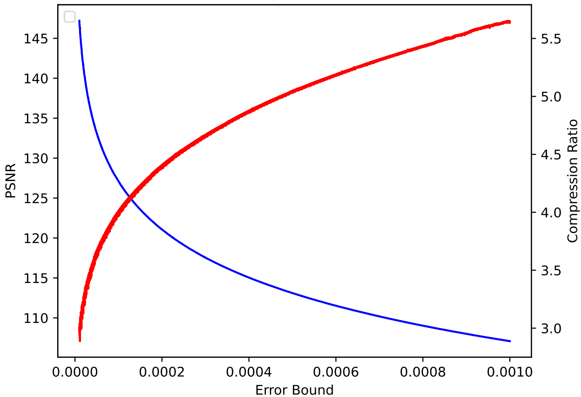
V 39 pressio:abs
