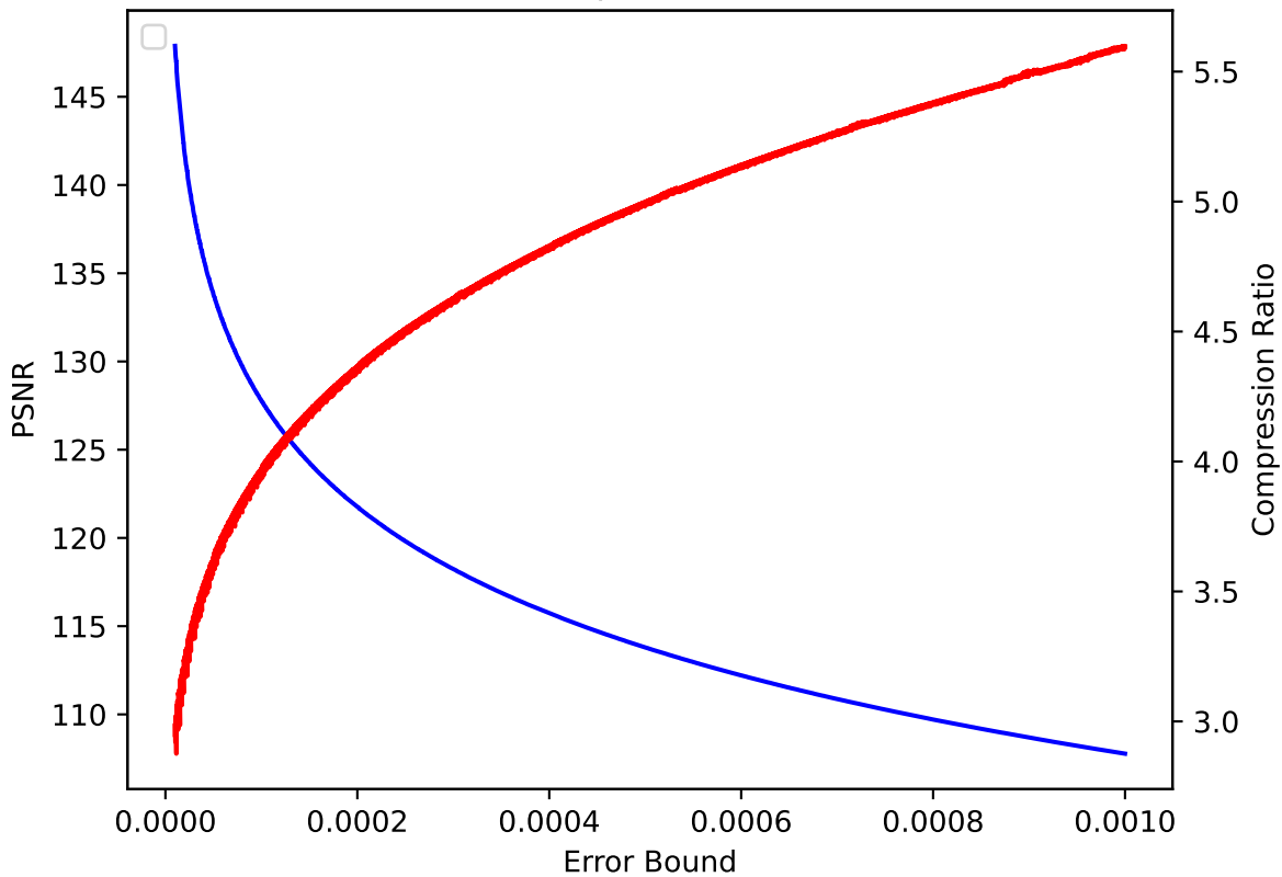
V 34 pressio:abs
