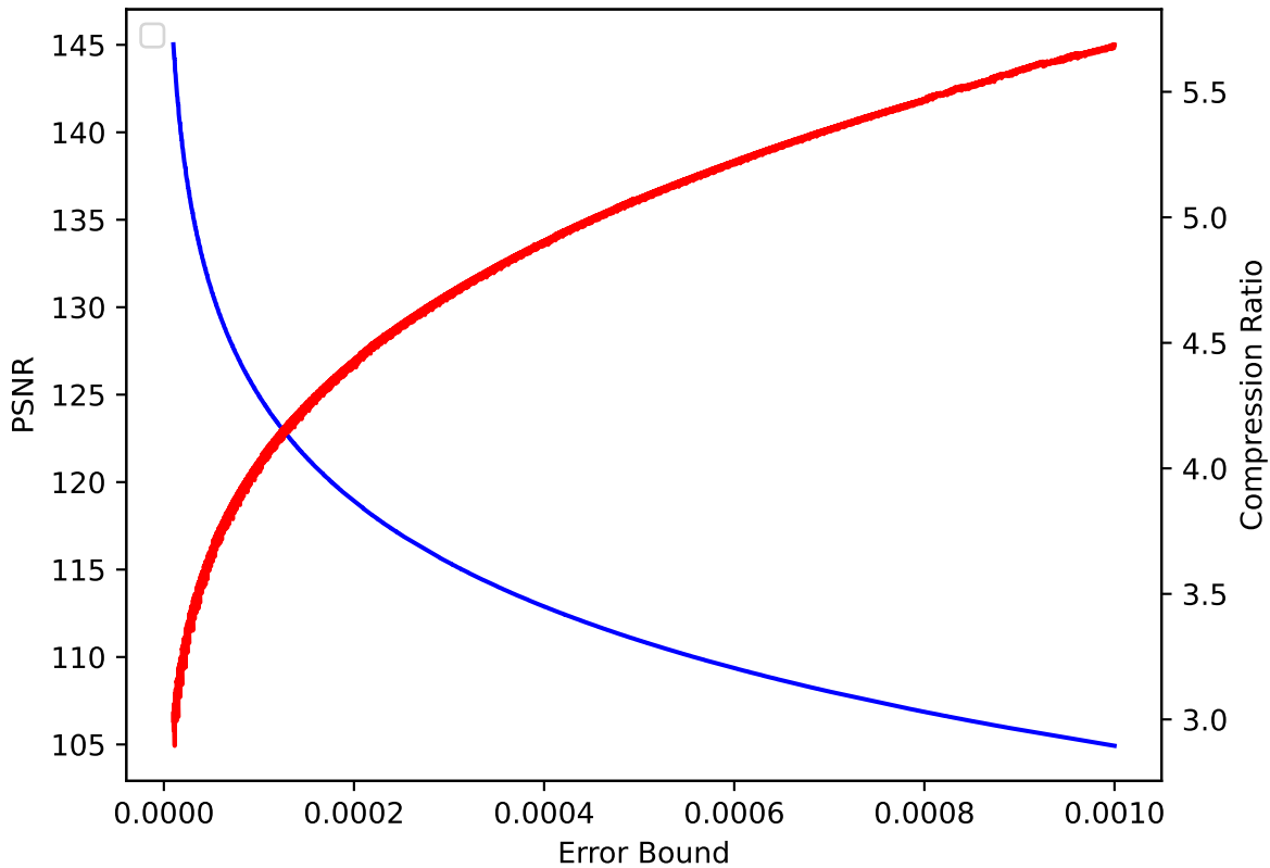
V 46 pressio:abs
