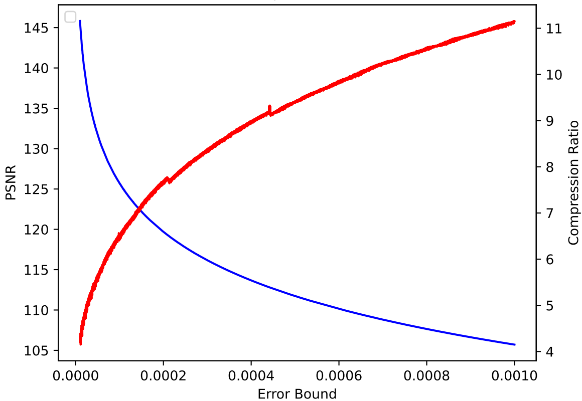
V 01 pressio:abs
