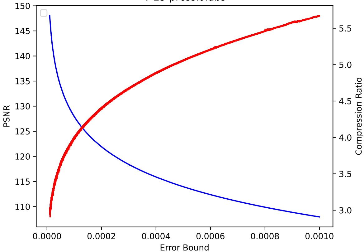
V 25 pressio:abs
