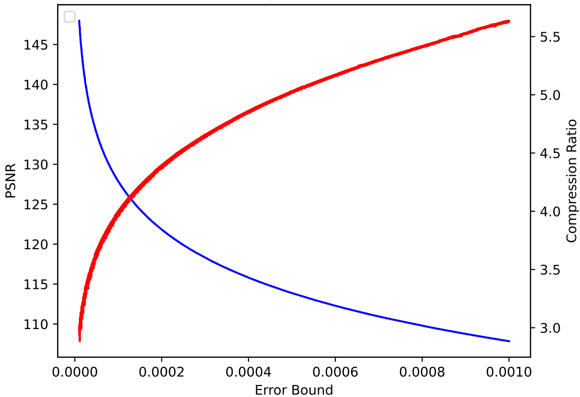
V 38 pressio:abs
