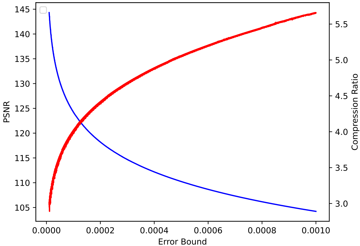
V 48 pressio:abs
