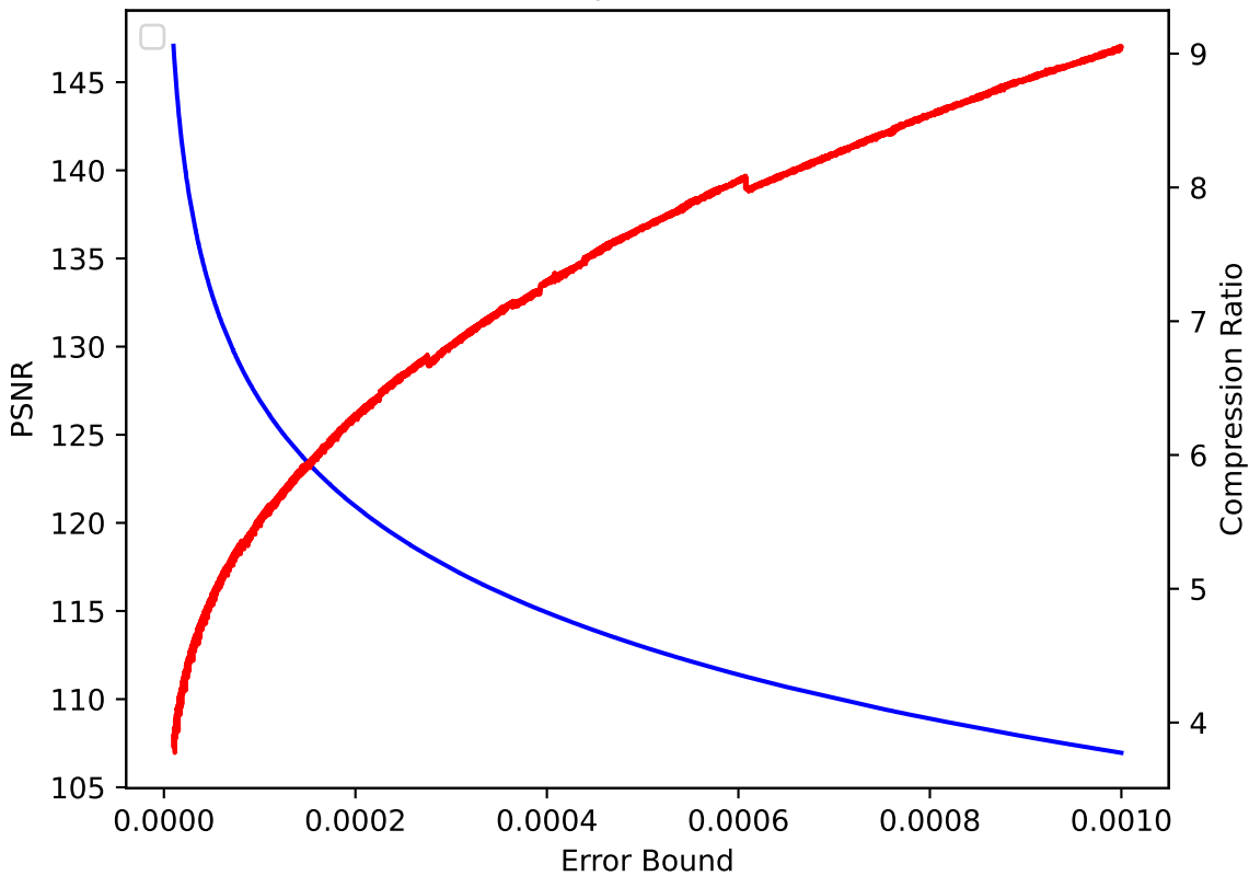
V 03 pressio:abs
