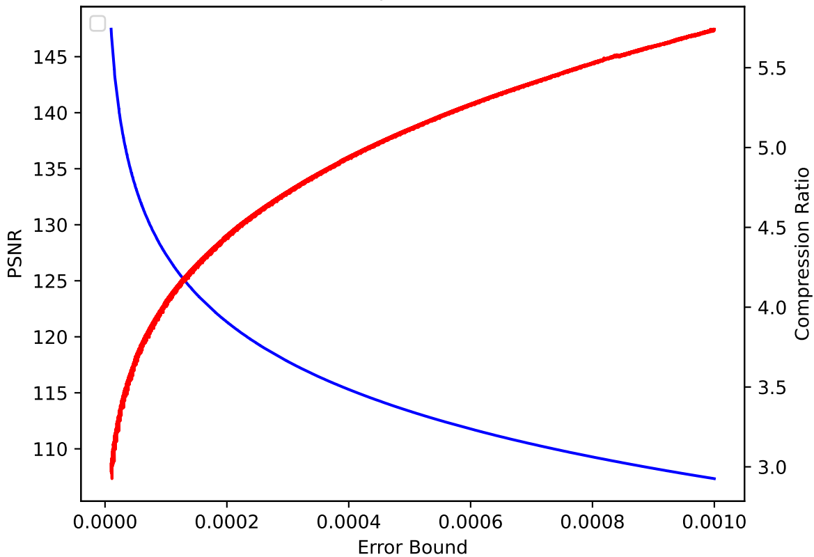
V 22 pressio:abs
