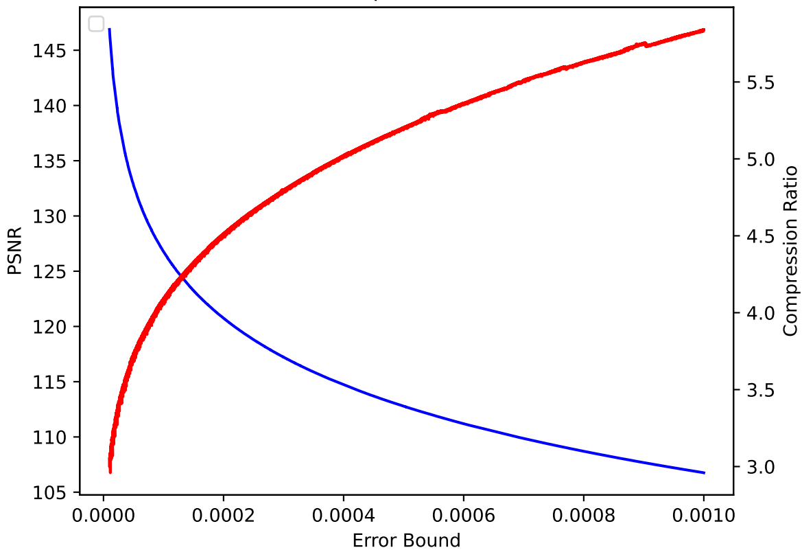
V 17 pressio:abs
