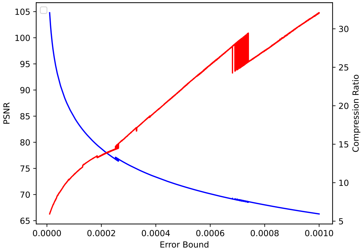
V 32 pressio:rel
