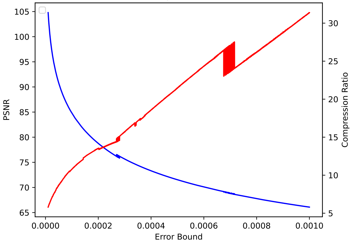
V 44 pressio:rel
