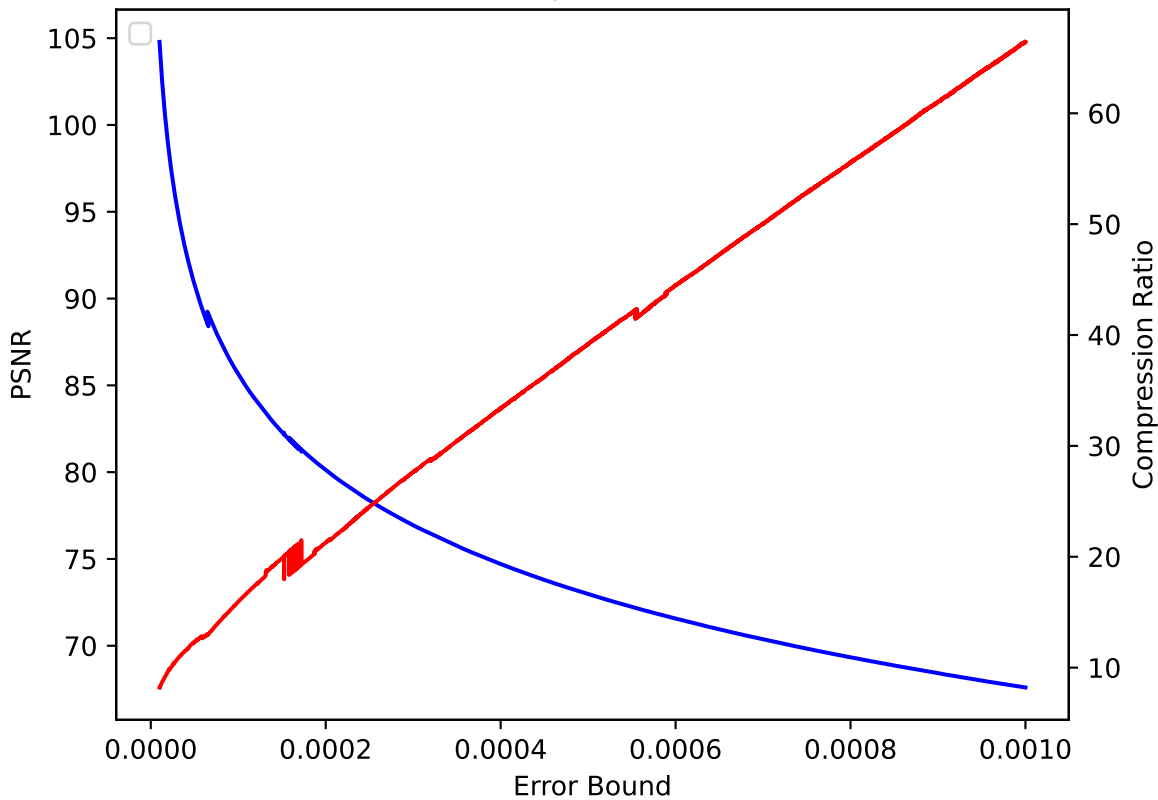
V 06 pressio:rel
