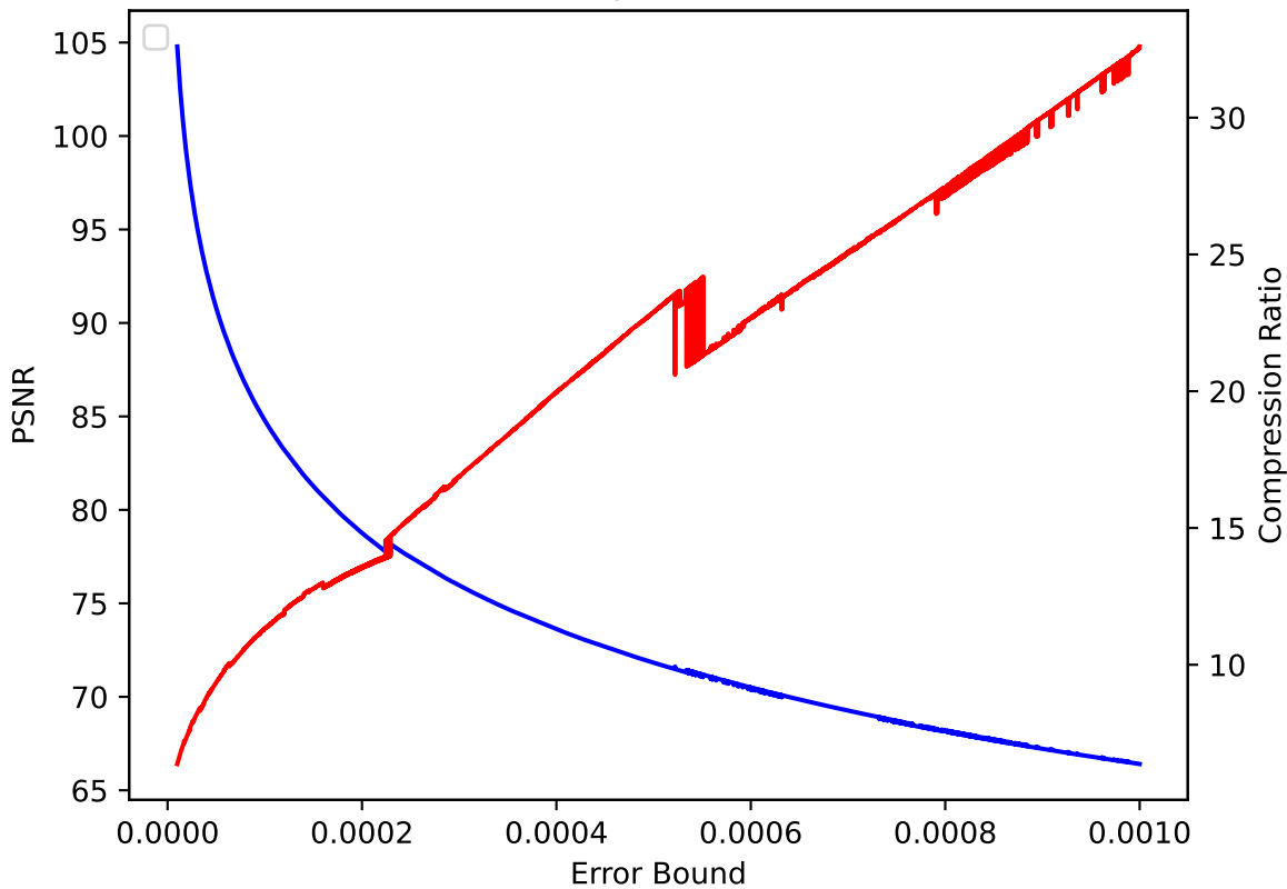
V 11 pressio:rel
