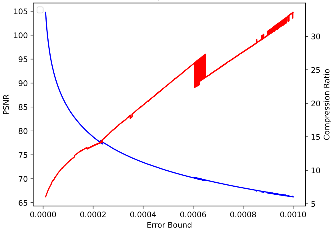
V 24 pressio:rel
