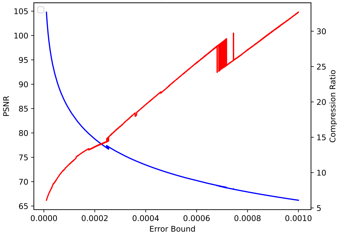
V 17 pressio:rel
