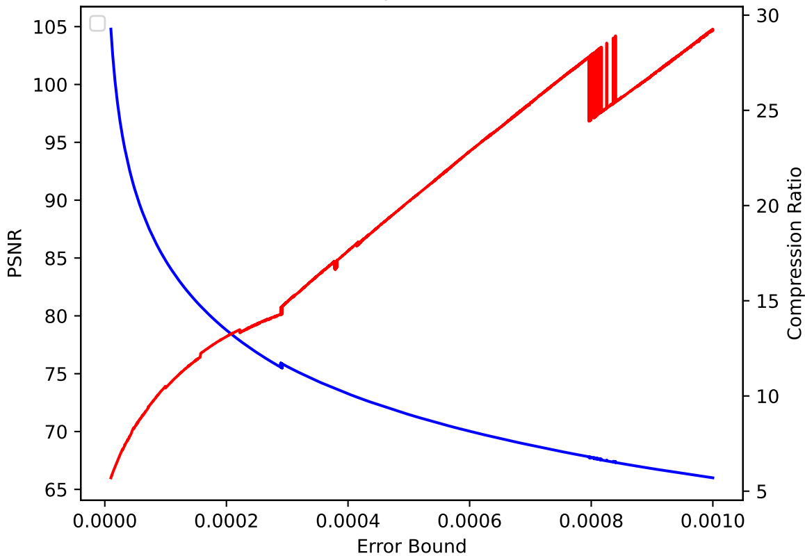
V 46 pressio:rel
