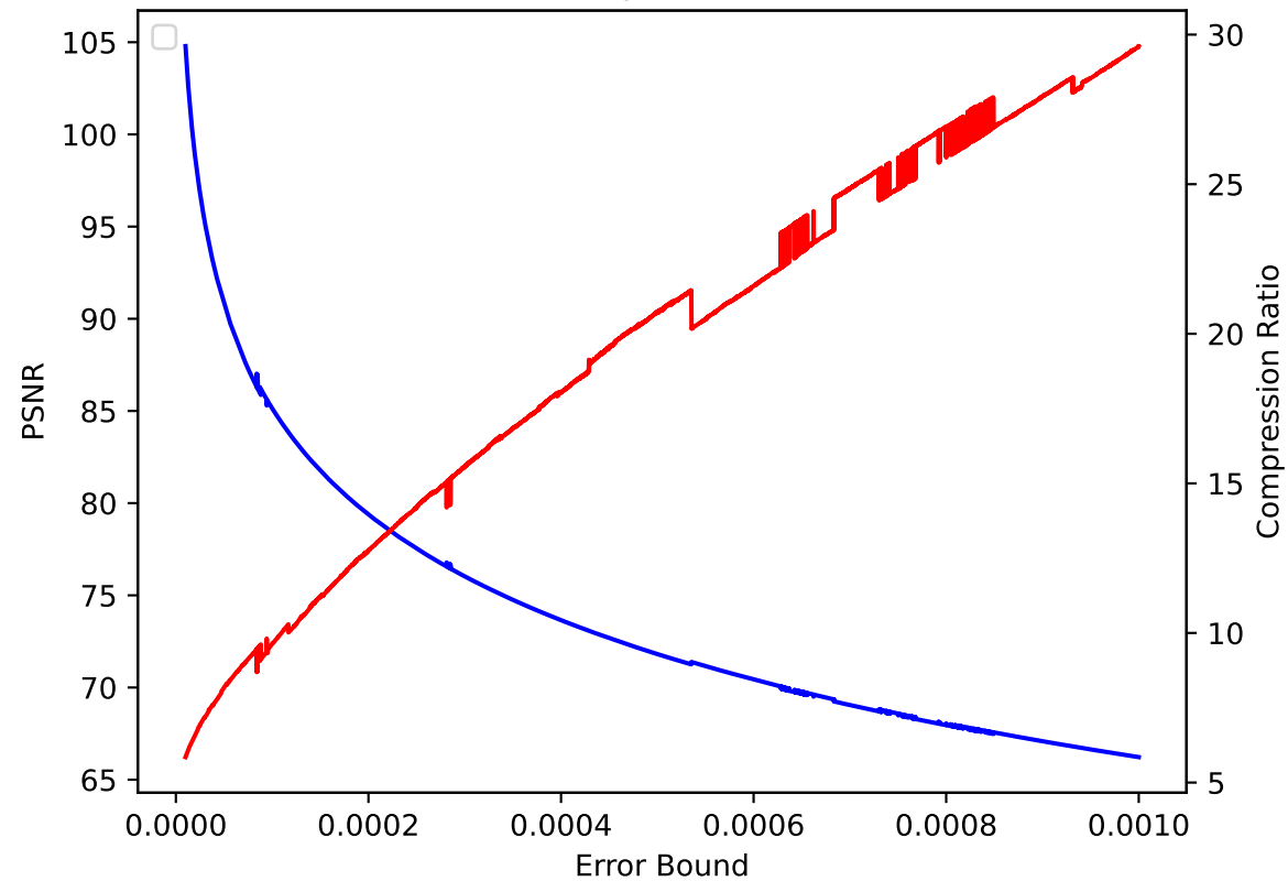
W 26 pressio:rel
