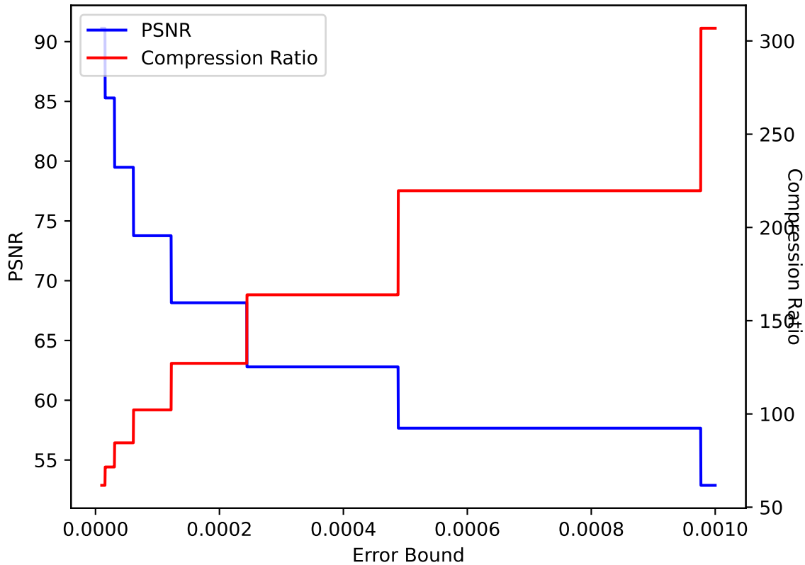
QCLLOUD 20 ZFP pressio:abs
