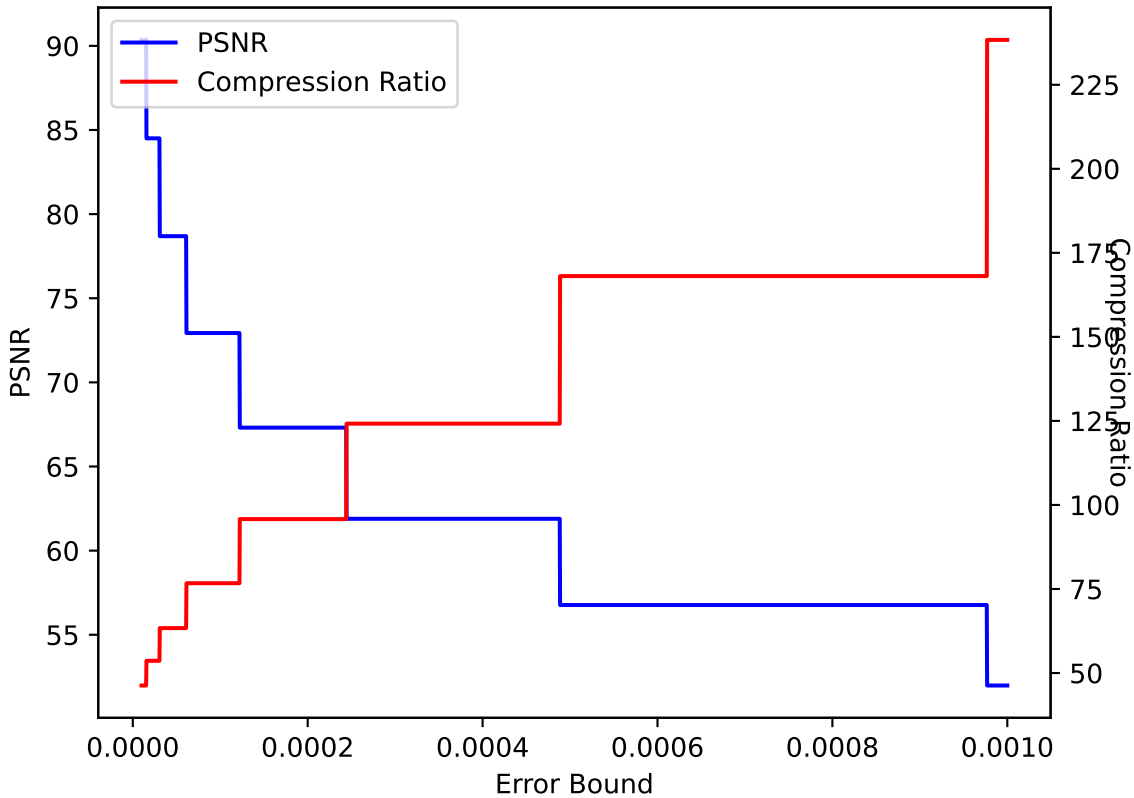
QCLoud 33 ZFP pressio:abs
