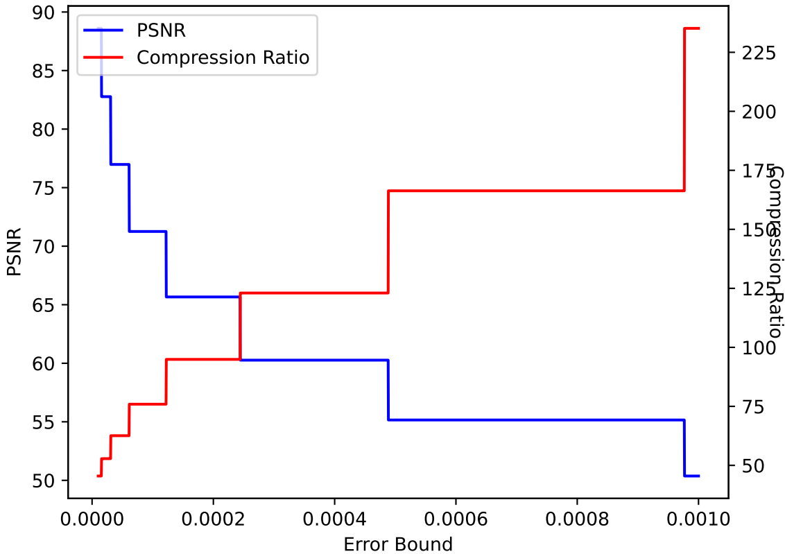
QCLoud 35 ZFP pressio:abs
