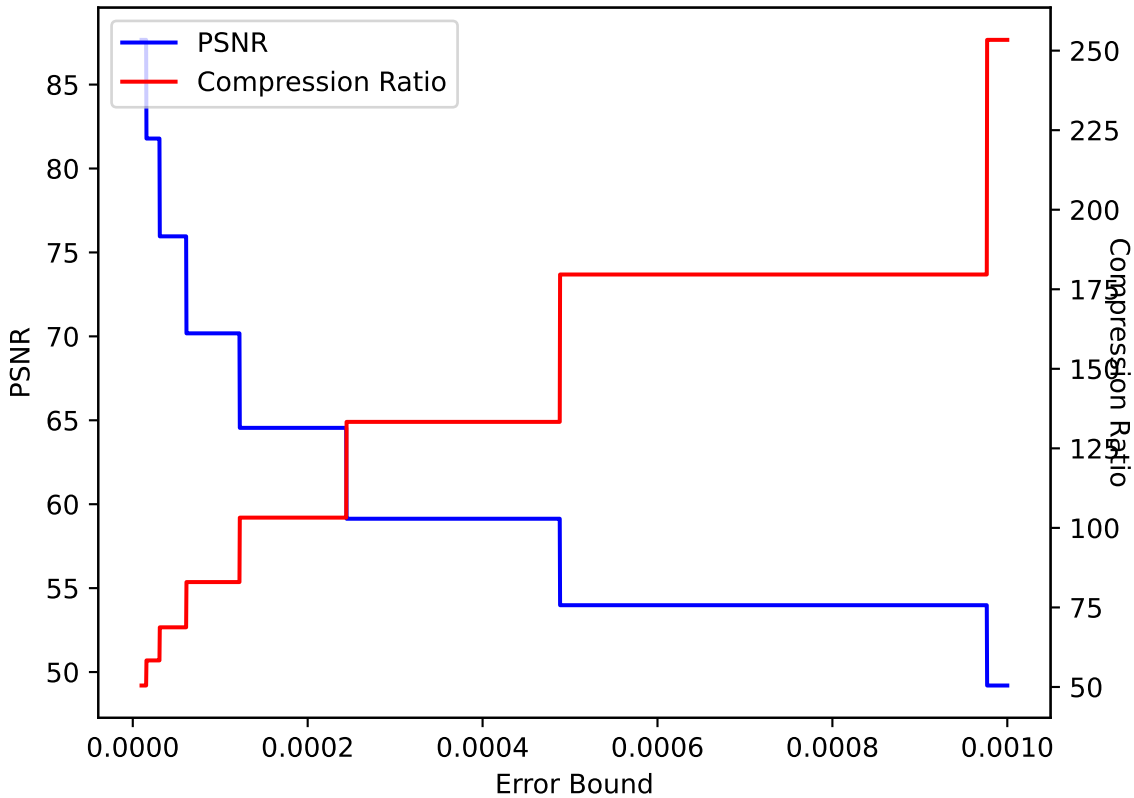
QCLLOUD 29 ZFP pressio:abs
