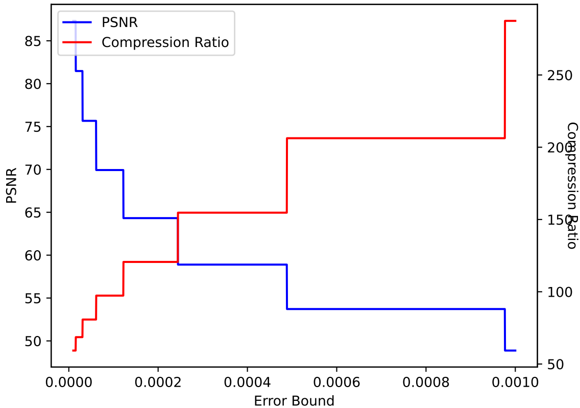
QCLoud 21 ZFP pressio:abs
