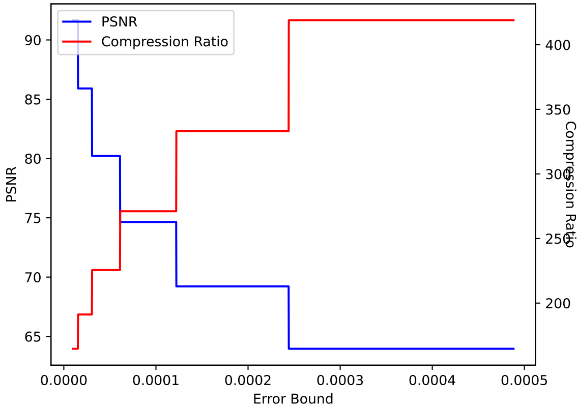
QCLLOUD 05 ZFP pressio:abs
