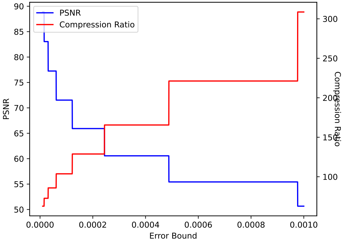
QCLLOUD 14 ZFP pressio:abs
