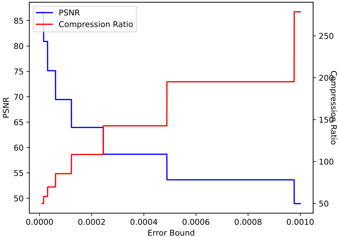
QCLLOUD 42 ZFP pressio:abs
