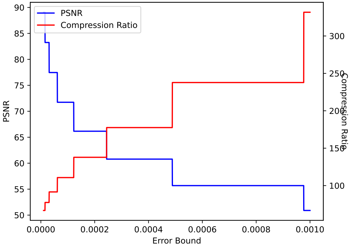
QCLLOUD 18 ZFP pressio:abs
