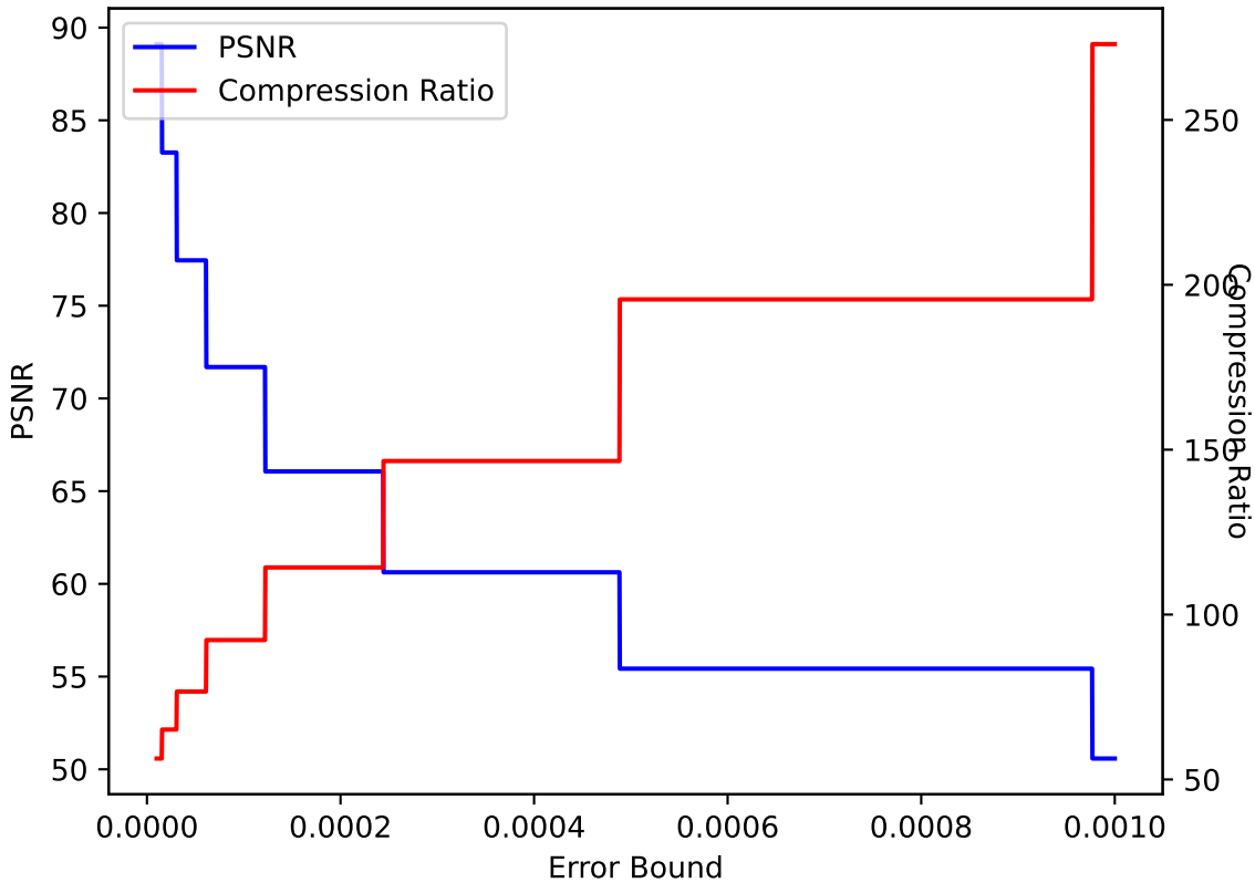
QCLOUD 22 ZFP pressio:abs
