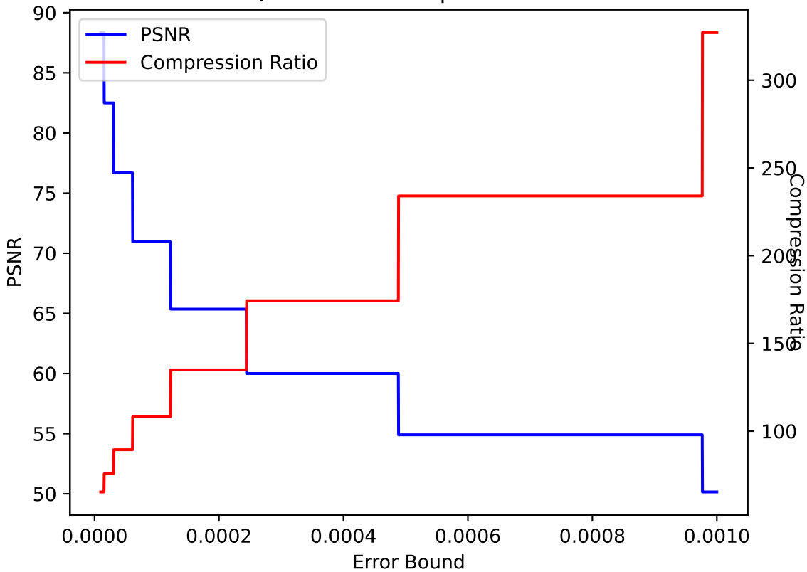
QCLLOUD 19 ZFP pressio:abs
