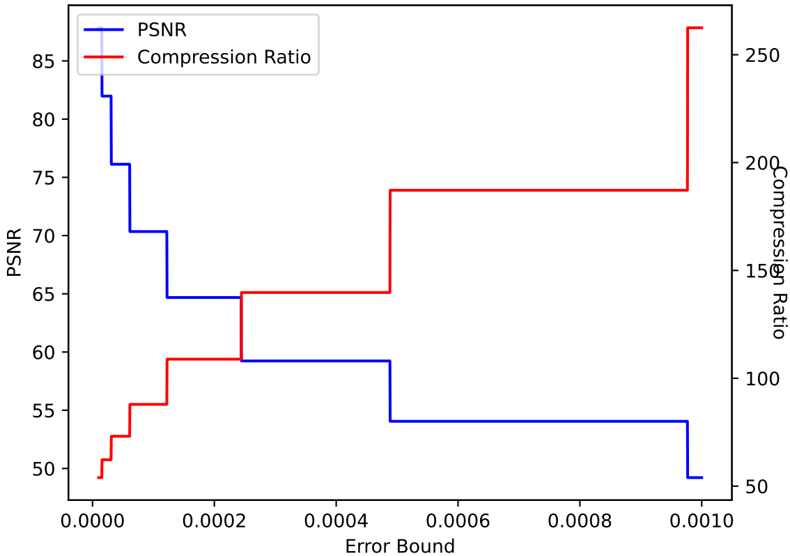
QCLoud 24 ZFP pressio:abs
