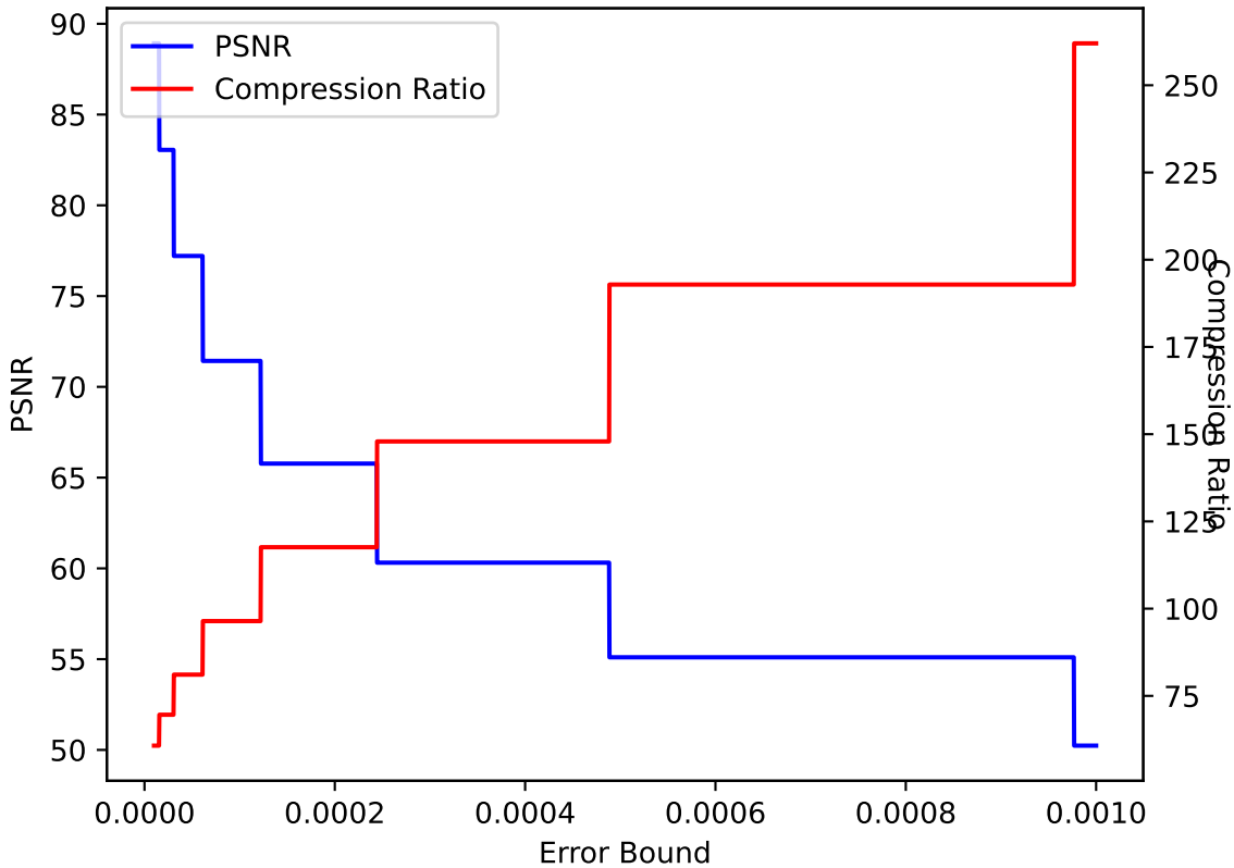
QCLoud 09 ZFP pressio:abs
