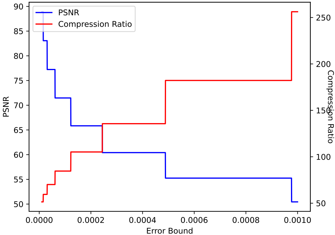
QCLLOUD 28 ZFP pressio:abs
