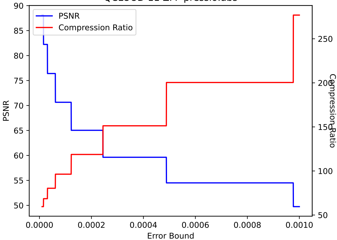
QCLLOUD 11 ZFP pressio:abs
