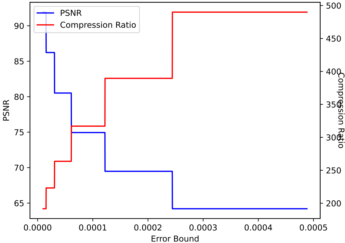
QCLOUD 04 ZFP pressio:abs
