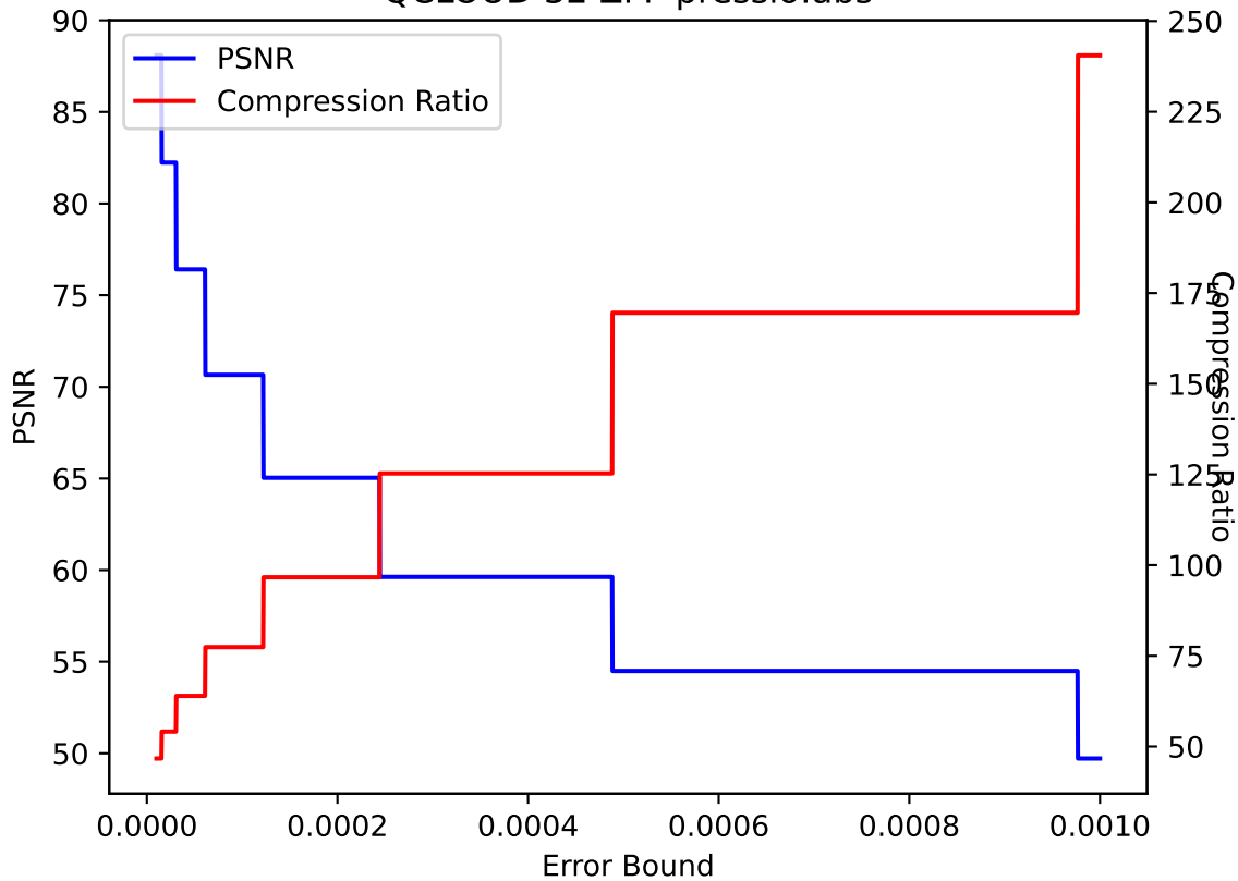
QCLoud 32 ZFP pressio:abs
