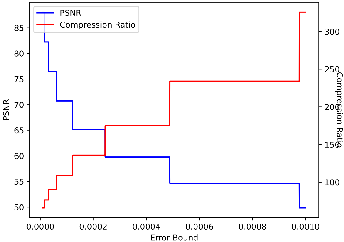
QCLOUD 17 ZFP pressio:abs
