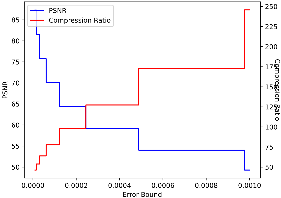
QCLLOUD 37 ZFP pressio:abs
