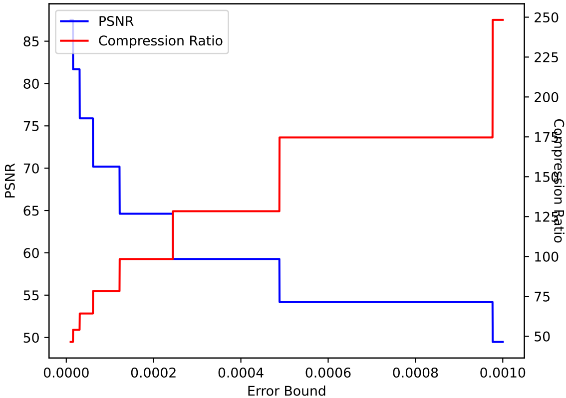
QCLoud 38 ZFP pressio:abs
