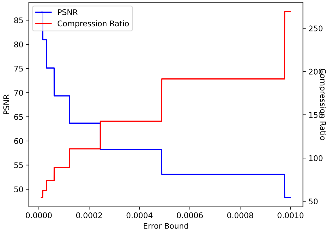
QCLoud 25 ZFP pressio:abs
