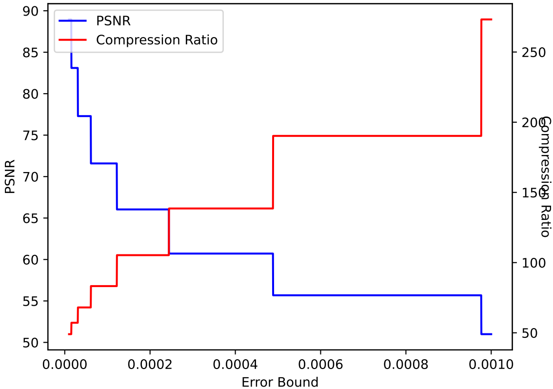
QCLOUD 47 ZFP pressio:abs
