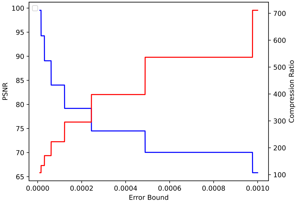
QGRAUP 48 pressio:abs
