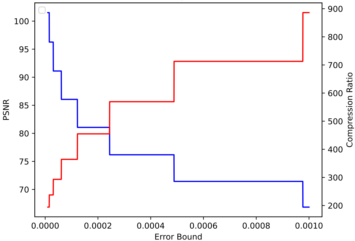
QGRAUP 04 pressio:abs
