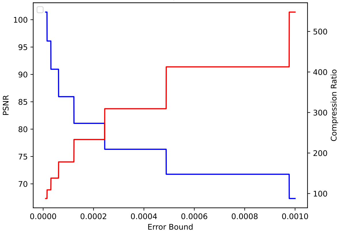
QGRAUP 35 pressio:abs
