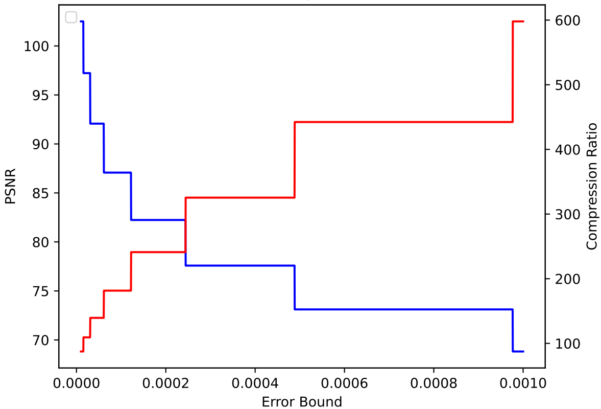
QGRAUP 41 pressio:abs
