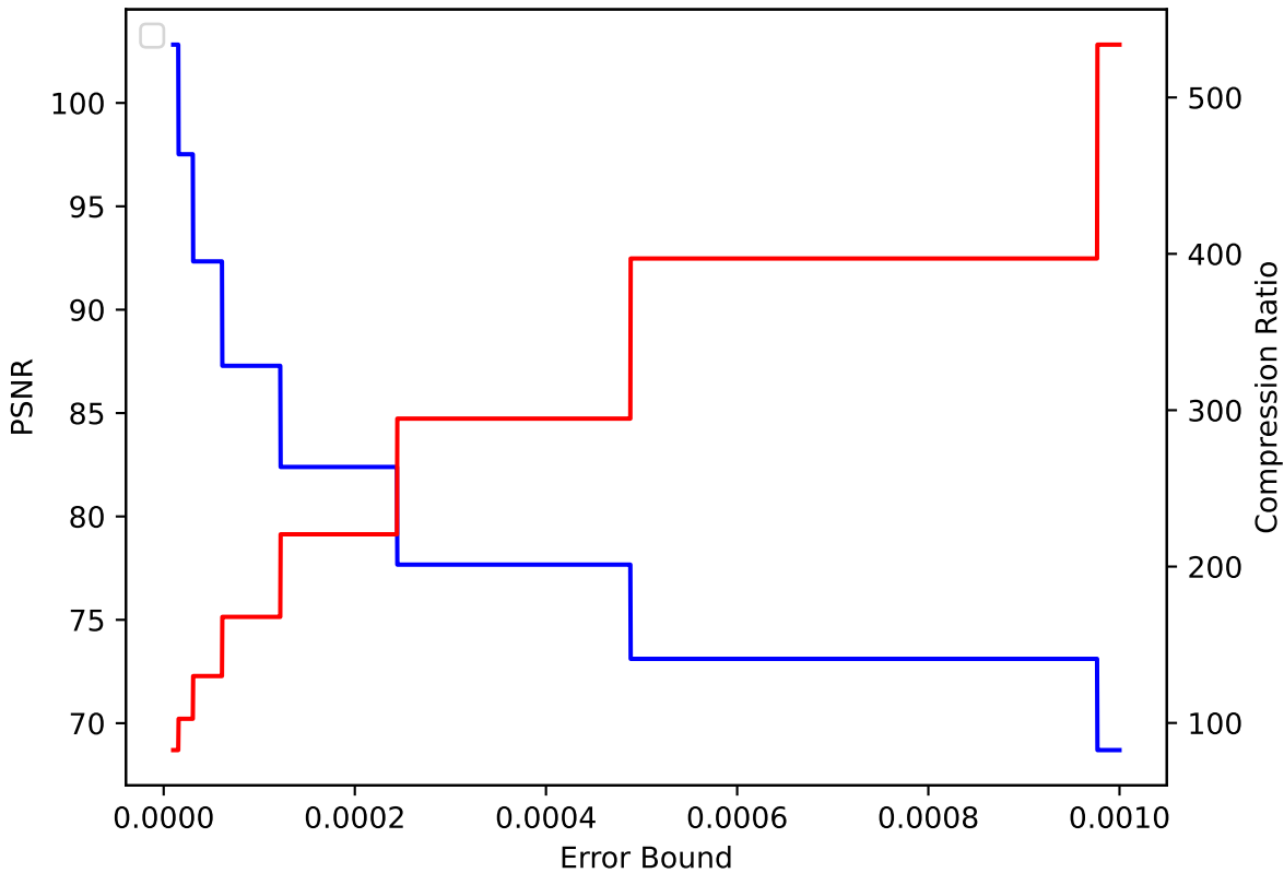
QGRAUP 38 pressio:abs
