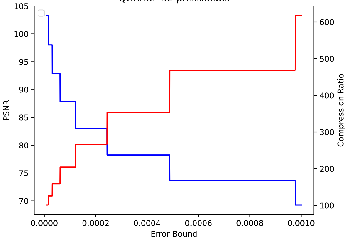
QGRAUP 32 pressio:abs
