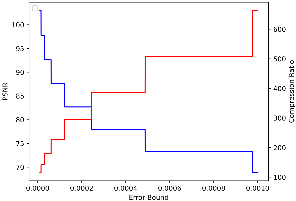
QGRAUP 24 pressio:abs
