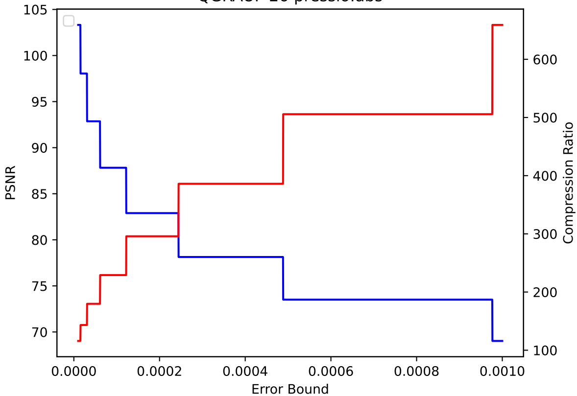
QGRAUP 26 pressio:abs
