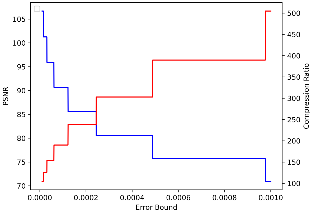
QGRAUP 09 pressio:abs
