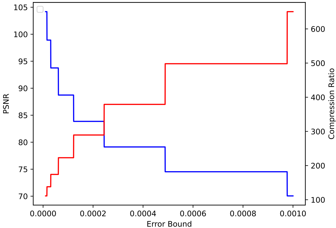
QGRAUP 17 pressio:abs
