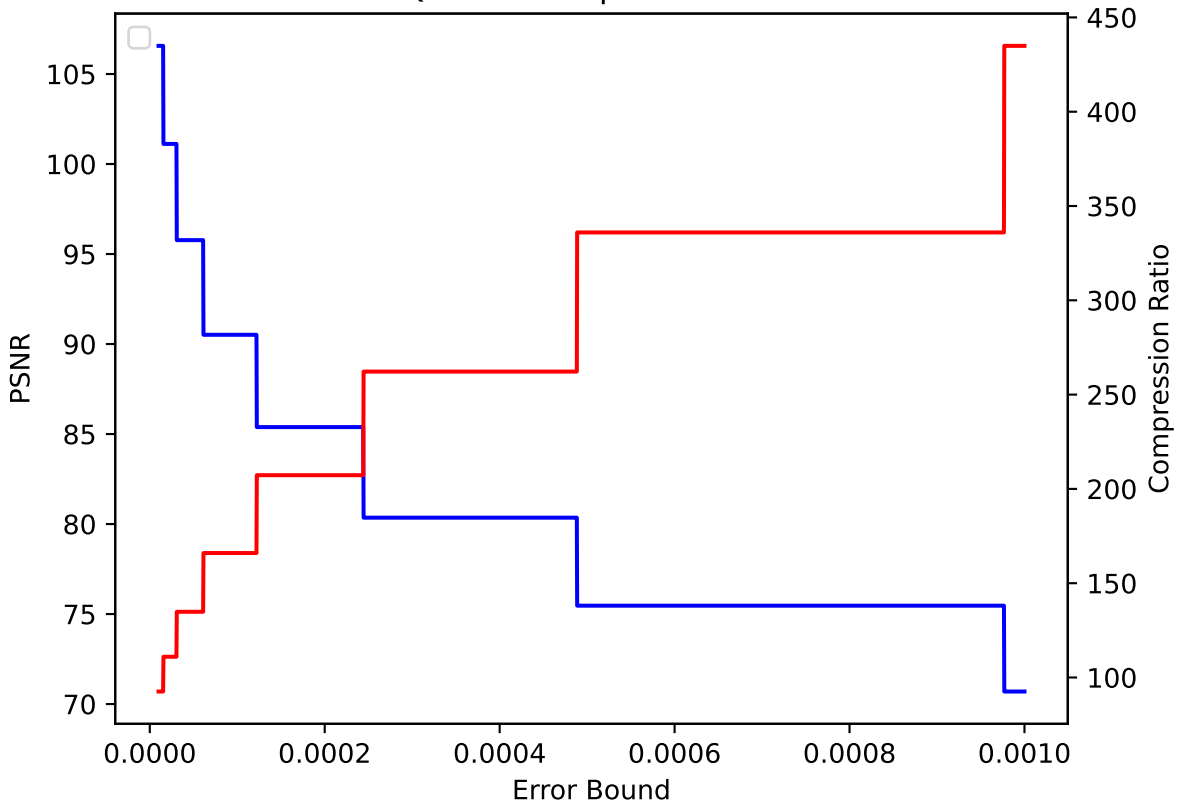
QGRAUP 10 pressio:abs
