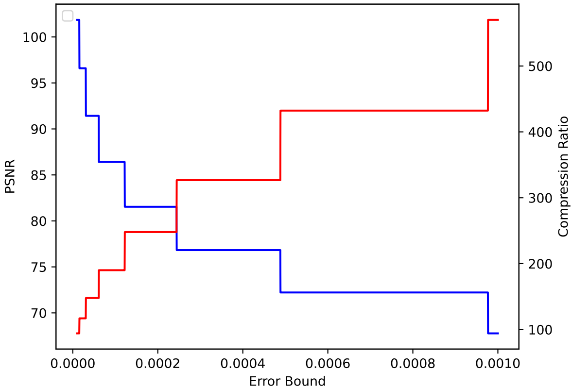
QGRAUP 34 pressio:abs
