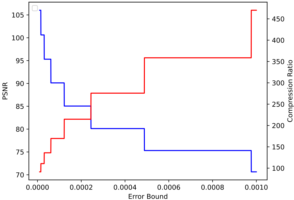
QGRAUP 12 pressio:abs
