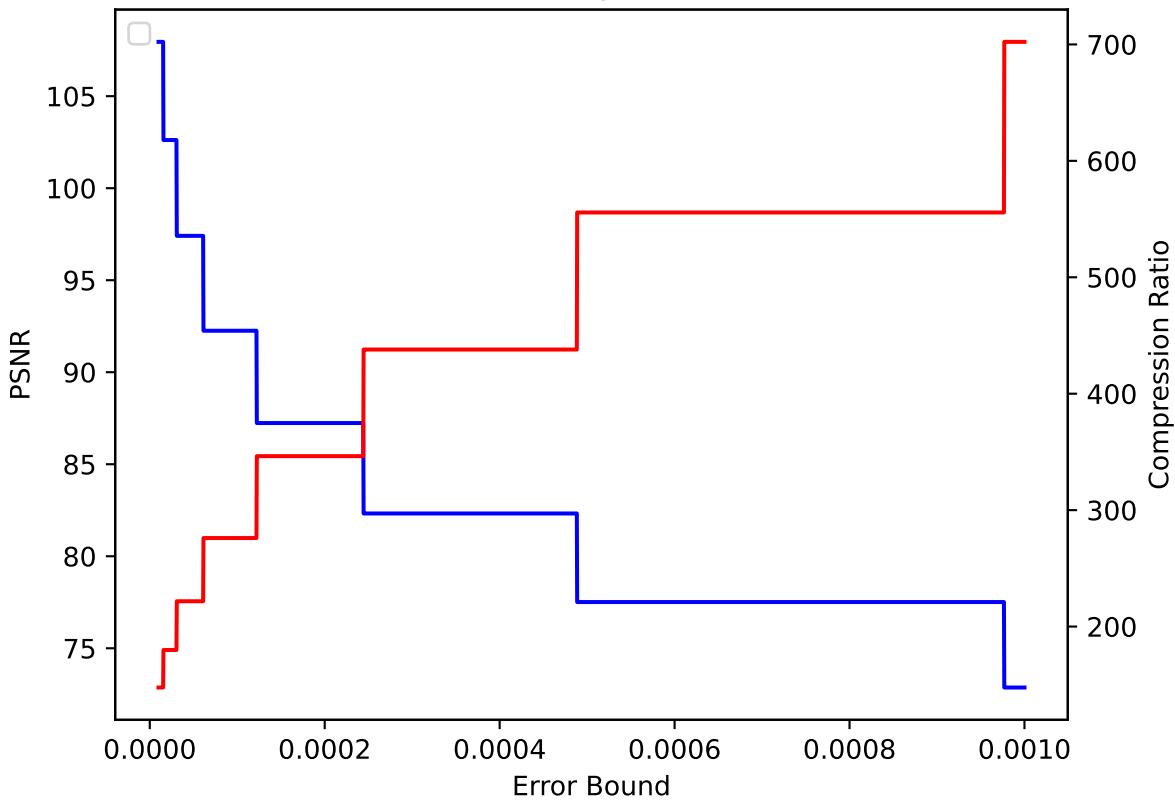
QGRAUP 07 pressio:abs
