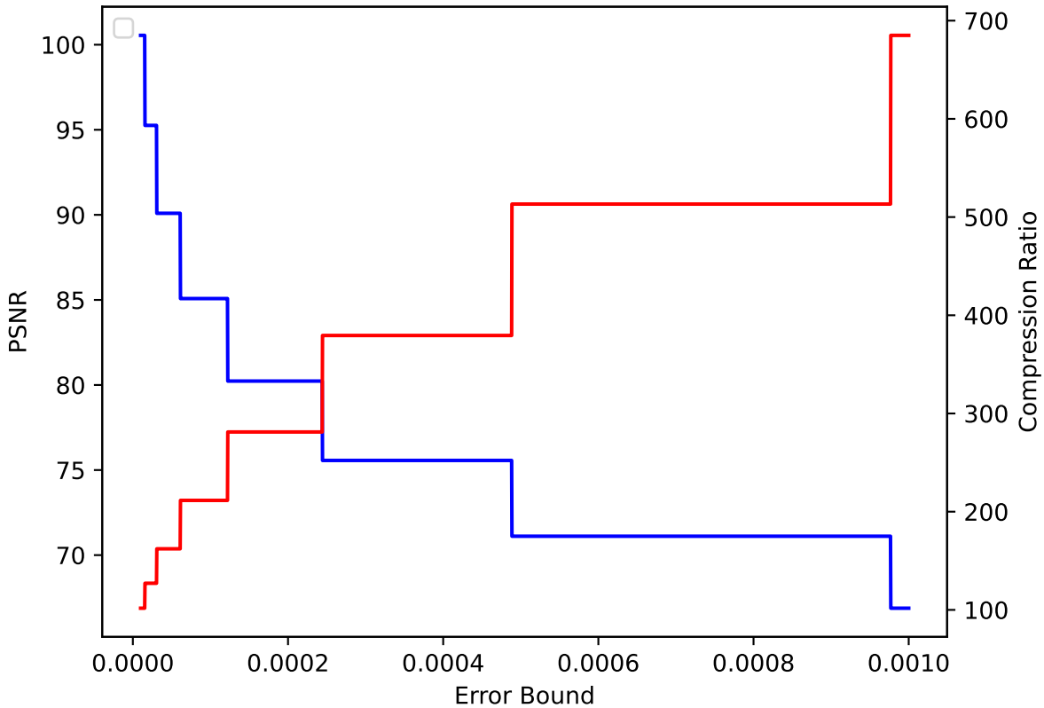
QGRAUP 46 pressio:abs
