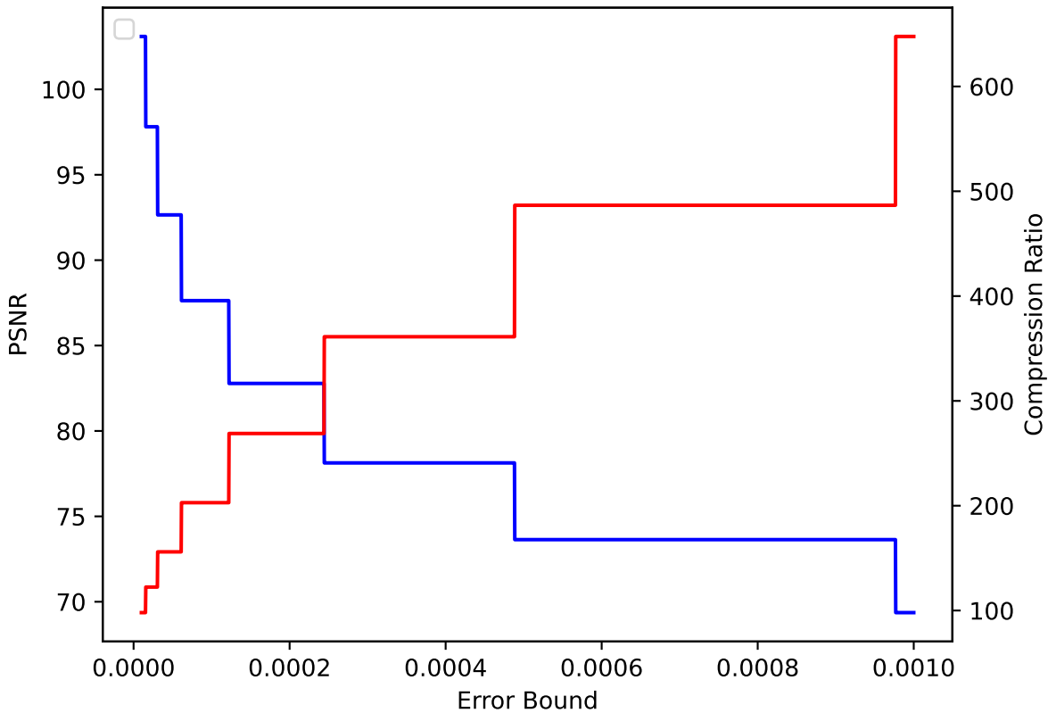
QGRAUP 45 pressio:abs
