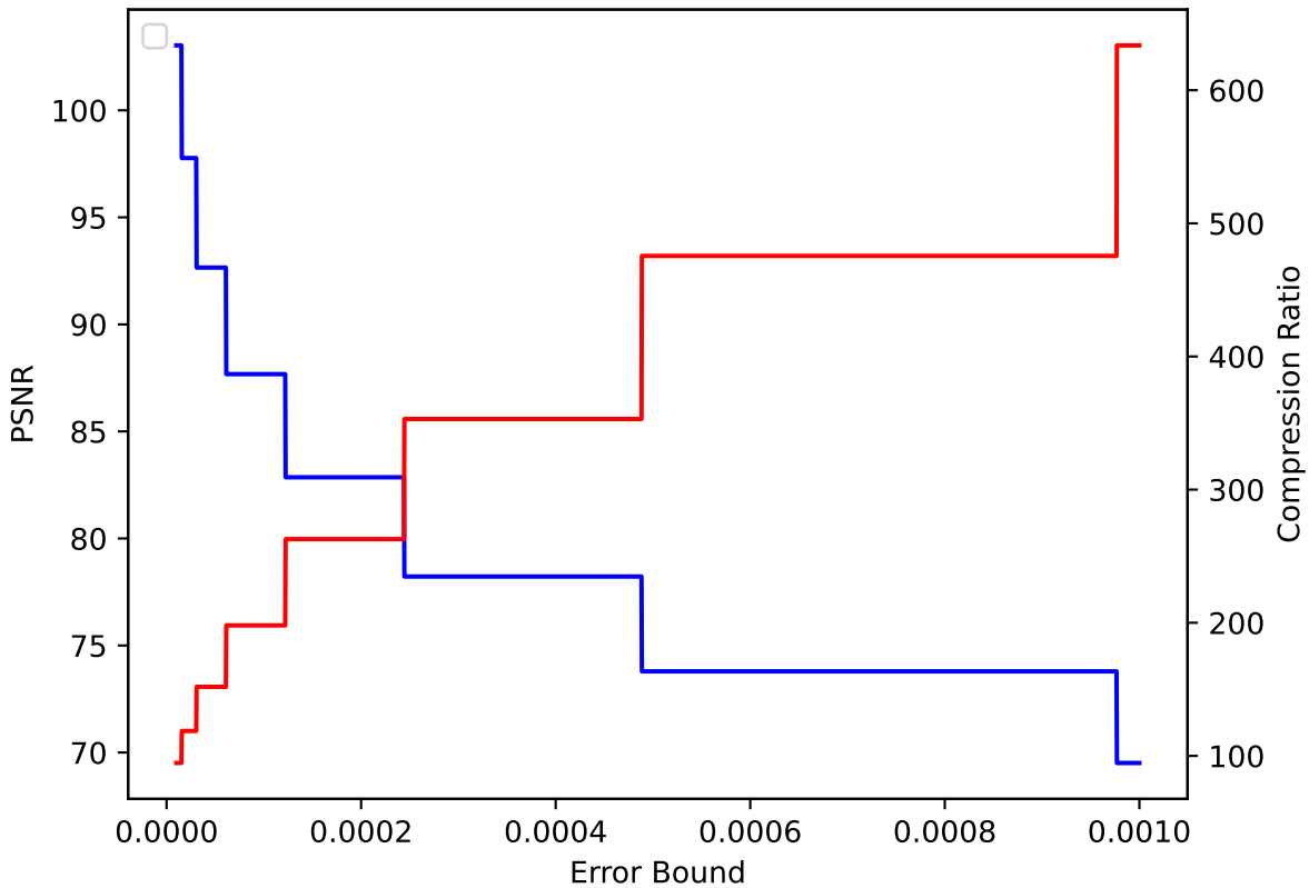
QGRAUP 43 pressio:abs
