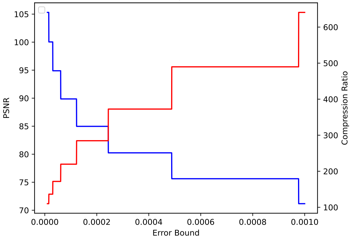
QGRAUP 29 pressio:abs
