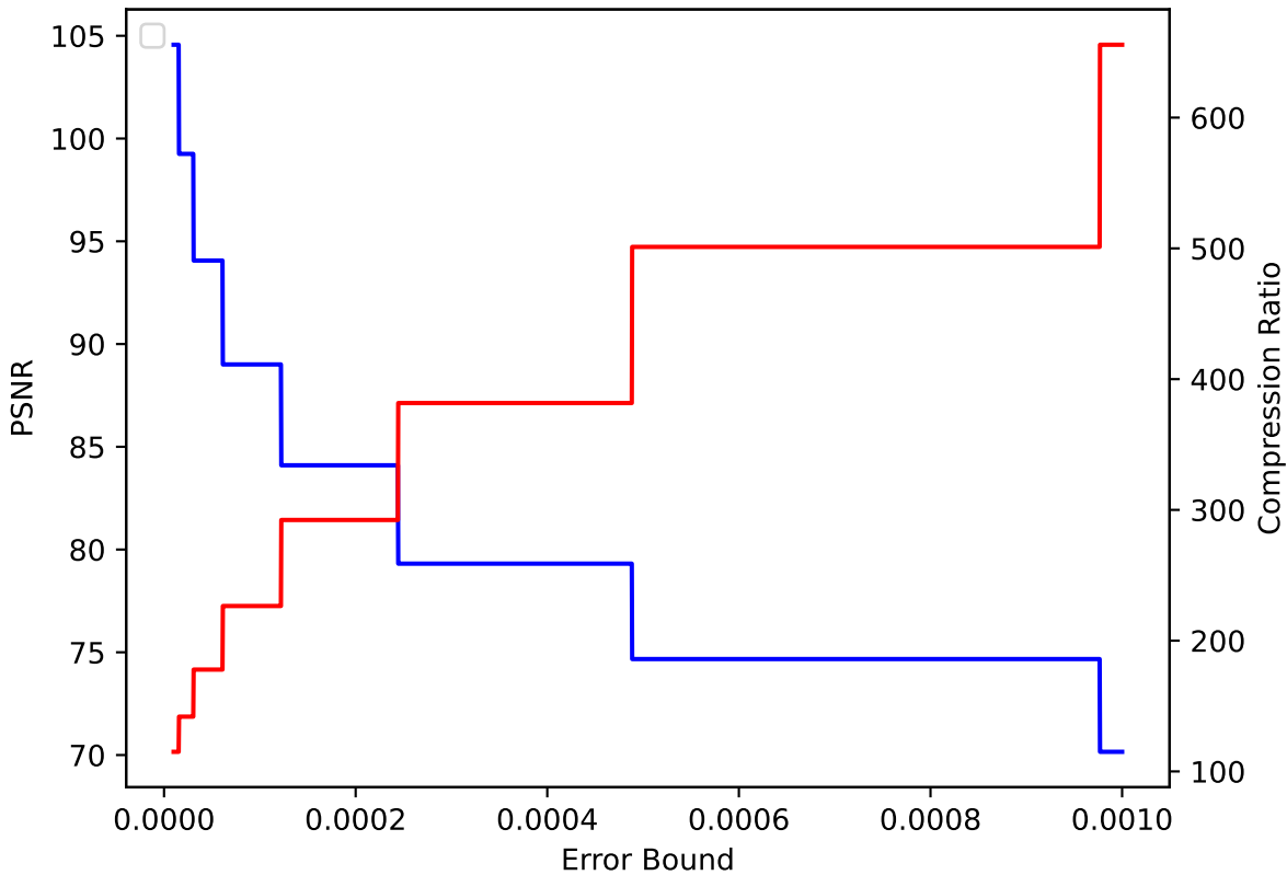
QGRAUP 19 pressio:abs
