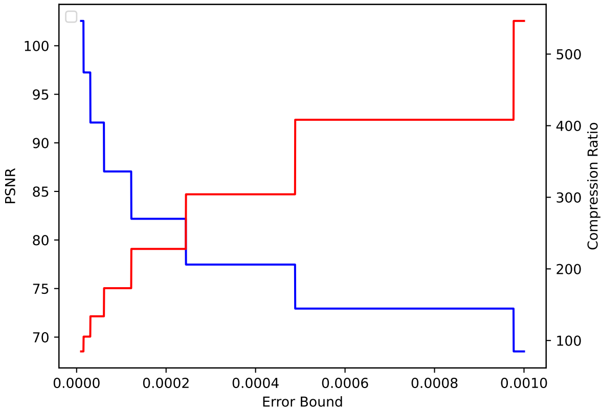
QGRAUP 36 pressio:abs
