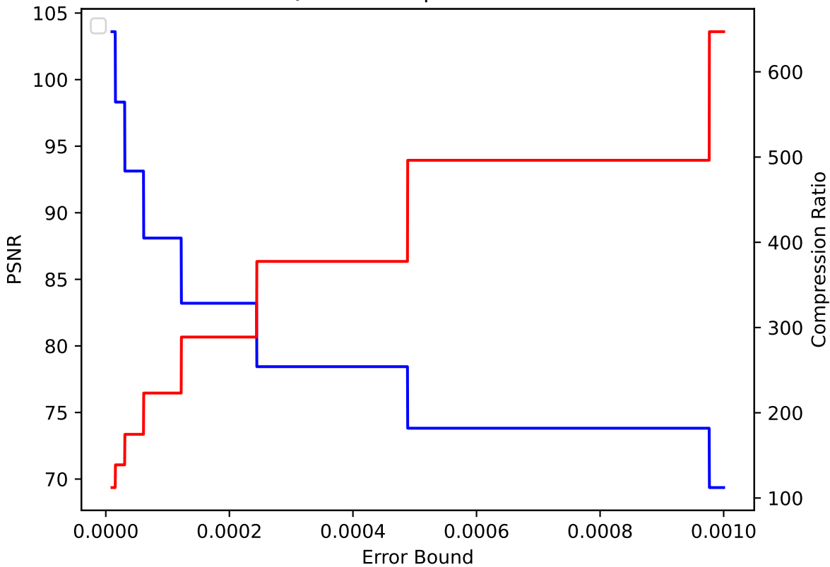
QGRAUP 27 pressio:abs
