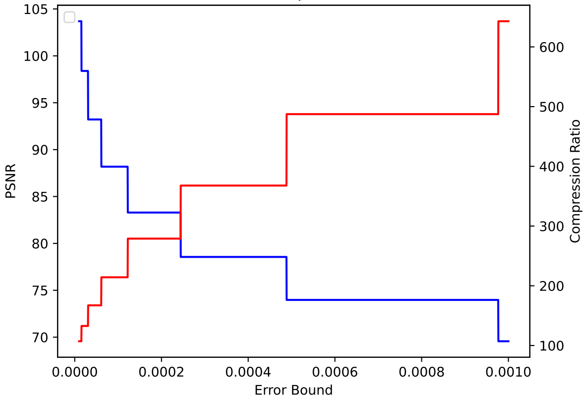
QGRAUP 15 pressio:abs
