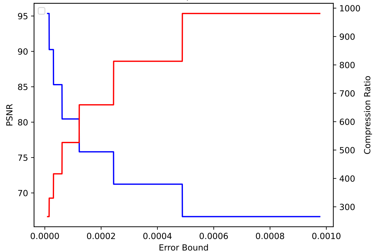
QGRAUP 01 pressio:abs
