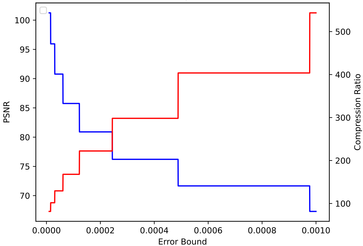
QGRAUP 39 pressio:abs
