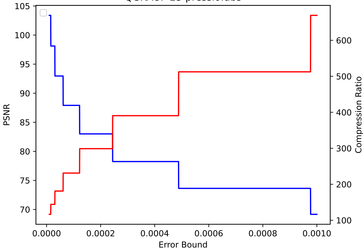
QGRAUP 25 pressio:abs
