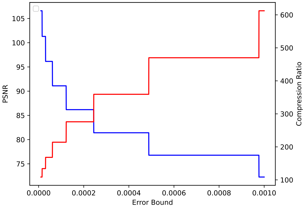
QGRAUP 22 pressio:abs
