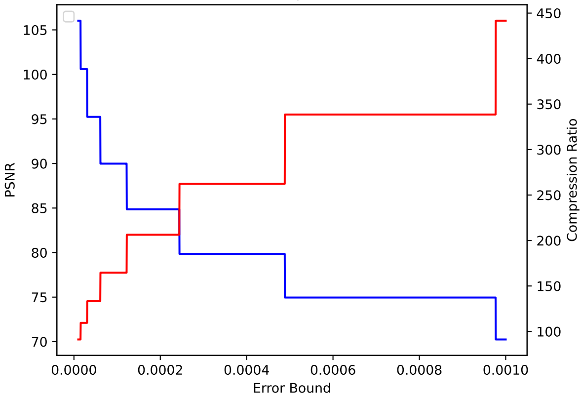
QGRAUP 11 pressio:abs
