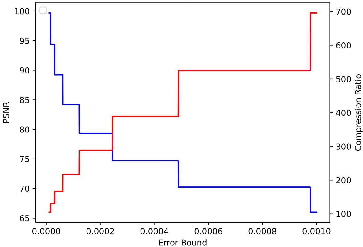
QGRAUP 47 pressio:abs
