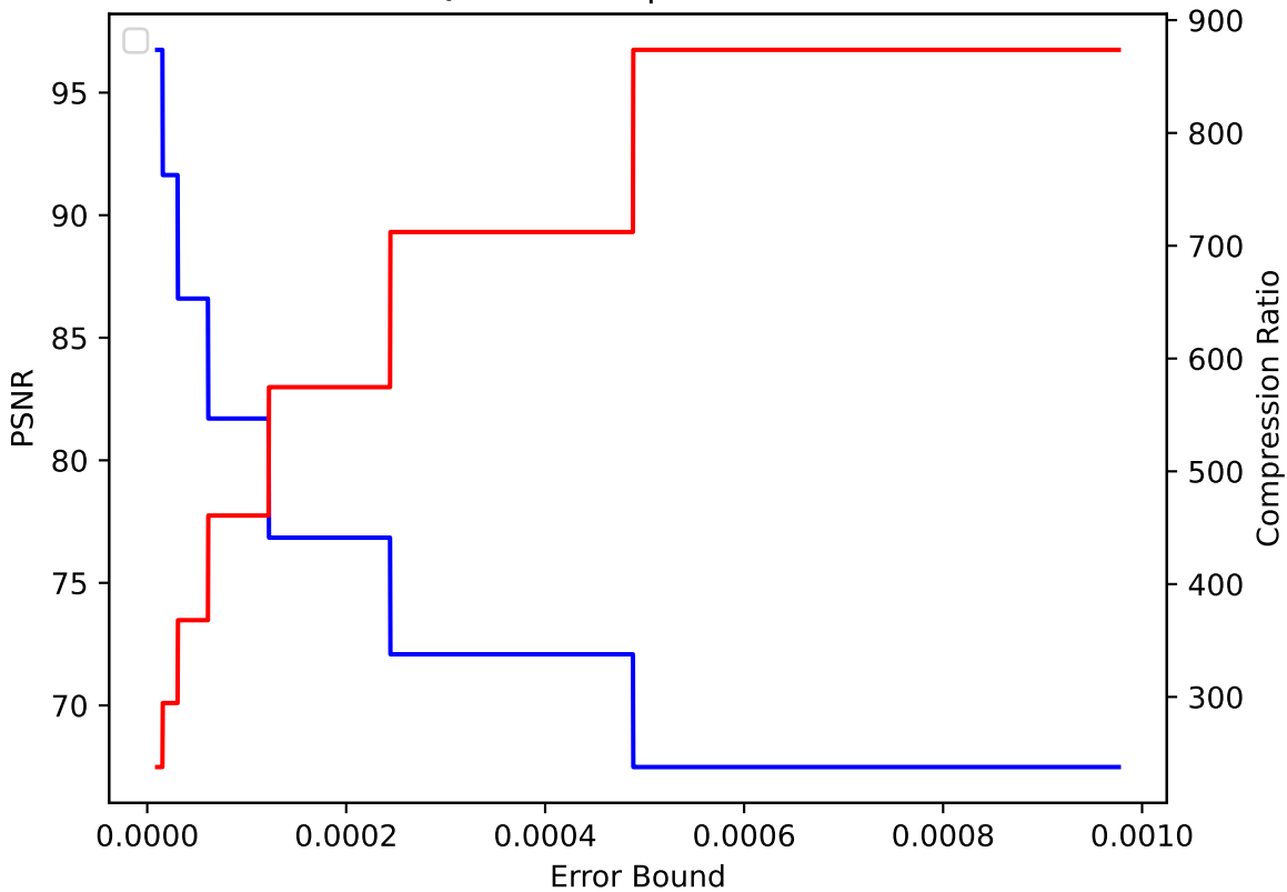
QGRAUP 02 pressio:abs
