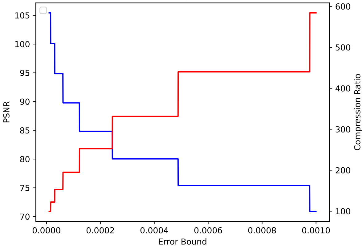
QGRAUP 14 pressio:abs
