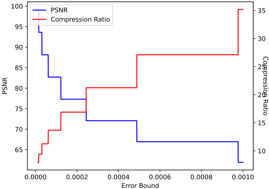
QVAPOR 21 ZFP pressio:abs
