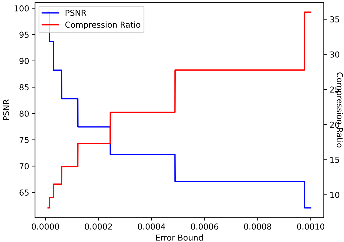
QVAPOR 16 ZFP pressio:abs
