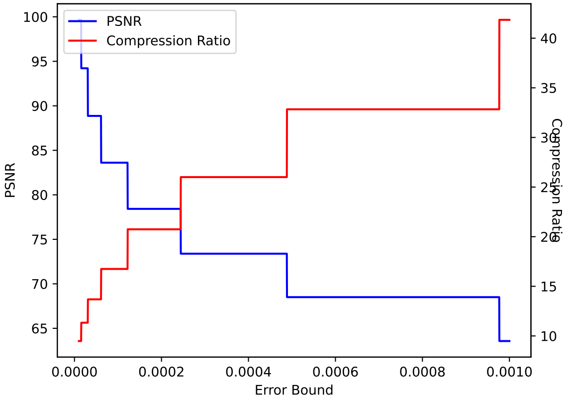
QVAPOR 07 ZFP pressio:abs
