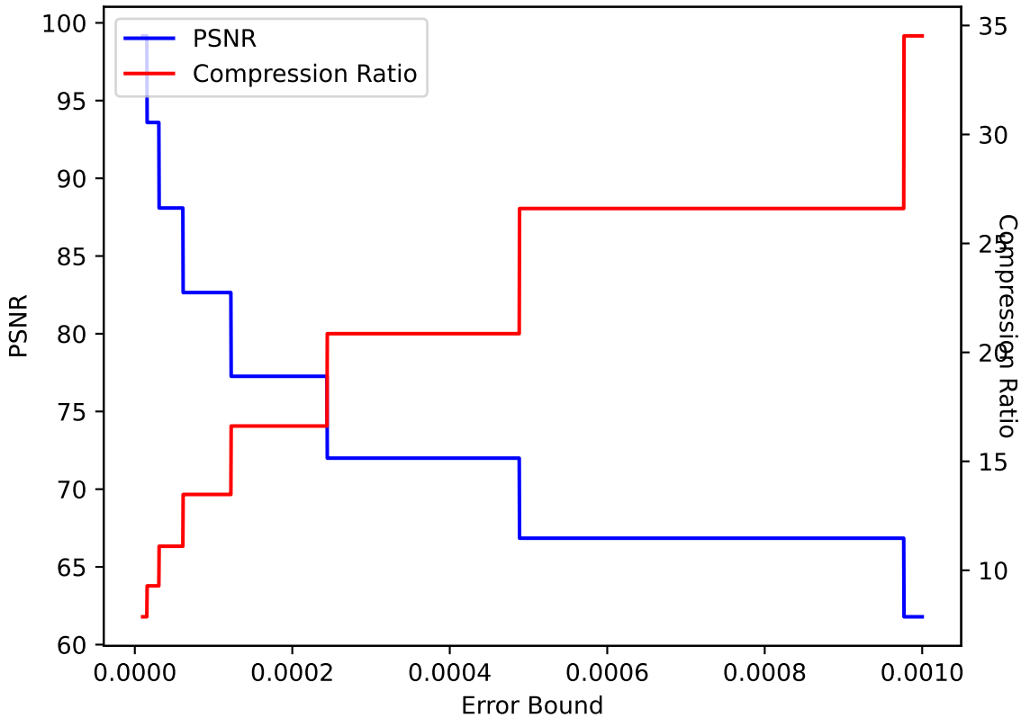
QVAPOR 23 ZFP pressio:abs
