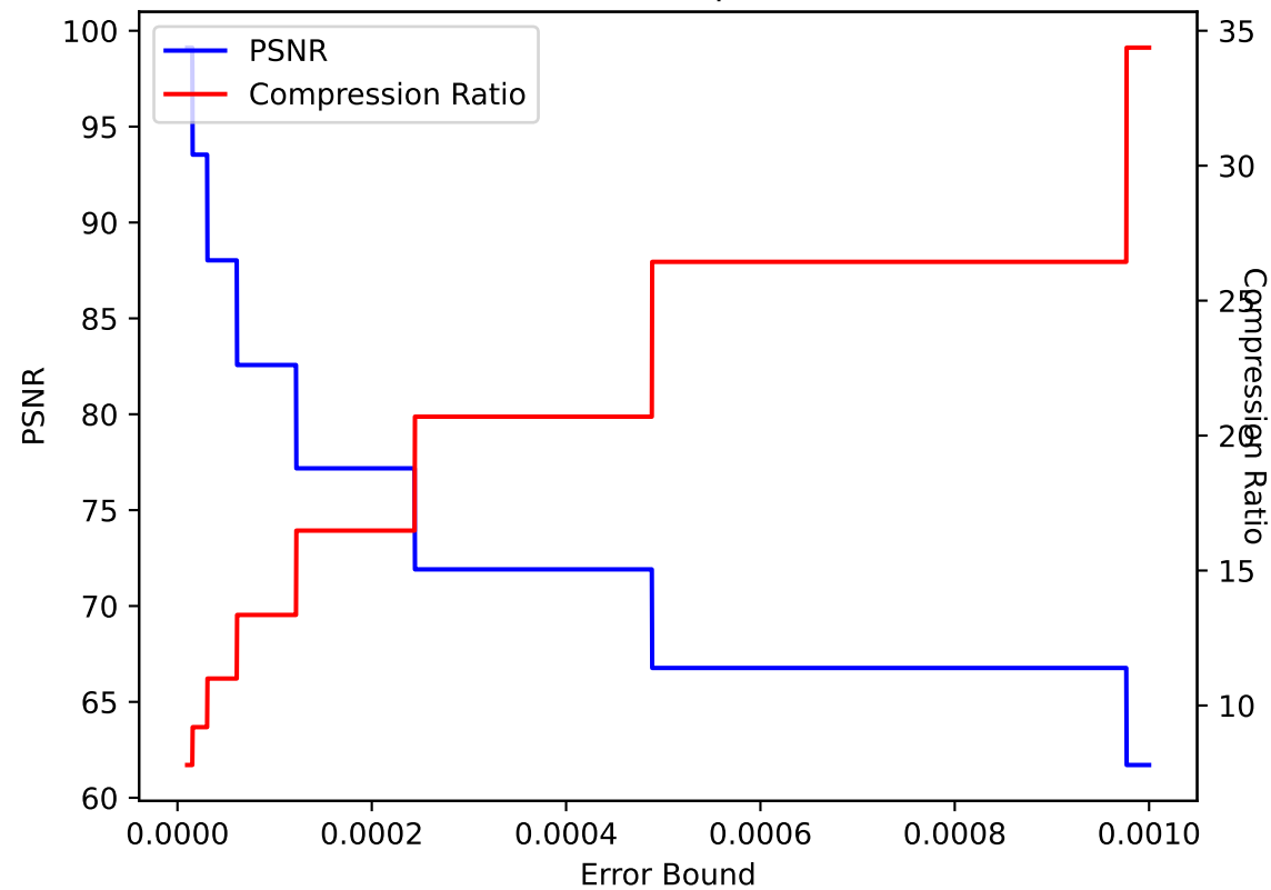
QVAPOR 25 ZFP pressio:abs
