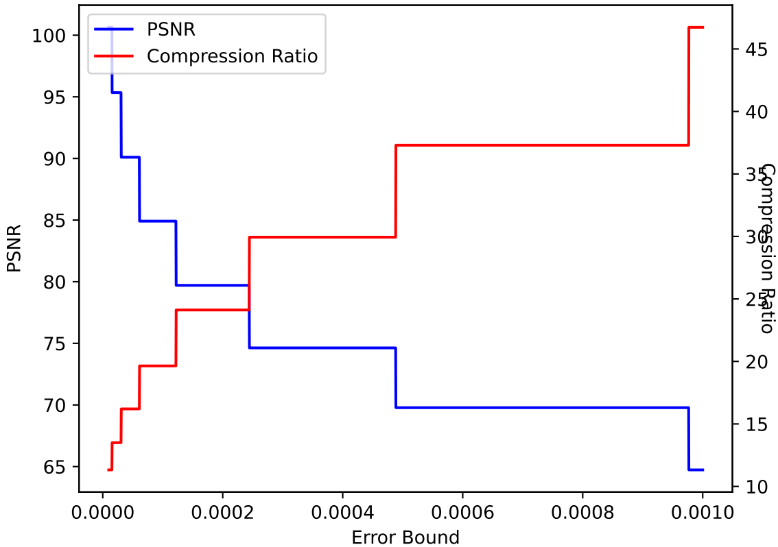
QVAPOR 02 ZFP pressio:abs
