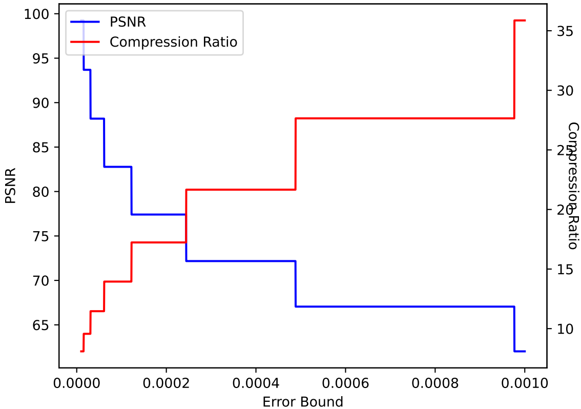
QVAPOR 17 ZFP pressio:abs
