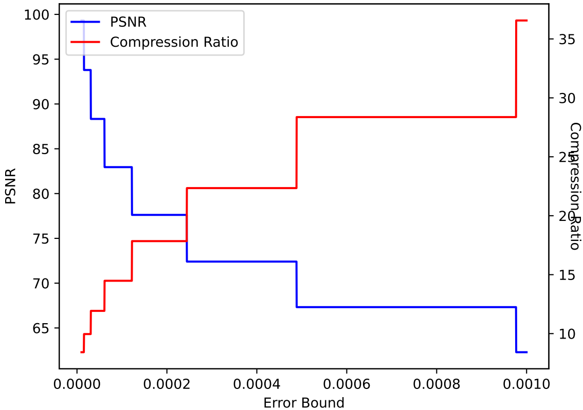
QVAPOR 11 ZFP pressio:abs
