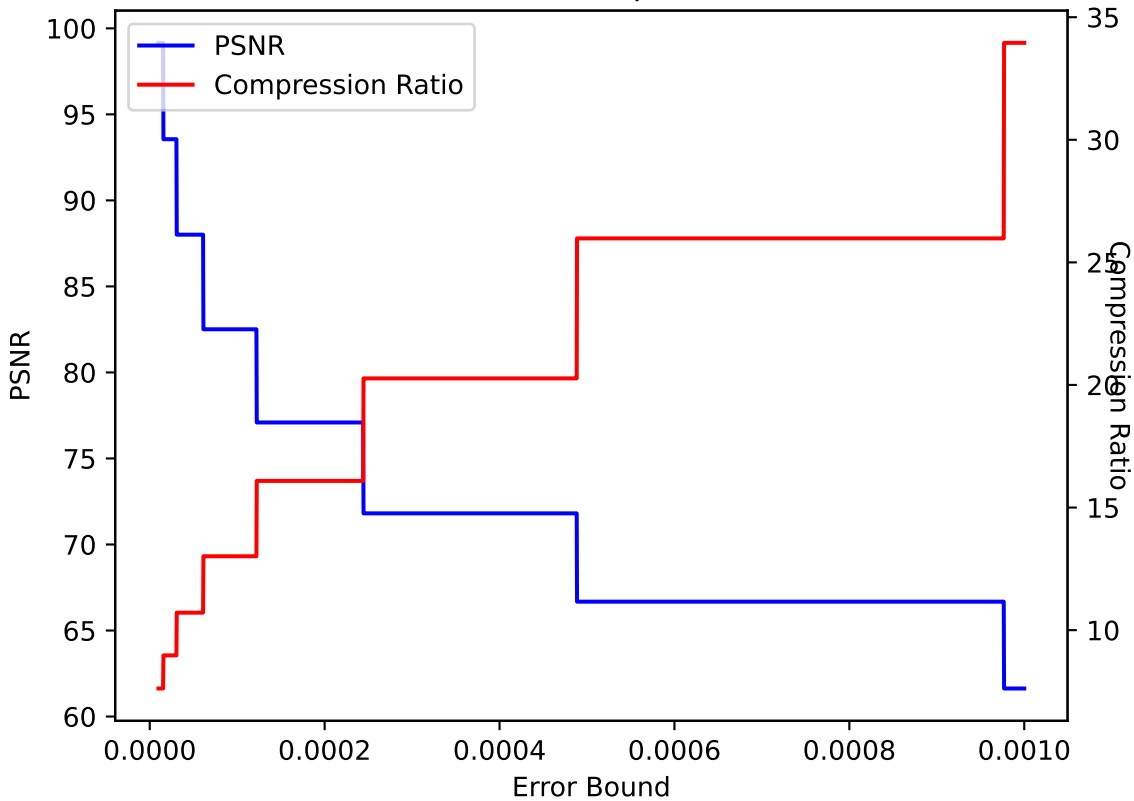
QVAPOR 37 ZFP pressio:abs
