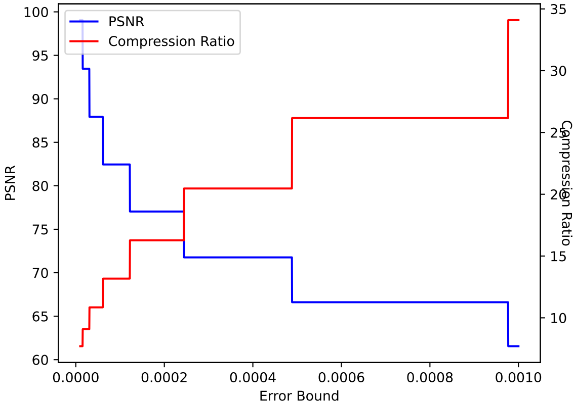
QVAPOR 31 ZFP pressio:abs
