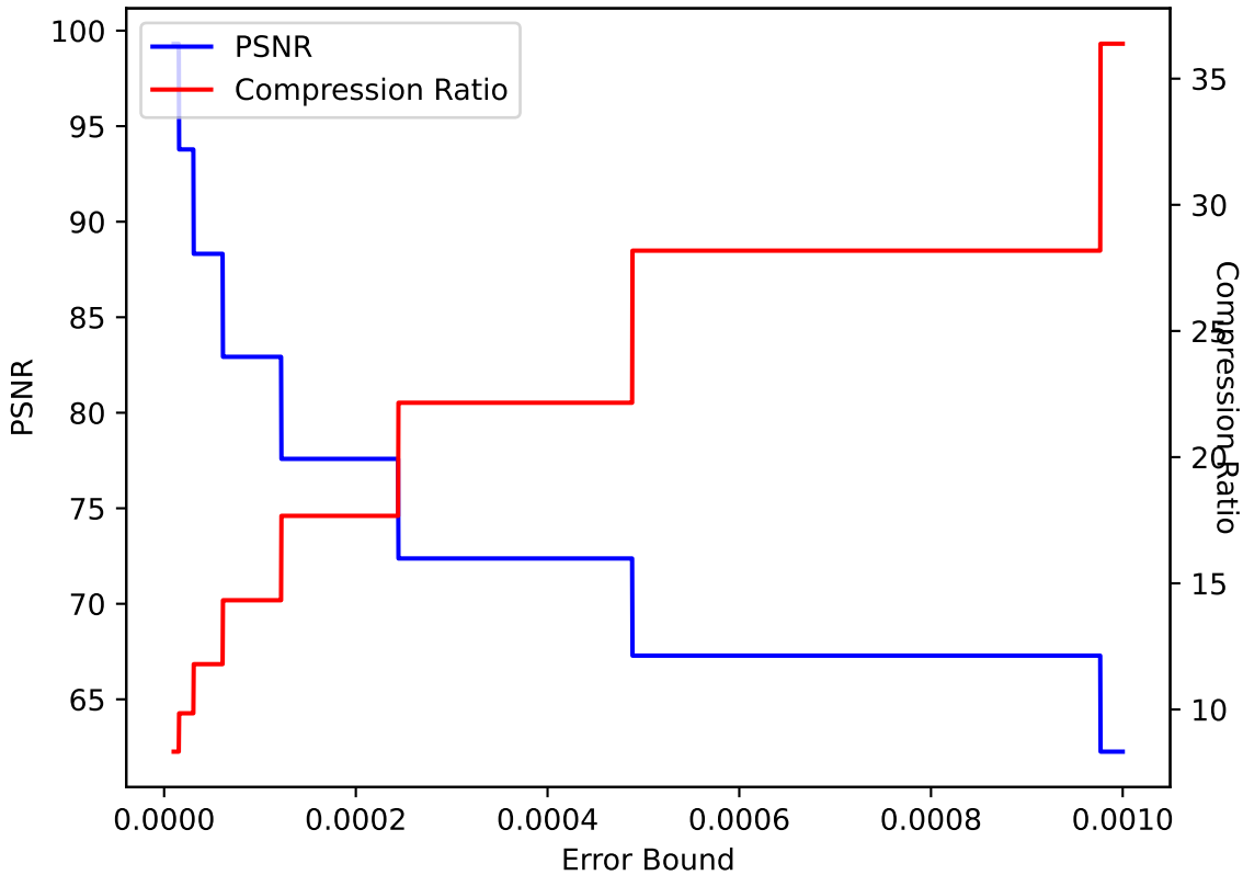
QVAPOR 12 ZFP pressio:abs
