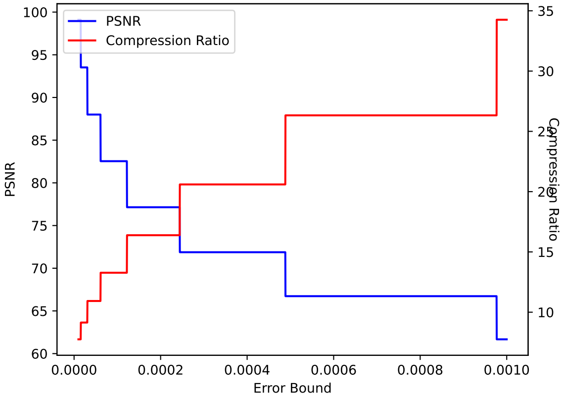
QVAPOR 27 ZFP pressio:abs
