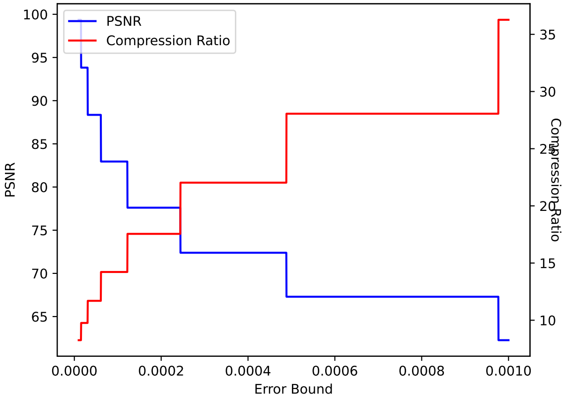
QVAPOR 13 ZFP pressio:abs
