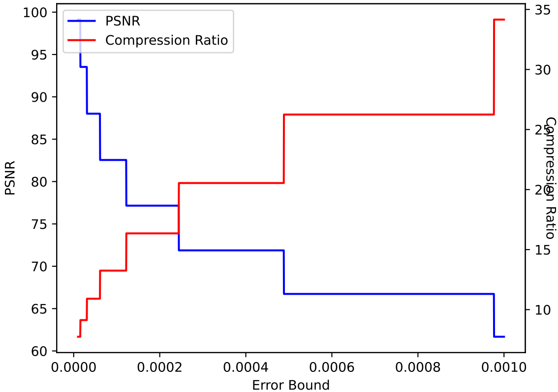
QVAPOR 28 ZFP pressio:abs
