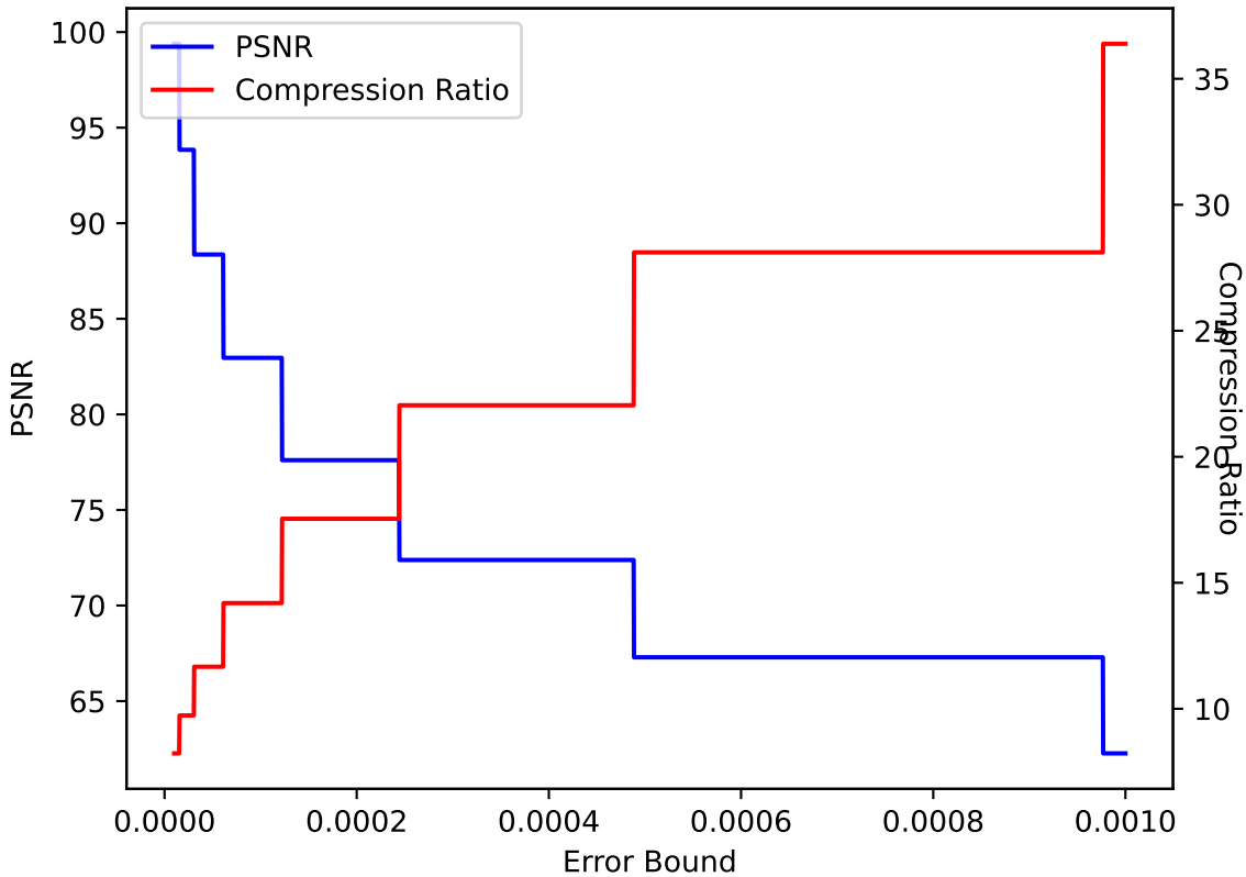
QVAPOR 14 ZFP pressio:abs
