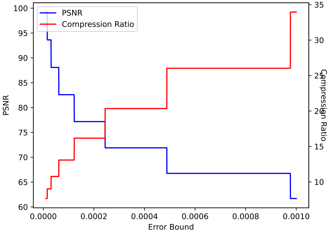
QVAPOR 33 ZFP pressio:abs
