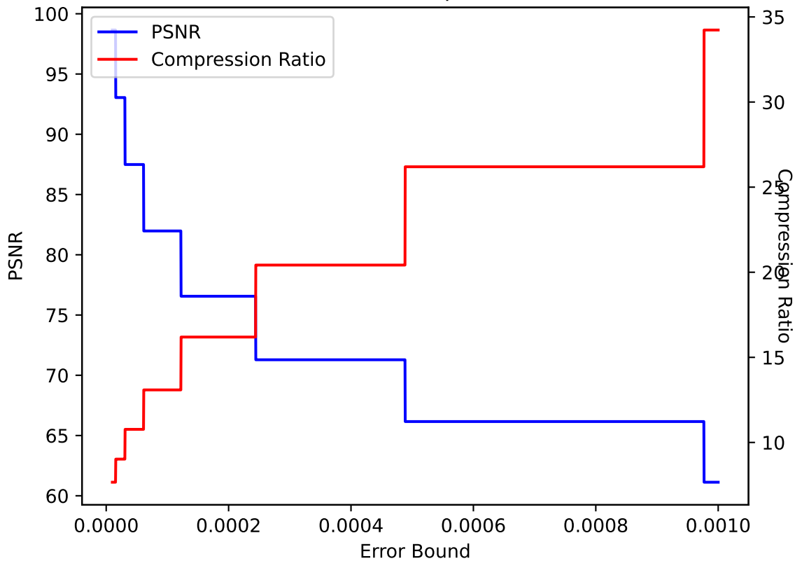
QVAPOR 44 ZFP pressio:abs
