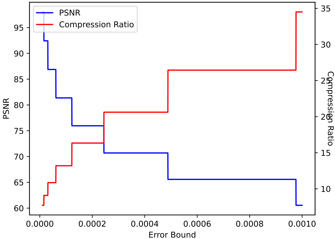
QVAPOR 47 ZFP pressio:abs
