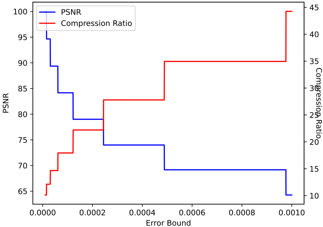
QVAPOR 05 ZFP pressio:abs
