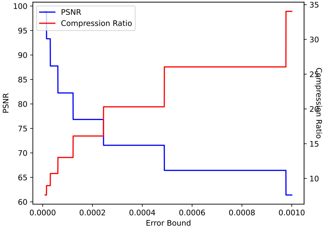
QVAPOR 41 ZFP pressio:abs
