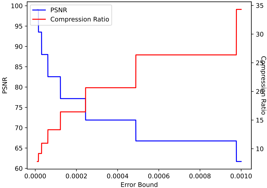
QVAPOR 26 ZFP pressio:abs
