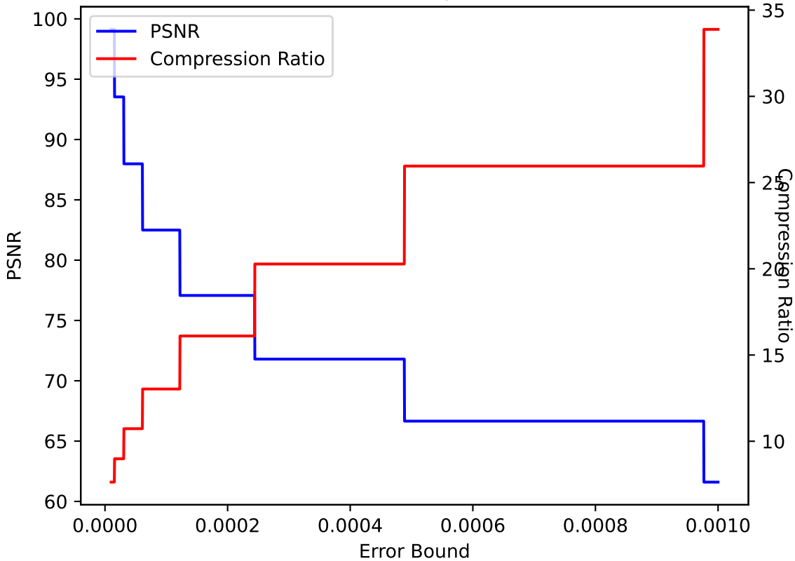
QVAPOR 34 ZFP pressio:abs
