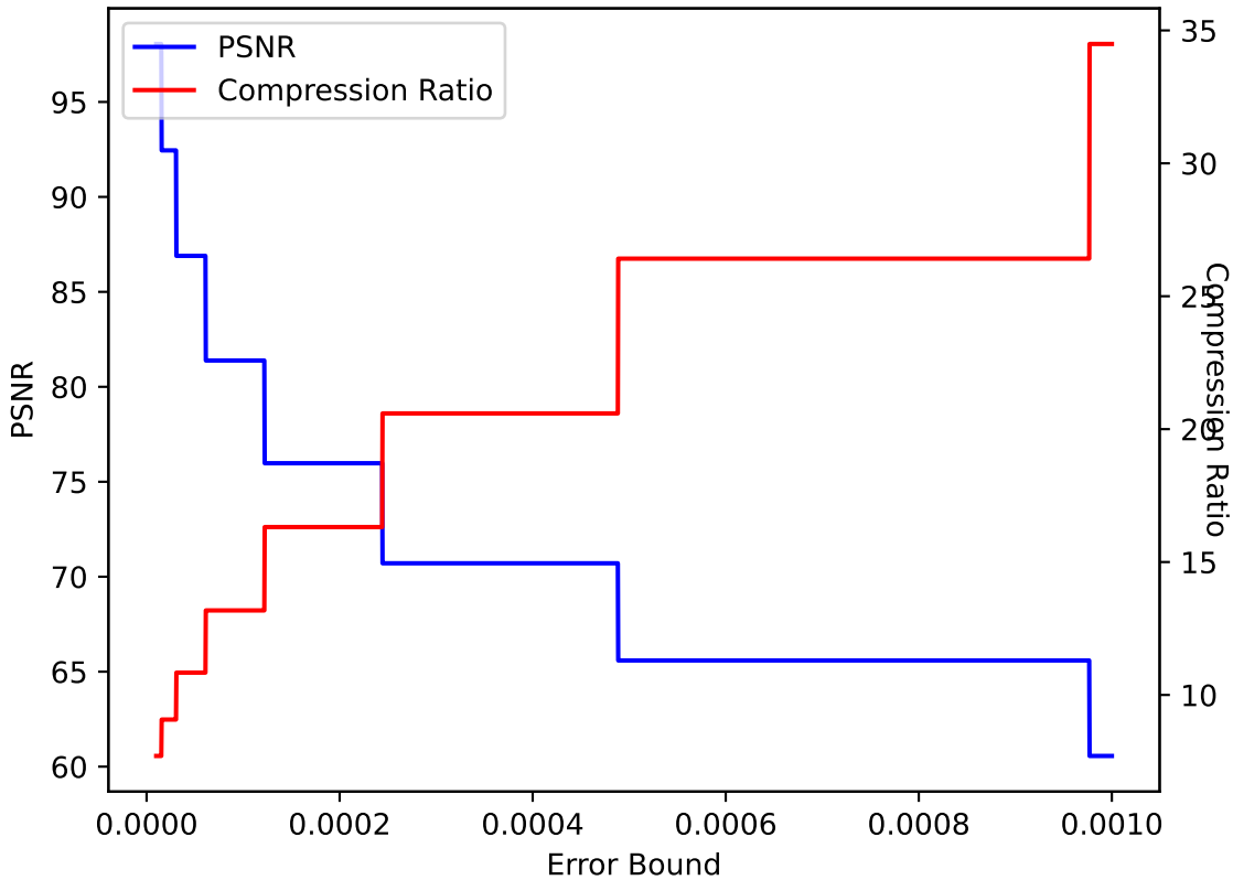
QVAPOR 46 ZFP pressio:abs
