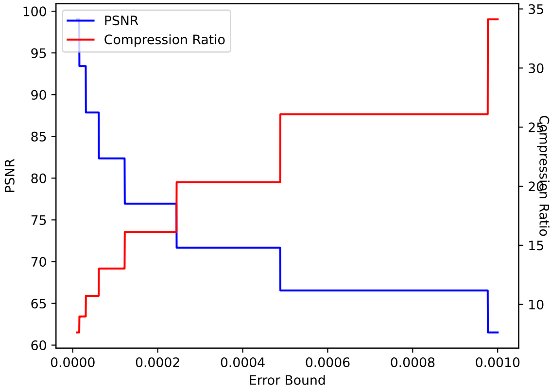
QVAPOR 40 ZFP pressio:abs
