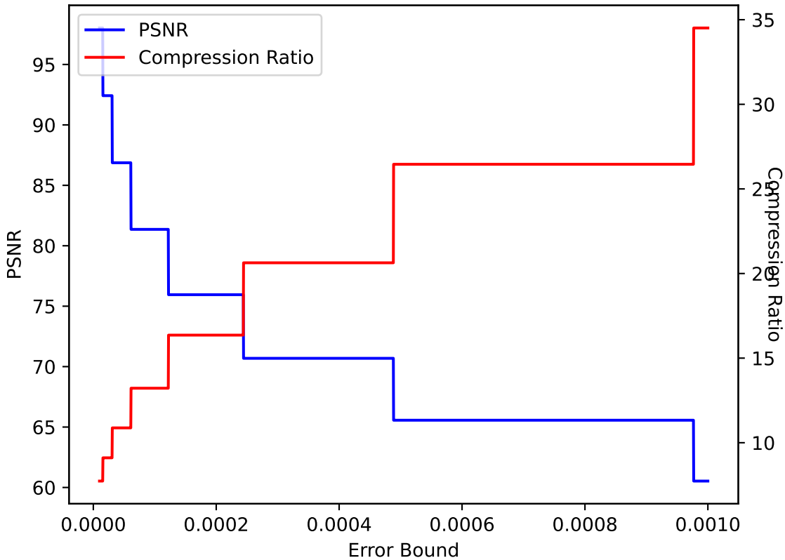
QVAPOR 48 ZFP pressio:abs
