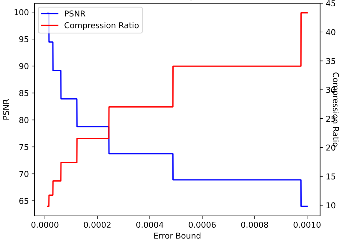
QVAPOR 06 ZFP pressio:abs
