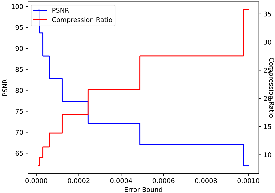
QVAPOR 19 ZFP pressio:abs
