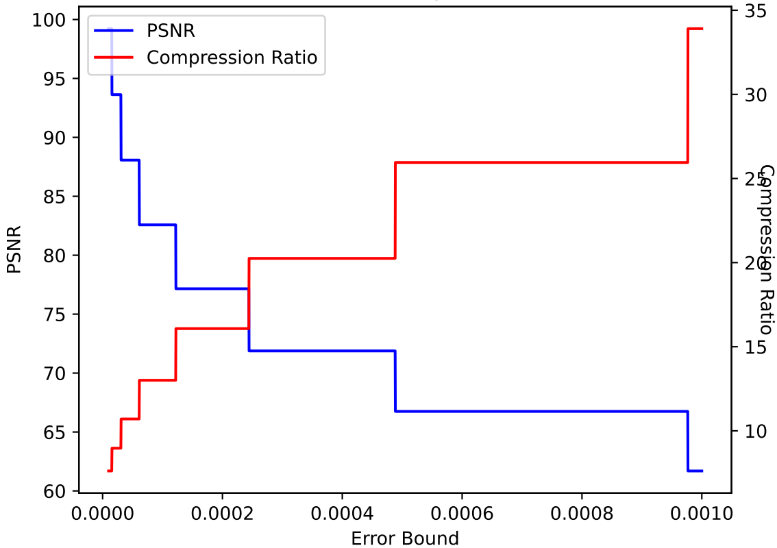
QVAPOR 36 ZFP pressio:abs
