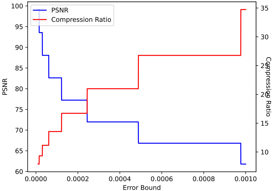
QVAPOR 22 ZFP pressio:abs
