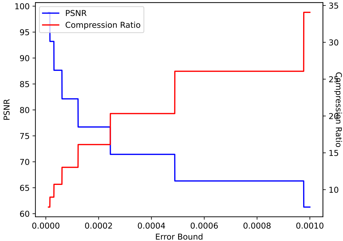
QVAPOR 43 ZFP pressio:abs
