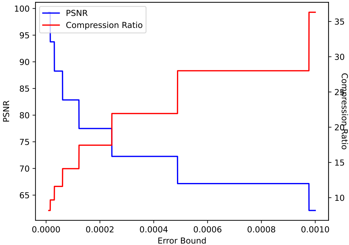
QVAPOR 15 ZFP pressio:abs
