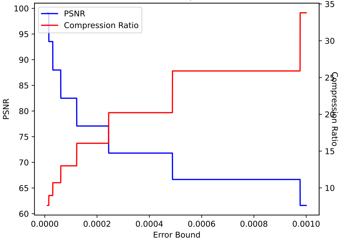
QVAPOR 35 ZFP pressio:abs
