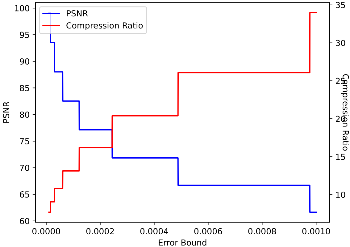
QVAPOR 32 ZFP pressio:abs
