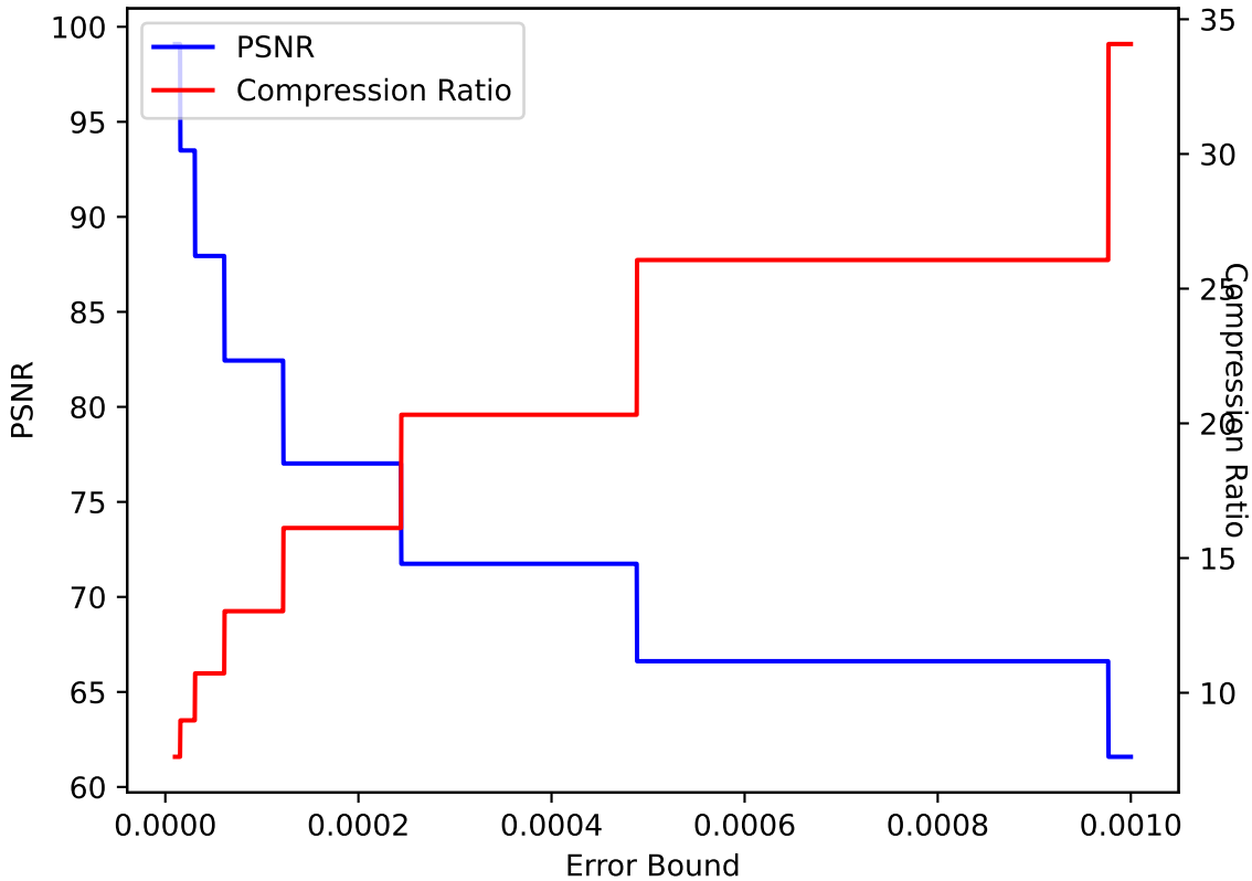
QVAPOR 39 ZFP pressio:abs
