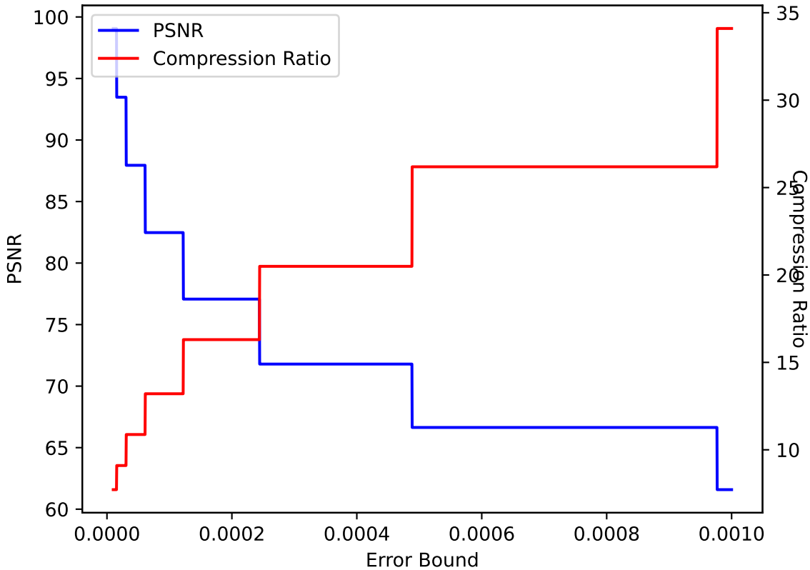
QVAPOR 30 ZFP pressio:abs
