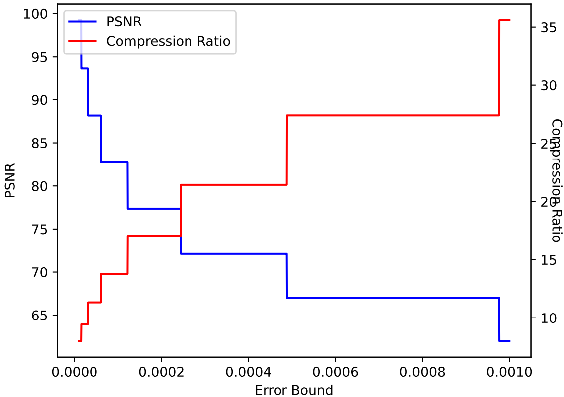
QVAPOR 20 ZFP pressio:abs
