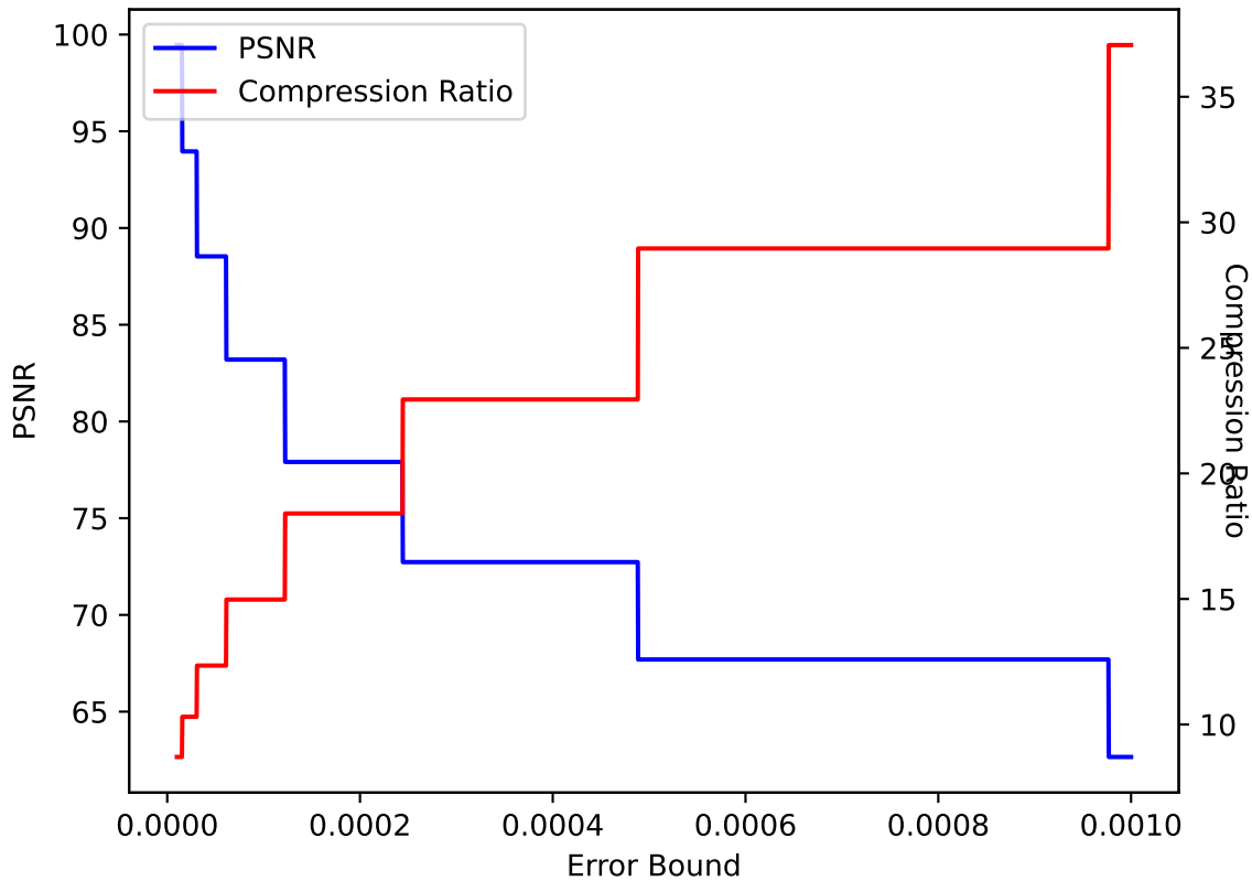
QVAPOR 09 ZFP pressio:abs
