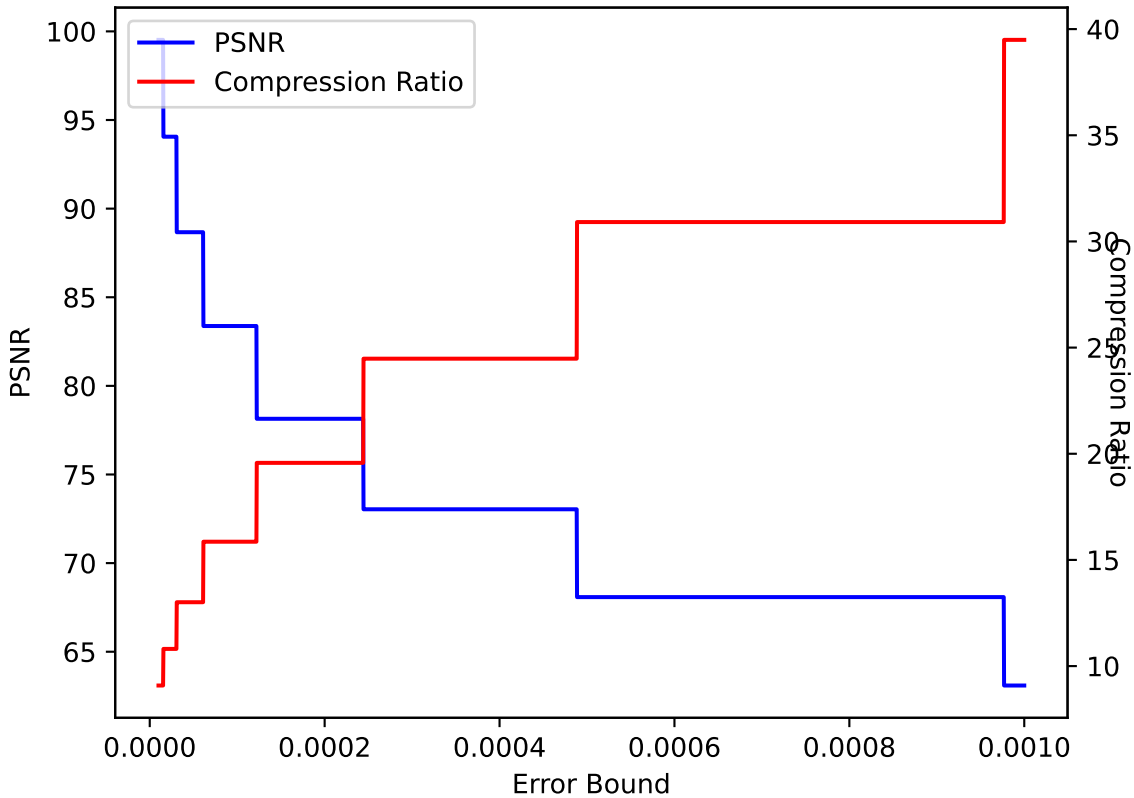
QVAPOR 08 ZFP pressio:abs
