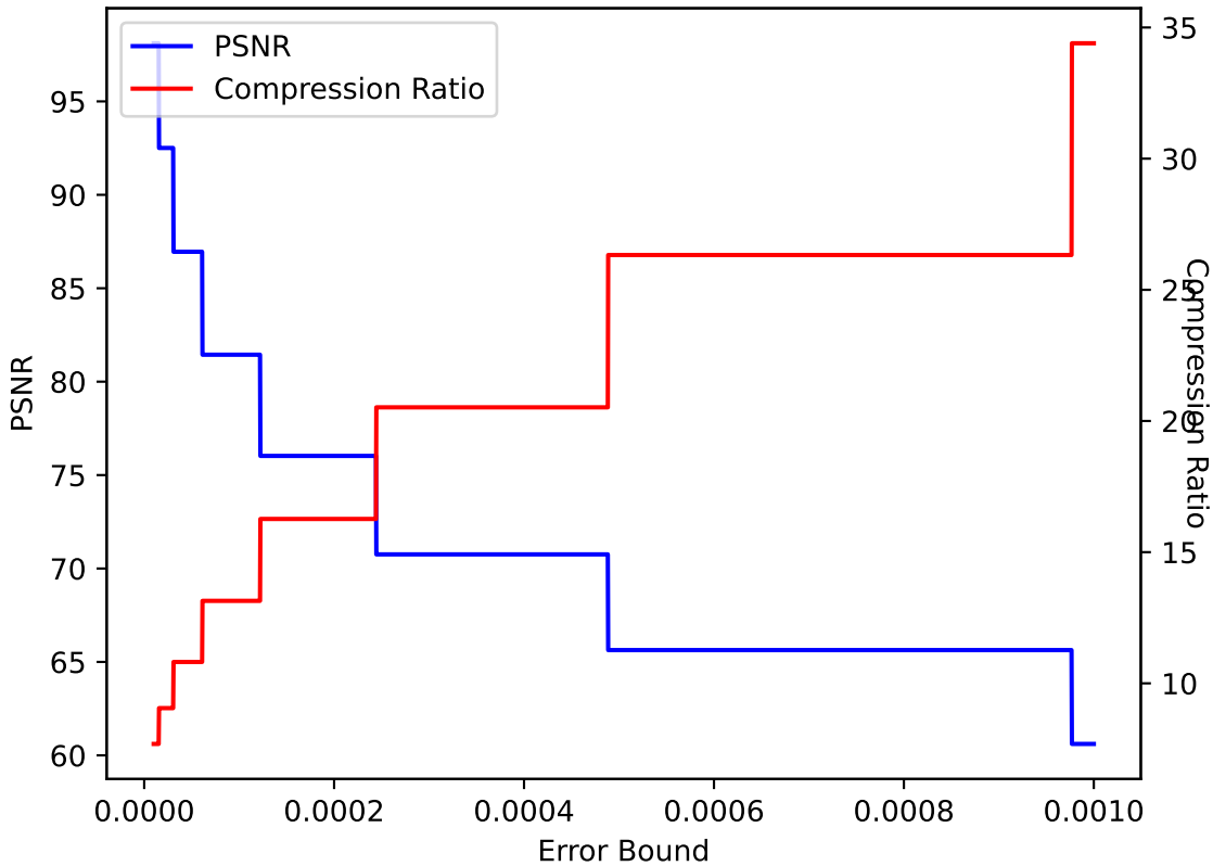
QVAPOR 45 ZFP pressio:abs
