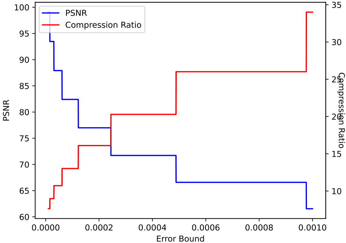
QVAPOR 38 ZFP pressio:abs
