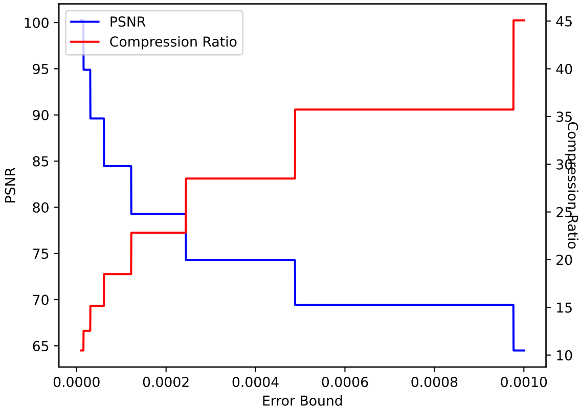
QVAPOR 04 ZFP pressio:abs
