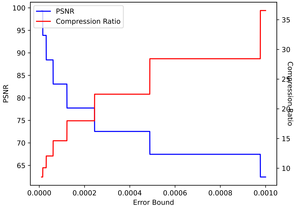
QVAPOR 10 ZFP pressio:abs
