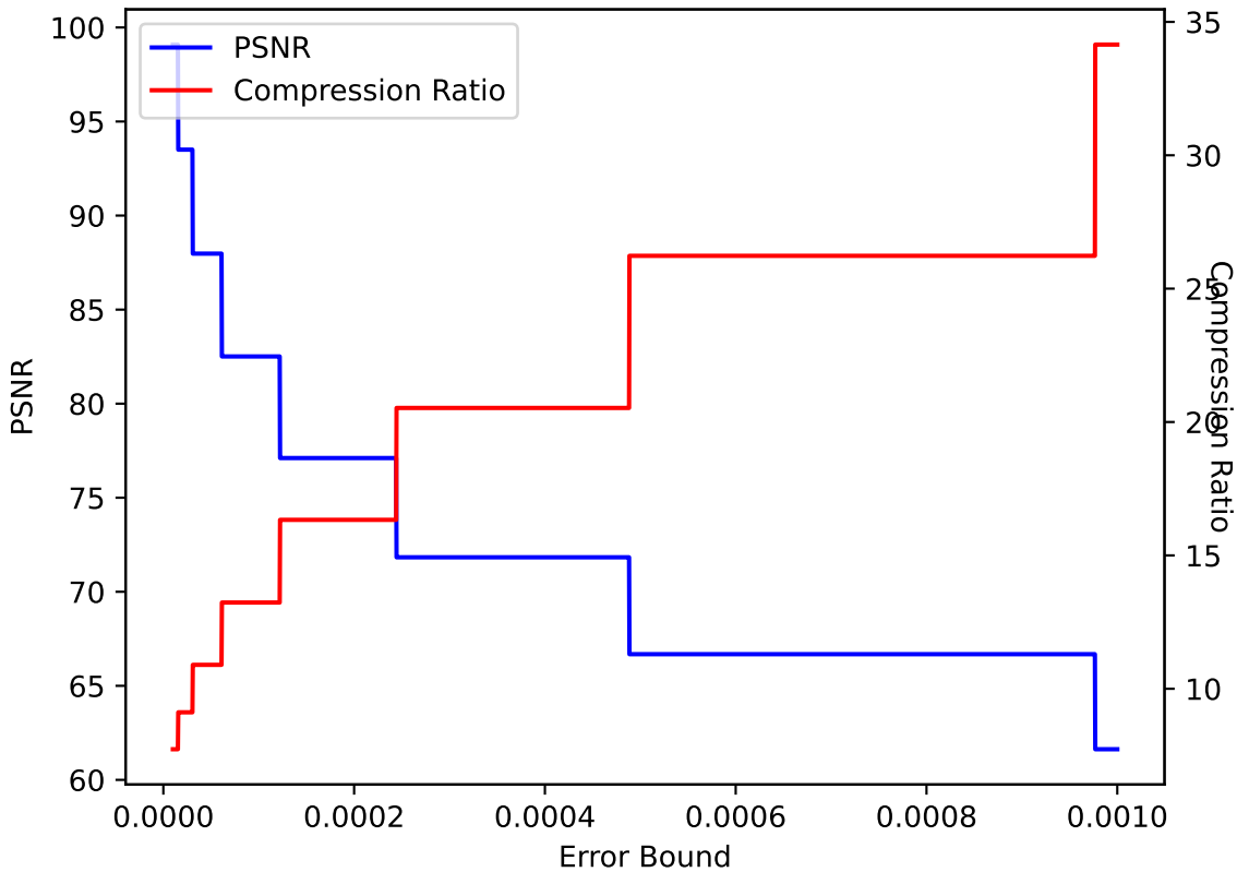
QVAPOR 29 ZFP pressio:abs
