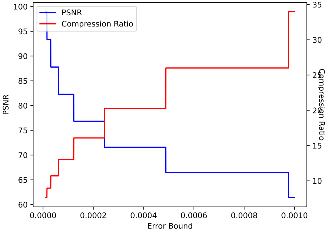
QVAPOR 42 ZFP pressio:abs
