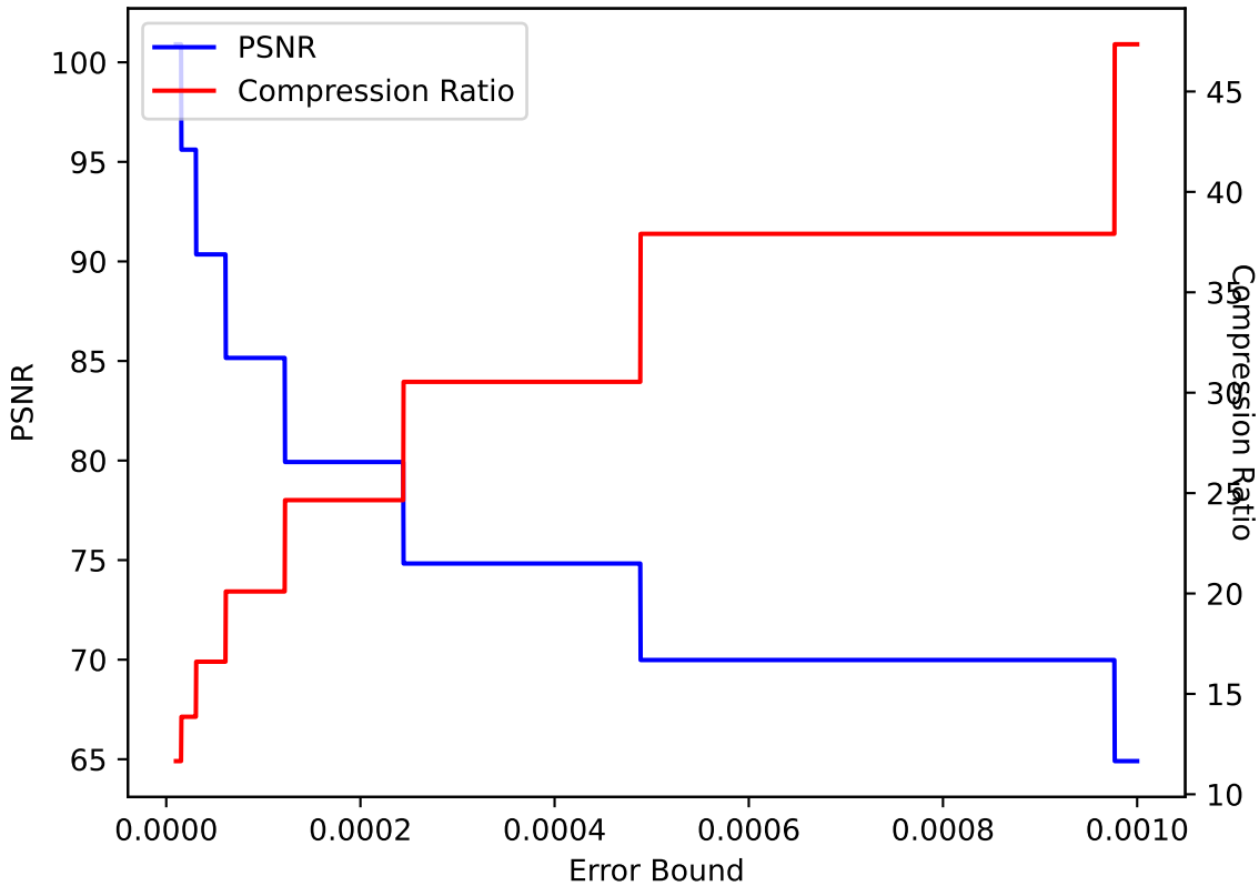
QVAPOR 01 ZFP pressio:abs
