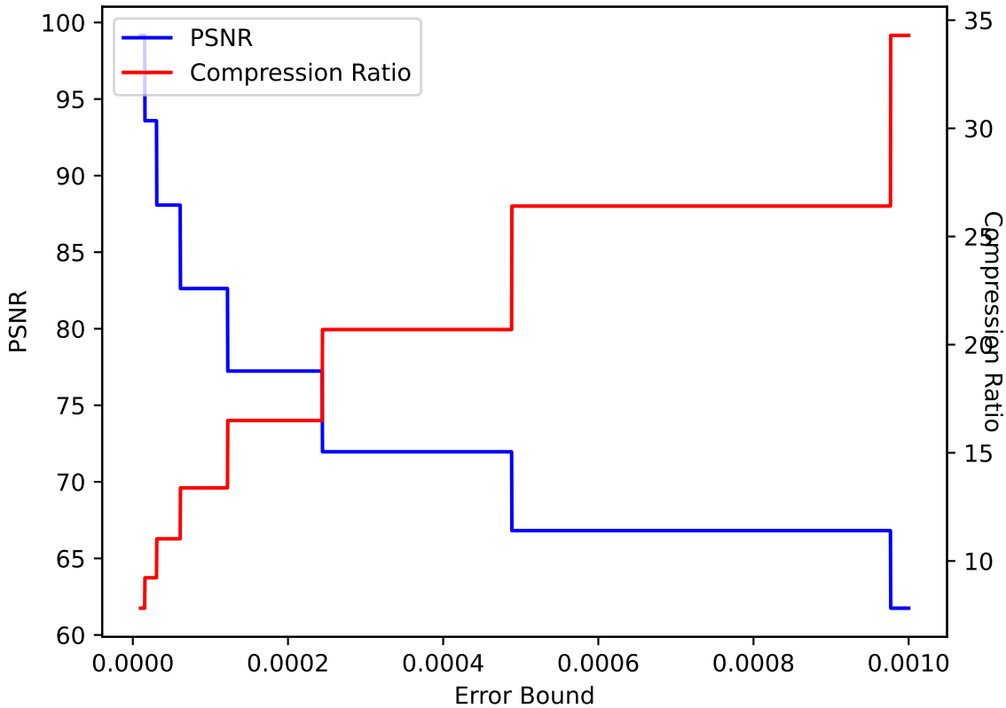
QVAPOR 24 ZFP pressio:abs
