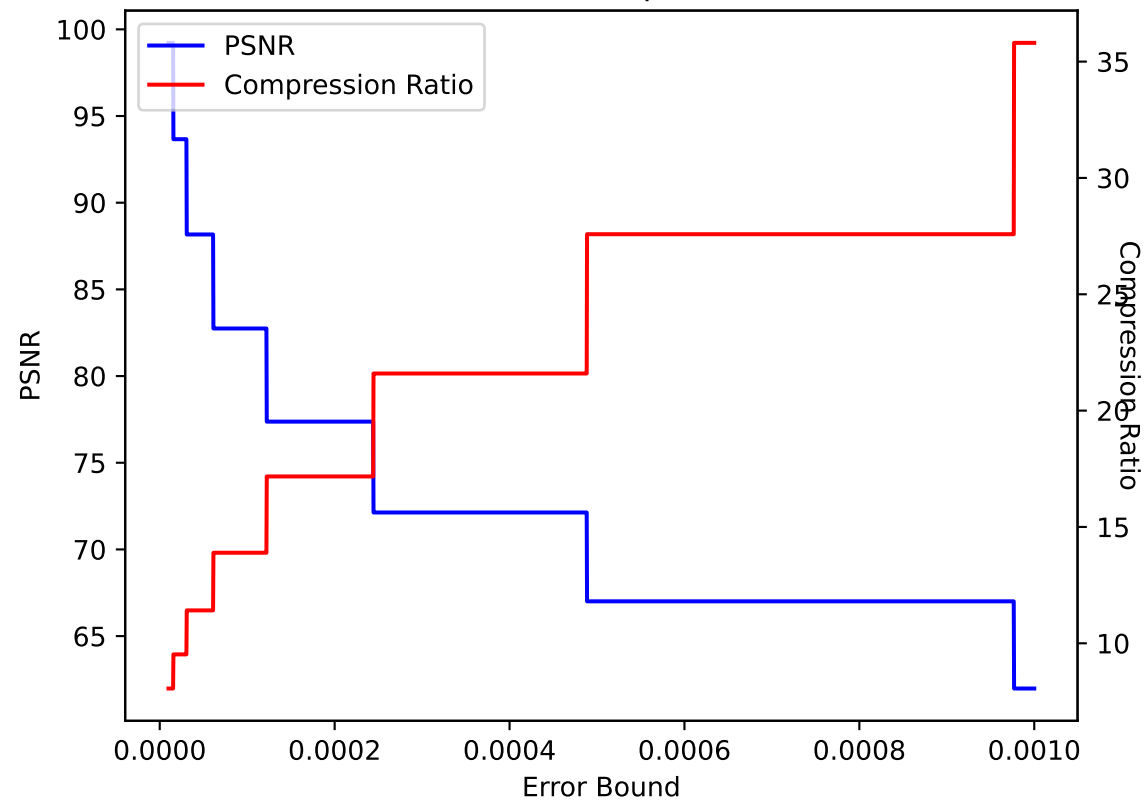
QVAPOR 18 ZFP pressio:abs
