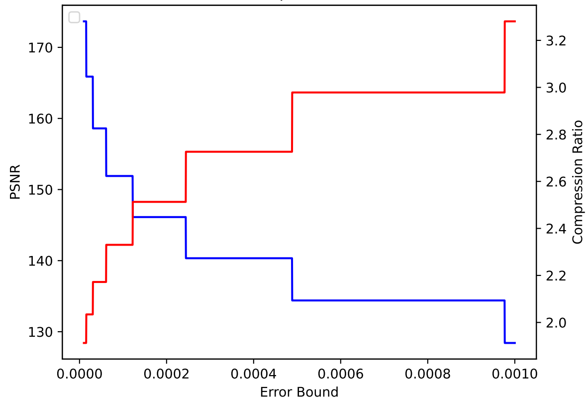
TC 10 pressio:abs
