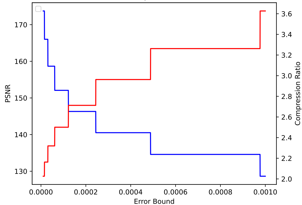
TC 06 pressio:abs
