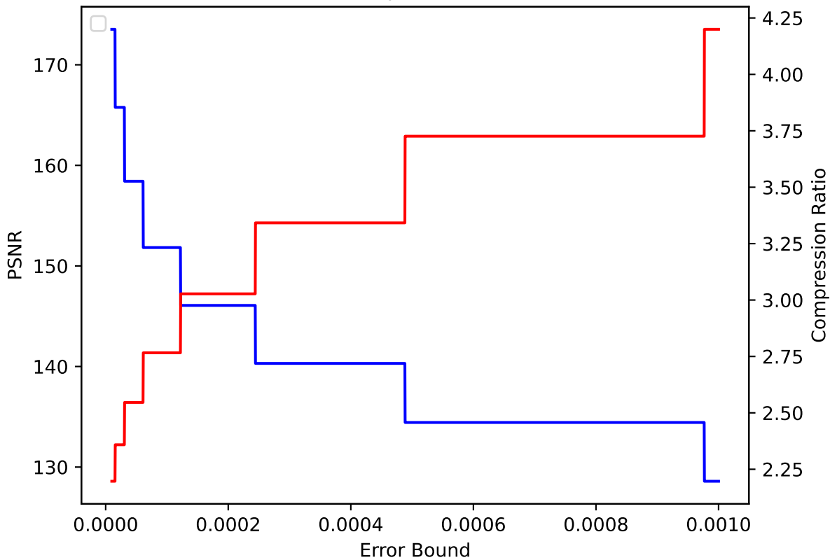
TC 02 pressio:abs
