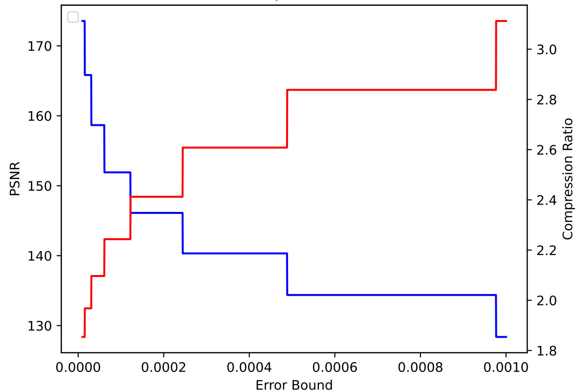
TC 40 pressio:abs
