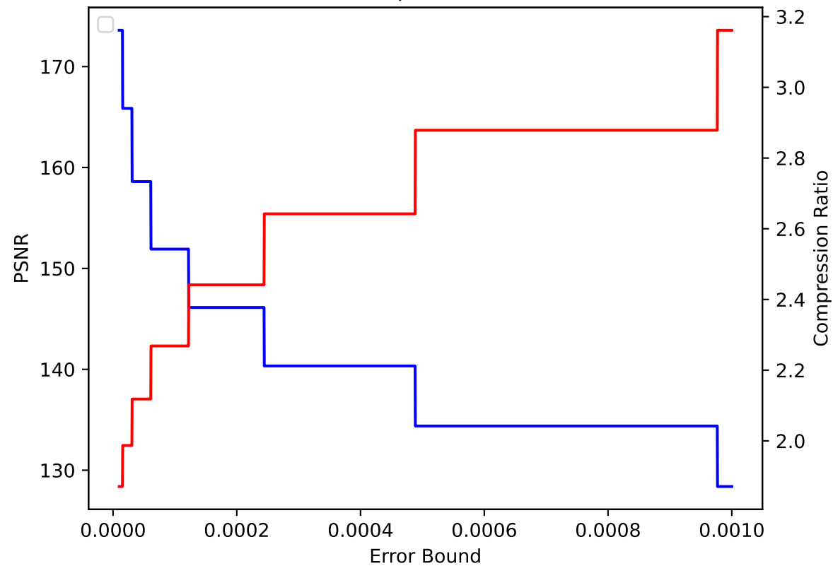
TC 18 pressio:abs
