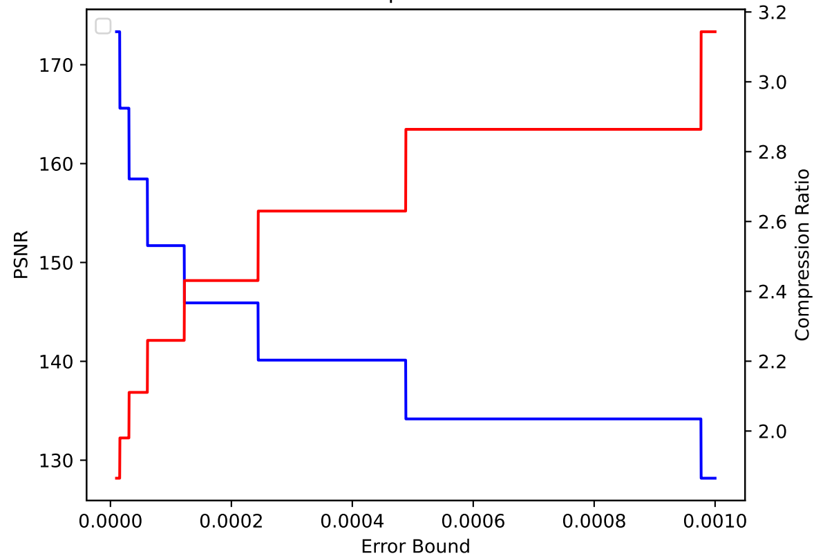
TC 47 pressio:abs
