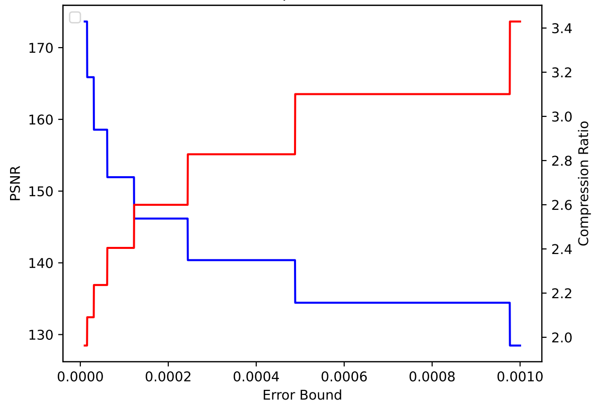
TC 08 pressio:abs
