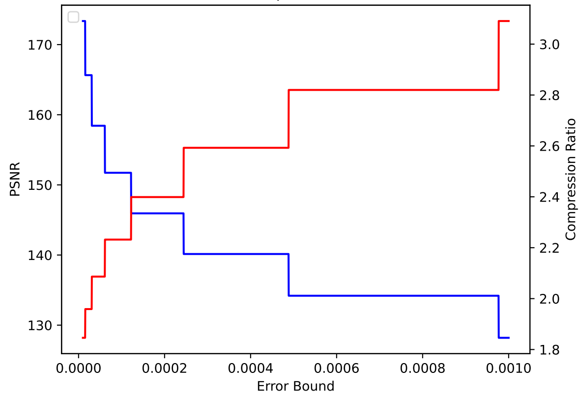
TC 28 pressio:abs
