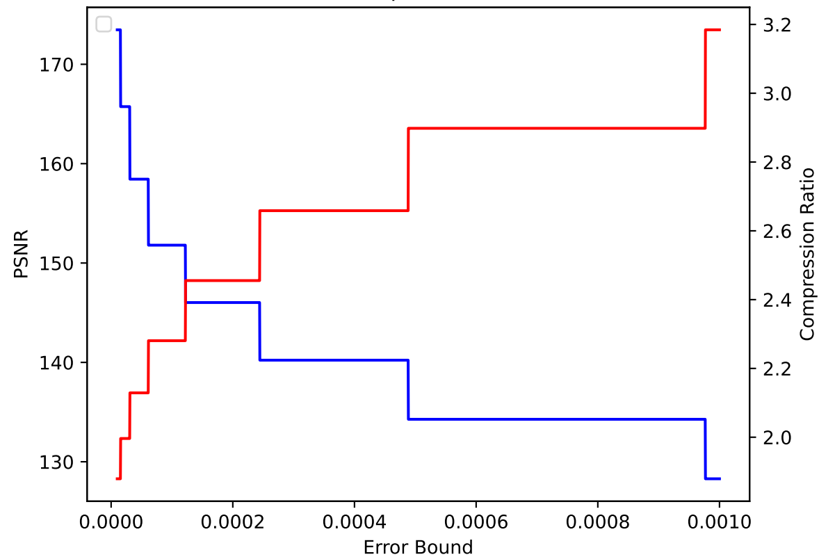
TC 13 pressio:abs
