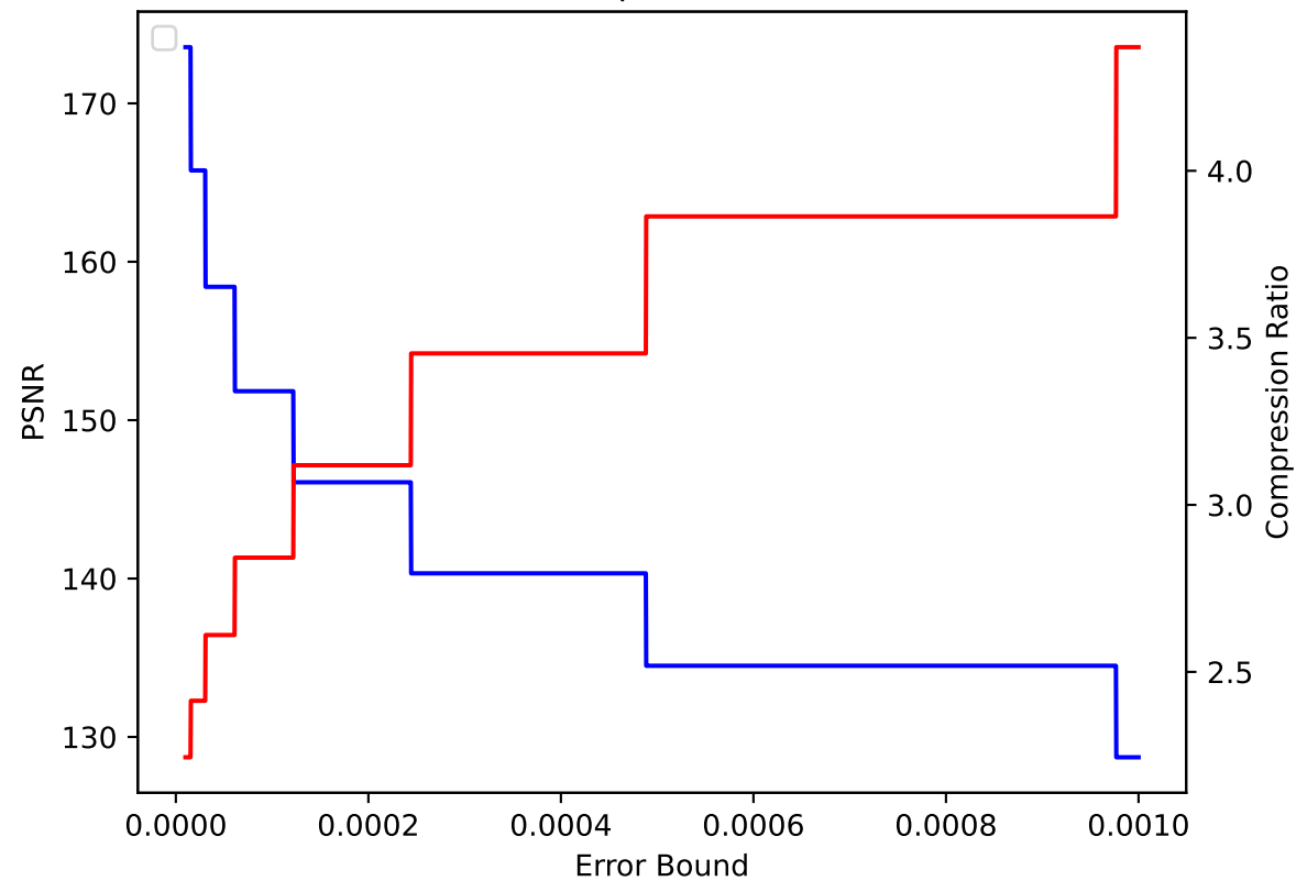
TC 01 pressio:abs
