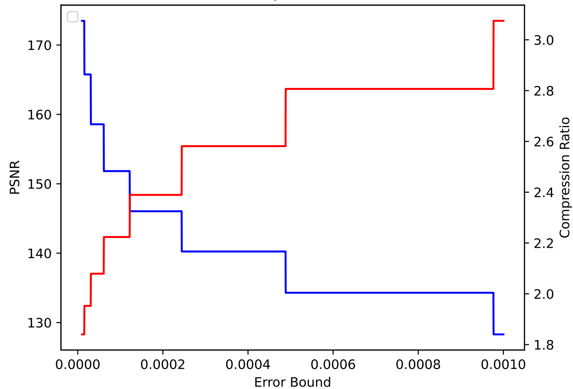
TC 34 pressio:abs
