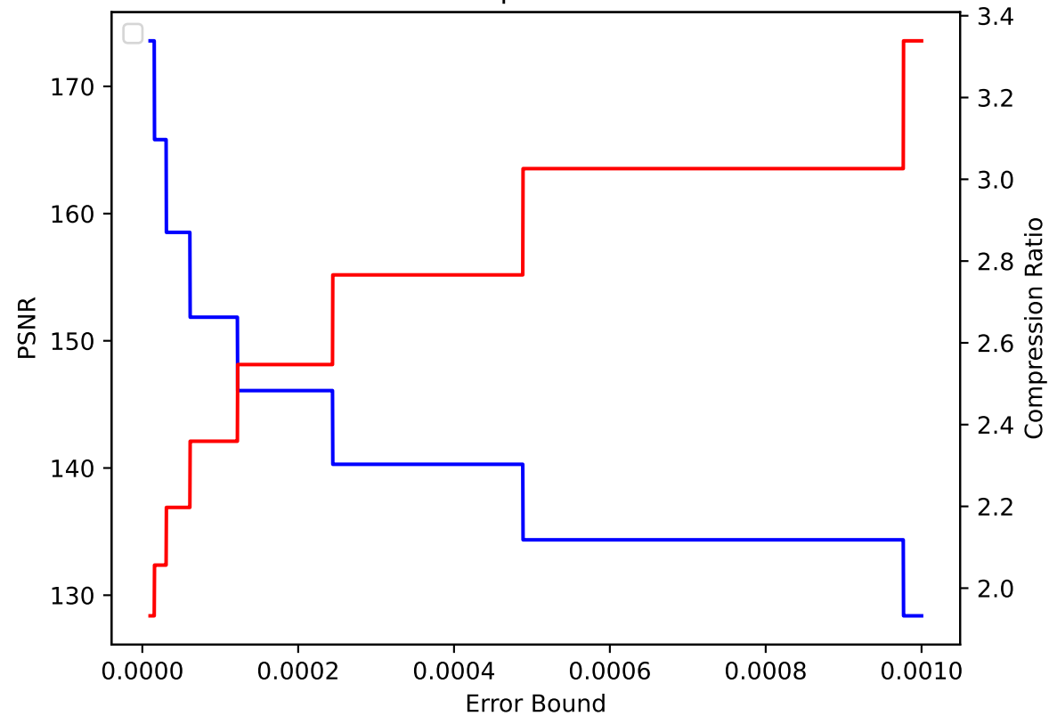
TC 09 pressio:abs
