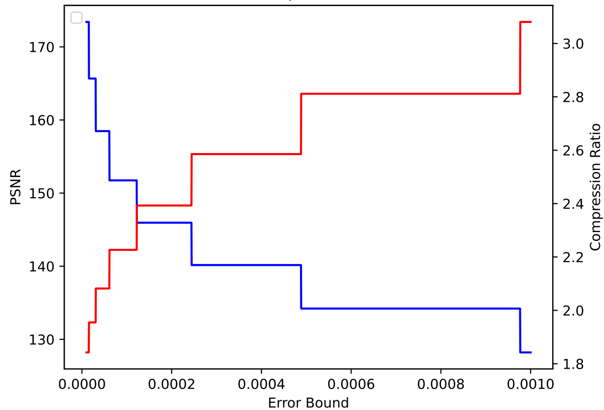
TC 32 pressio:abs
