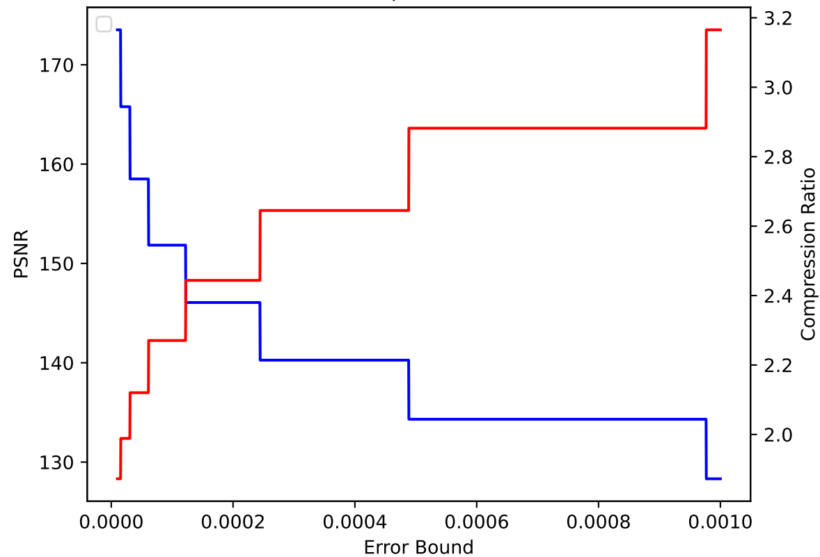
TC 16 pressio:abs
