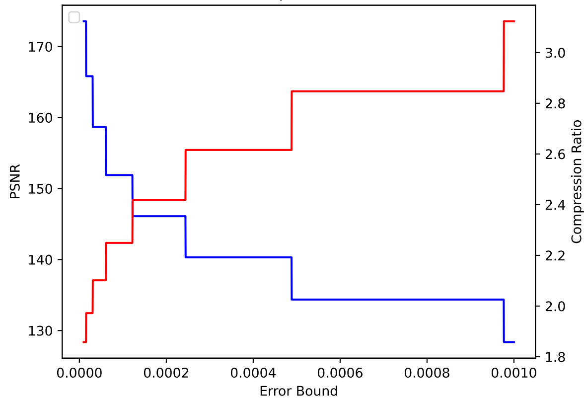
TC 42 pressio:abs
