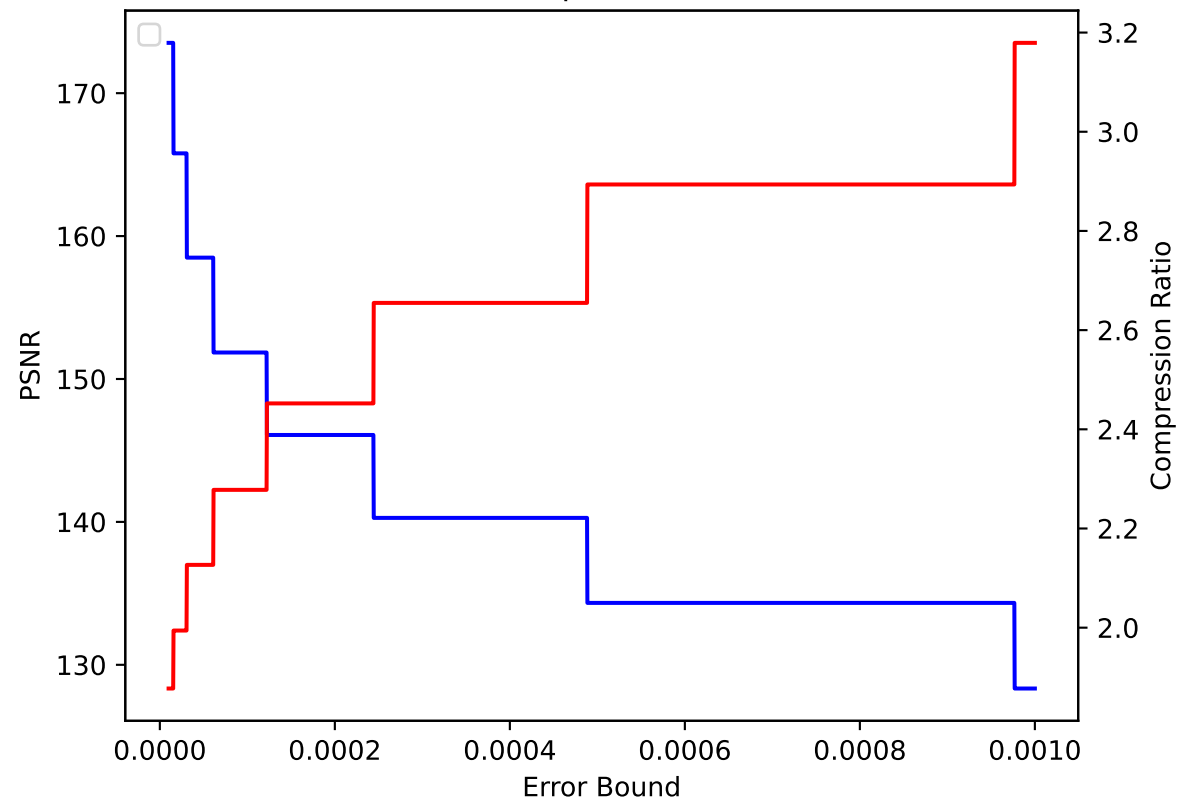
TC 14 pressio:abs
