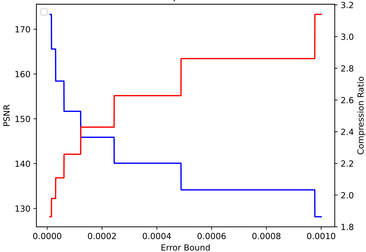
TC 48 pressio:abs
