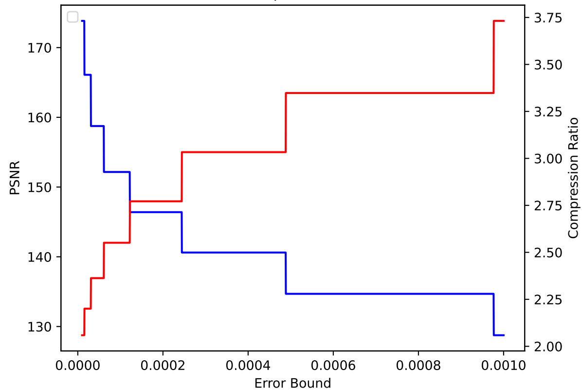
TC 05 pressio:abs
