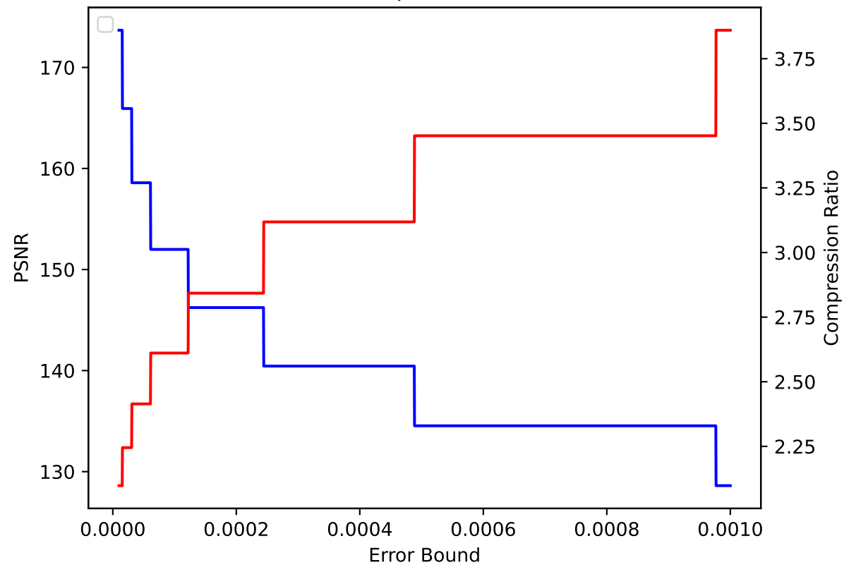
TC 04 pressio:abs
