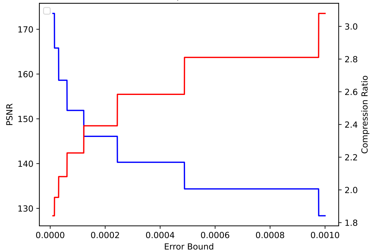
TC 33 pressio:abs
