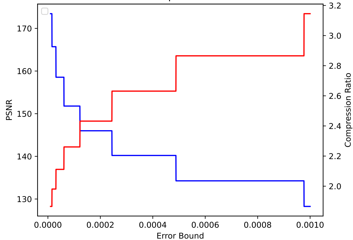
TC 45 pressio:abs
