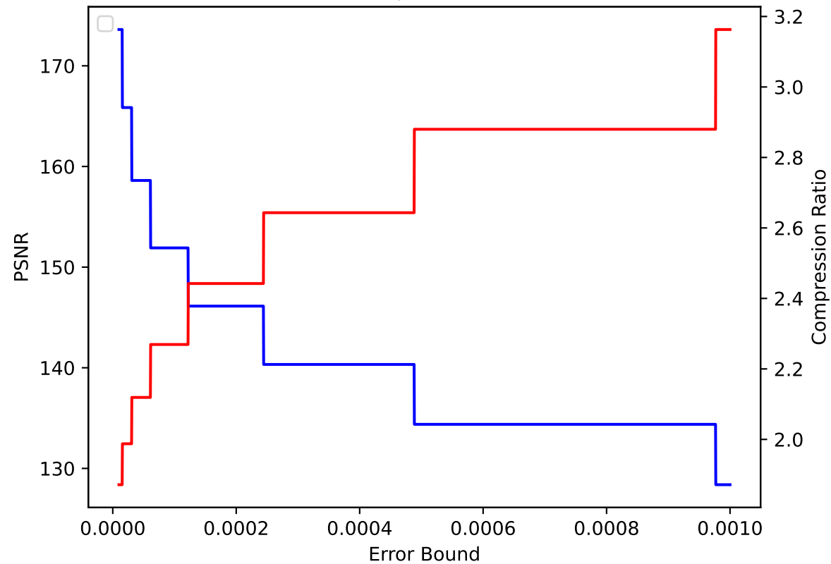
TC 19 pressio:abs
