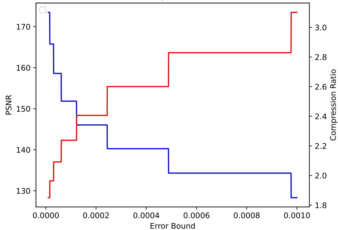
TC 39 pressio:abs
