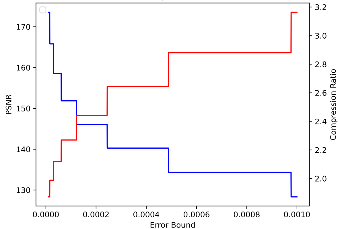
TC 17 pressio:abs
