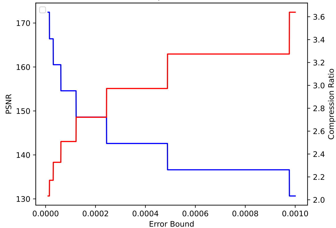
V 04 pressio:abs
