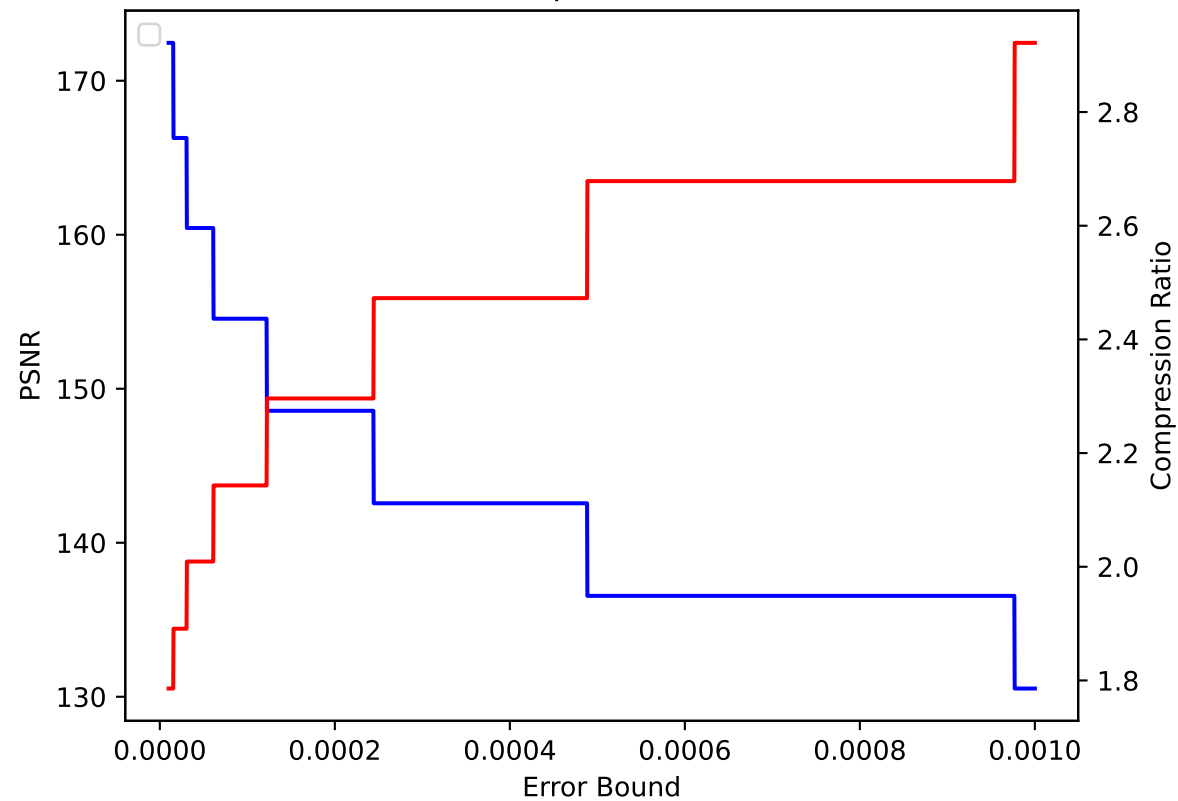
V 32 pressio:abs
