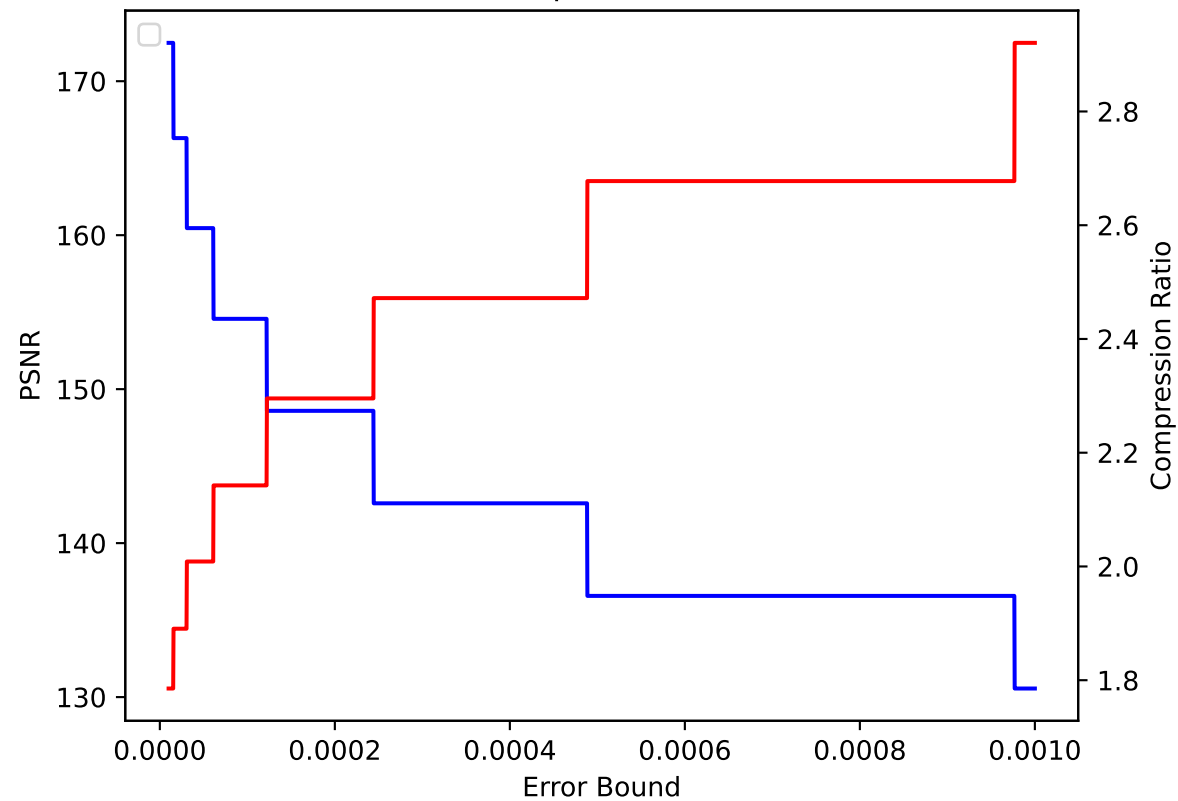
V 33 pressio:abs
