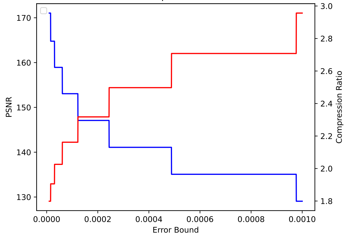
V 43 pressio:abs
