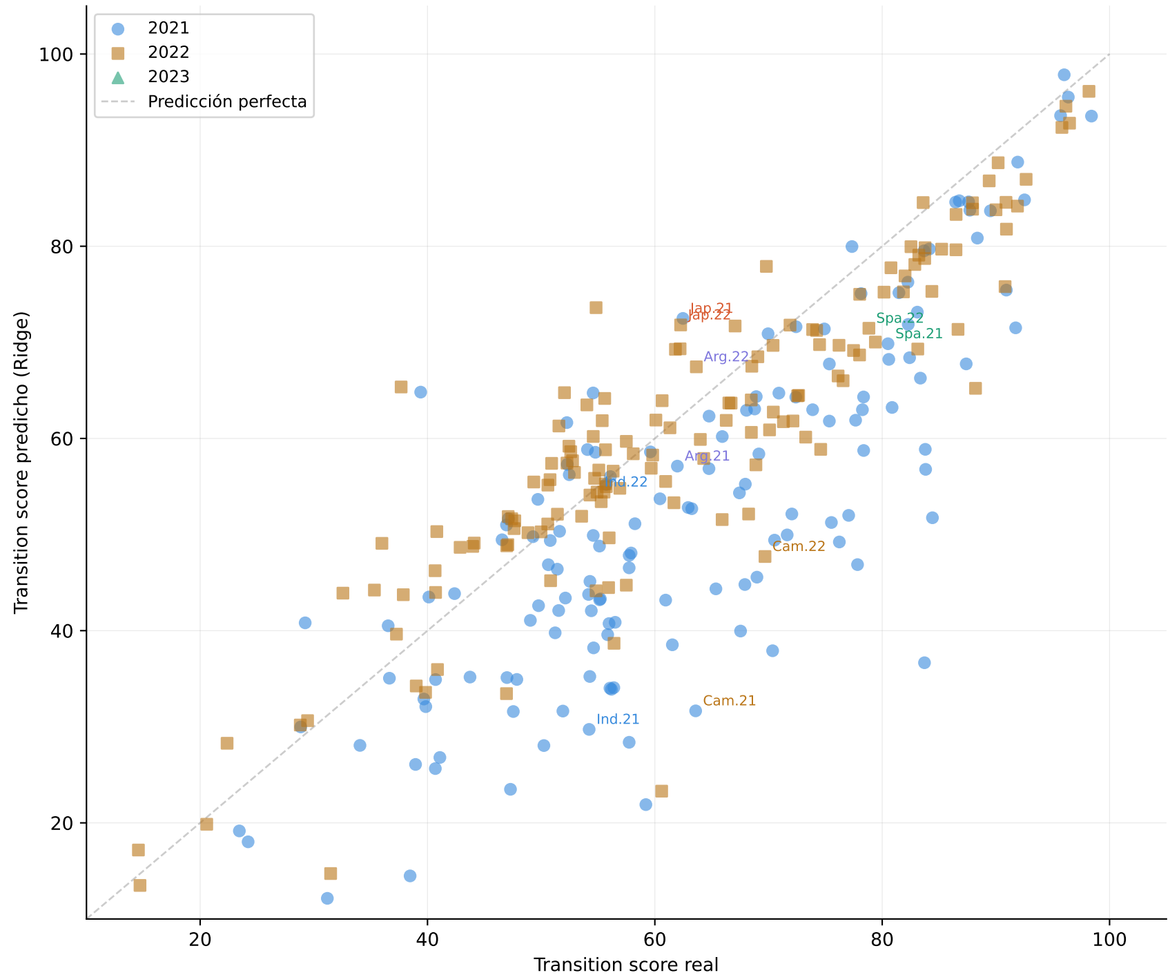
Predicho vs Real — países con datos completos MAE = 9.28 pts | n = 296 observaciones
