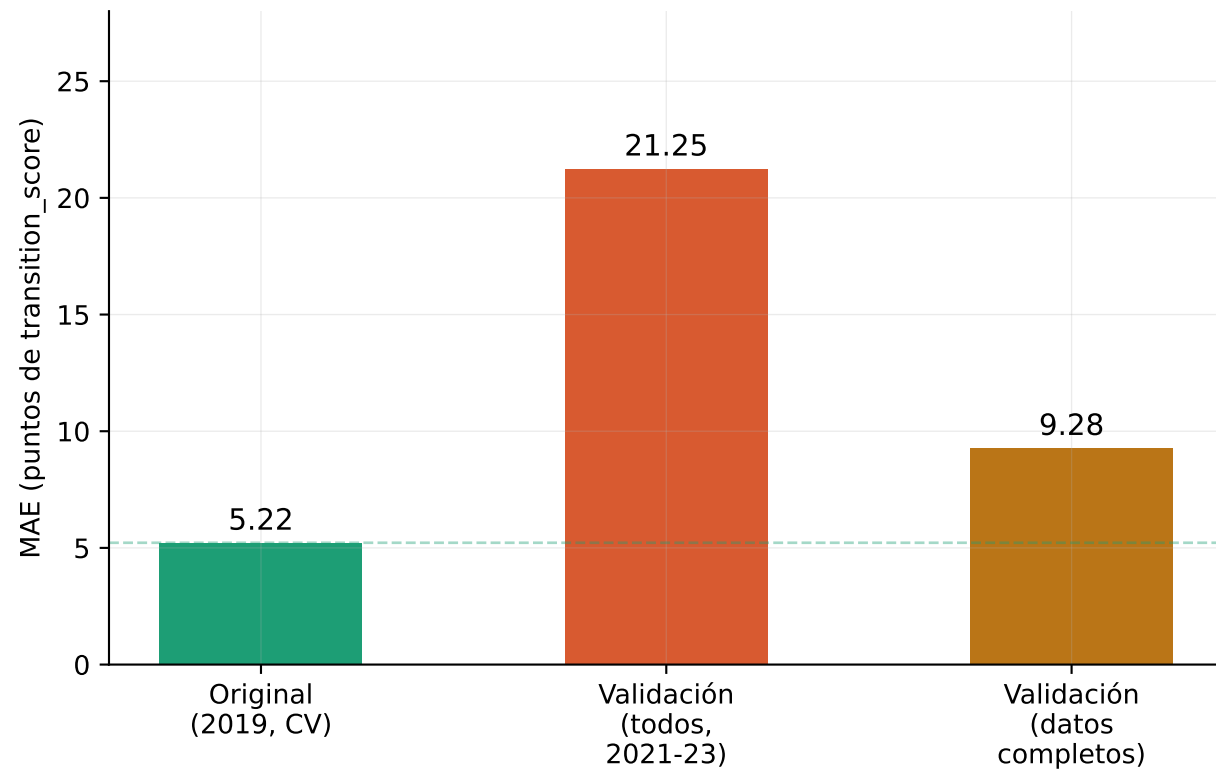
Error medio absoluto (MAE)
