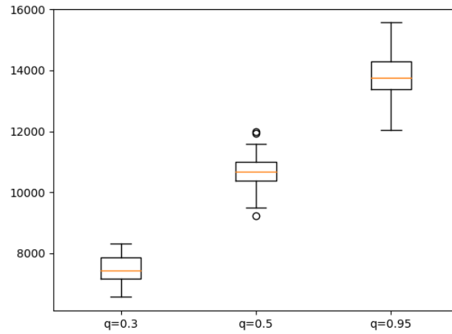
Abbildung 16: Cigar Vergleich q
