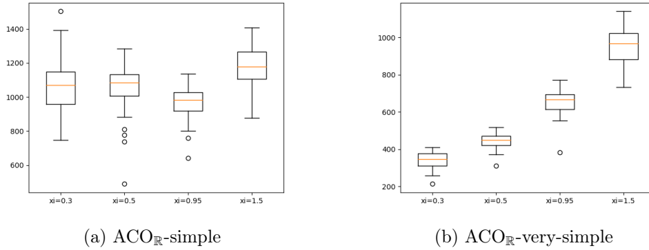
Abbildung 10: Ellipsoid Vergleich \xi
