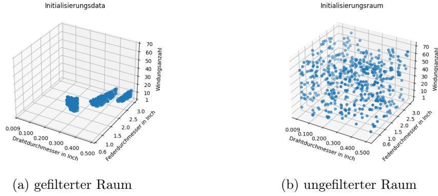
Abbildung 5: gefilterter und ungefilterter Suchraum für das CSD-Problem
