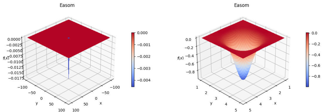
Abbildung 1: Easom-Testfunktion: Vergleich zwischen gesamtem Suchraum (links) und Umgebung um das Optimum (rechts)
