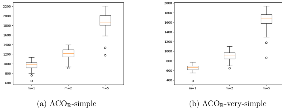
Abbildung 8: Ellipsoid Vergleich m
