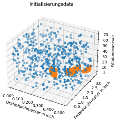
Abbildung 6: gefilterter und ungefilterter Raum
