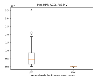
Abbildung 17: Verhältnis zwischen den benötigten Funktionsauswertungen für Vorfiltern, zusätzlichem Filtern und realen Iterationsschritten der Algorithmen für den Fall „exact-penalty“ und NSS-adapt, Teil 1
