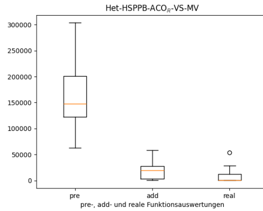
Abbildung 12: Verhältnis zwischen den benötigten Funktionsauswertungen für Vorfiltern, zusätzlichem Filtern und realen Iterationsschritten der Algorithmen für den Fall „exact-exact“ und NSS-f0, Teil 2
