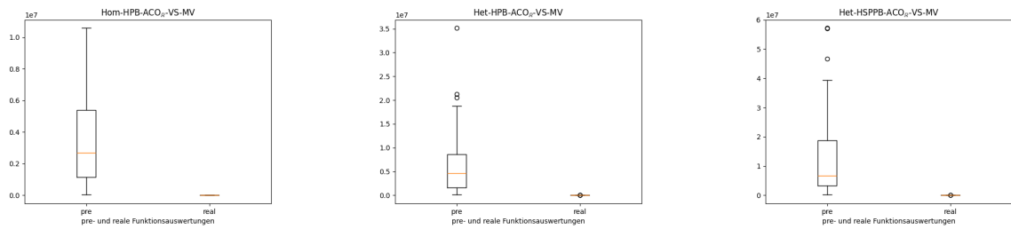
Abbildung 14: Verhältnis zwischen den benötigten Funktionsauswertungen für Vorfiltern, zusätzlichem Filtern und realen Iterationsschritten der Algorithmen für den Fall „exact-penalty“ und NSS-adapt
