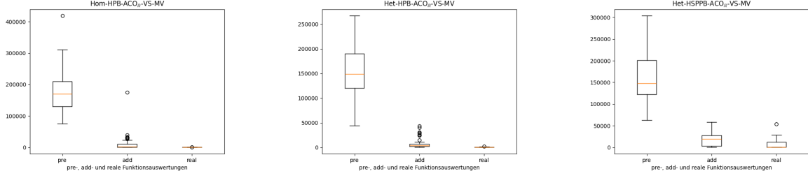
Abbildung 11: Verhältnis zwischen den benötigten Funktionsauswertungen für Vorfiltern, zusätzlichem Filtern und realen Iterationsschritten der Algorithmen für den Fall „exact-exact“ und NSS-f0
