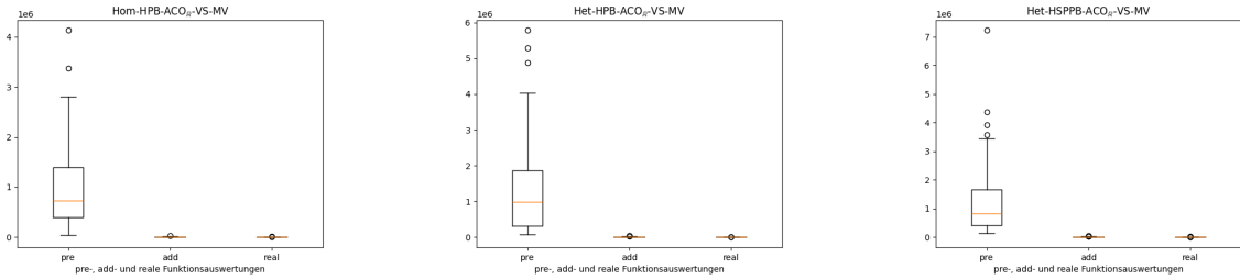
Abbildung 12: Verhältnis zwischen den benötigten Funktionsauswertungen für Vorfiltern, zusätzlichem Filtern und realen Iterationsschritten der Algorithmen für den Fall „exact-exact“ und NSS-adapt
