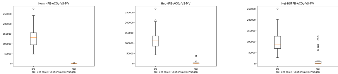
Abbildung 13: Verhältnis zwischen den benötigten Funktionsauswertungen für Vorfiltern, zusätzlichem Filtern und realen Iterationsschritten der Algorithmen für den Fall „exact-penalty“ und NSS-f0
